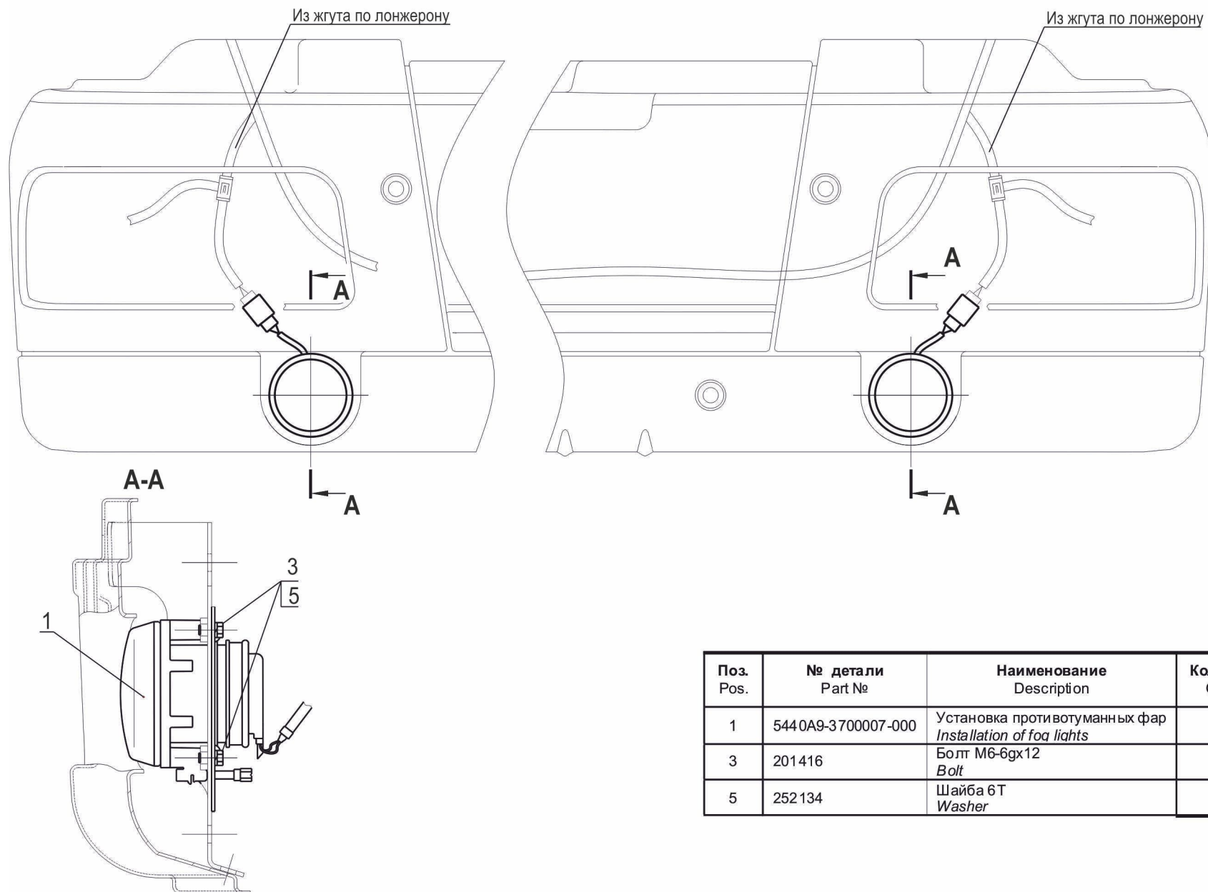
Рис.182 Установка противотуманных фар 643019-3700007 Fig. 182 Installation of fog lights 643019-3700007
