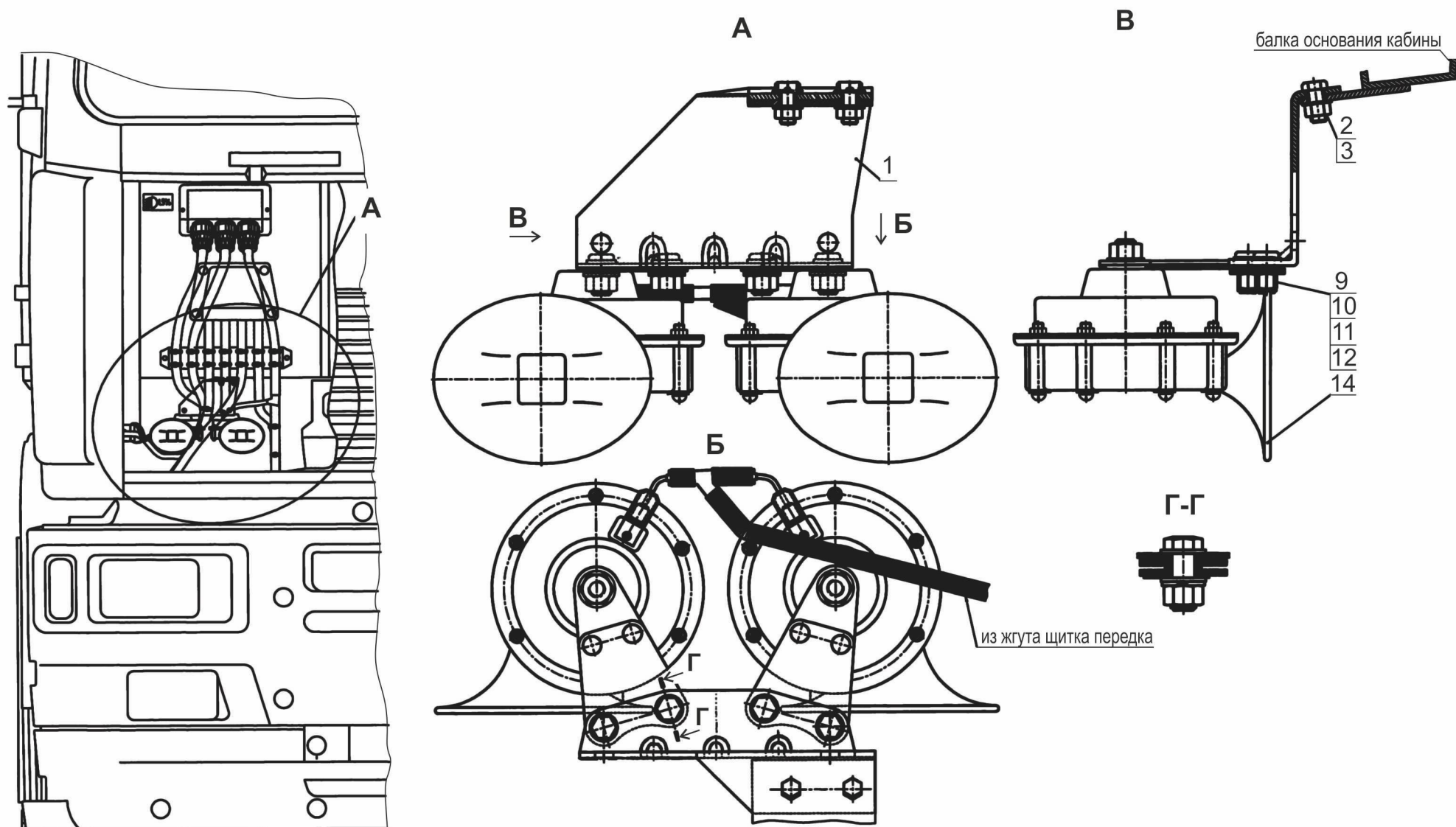
Рис. 193 Установка звуковых сигналов 544008-3700024-700 Fig.193 Installation of audible signals 544008-3700024-700
