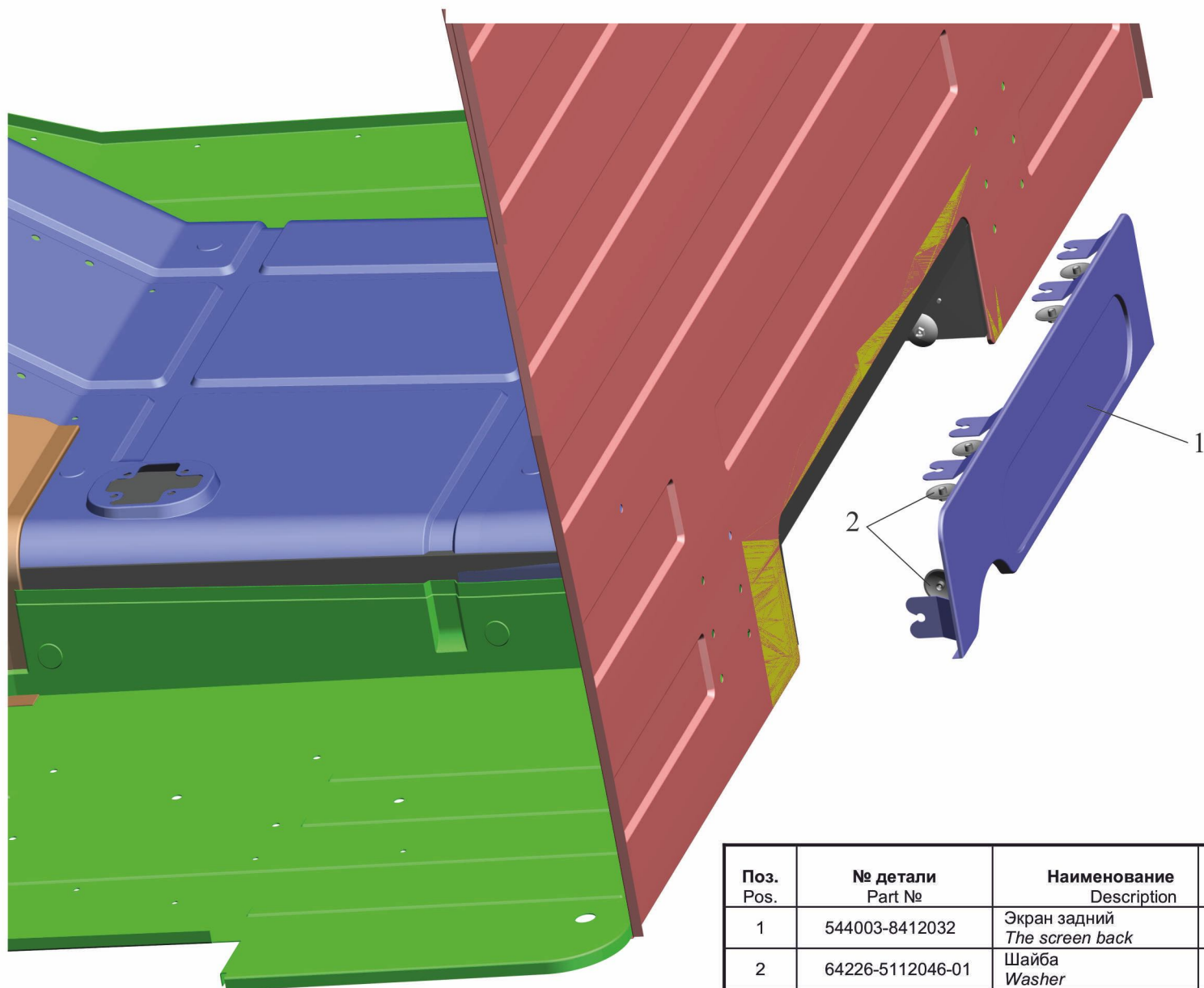
Рис.305 Установка экранов 544003-8400026 Fig. 305 Installation of screens 544003-8400026
