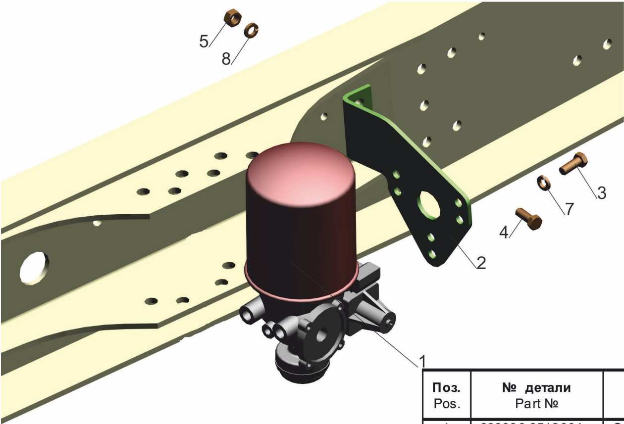
Рис. 177 Крепление осушителя воздуха 650107-3536004 Fig. 177 Installation of air dehumidifier 650107-3536004
