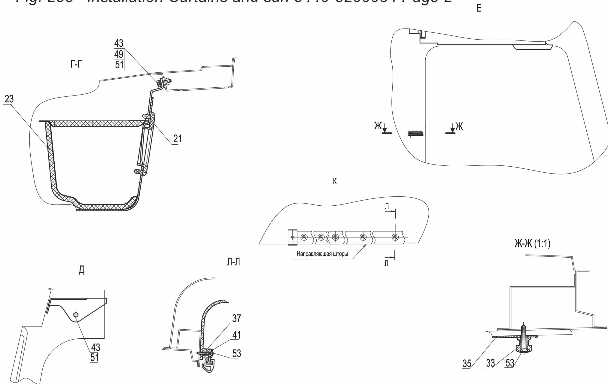
Рис. 258 Установка полки, штор 5440-8200034 Лист 2 Fig. 258 Installation Curtains and sun 5440-8200034 Page 2
