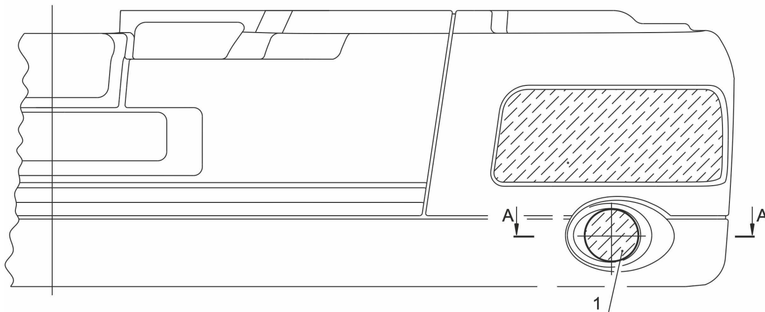
Рис. 101 Установка противотуманной фары 447131-3700007-010 Fig. 101 Installation of fog light 447131-3700007-010
