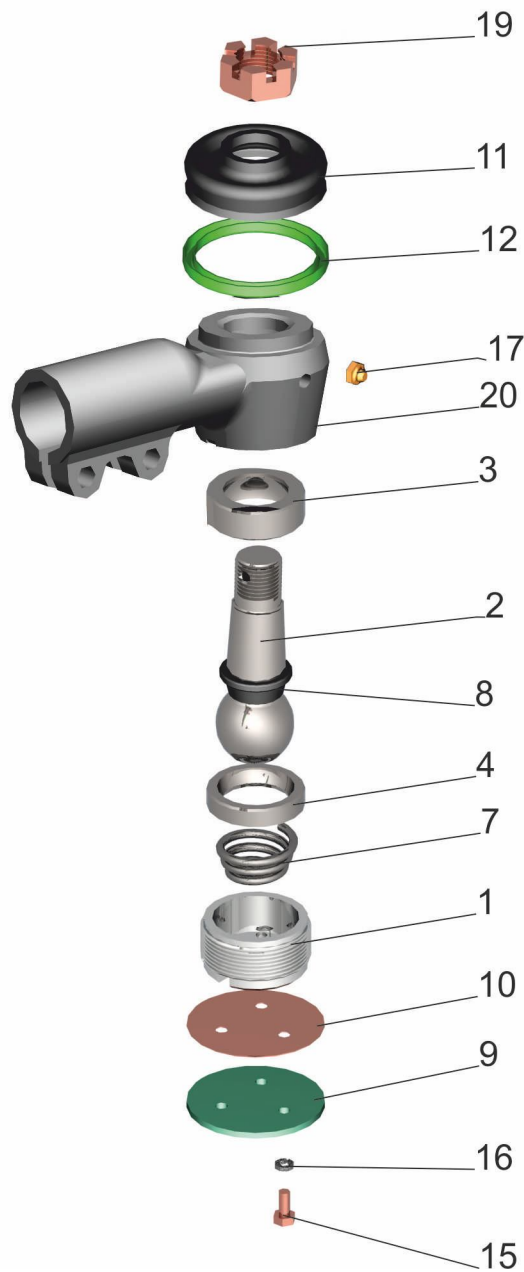
Рис.129 Наконечник 6422-3003057 Fig.129 Nozzle 6422-3003057
