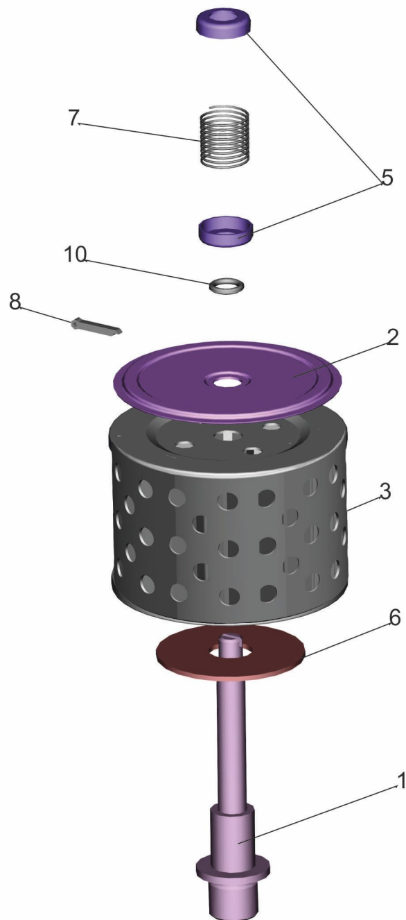
Рис. 158 Фильтр с клапаном 5336-3410051 Fig. 158 Filter with the valve 5336-3410051
