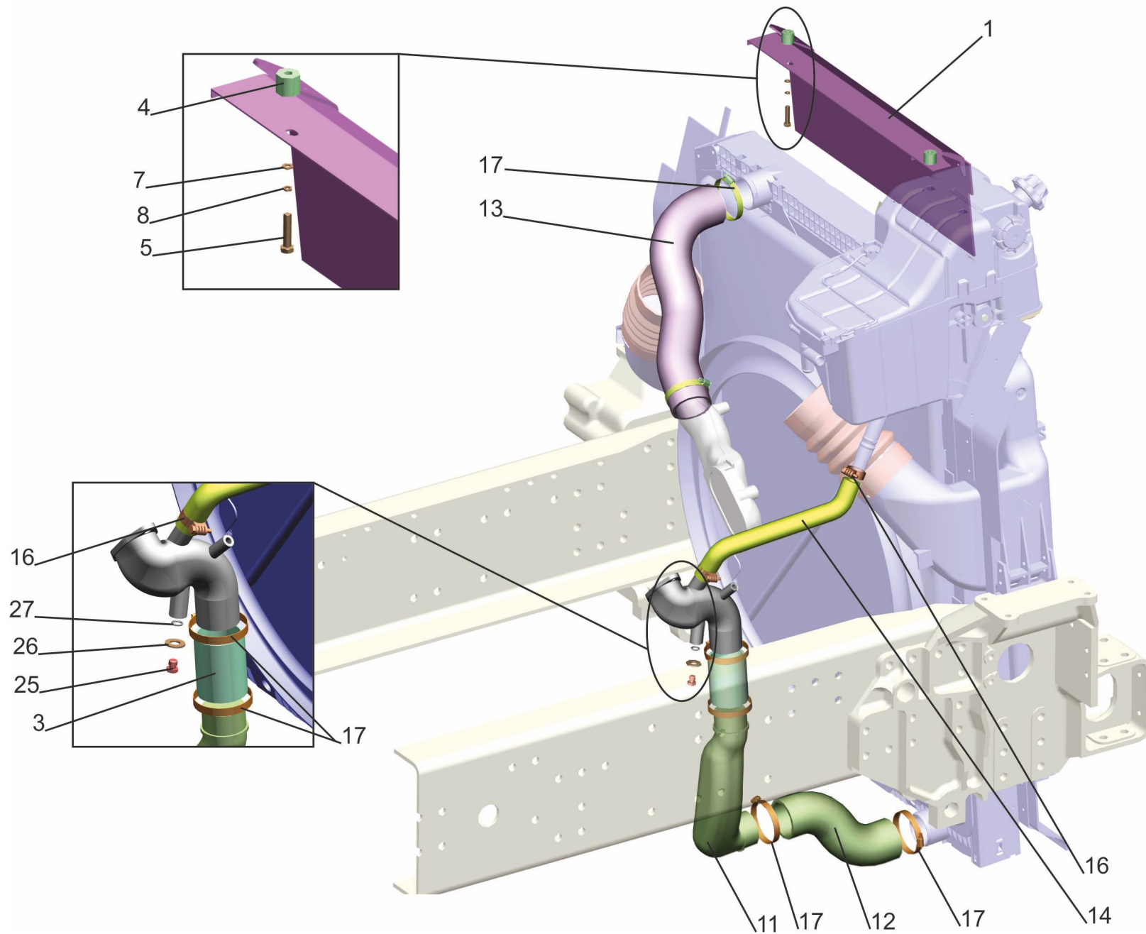
Рис. 26 Установка системы охлаждения 544019-1300005-010 Fig. 26 Installation of cooling system set 544019-1300005-010
