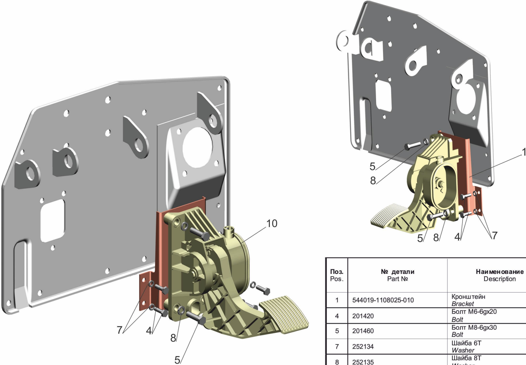
Рис. 22 Установка педали управления двигателем 544019-1108002-010 Fig. 22 Installation of the shift pedal by the engine 544019-1108002-010
