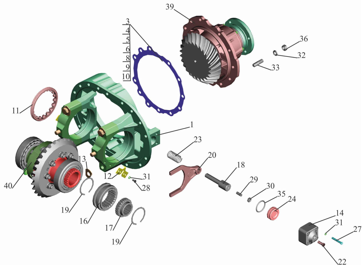
Рис. 67 Редуктор Fig. 67 Reducer gear
