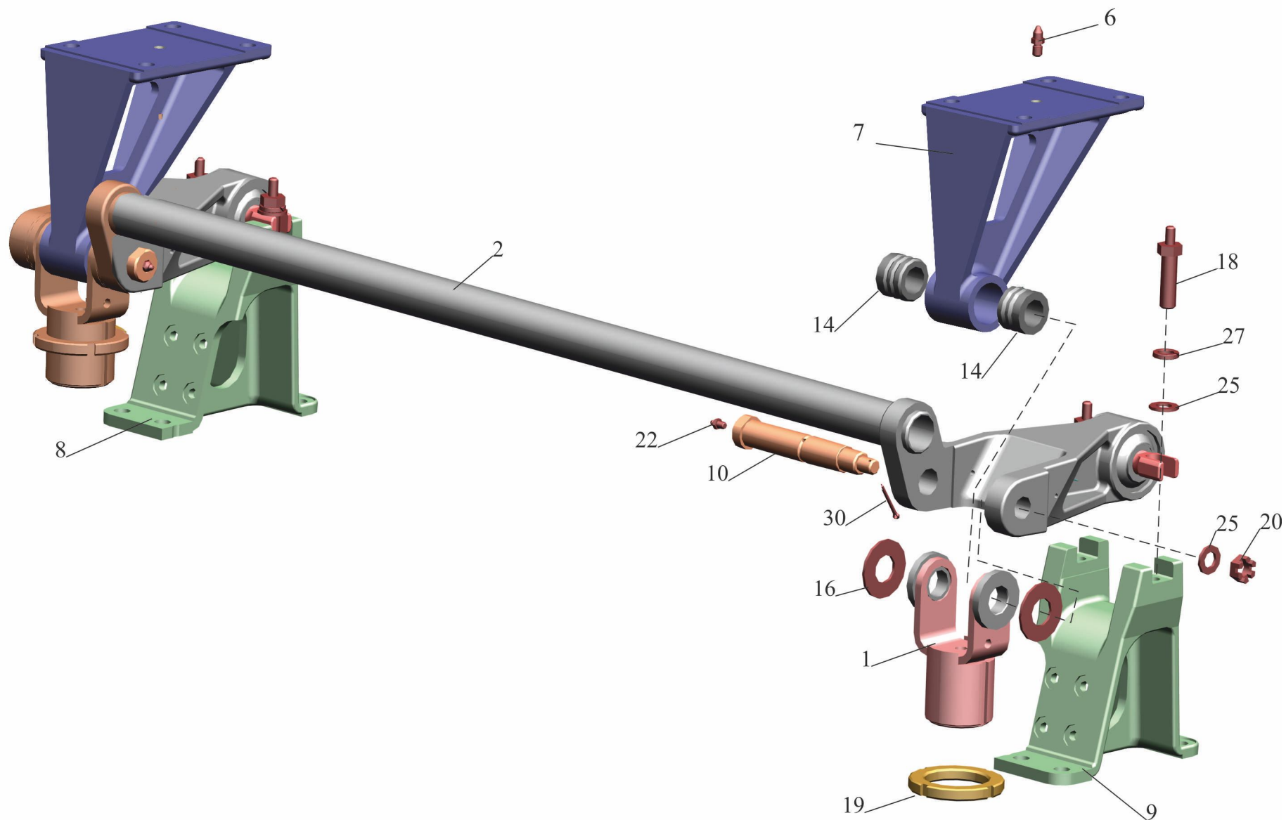
Рис. 222 Переднее подрессоривание 643019-5001702-010 Fig. 222 Front springing 643019-5001702-010
