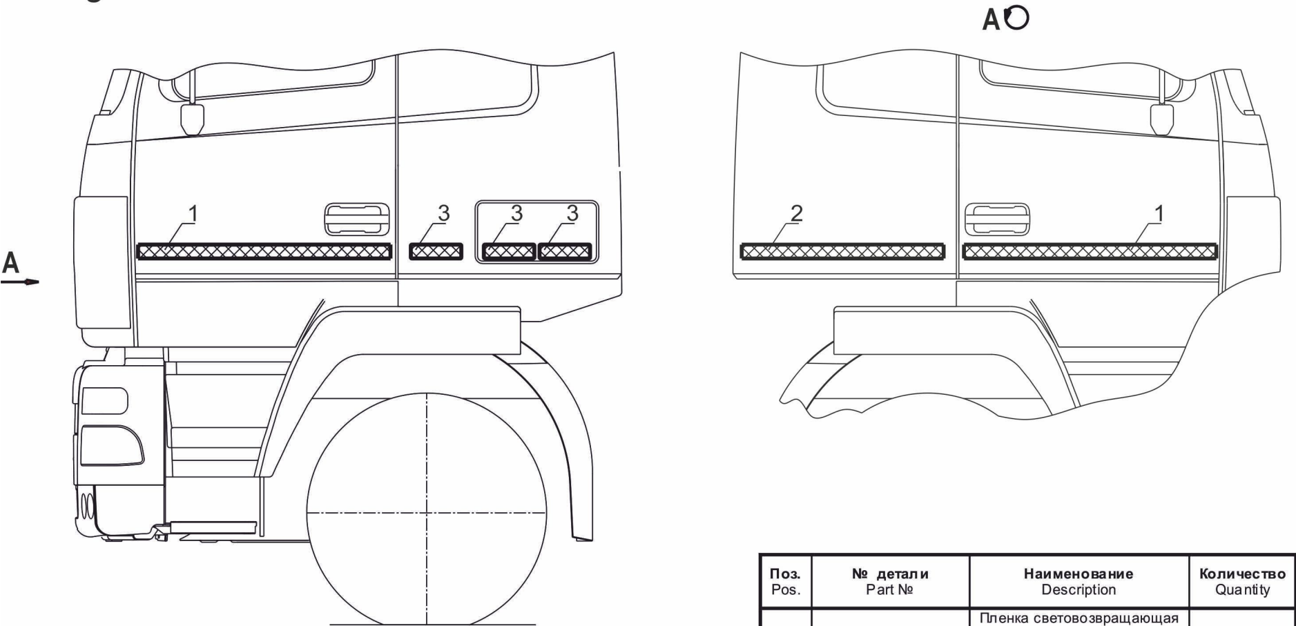
Рис. 212 Установка светоотражающей маркировки 6430-8200002 Fig.212 Installation of switches 6430-8200002
