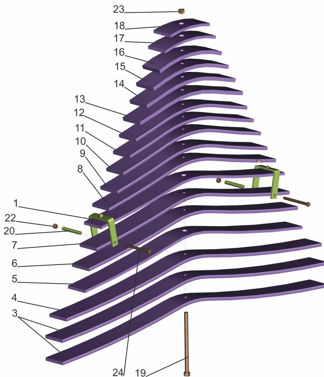
Рис. 118 Рессора задняя 5516-2912012 Fig. 118 Back leaf spring 5516-2912012
