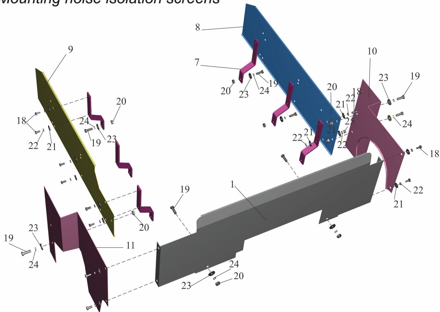
Рис.13 Установка шумоизоляционных экранов 544019-1061003-006 Fig.13 Mounting noise isolation screens
