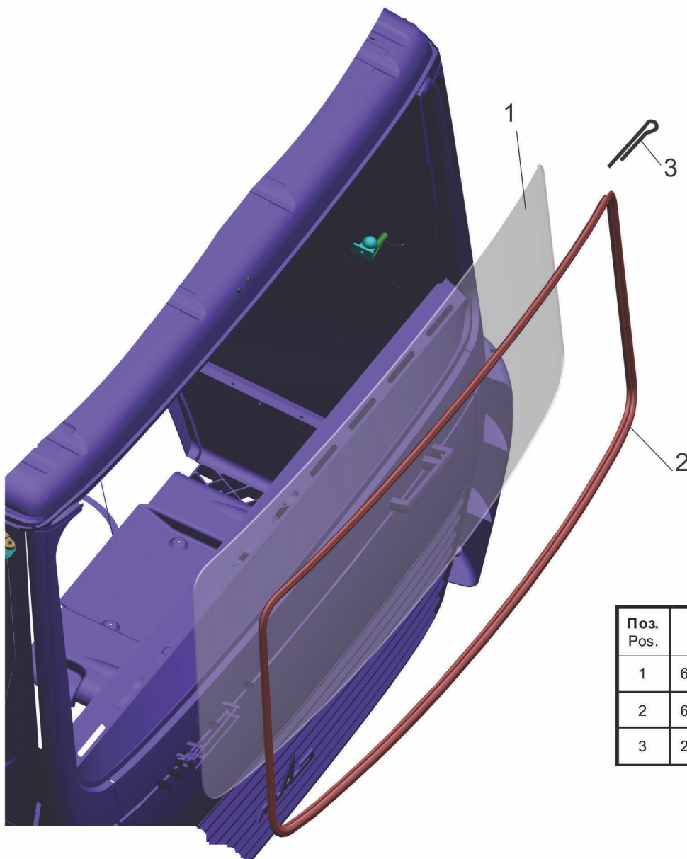
Рис. 236 Установки стекла 6430-5200010 Fig. 236 Installation of a glass 6430-5200010
