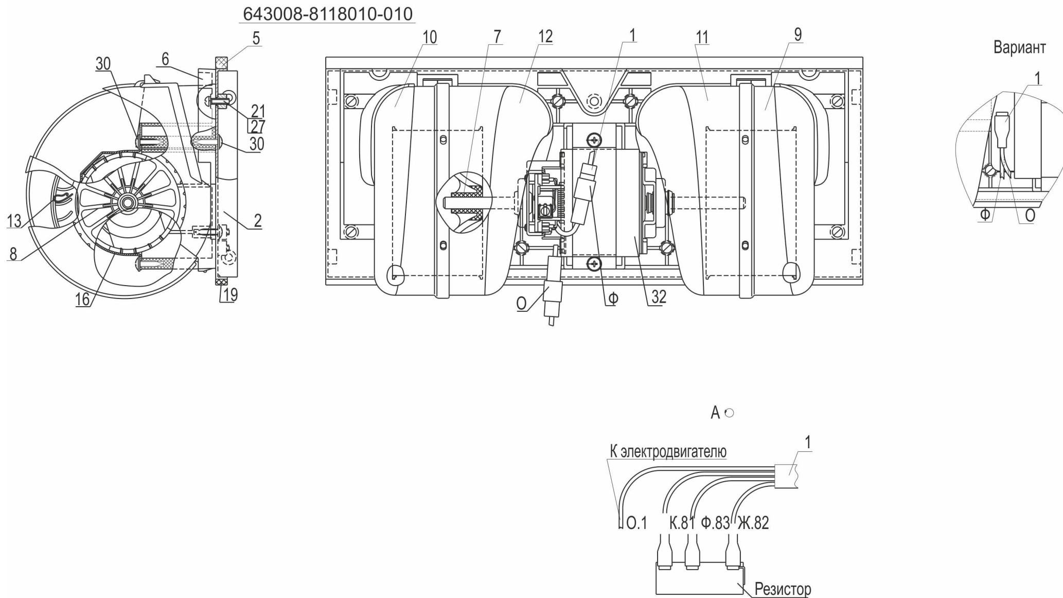
Рис. 284 Блок вентиляторный 643008-8118010-010, (-030) Fig. 284 Fan unit 643008-8118010-010, (-030)
