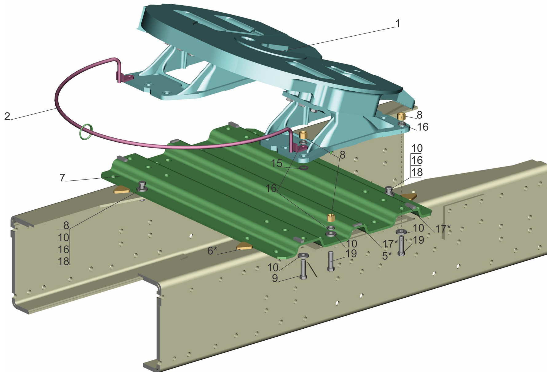
Рис. 94 Установка седельного устройства Fig. 94 Installation of coupling device
