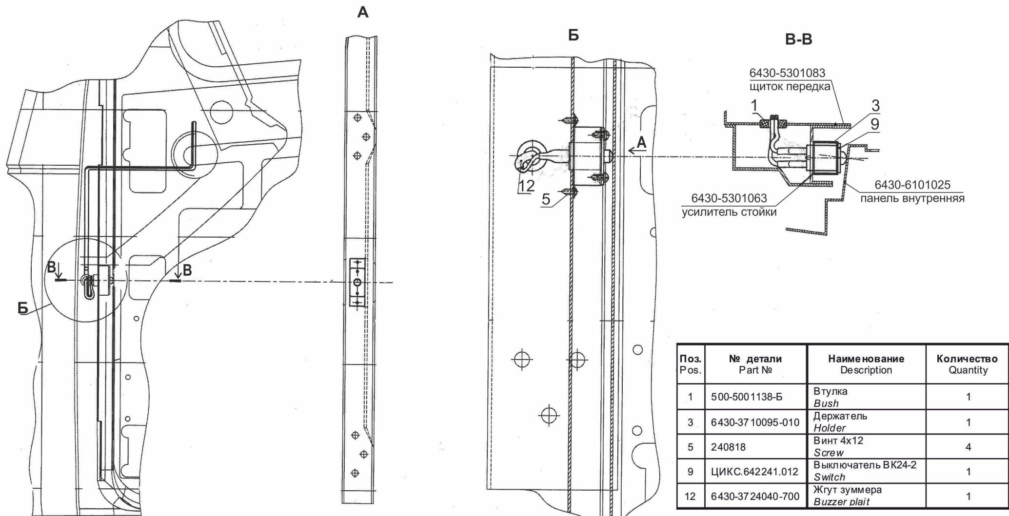
Рис. 195 Установка датчика открытой двери 6430-3700218-710 Fig.195 Installation of the gauge of an open door 6430-3700218-710
