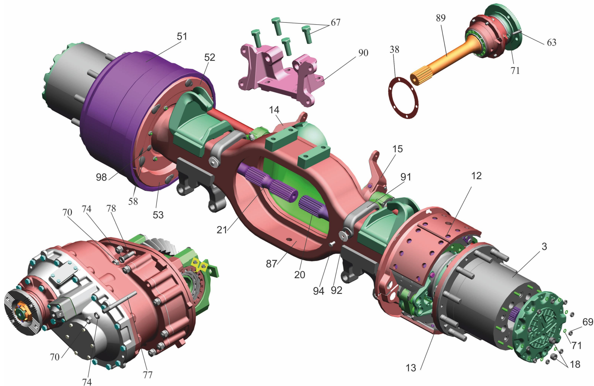
Рис.77 Мост средний Лист 1 Fig.77 Intermediate axle Page 1
