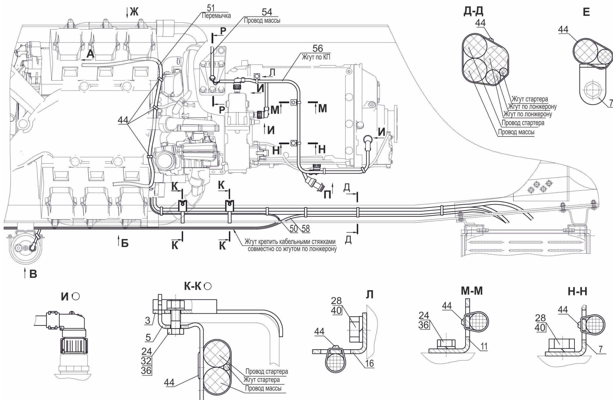
Рис.199 Установка электрооборудования на двигателе 544019-3700098 (лист 1) Fig. 199 Electric equipment installation on the engine 544019-3700098 (page 1)
