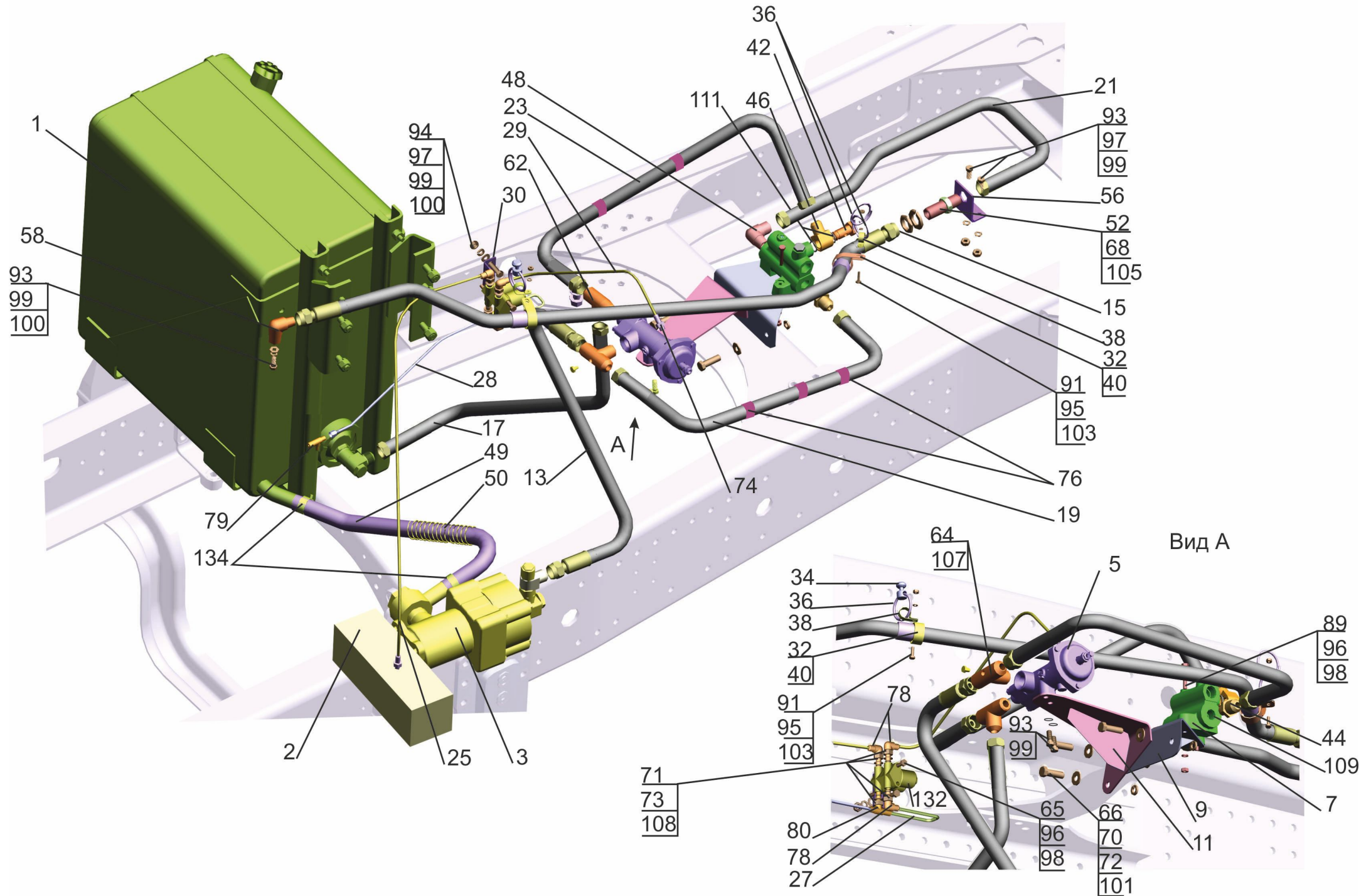
Рис.311 Установка гидрооборудования 643019-8600005-069 Fig.311 Installation of hydroequipment 643019-8600005-069
