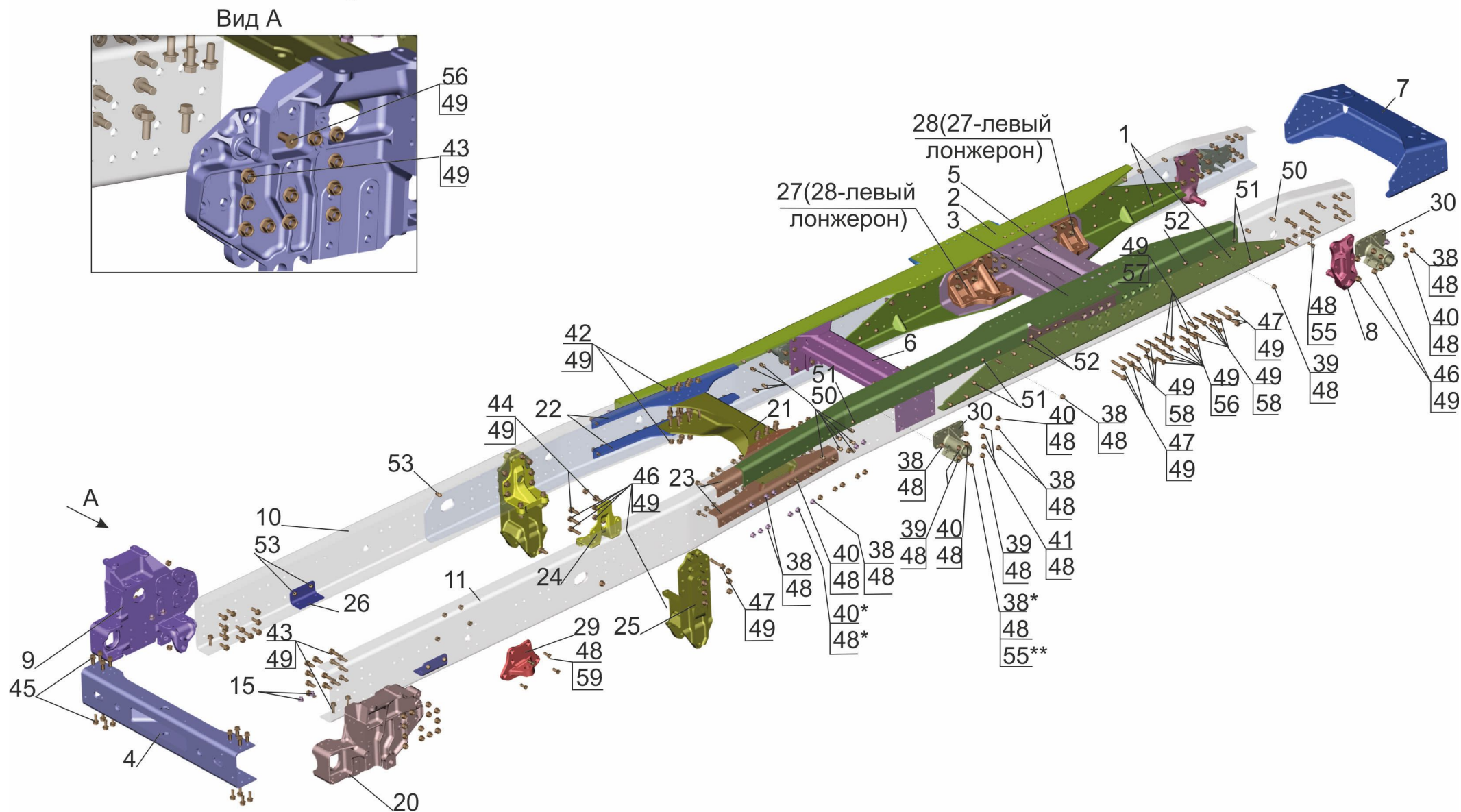
Рис.104 Рама 643018-2801002-010. Fig.104 Frame 643018-2801002-010.
