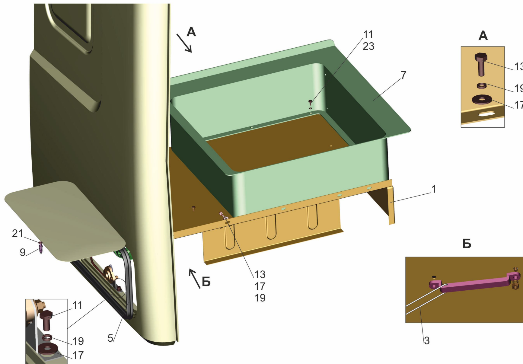
Рис. 233 Установка инструментального ящика 6430-5000115-020 Fig. 233 Installation of a tool box 6430-5000115-020
