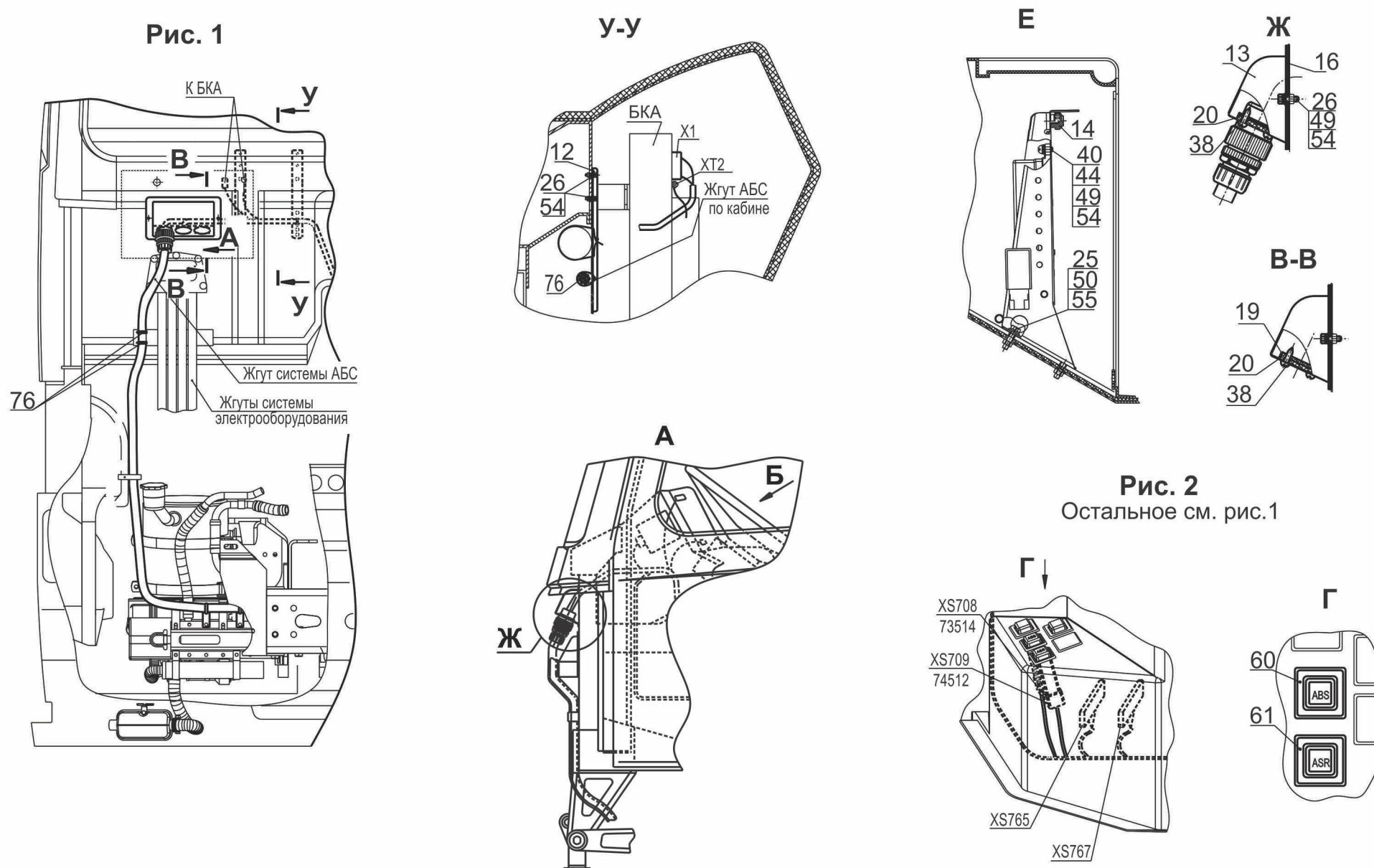
Рис. 215 Установка электрооборудования АБС по кабине 5440Е9-3700120 (лист 2) Fig. 215 Setting electrical equipment ABS on cabin 5440E9-3700120 (page 2)
