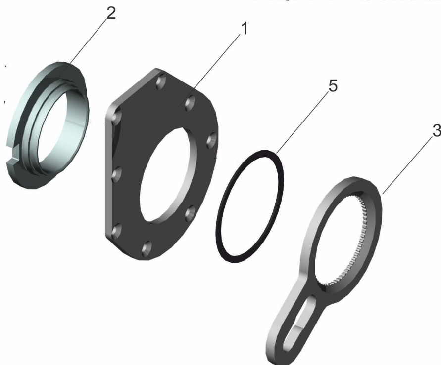
Рис. 74 Привод управляющий 64226-3501166 Fig. 74 Control drive 64226-3501166
