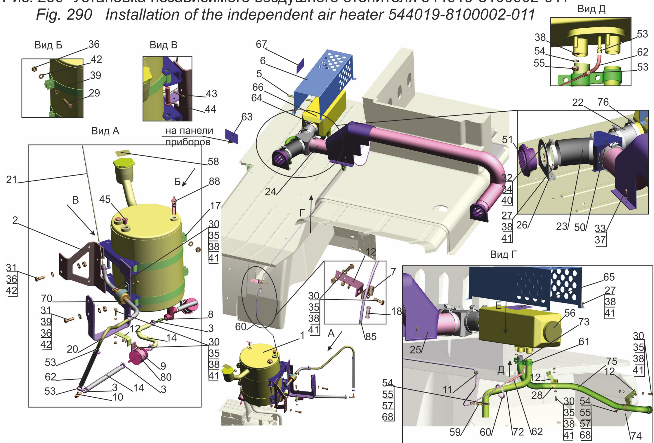
Рис. 290 Установка независимого воздушного отопителя 544019-8100002-011
