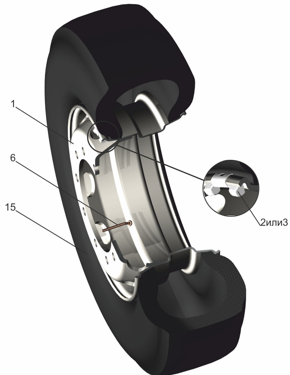
Рис. 140 Колесо и шина Fig. 140 Wheel and trunk
