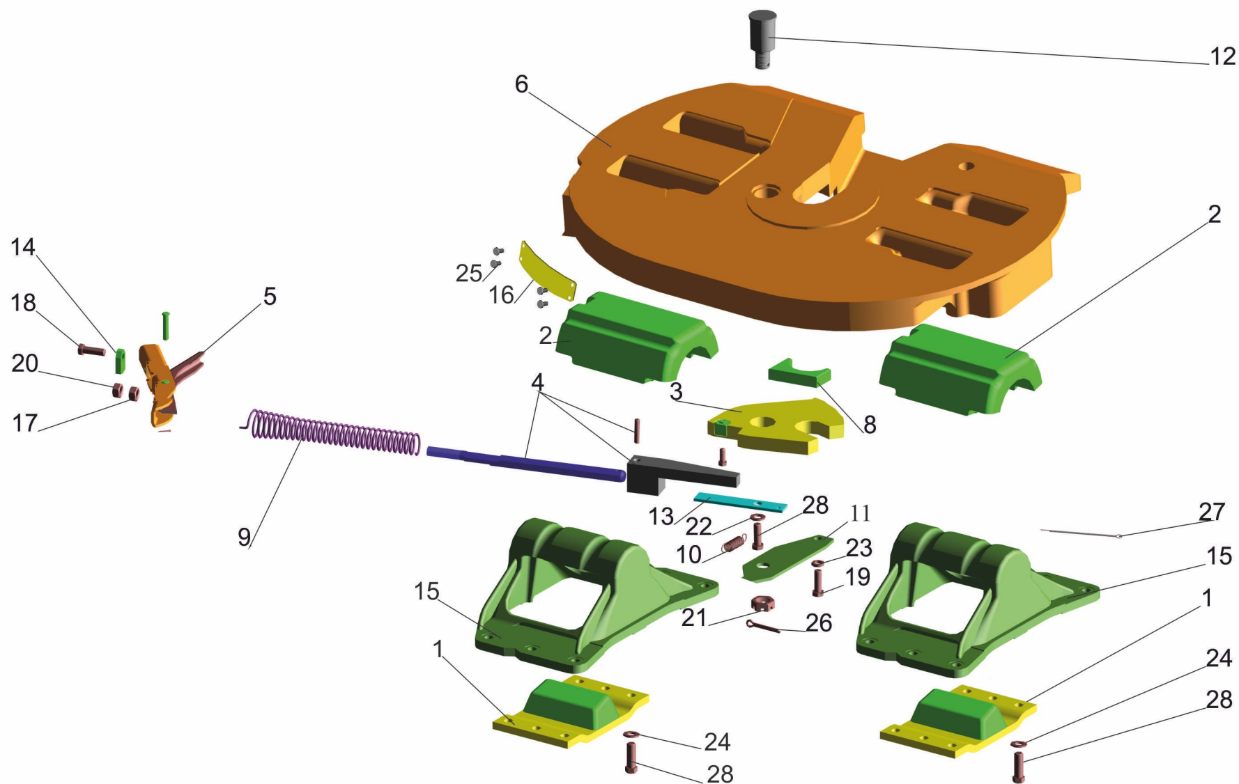
Рис. 96 Седельно-сцепное устройство 64221-2702010-01 Fig. 96 Coupling device 64221-2702010-01
