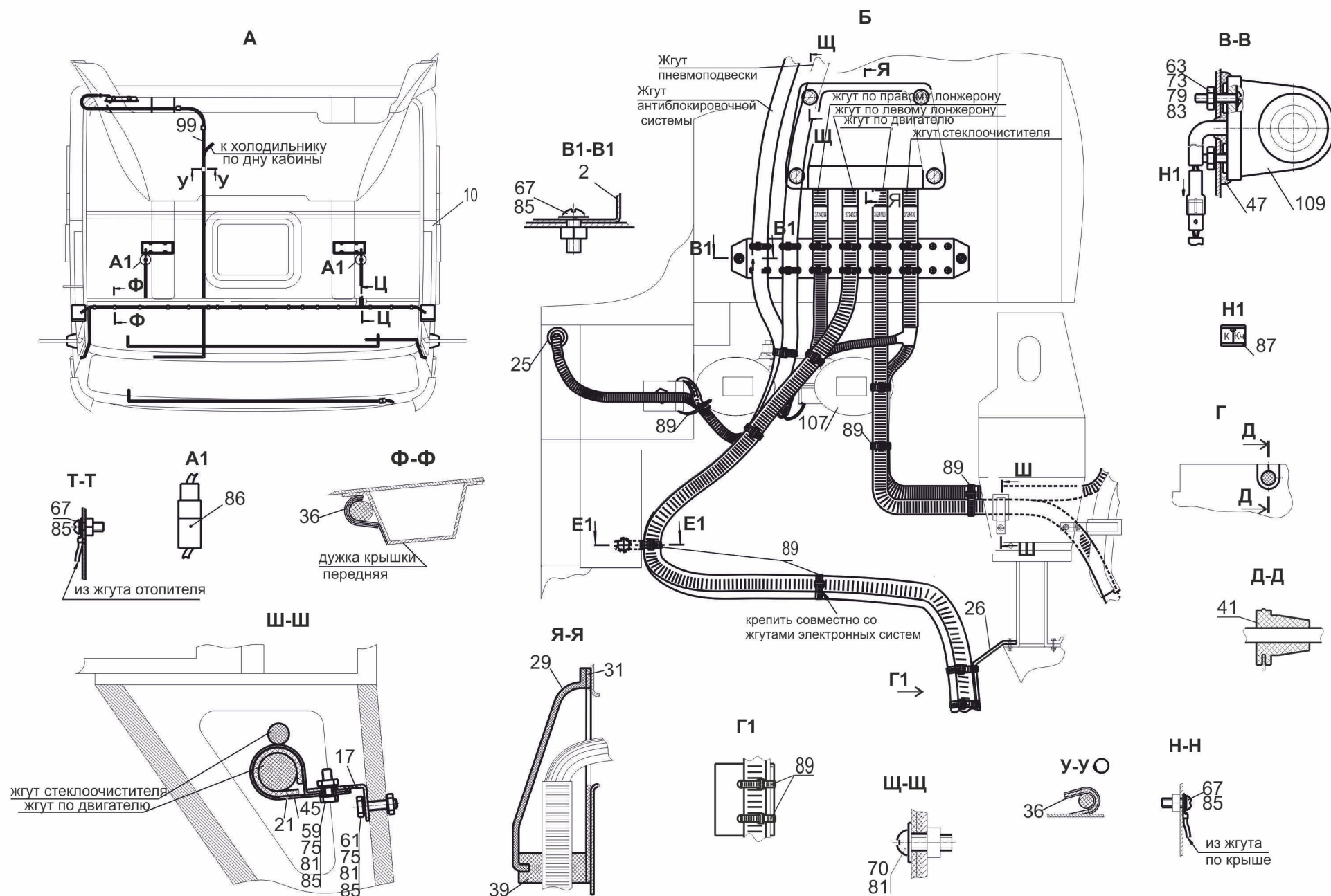
Рис.189 Установка электрооборудования в кабине 5340А5-3700076 (лист 2) Fig.189 Installation of an electrical equipment in a cabin 5340А5-3700076 (page2)
