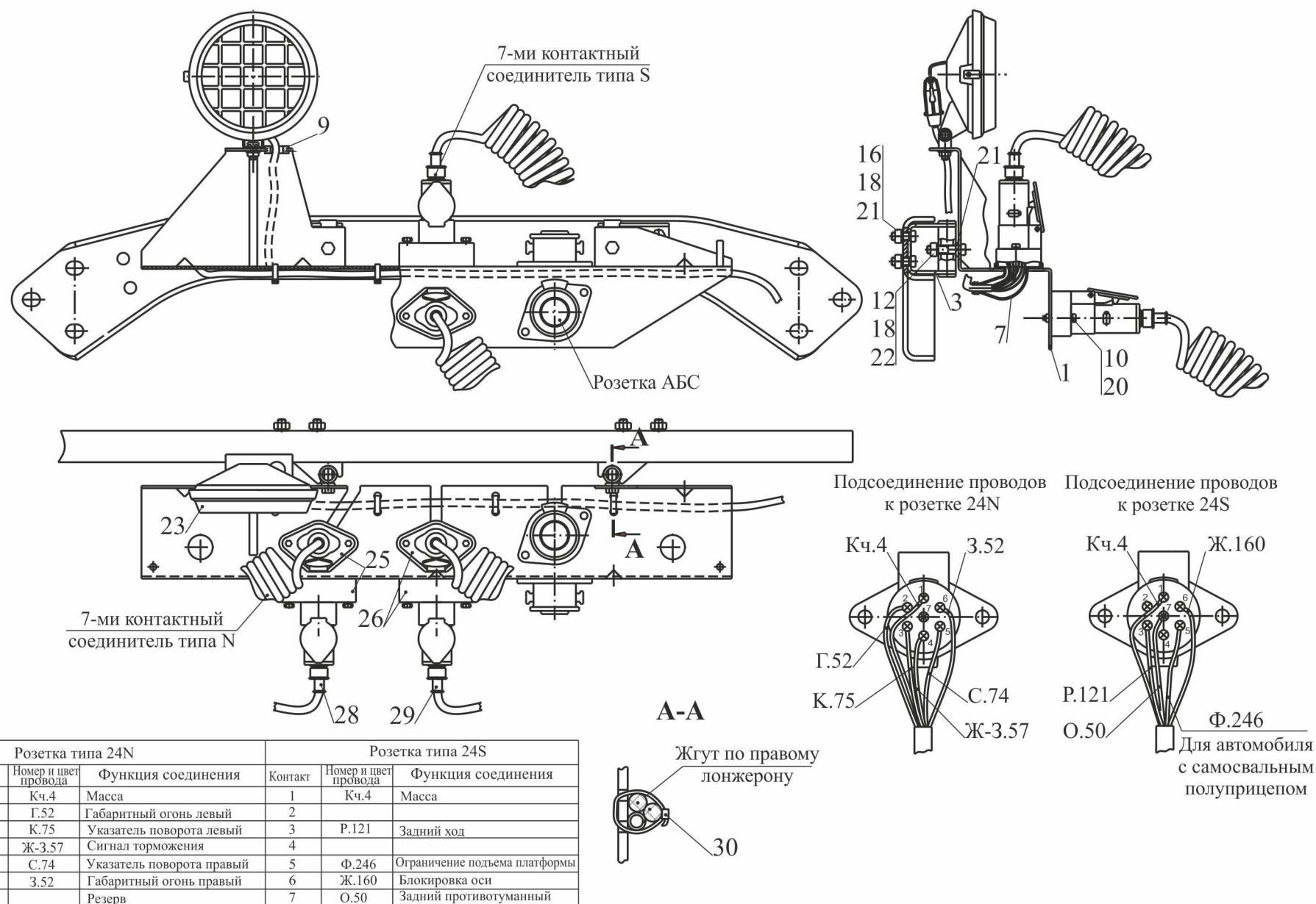
Рис. 187 Установка штепсельных розеток 544019-3700015 Fig. 187 Installation of plug receptacles 544019-3700015
