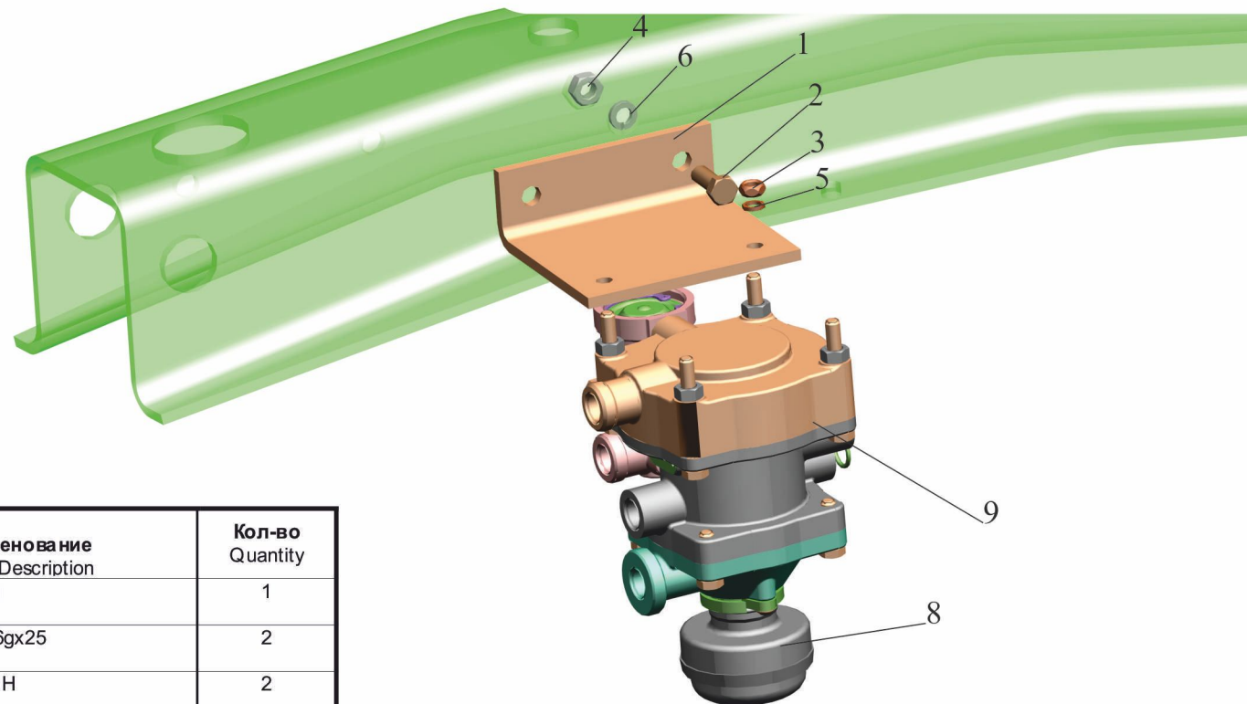
Рис. 176 Установка клапана управления тормозами прицепа 54401-3522005 Fig. 176 Installation of trailer brake control valve 54401-3522005
