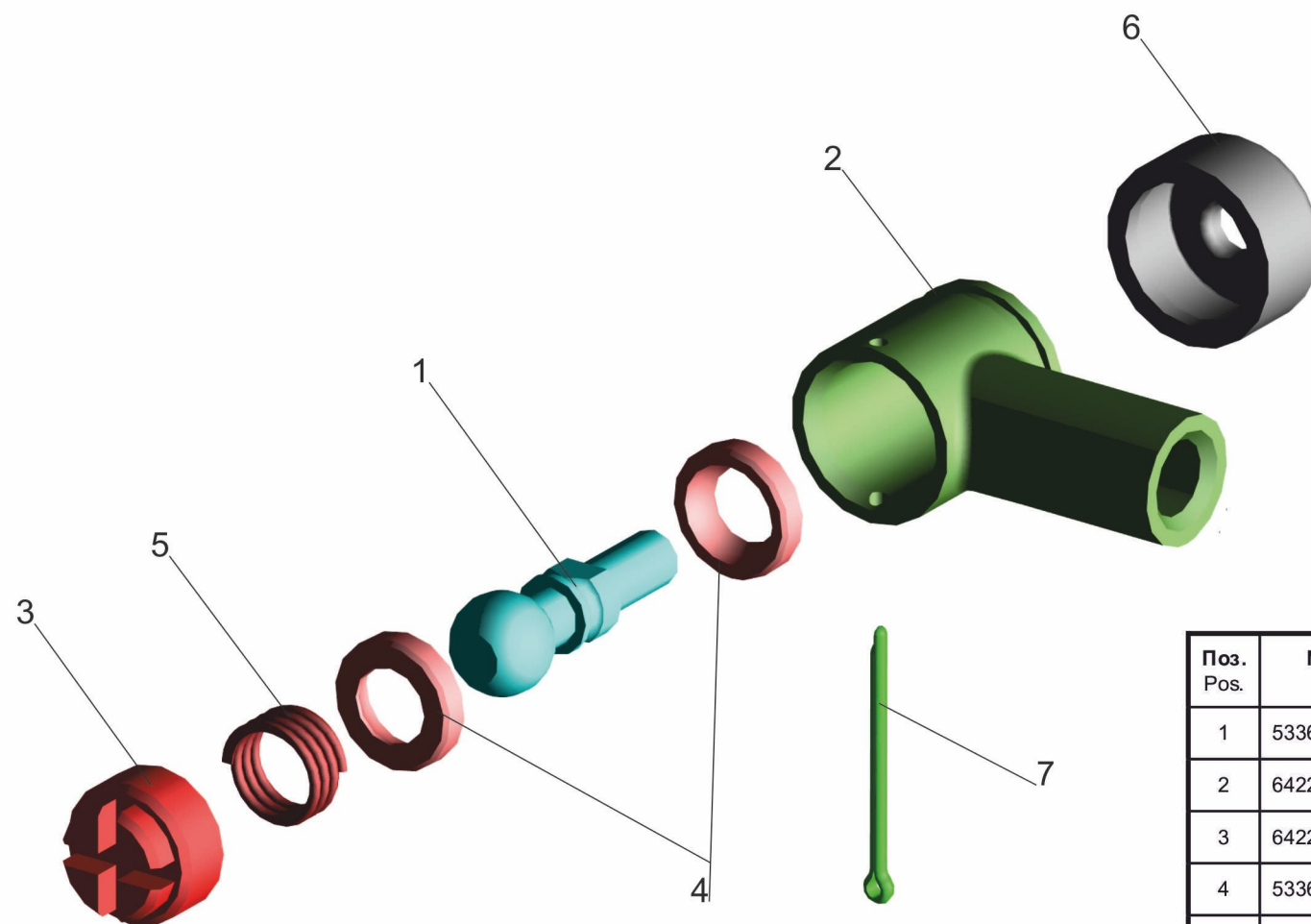
Рис. 52 Наконечник 6422-1703250 Fig. 52 Nozzle 6422-1703250
