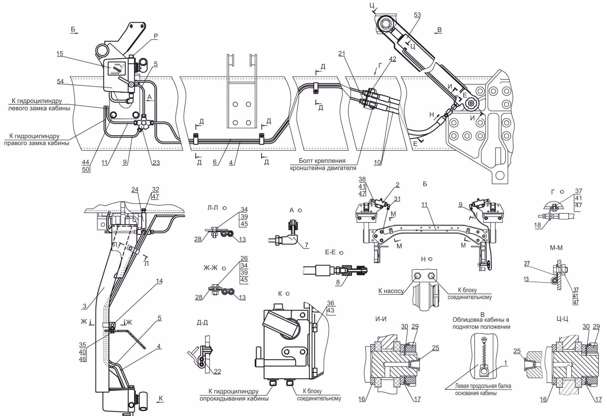
Рис. 268 Установка механизма подъема кабины 544019-5000040-010 Fig. 268 Installation cab tilting mechanism 544019-5000040-010
