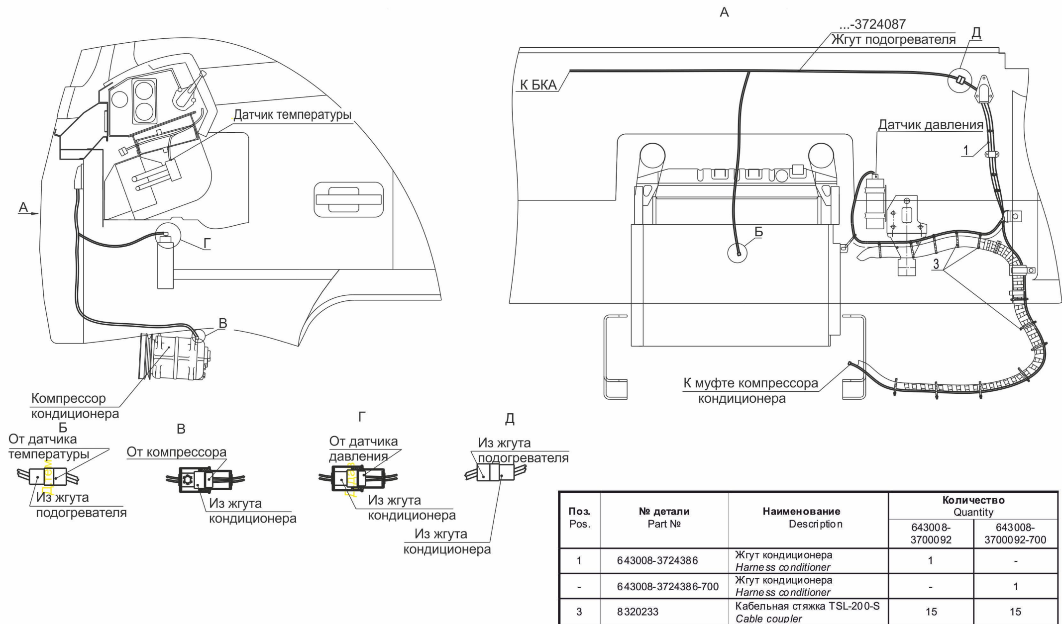
Рис. 300 Установка электрооборудования кондиционера 643008-3700092, (-700) Fig. 300 Installation of an electric equipment of the air conditioner 643008-3700092, (-700)
