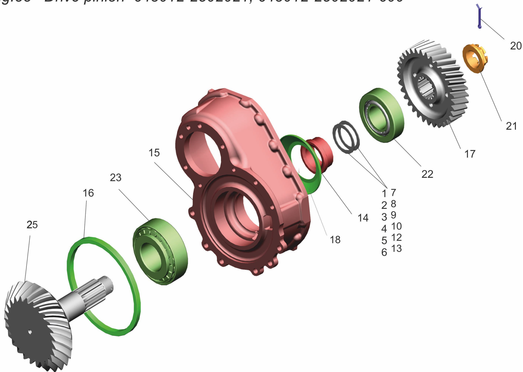
Рис. 88 Шестерня ведущая 643012-2502021, 643012-2502021-600 Fig.88 Drive pinion 643012-2502021, 643012-2502021-600
