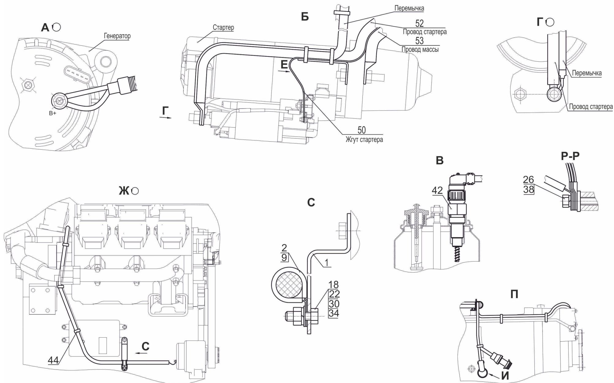
Рис.199 Установка электрооборудования на двигателе 544019-3700098 (лист 2) Fig. 199 Electric equipment installation on the engine 544019-3700098 (page 2)
