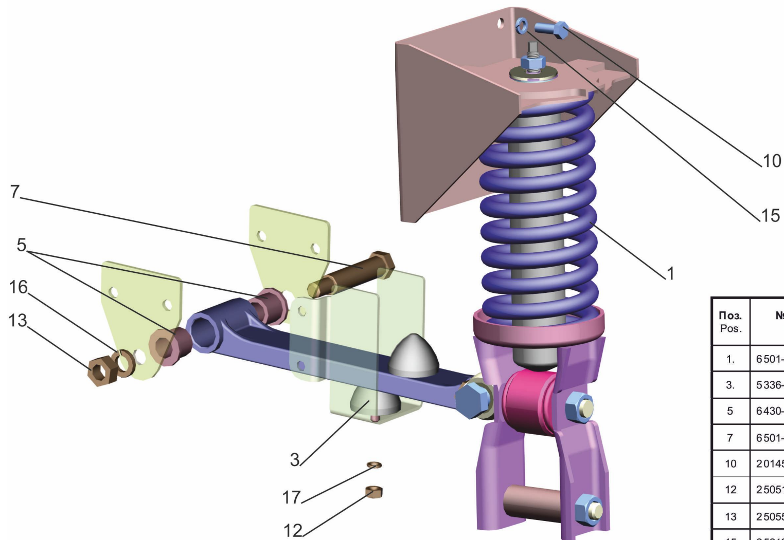
Рис.223 Заднее подрессоривание 6501-5001800-010 Fig.223 Rear springing 6501-5001800-010
