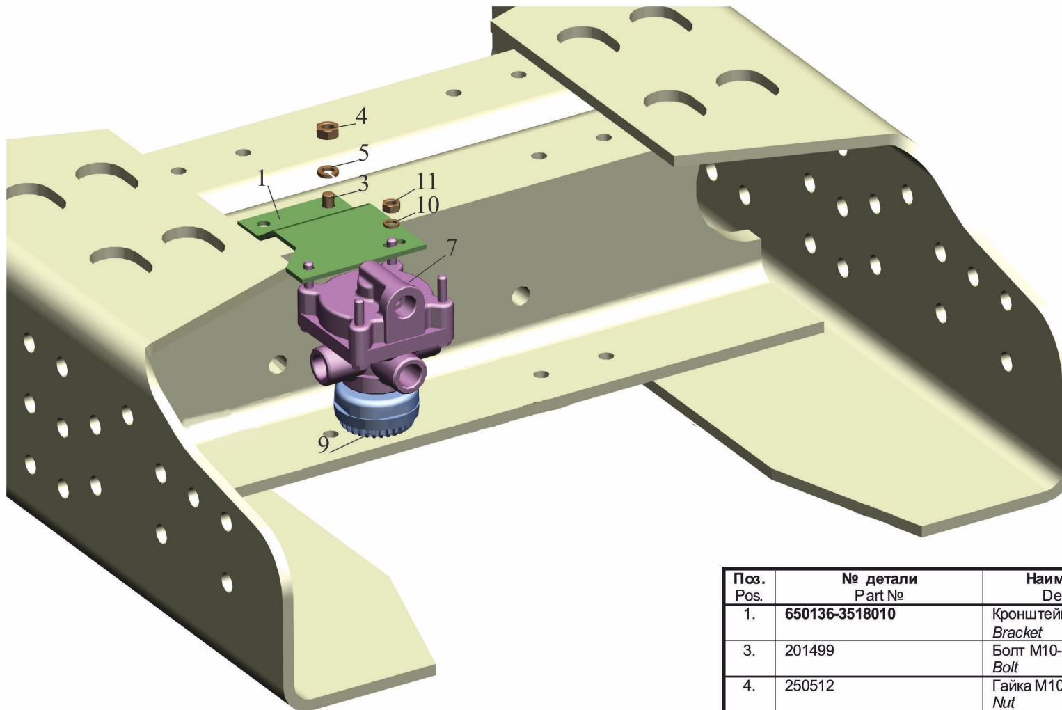
Рис. 170 Крепление клапана ускорительного 643018-3518004 Fig. 170 Installation of relay valve 643018-3518004
