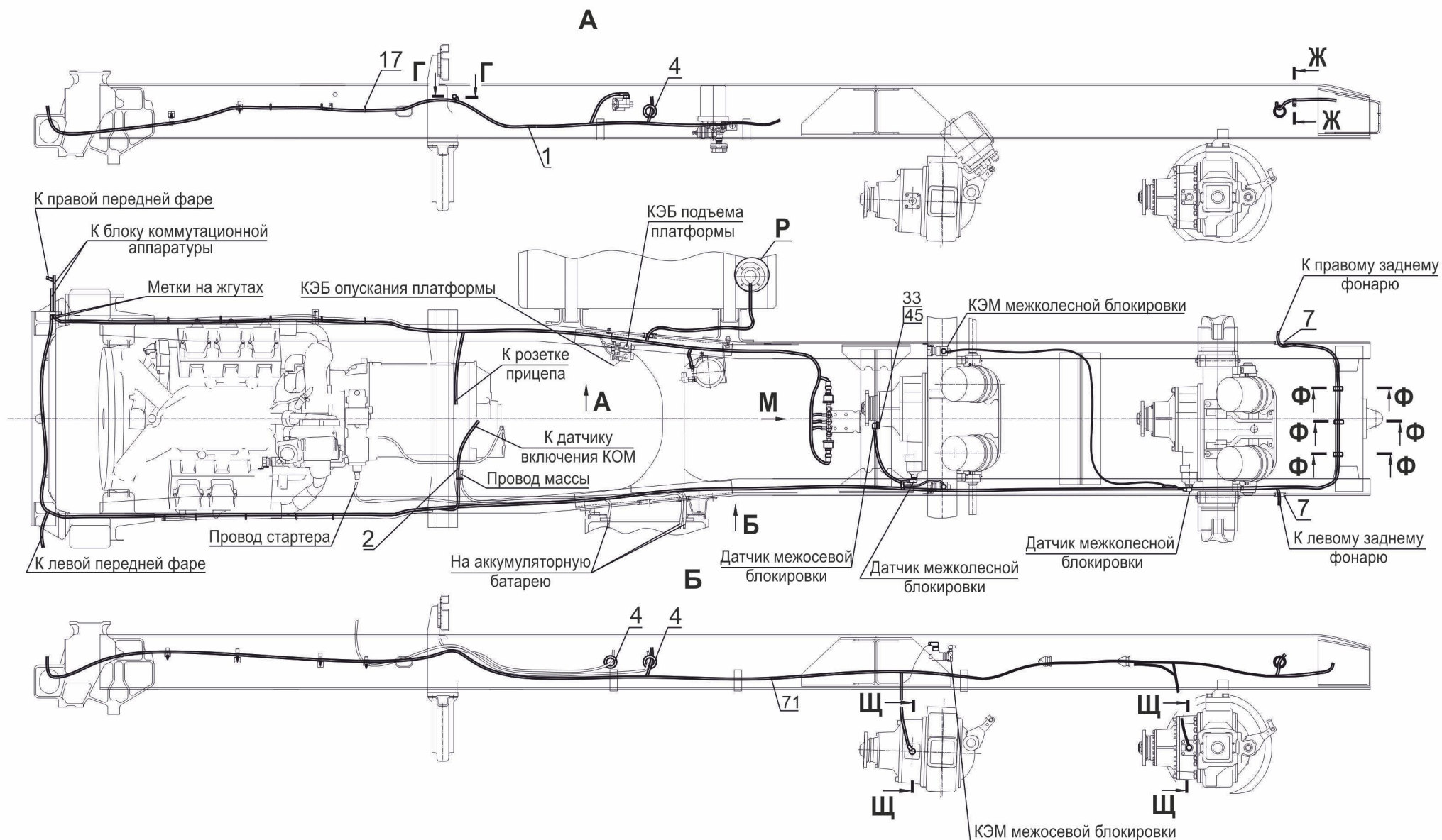
Рис. 186 Установка электрооборудования на шасси 643018-3700010-090, (-790) (лист 1) Fig. 186 Installation of electrical equipment on the chassis 643018-3700010-090, (-790) (page 1)
