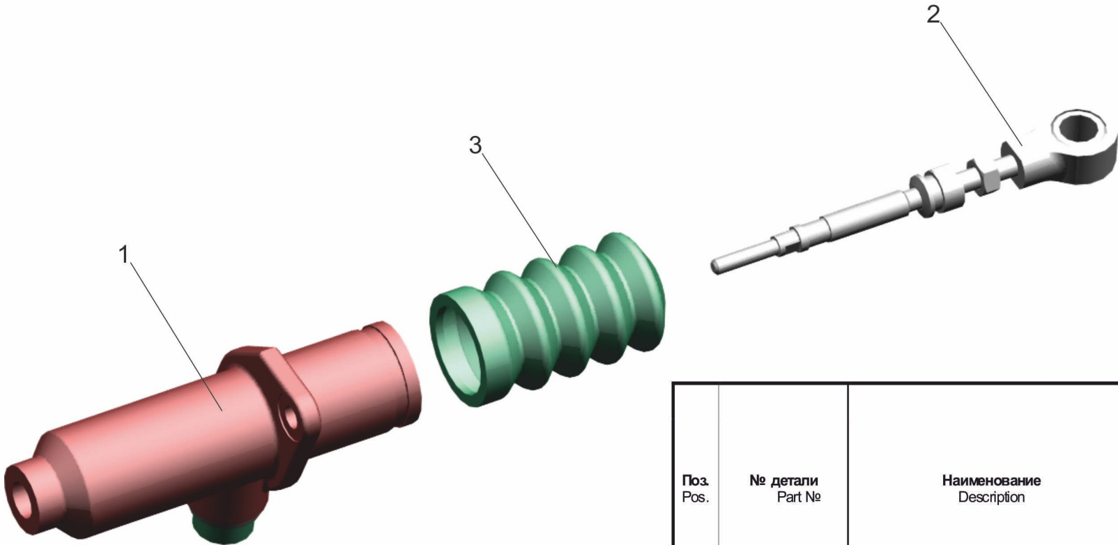
Рис. 36 Цилиндр подпедальный с толкателем 6430-1602500-000 (6430-1602500-001, 6430-1602500-020, 6430-1602500-002) Fig. 36 Under pedal cylinder with a pusher 6430-1602500-000 (6430-1602500-001, 6430-1602500-020, 6430-1602500-002)
