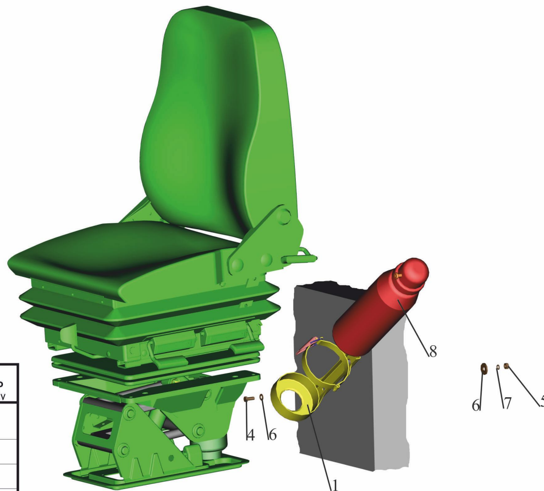
Рис. 218 Установка огнетушителя 6430-3910040 Fig.218 Installation of fire extinguisher 6430-3910040
