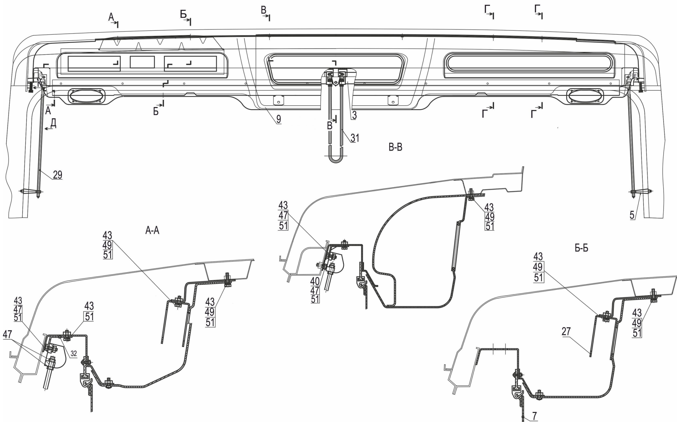
Рис. 257 Установка полки, штор 5440-8200034-010 Лист 1 Fig. 257 Installation Curtains and sun 5440-8200034-010 Page 1
