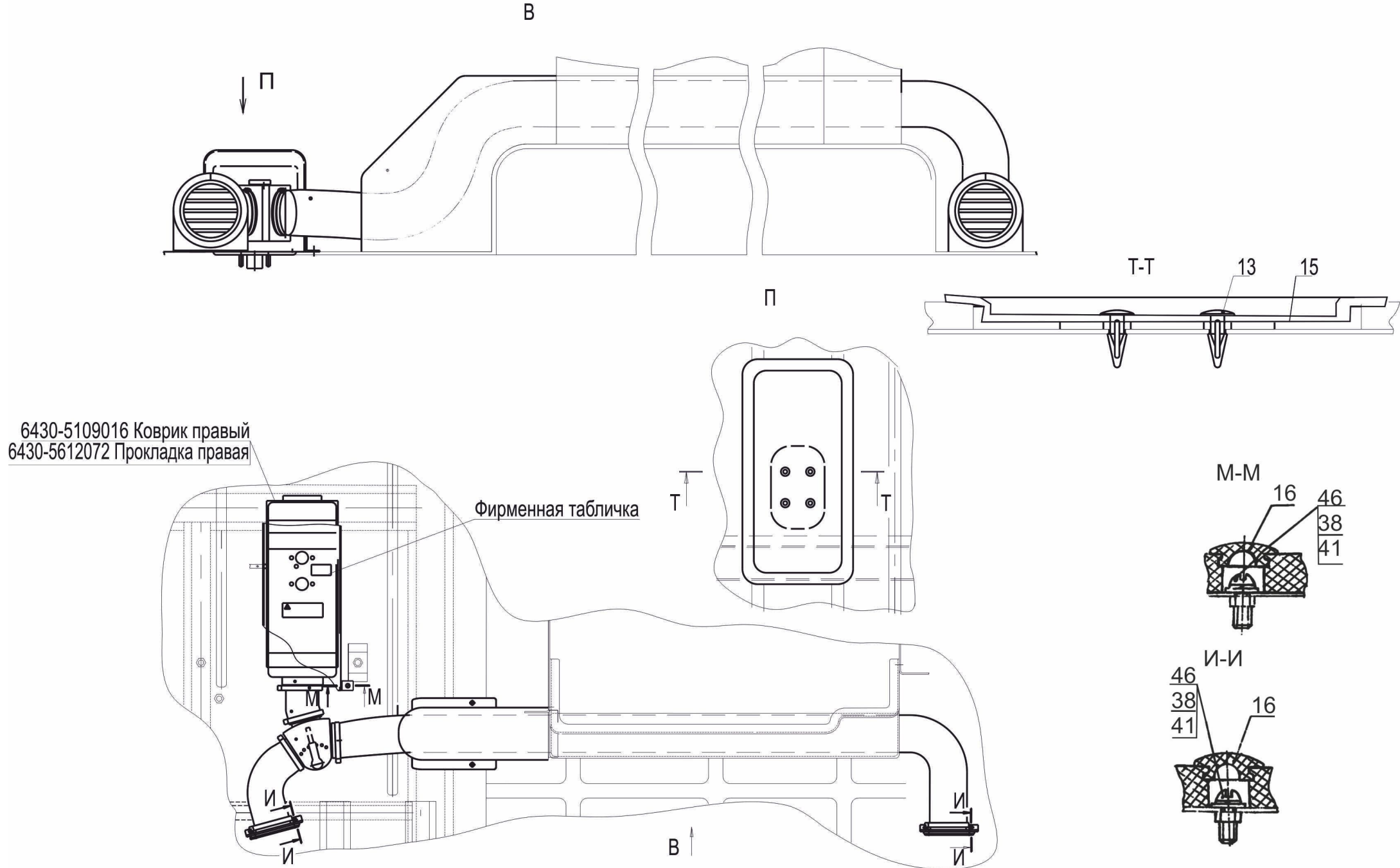
Рис. 293 Установка независимого воздушного отопителя 6430-8100002-021 Fig.293 Installation of the independent air heater 6430-8100002-021
