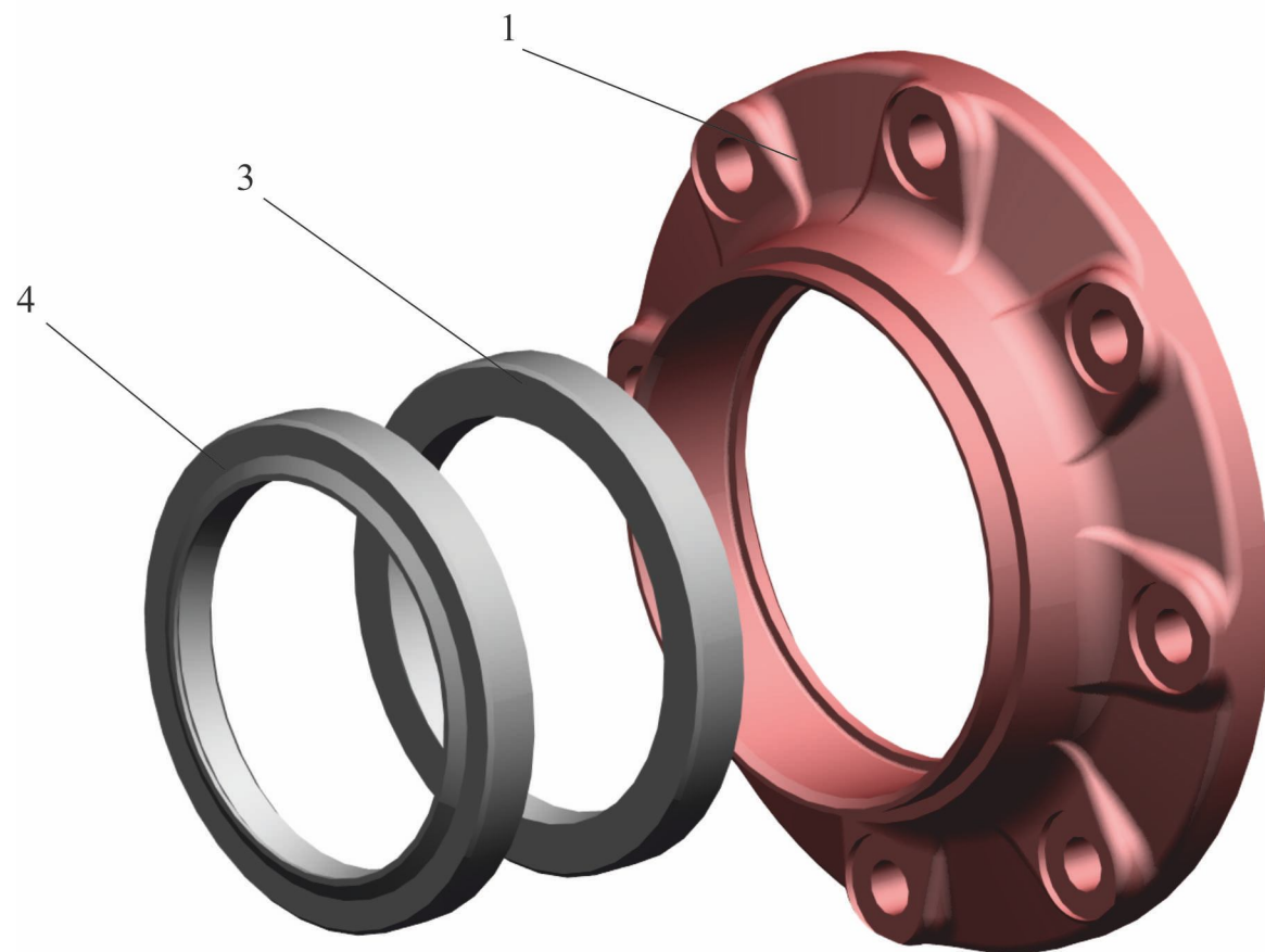
Рис.85 Крышка 6430-2502140 Fig.85 Cover 6430-2502140
