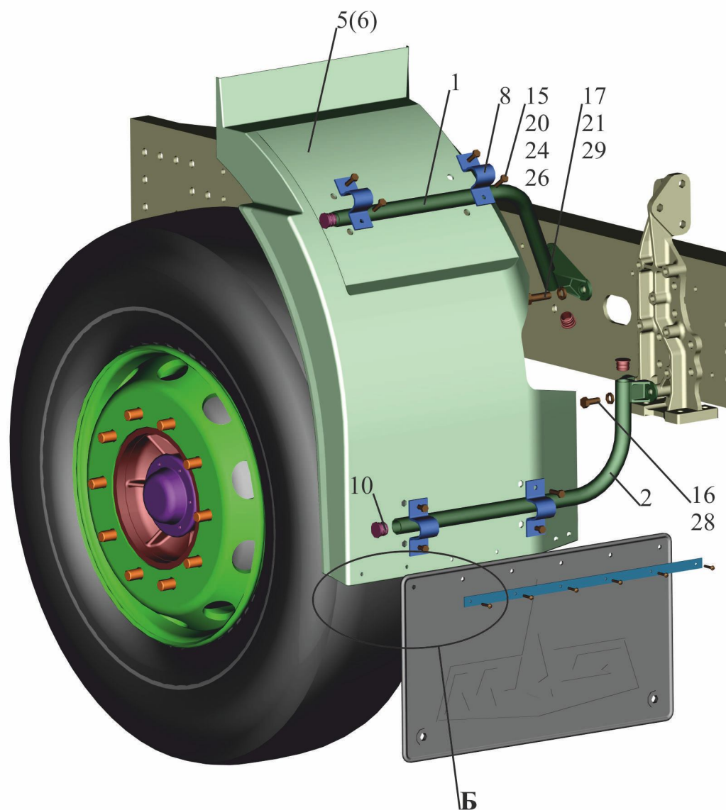
Рис. 306 Установка брызговиков передних колес 643019-8400030 Fig. 306 Installation of front wheels mudguards 643019-8400030
