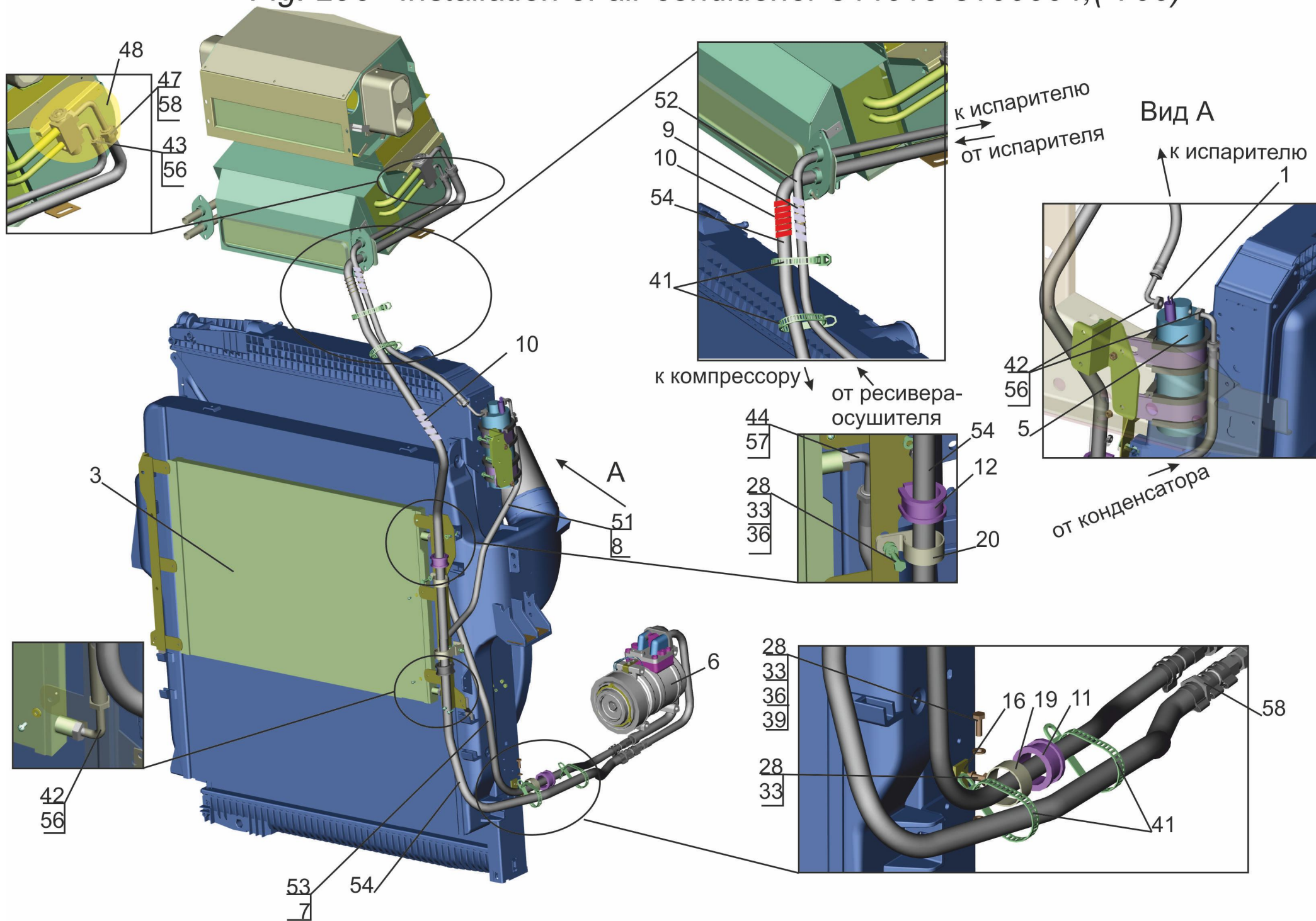
Рис. 296 Установка кондиционера 544019-8100004, (-700) Fig. 296 Installation of air-conditioner 544019-8100004, (-700)
