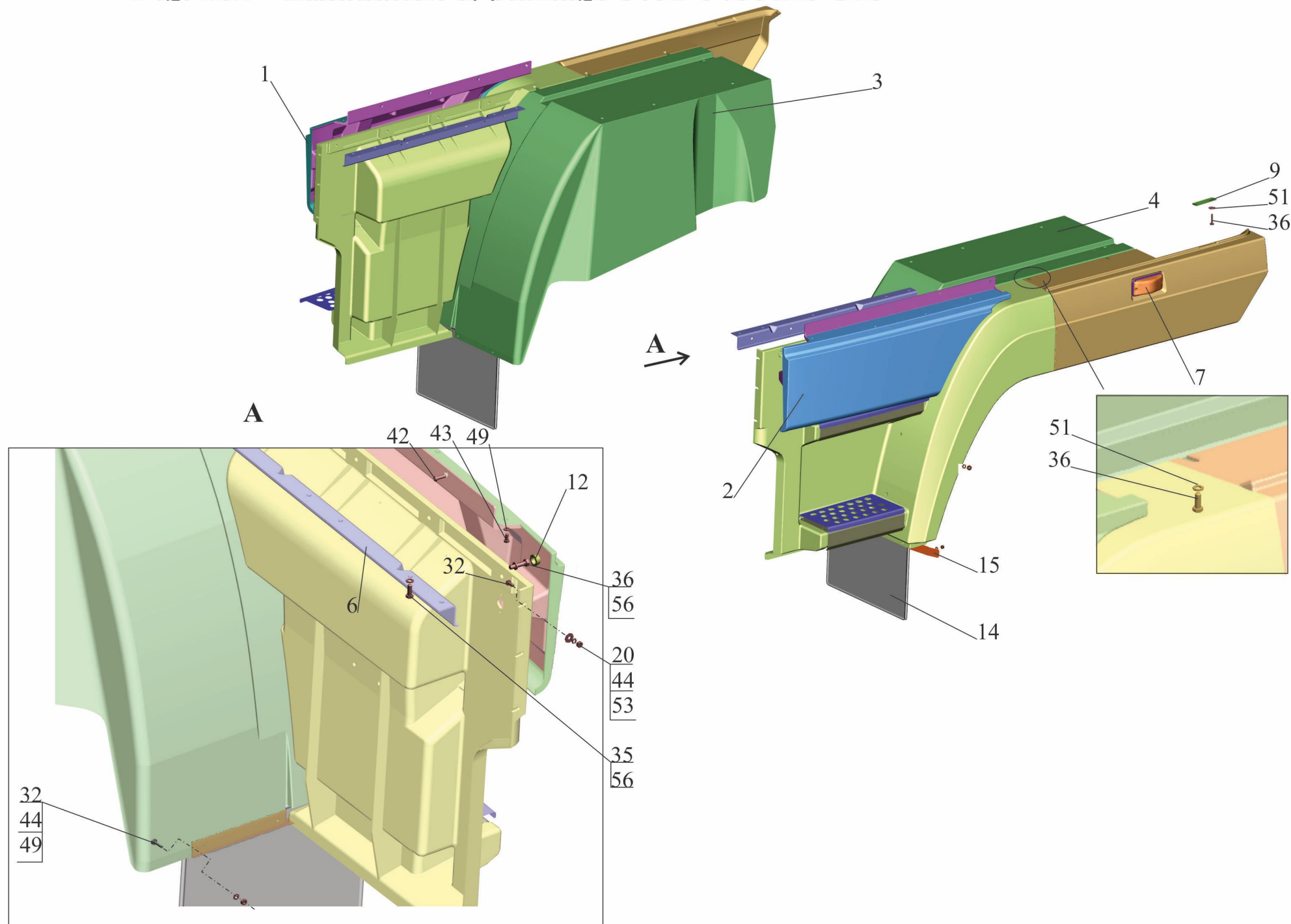
Рис. 262 Установка оперения 6431-8400020-010 Fig. 262 Installation of plumage 6431-8400020-010
