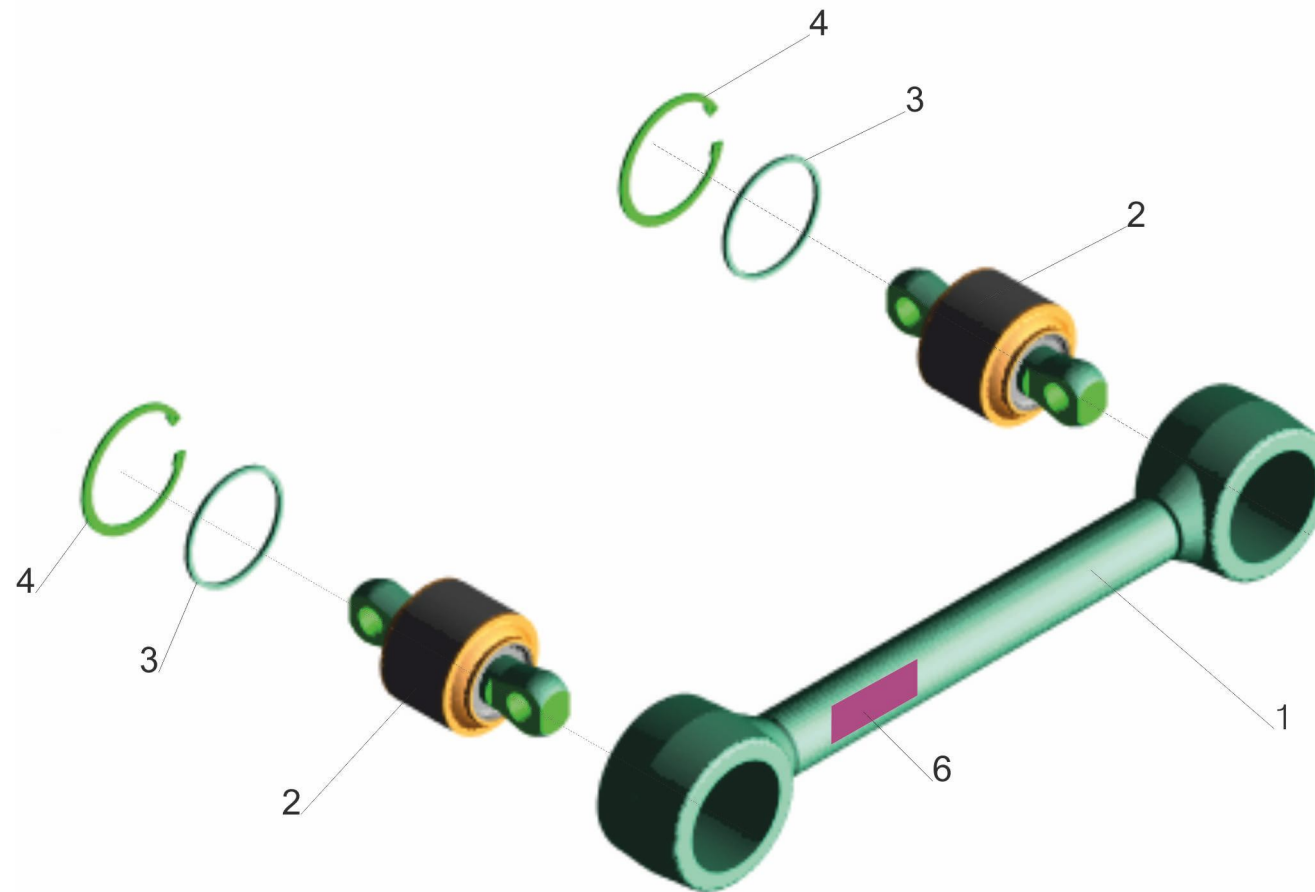
Fig.114 Torque rod 6430-2919014
