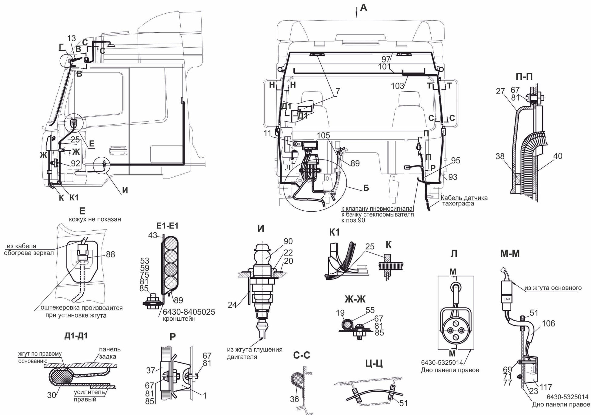
Рис.189 Установка электрооборудования в кабине 5340А5-3700076 (лист 1) Fig.189 Installation of an electrical equipment in a cabin 5340А5-3700076 (page 1)
