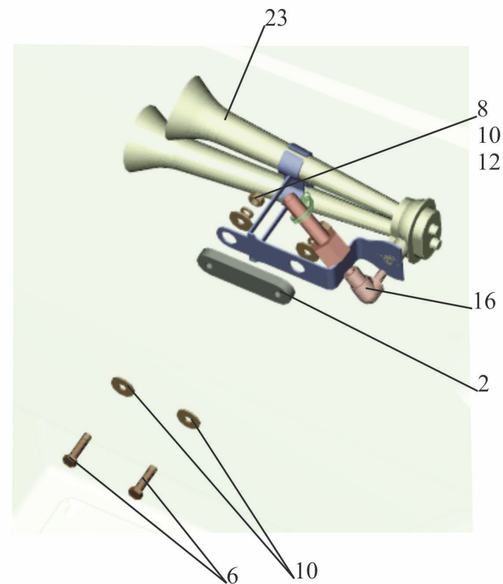
Вид А
