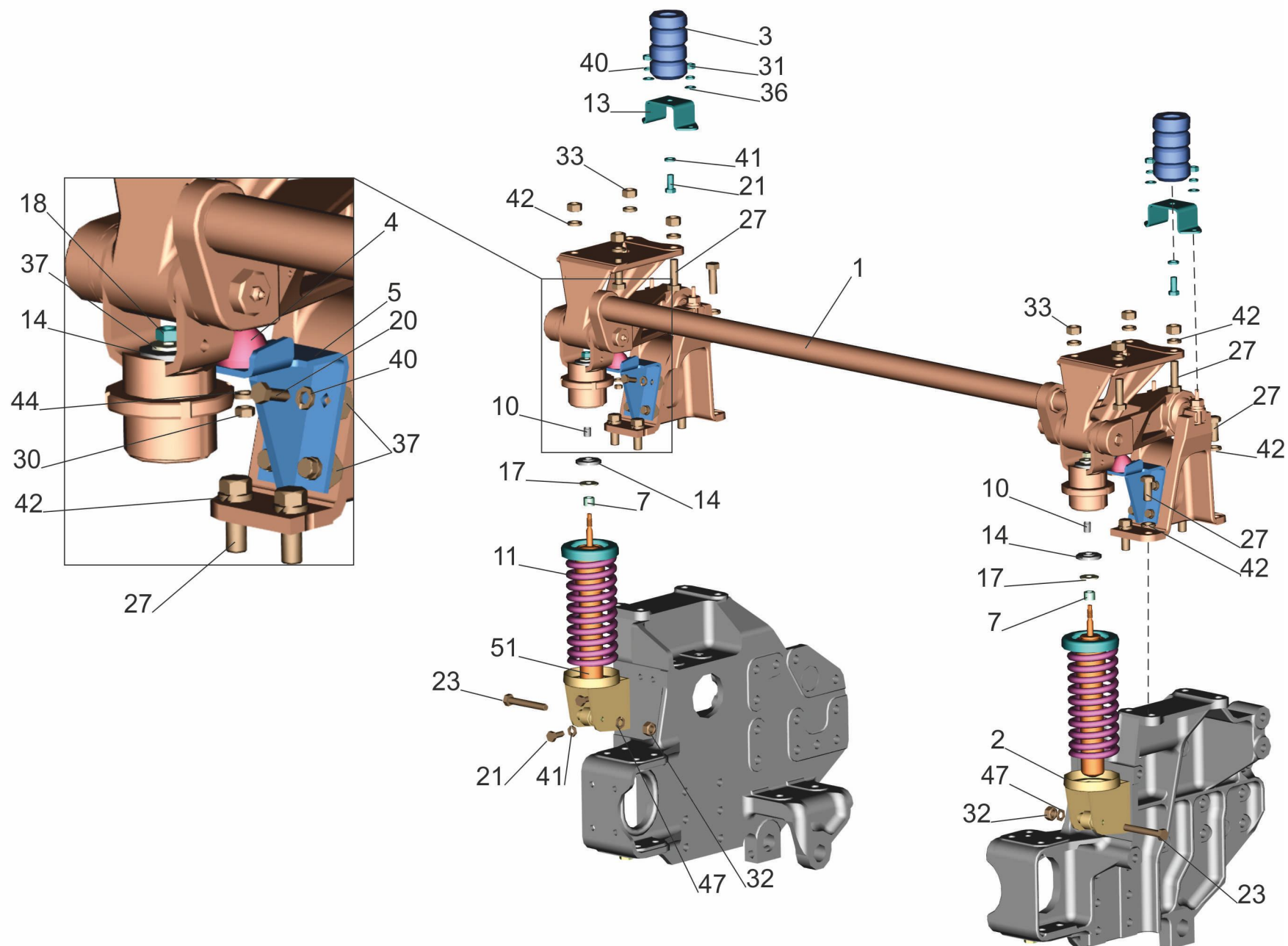
Рис. 221 Переднее подрессоривание кабины 643019-5001700-010 Fig. 221 Front springing the cab 643019-5001700-010
