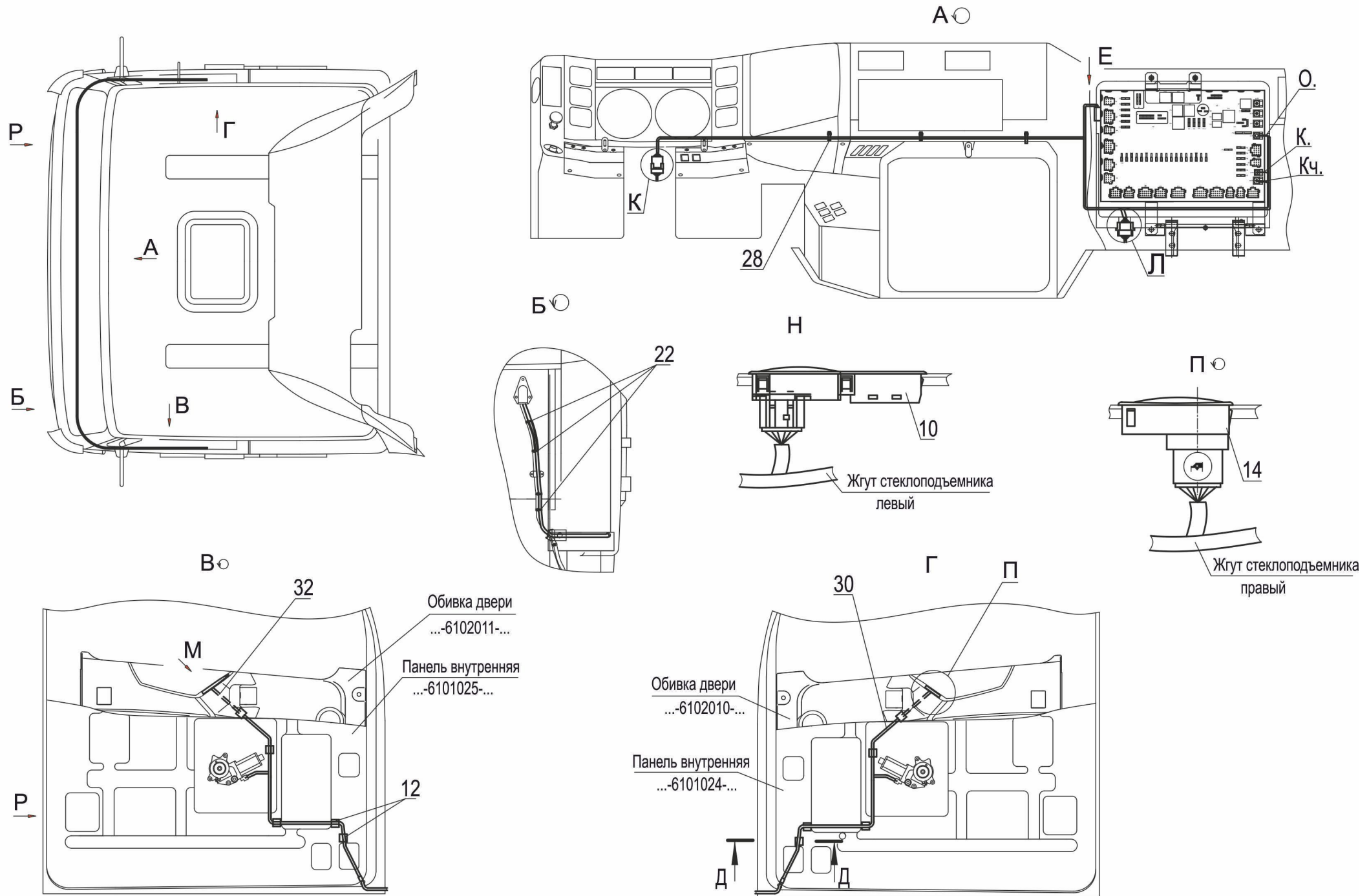
Рис.231 Установка электрооборудования стеклоподъемников Лист 1 Fig. 231 Installation of an electric equipment lève-glaze Page 1
