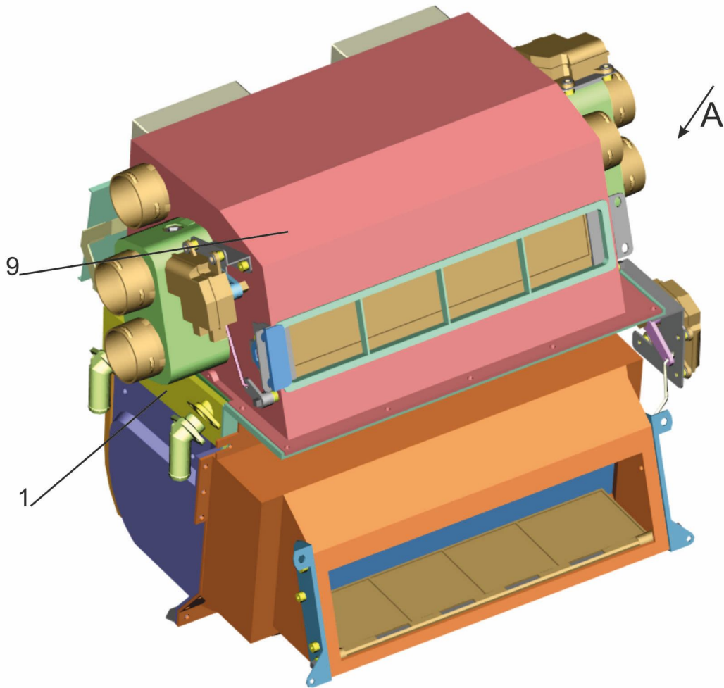
Рис. 280 Отопитель 643008-8101010 Fig. 280 Heater 643008-8101010
