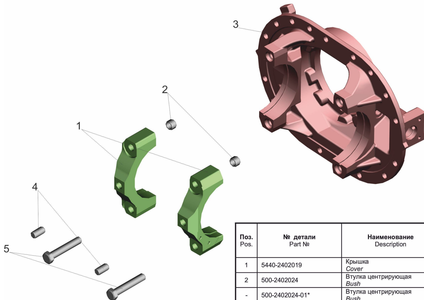
Рис. 68 Картер редуктора 5440-2402015-010 Fig. 68 Reducer gear housing 5440-2402015-010
