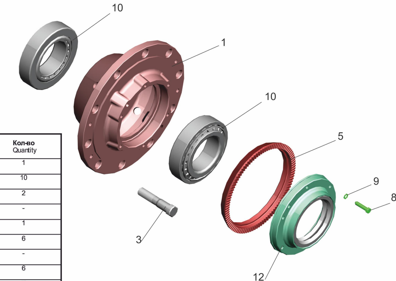
Рис.60 Ступица с крышкой 544019-3104006-600 Fig.60 Rear with cover
