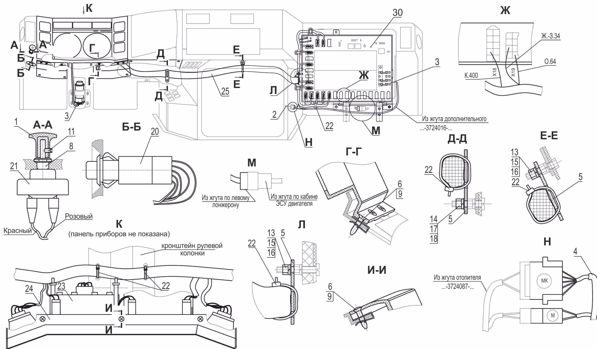
Рис. 204 Установка щитка приборов и коммутационной аппаратуры 555035-3800001, (-700) Fig. 204 Installation board devices and switching instrumentation 555035-3800001, (-700)
