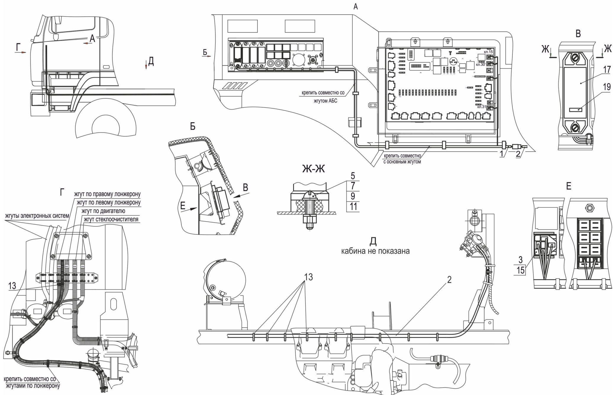
Рис.201 Установка нагревателей на двигателе 5440E9-3700101-000 Fig. 201 Installation of heaters on the engine 5440E9-3700101-000
