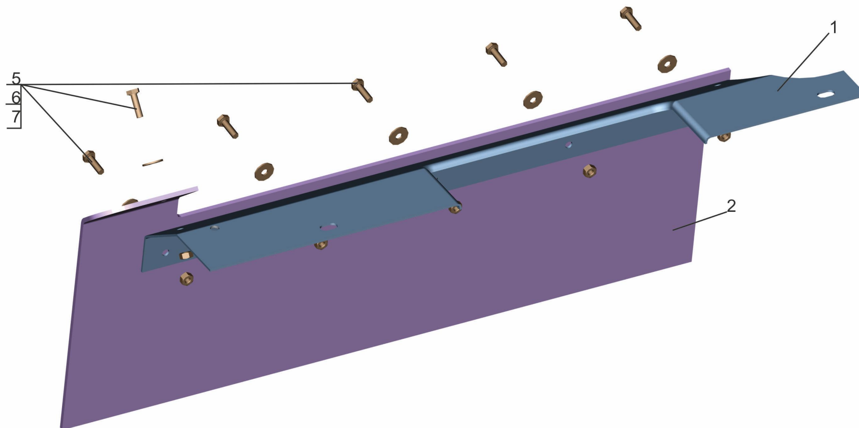
Рис. 27 Уплотнитель с пластиной 544019-1310068-010 Fig. 27 Seal with plate 544019-1310068-010
