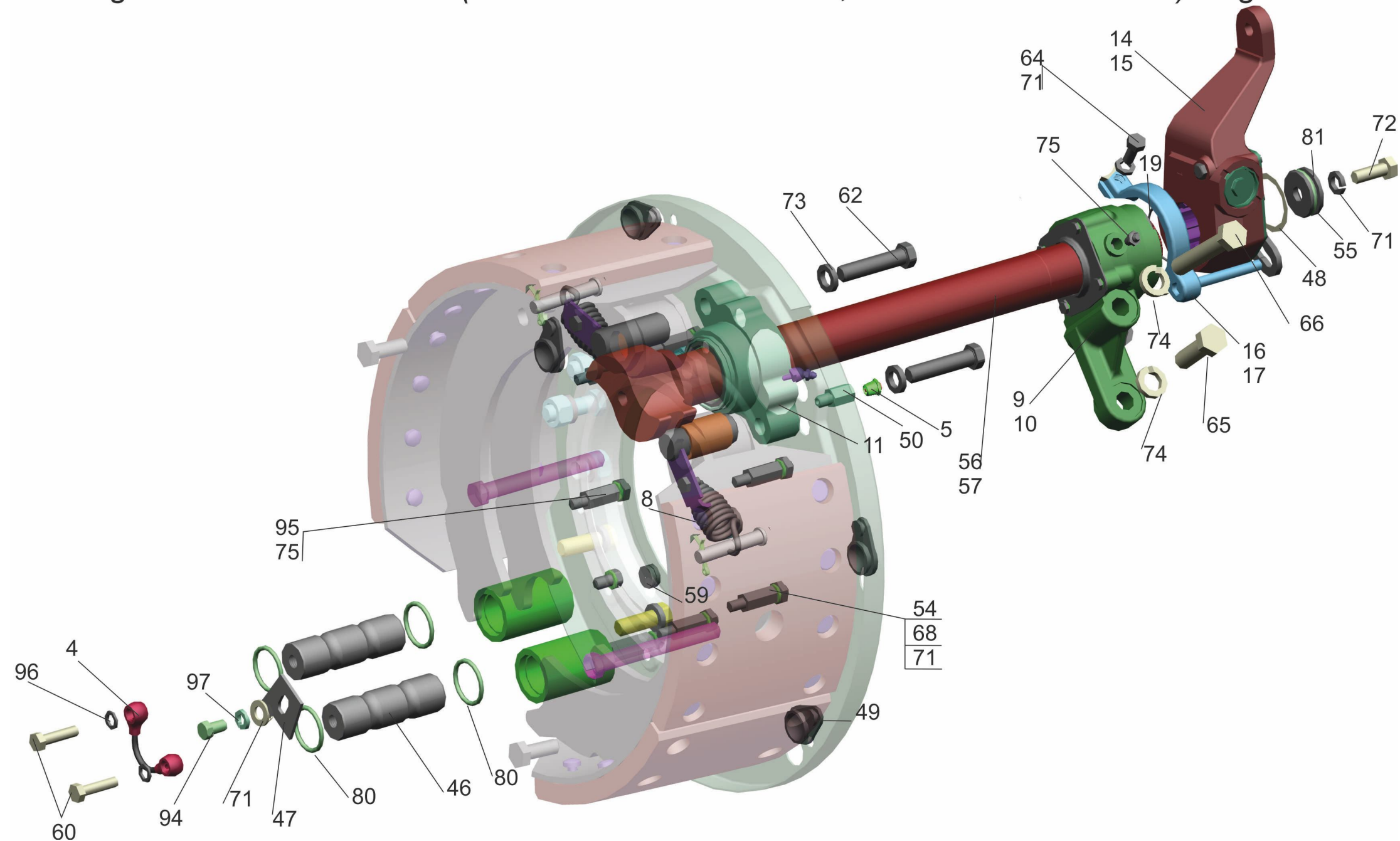
Рис.77 Мост средний(для мостов 643011-2500012, 643011-2500012-600) Лист 2 Fig.77 Intermediate axle (for axle 643011-2500012, 643011-2500012-600) Page 2
