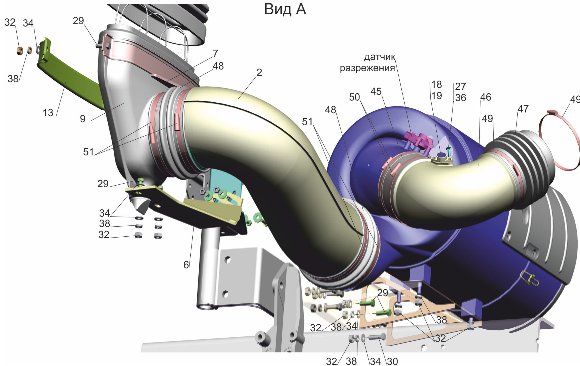
Рис. 23 Крепление воздушного фильтра 544018-1109002 (лист 2) Fig. 23 Air filter mounting 544018-1109002 (page 2)
