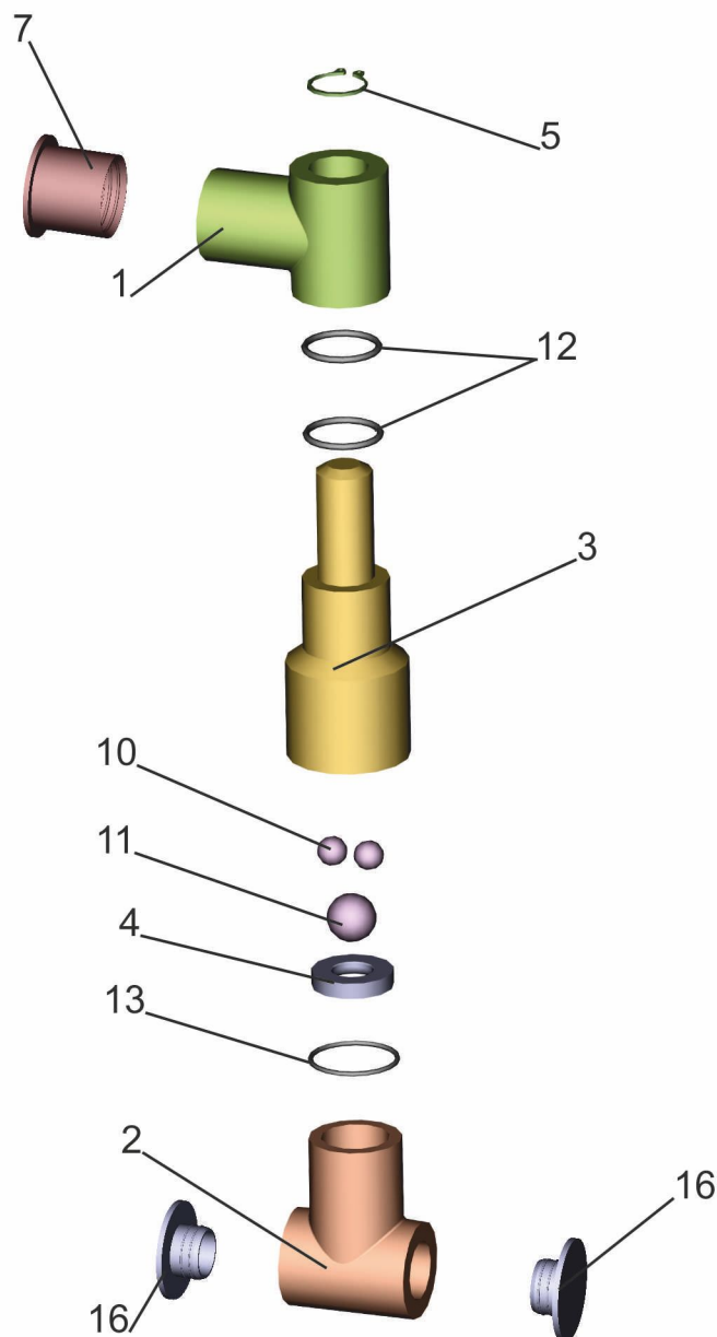
Рис.315 Клапан обратный с арматурой 551639-8609238. Fig.315 Return valve 551639-8609238.
