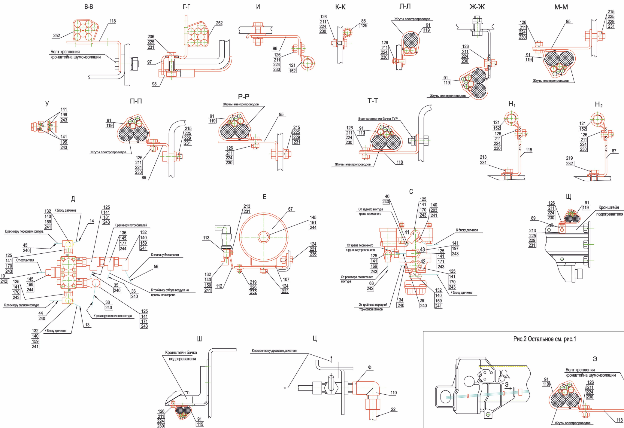
Рис. 165 Установка пневмотормозов 643018-3500003(-001) (лист-2) Fig. 165 Installation pneumobrakes
