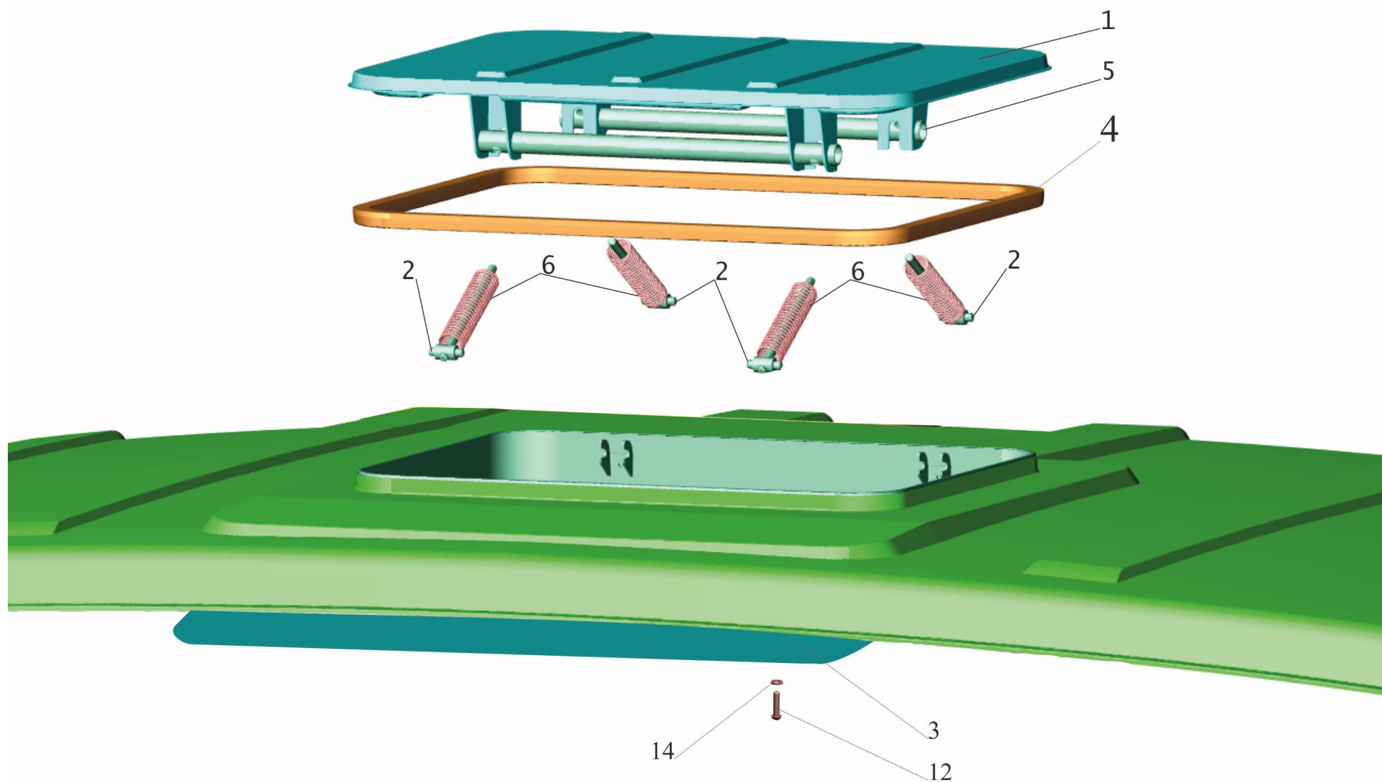
Рис.239 Установка люка 6430-5700010-020 Fig.239 Installation hatch 6430-5700010-020
