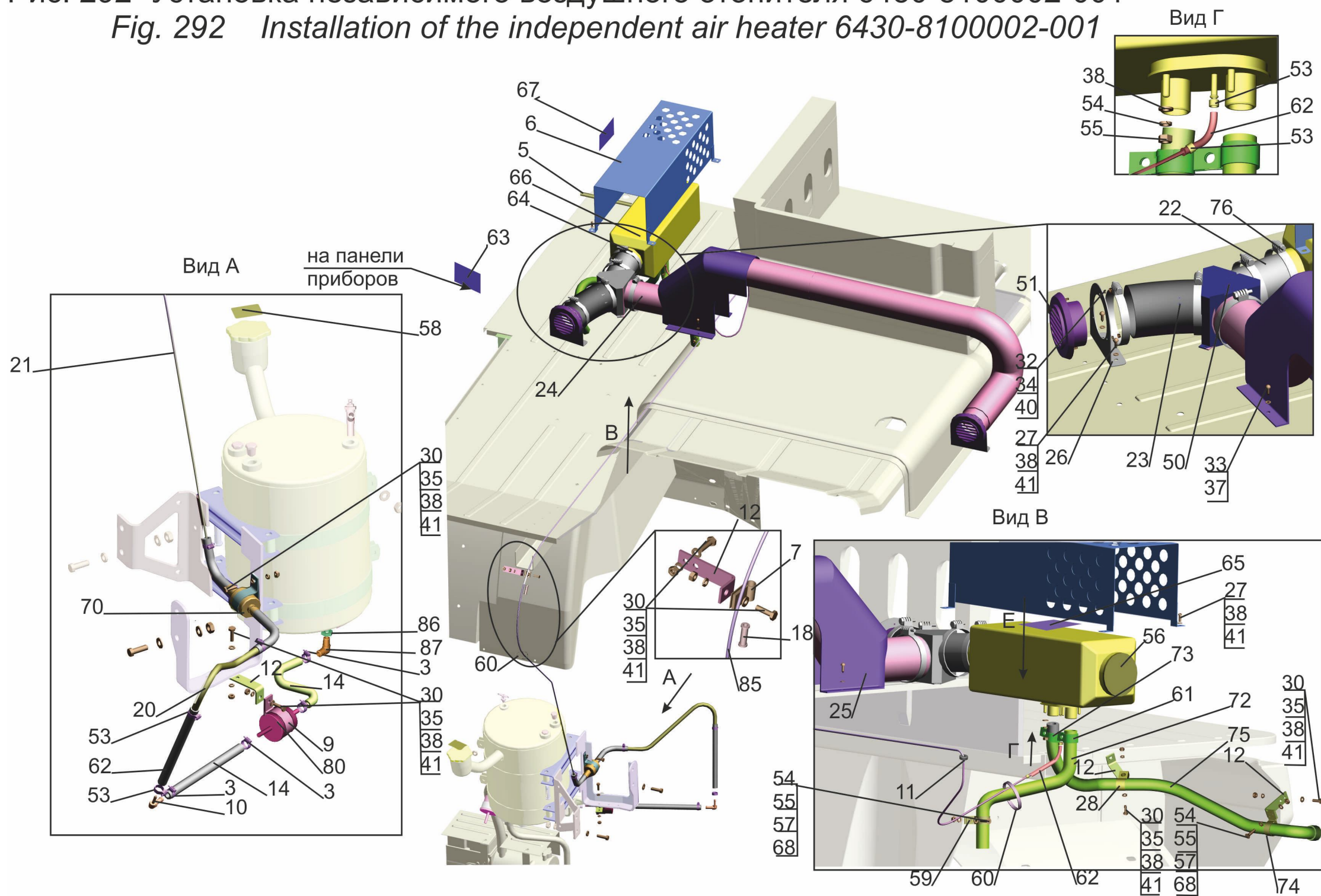
Рис. 292 Установка независимого воздушного отопителя 6430-8100002-001
