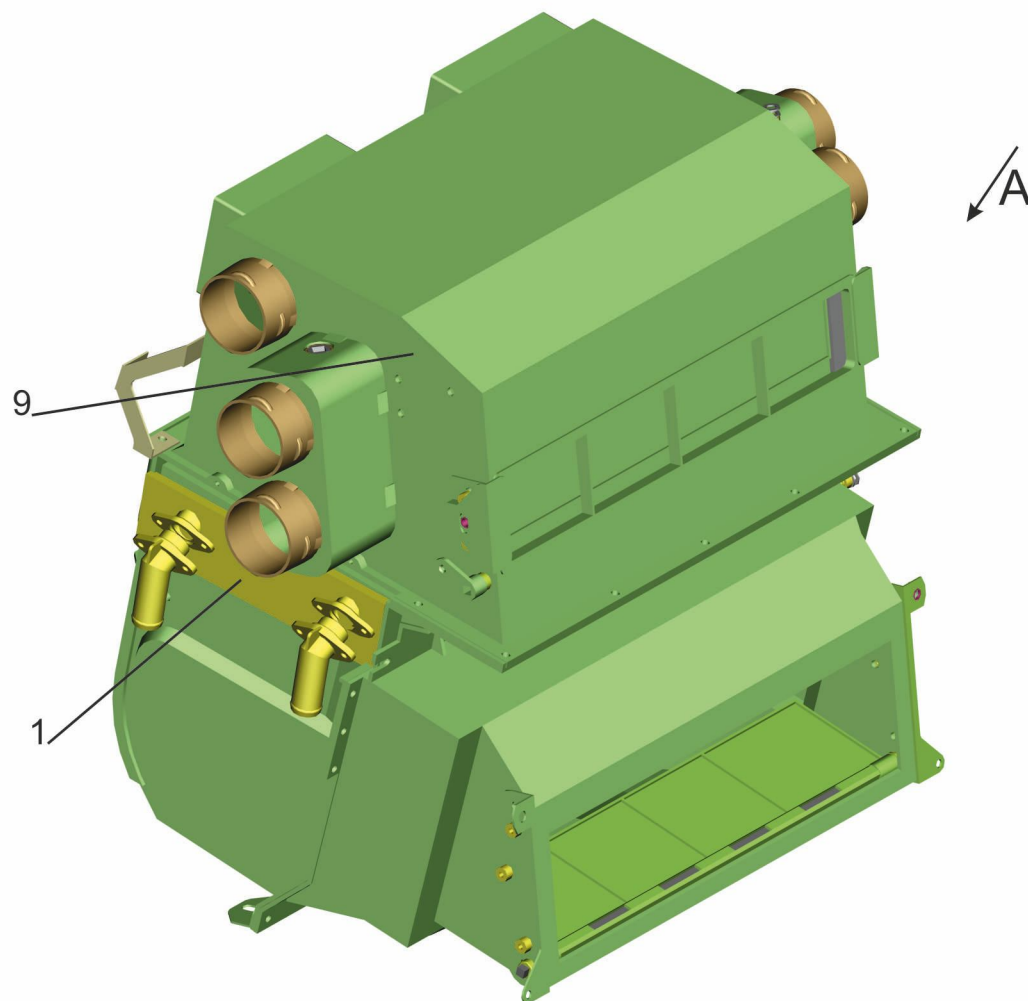
Рис 279 Отопитель 650118-8101010 Fig 279 Heater 650118-8101010
