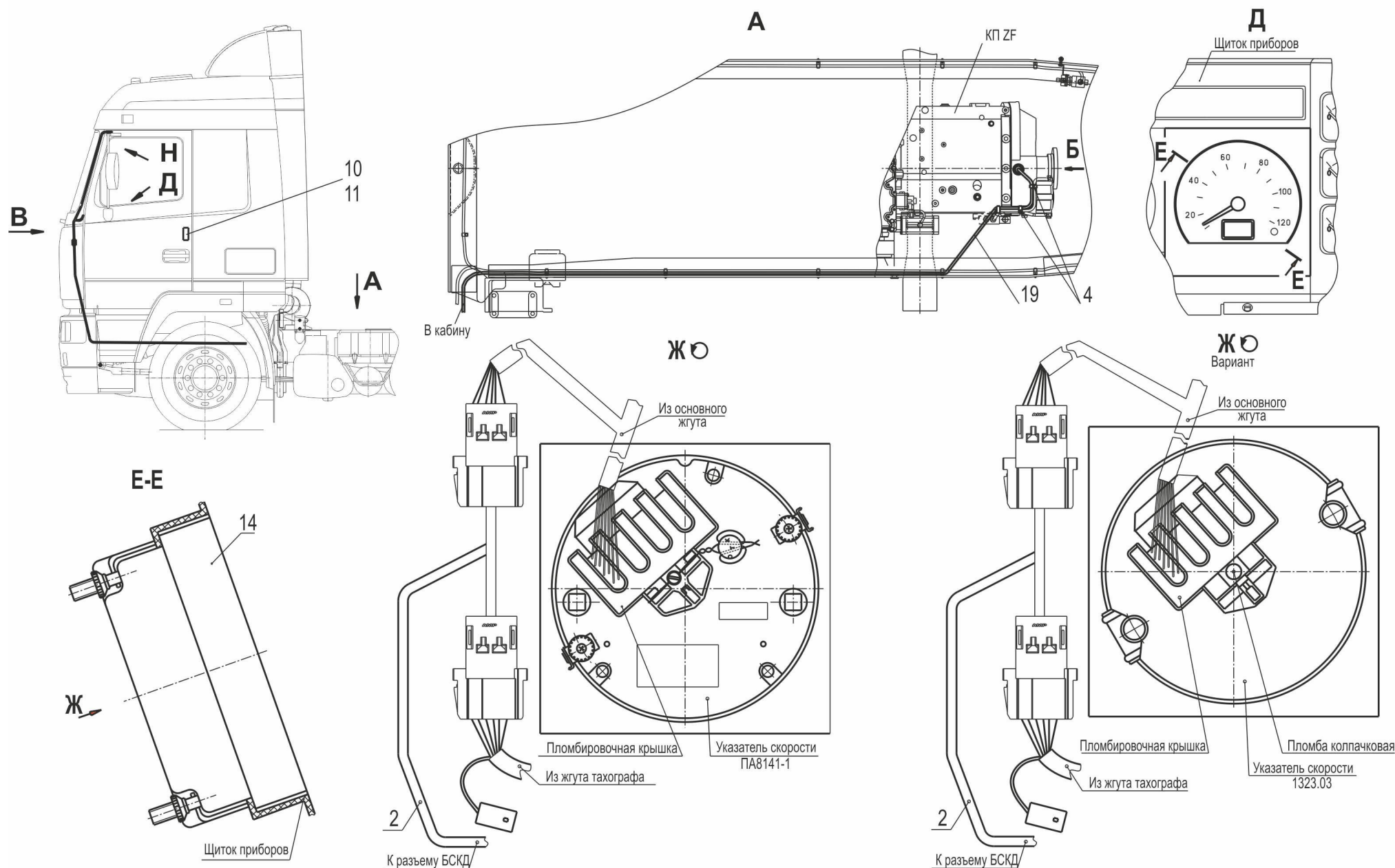
Рис. 209 Установка и пломбировка тахографа 544069-3800005 (лист 1) Fig.209 Installation and identification seal of tachograph 544069-3800005 (page 1)
