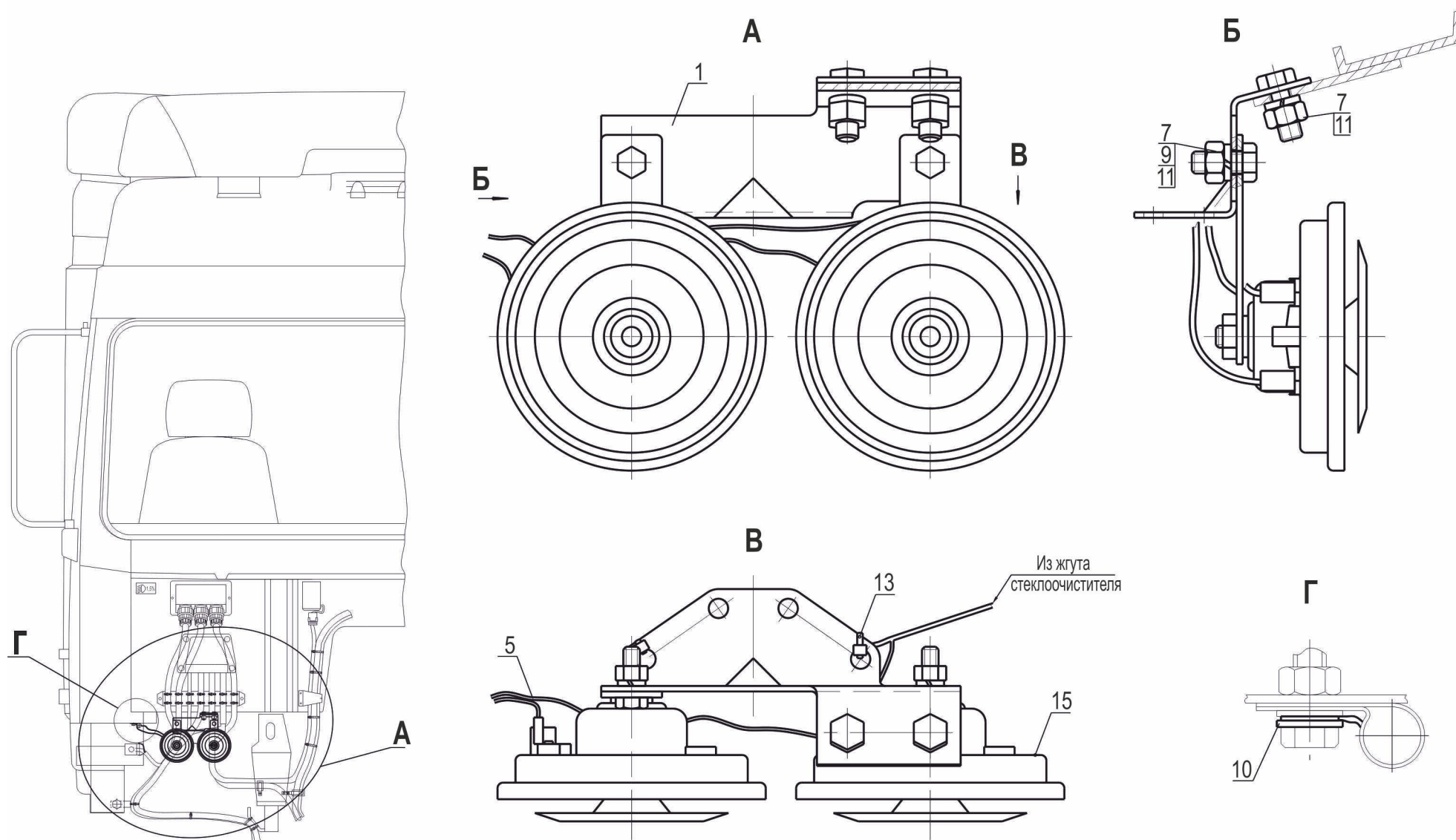
Рис. 194 Установка звуковых сигналов 643008-3700024-000 Fig.194 Installation of audible signals 643008-3700024-000
