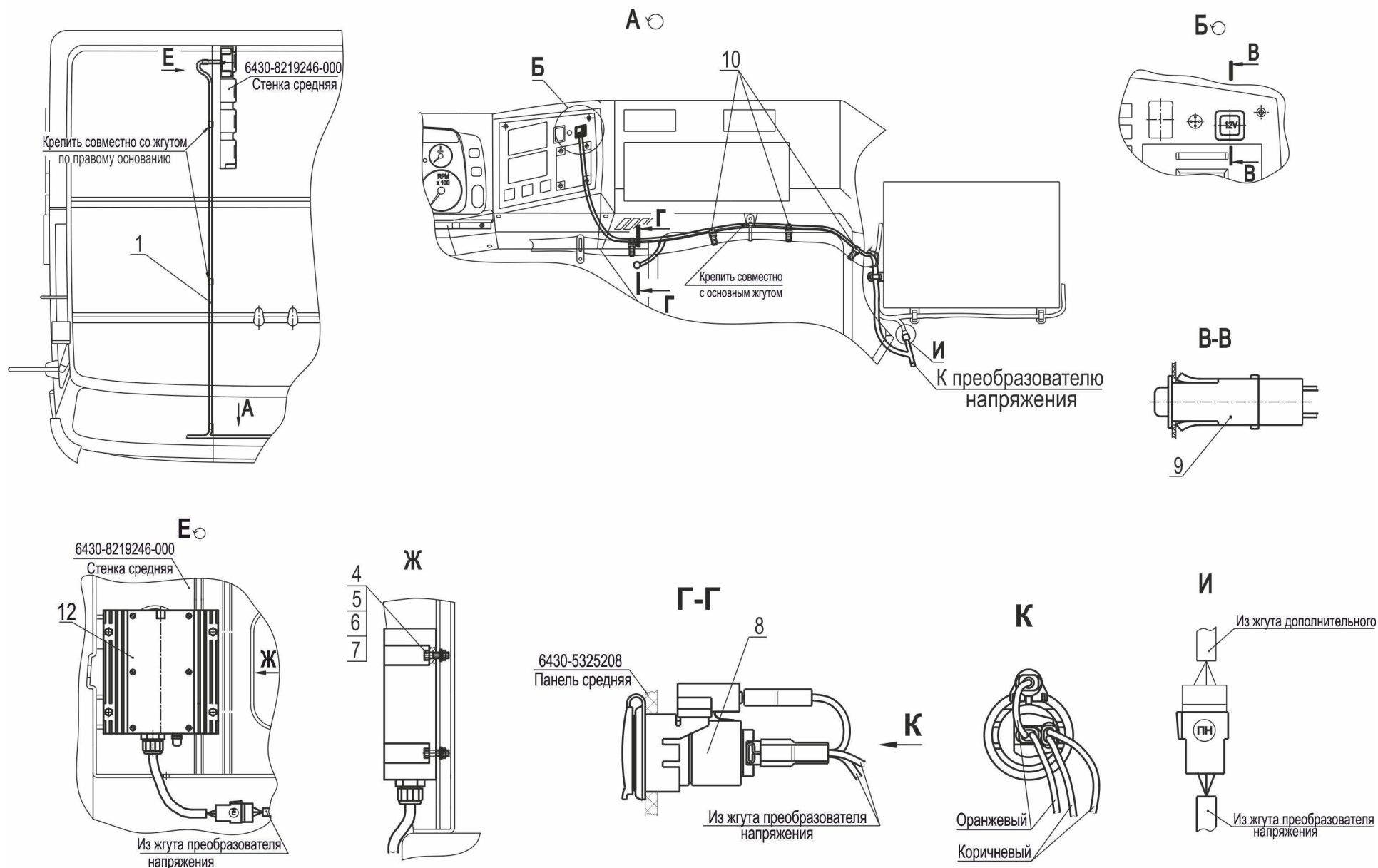
Рис.202 Установка преобразователя напряжения 6430-3700109 Fig. 202 Installation of a voltage changer 6430-3700109
