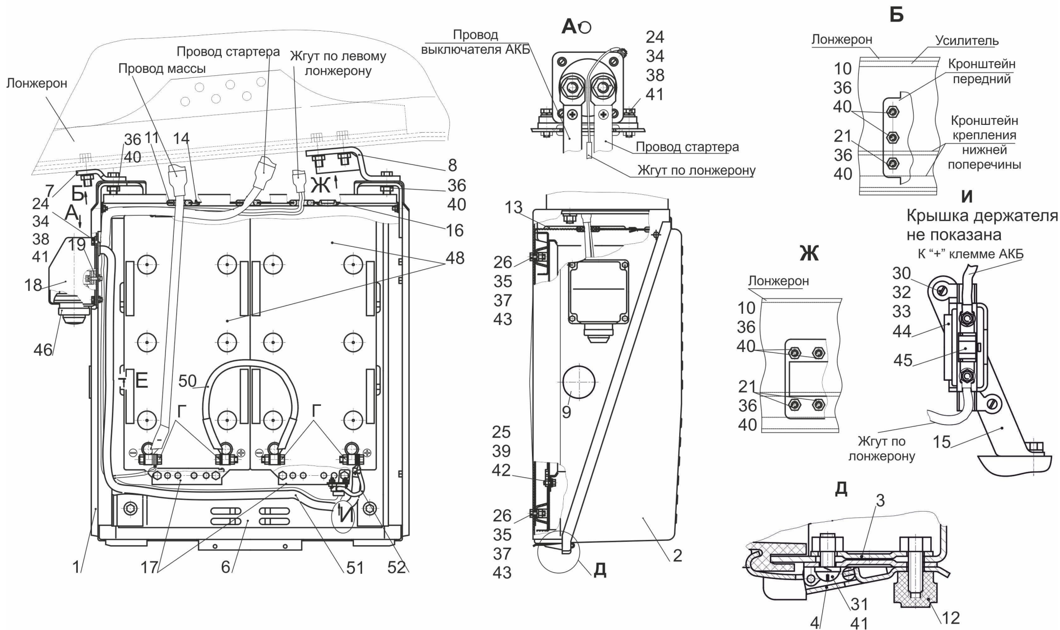
Рис. 184 Установка аккумуляторных батарей 650119-3700008, (-700) Fig. 184 Installation of storage batteries 650119-3700008, (-700)
