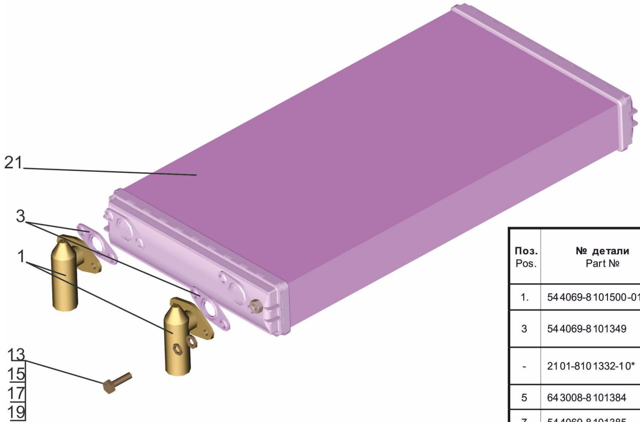
Рис. 283 Радиатор отопителя 643008-8101060-010 Fig. 283 Radiator of heating 643008-8101060-010
