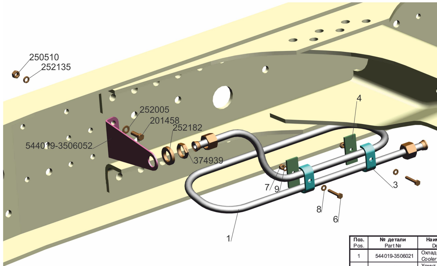
Рис. 166 Крепление охладителя 544019-3506020 Fig. 166 Mounting of cooler 544019-3506020
