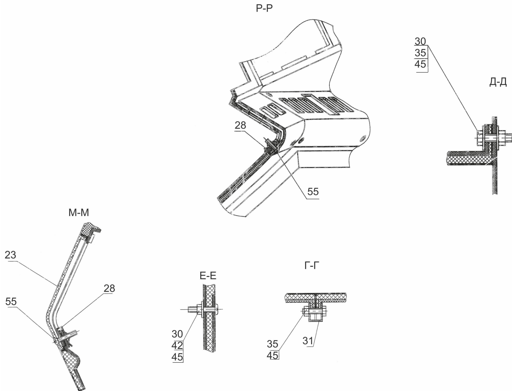
Рис. 238 Панели приборов 6430-5300016 Лист 2 Fig. 238 Installing of instrument panel 6430-5300016 Page 2
