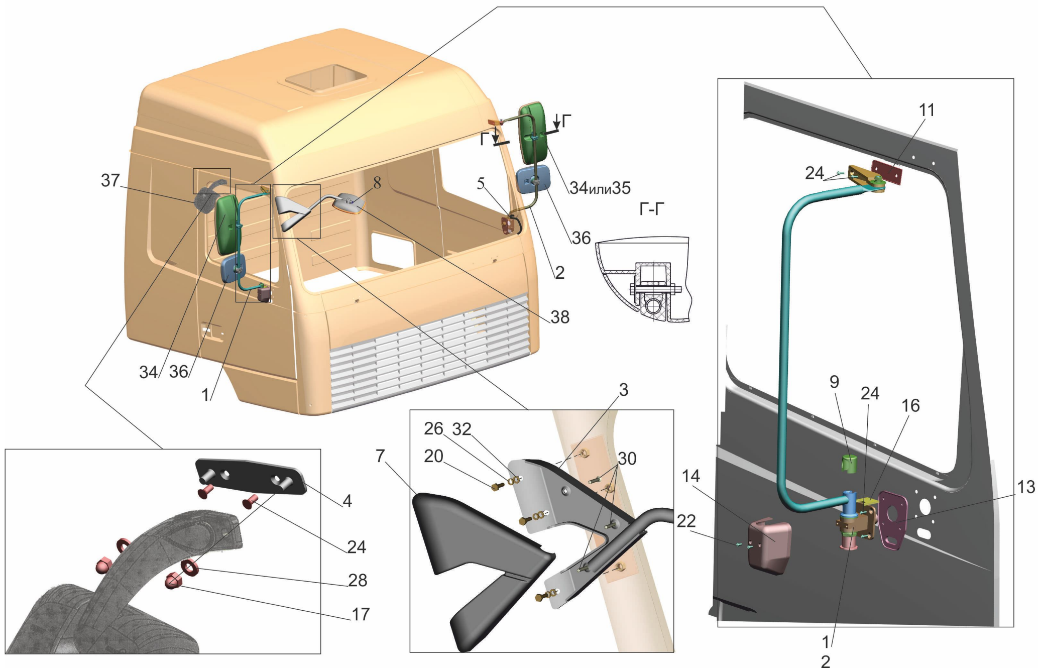
Рис. 254 Установка зеркал 6430-8200005-010,(-012) Fig. 254 Installation mirrors 6430-8200005-010,(-012)
