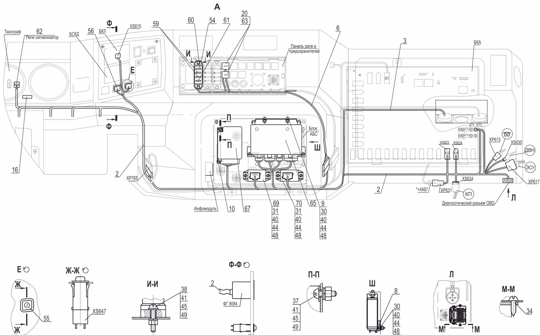
Рис. 216 Установка электрооборудования ЭСУ двигателя 544018-3800060, (-010) (лист 2) Fig. 216 Installation of electronic control system of the engine 544018-3800060, (-010) (page 2)
