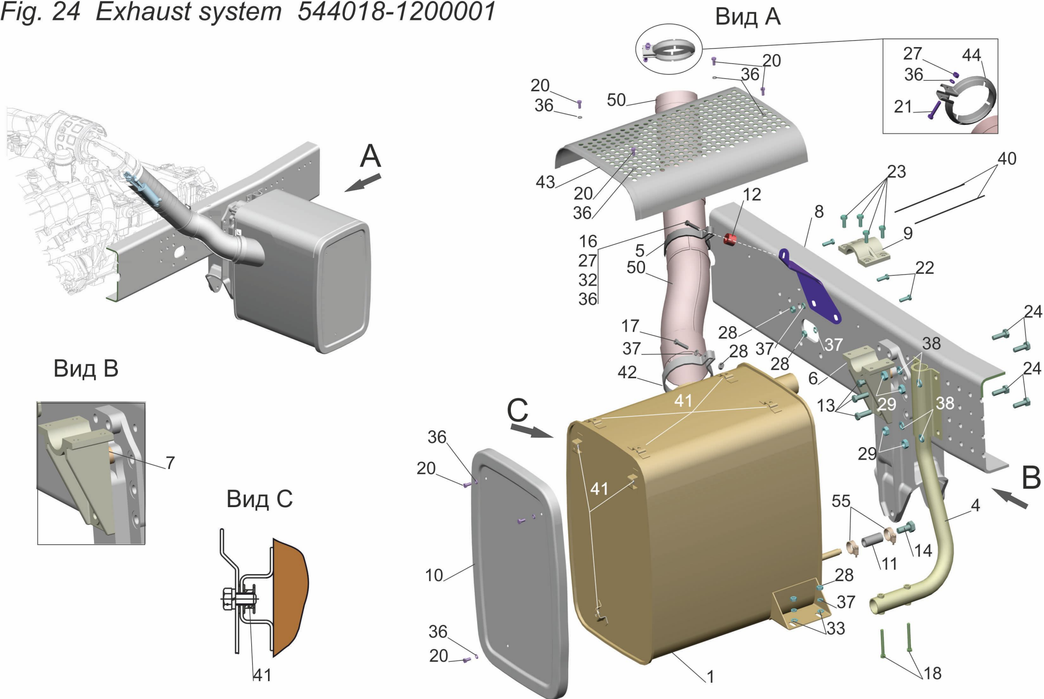
Рис. 24 Установка системы выпуска газов 544018-1200001
