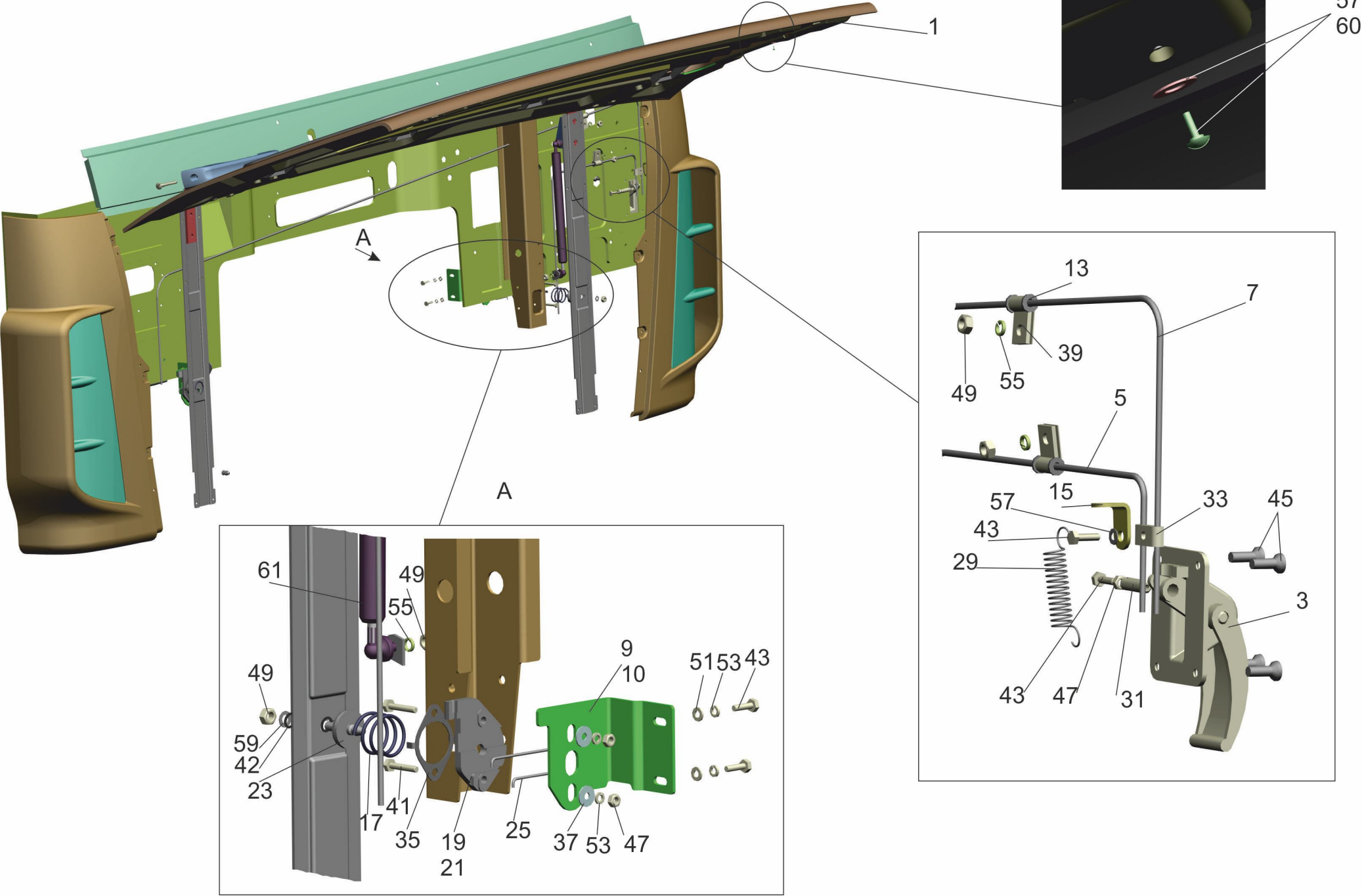
Рис. 261 Установка облицовки 6431-8400018-000 Fig.261 Installation of facing 6431-8400018-000
