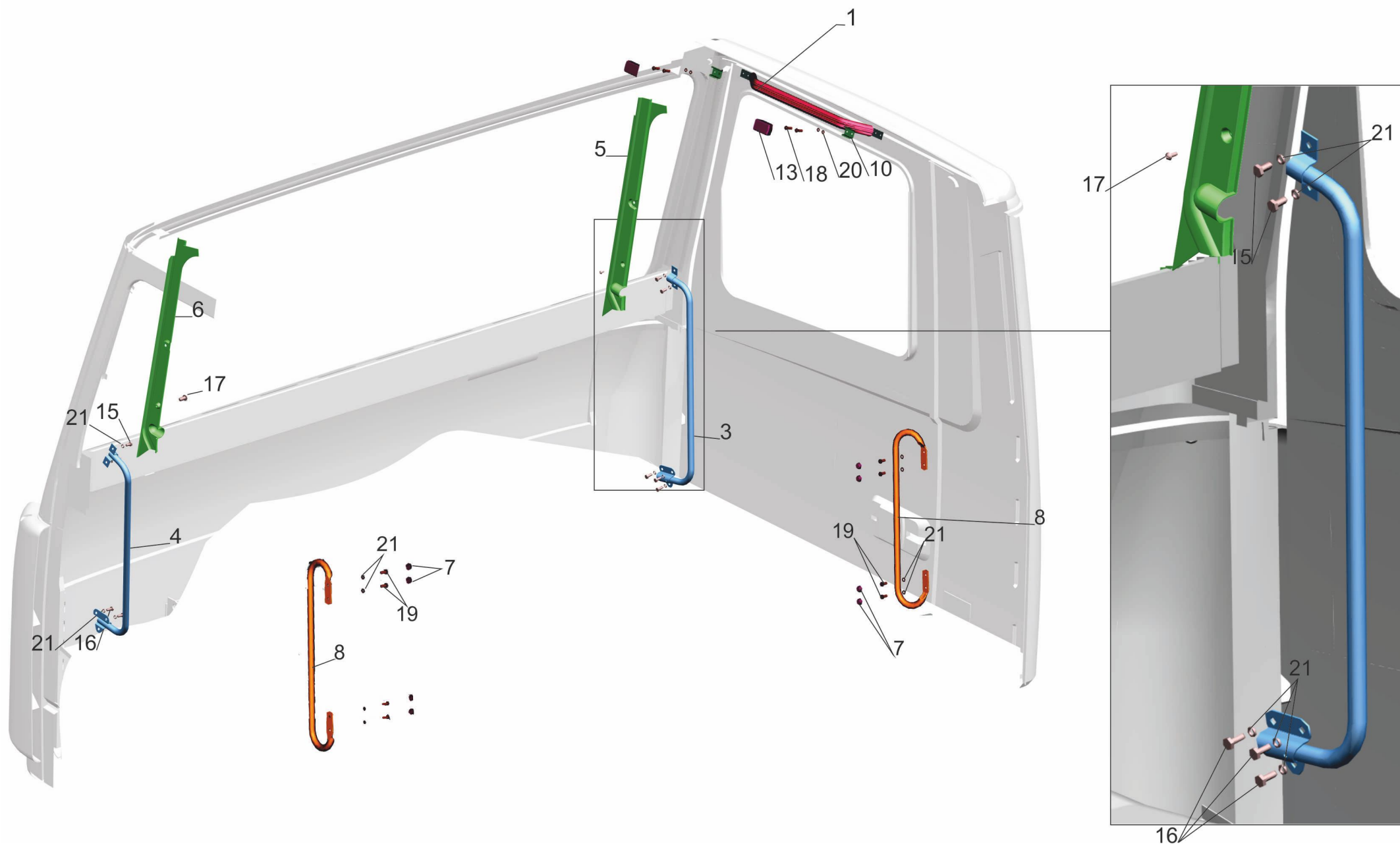
Рис. 256 Установка поручней в кабине 6430-8200030. Fig. 256 Installation of grab handles in cab 6430-8200030.
