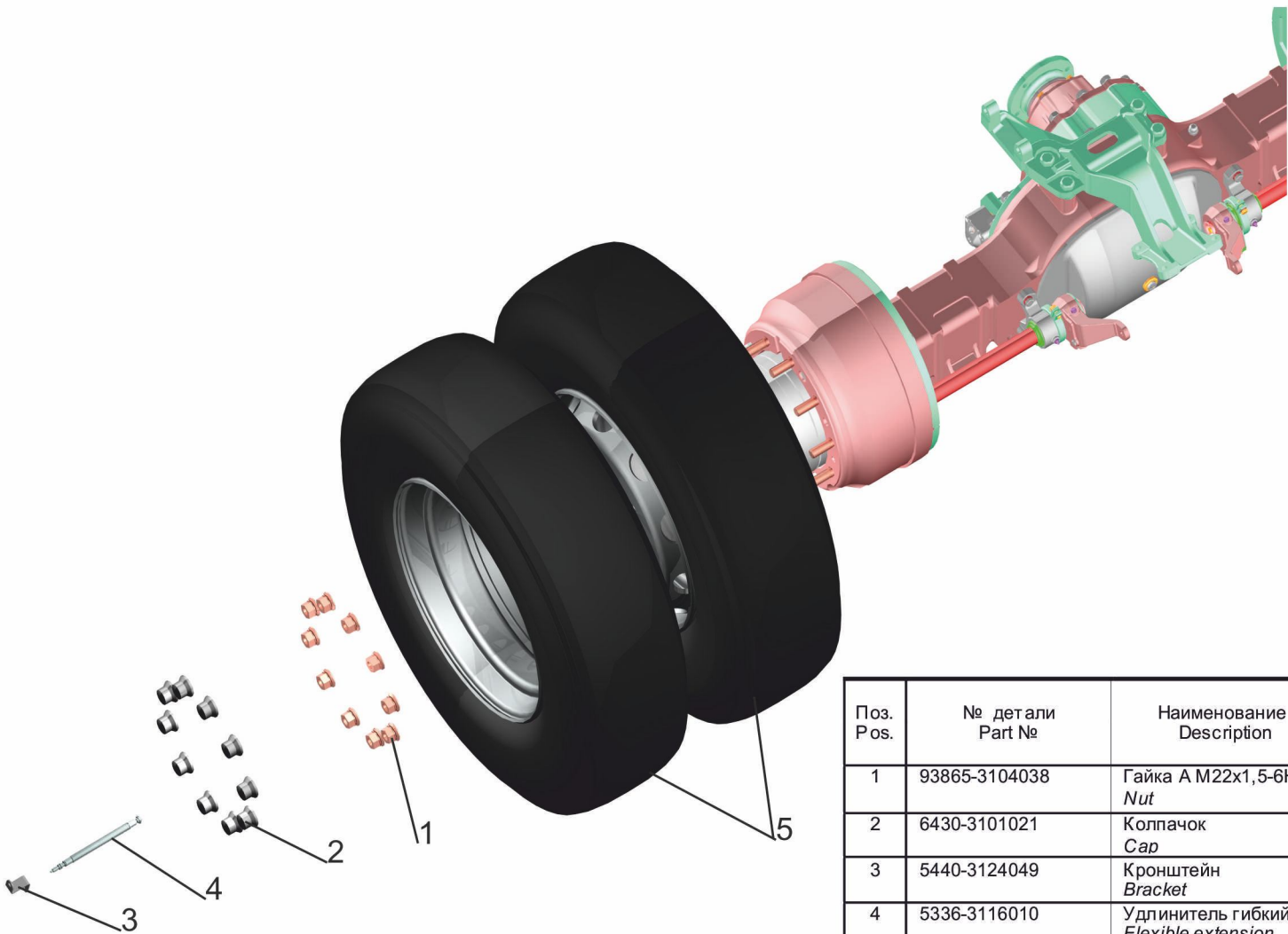
Рис. 138 Установка задних колес Fig. 138 Installation rear wheels
