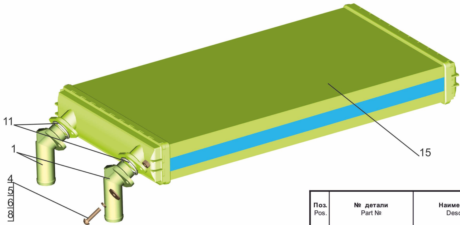
Рис. 282 Радиатор отопителя 631019-8101060 Fig. 282 Radiator of heating 631019-8101060
