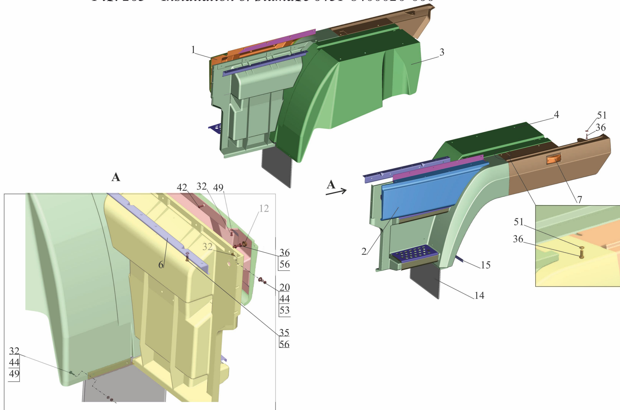
Рис. 263 Установка оперения 6431-8400020-000 Fig. 263 Installation of plumage 6431-8400020-000
