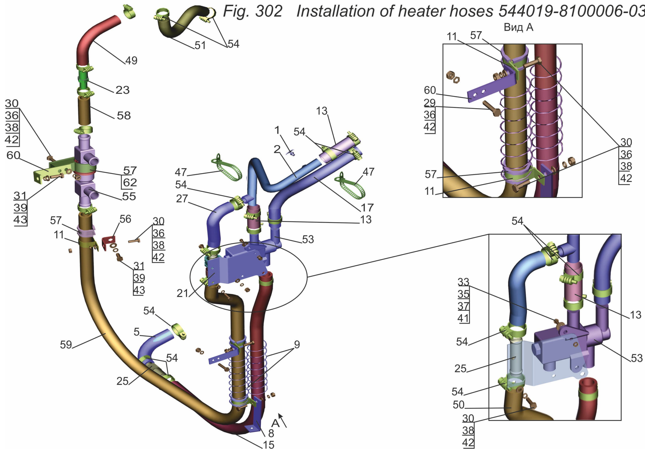
Рис. 302 Установка шлангов отопителя 544019-8100006-030
