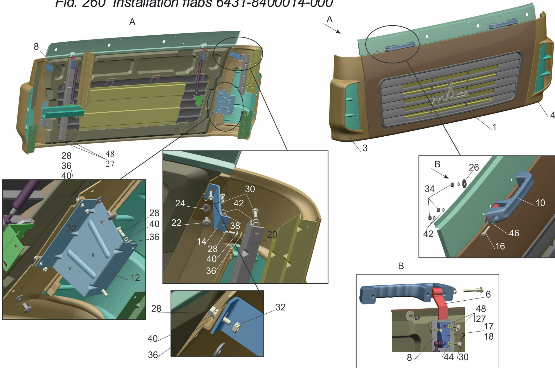
Рис.260 Установка щитков 6431-8400014-000
