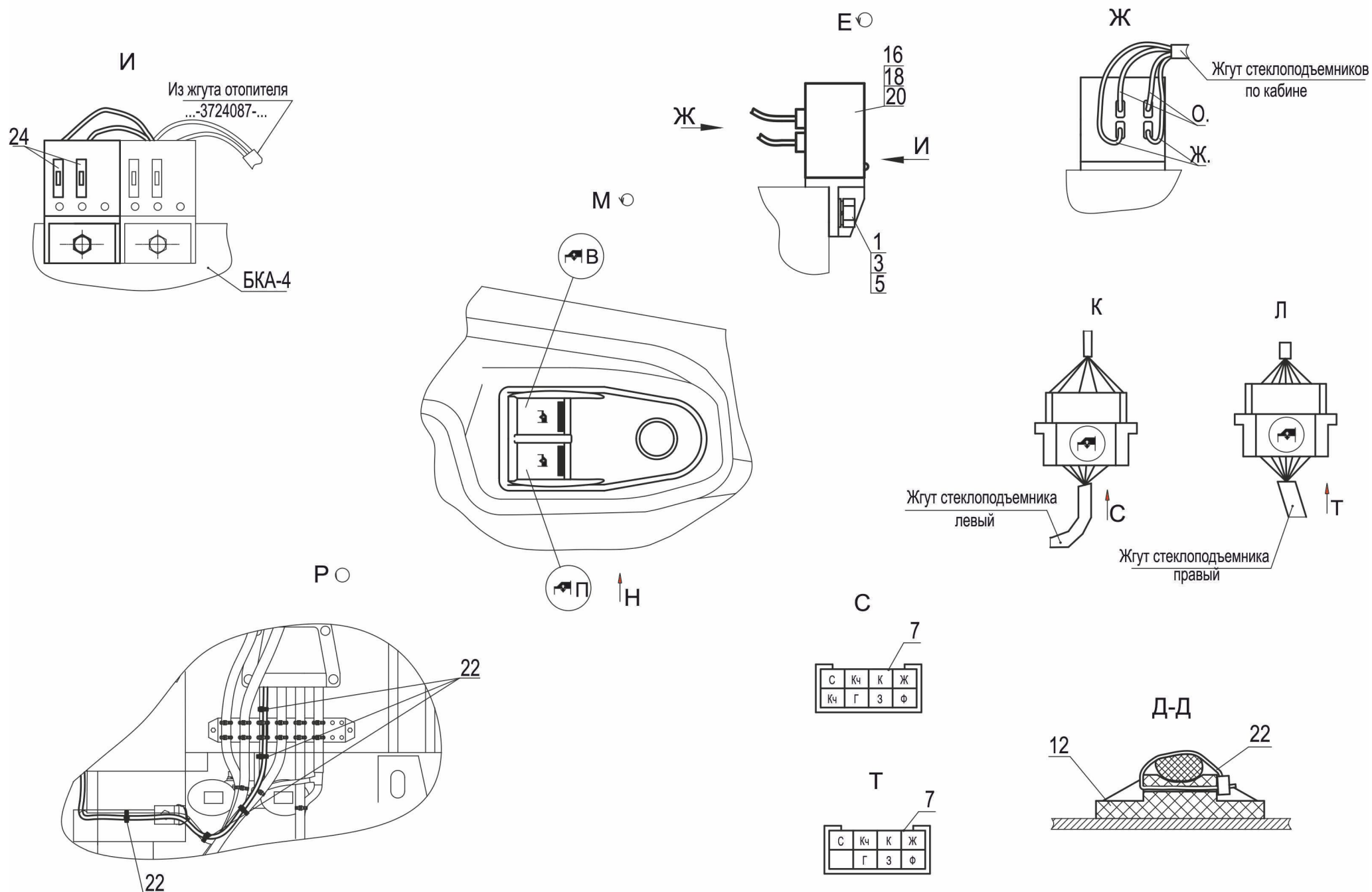
Рис.231 Установка электрооборудования стеклоподъемников Лист 2 Fig.231 Installation of an electric equipment lève-glace Page 2
