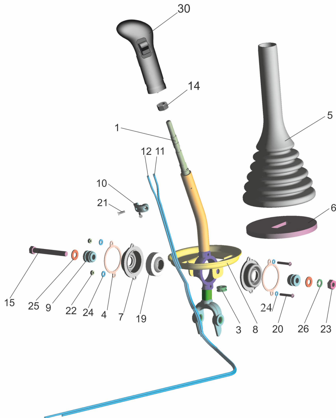
Fig. 45 Lever 64301-1703410-050
