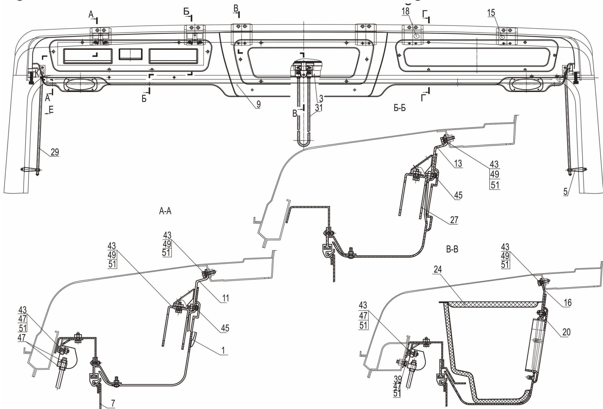
Рис. 258 Установка полки, штор 5440-8200034 Лист 1 Fig. 258 Installation Curtains and sun 5440-8200034 Page 1
