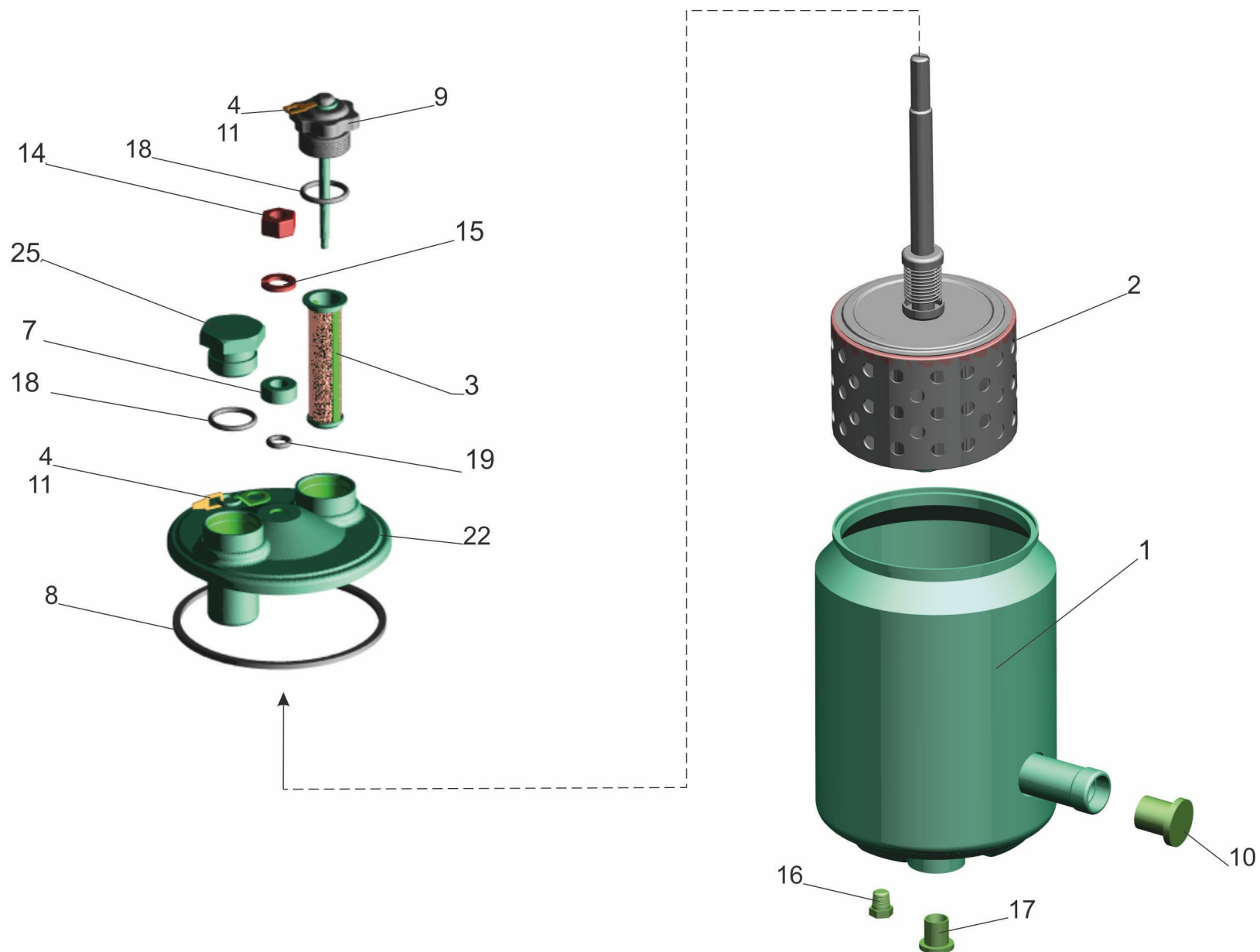
Рис. 146 Бак масляный 5336-3410010-10 Fig. 146 Oil tank 5336-3410010-10
