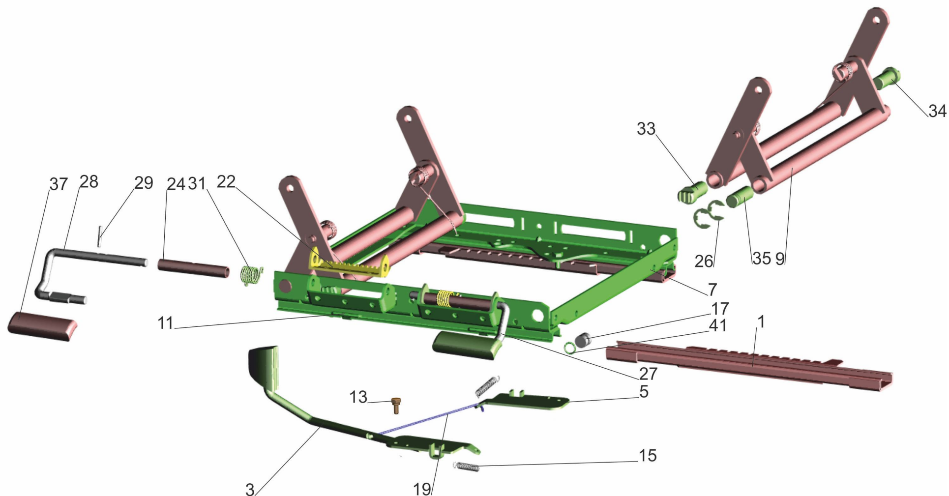
Рис. 249 Механизм регулирования высоты 6430-6804100-010 Fig. 249 Adjusting mechanisms of seat height 6430-6804100-010
