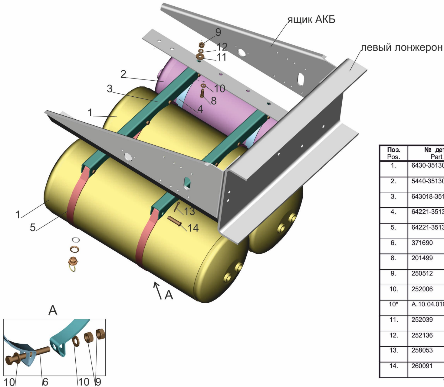
Рис. 167 Установка ресиверов 643018-3513004 Fig. 167 Installation of receivers 643018-3513004
