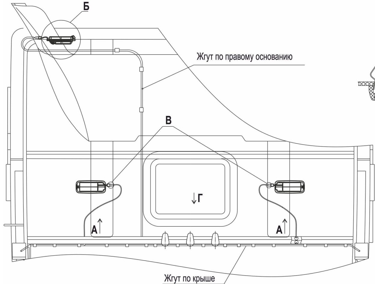
Рис. 190 Установка светильников в кабине 544008-3700136 Fig.190 Installation of fixtures in a cabin 544008-3700136
