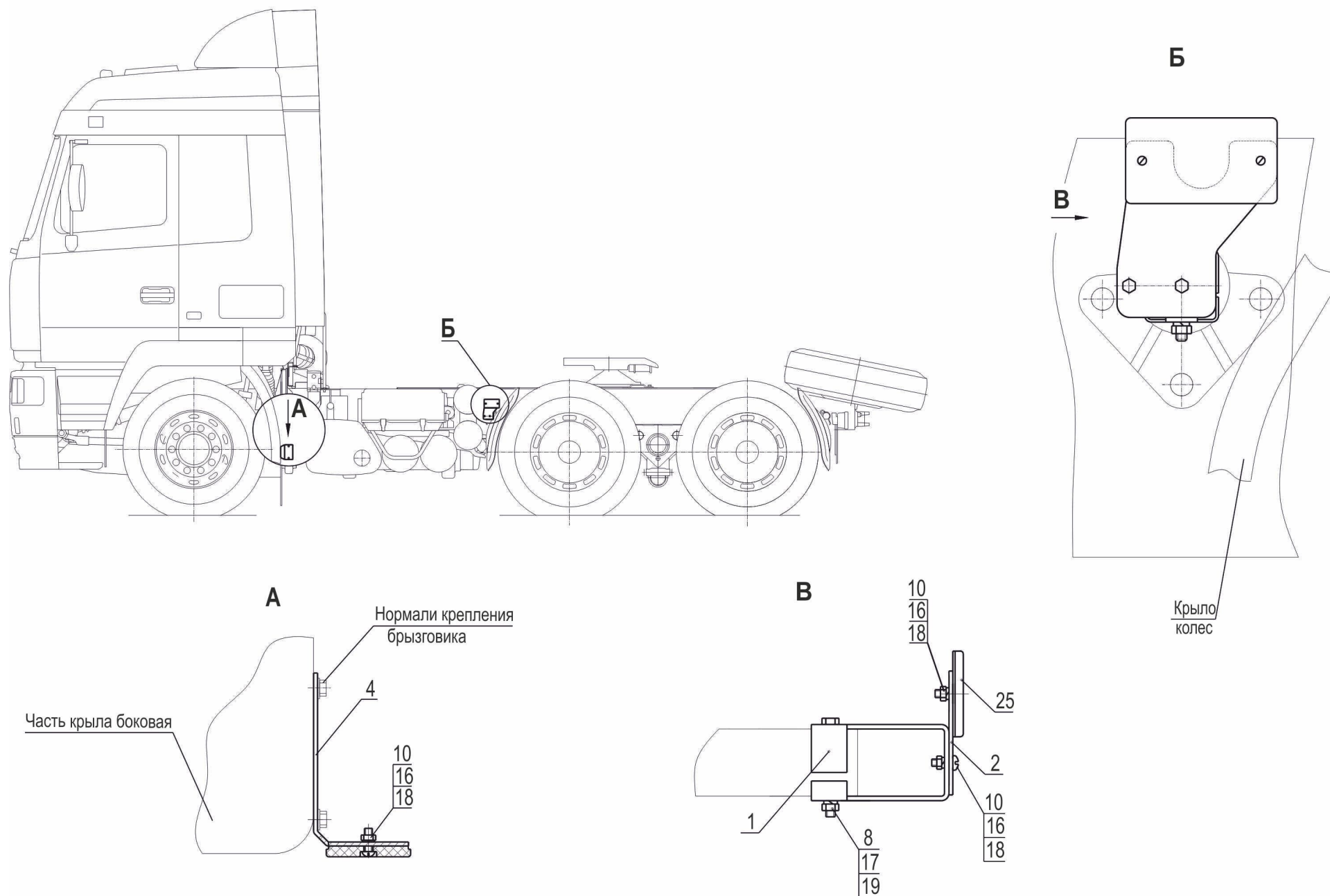
Рис. 197 Установка световозвратателей 643008-3700079 Fig. 197 Setting of retro-reflectors 643008-3700079
