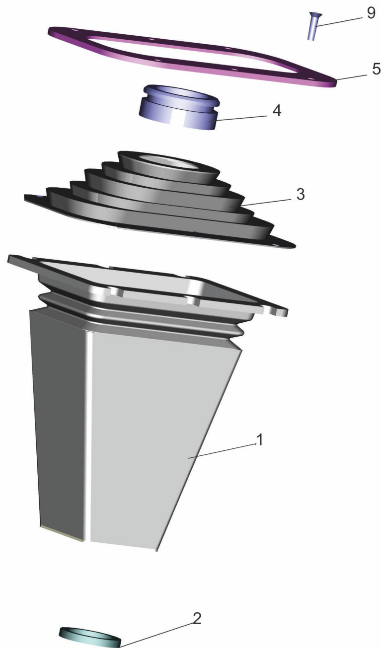
Рис.164 Уплотнение люка кабины 5440-3444256-010 Fig. 164 Sealing hatch of cabin 5440-3444256-010
