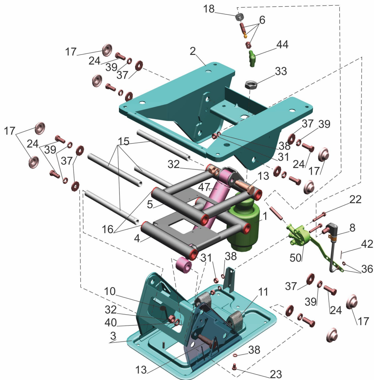
Рис. 244 Подставка сиденья с пневмооборудованием 6430-6807006-010 Fig. 244 Seat support with pneumatic equipment 6430-6807006-010
