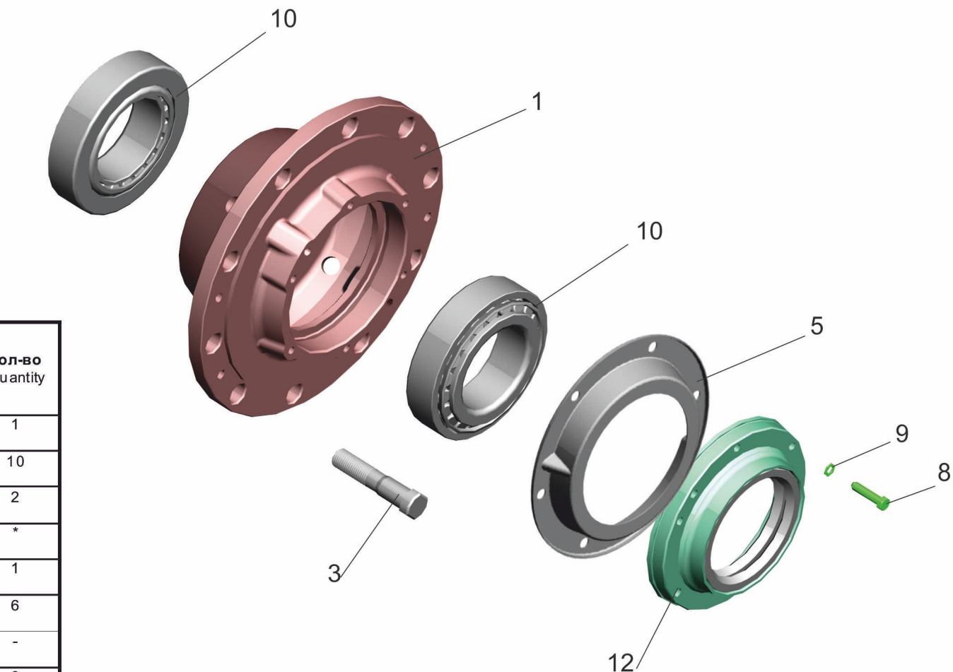
Рис.78 Ступица с крышкой 544019-3104006-010 Fig.78 Rear with cover 544019-3104006-010
