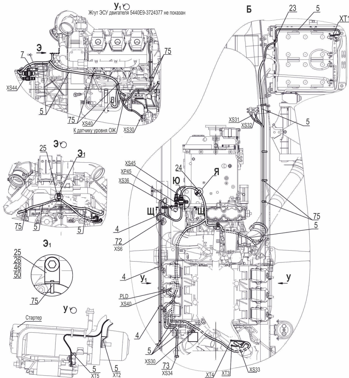
Рис. 216 Установка электрооборудования ЭСУ двигателя 544018-3800060, (-010) (лист 3) Fig. 216 Installation of electronic control system of the engine 544018-3800060, (-010) (page 3)
