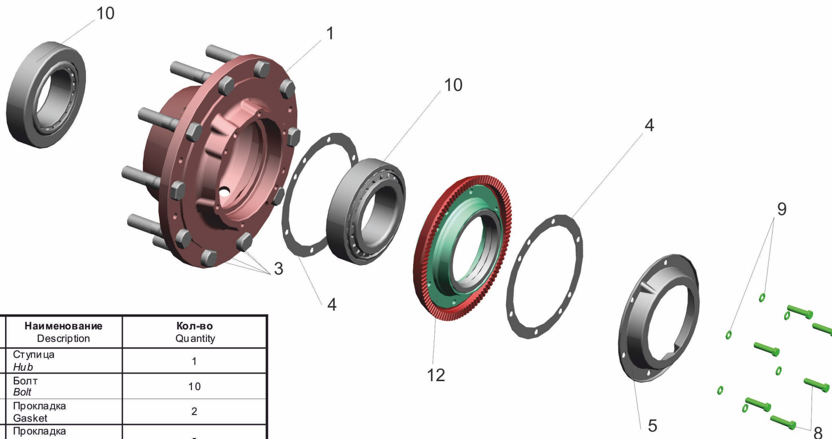
Рис.61 Ступица с крышкой 543266-3104006-600 Fig.61 Rear axle hub
