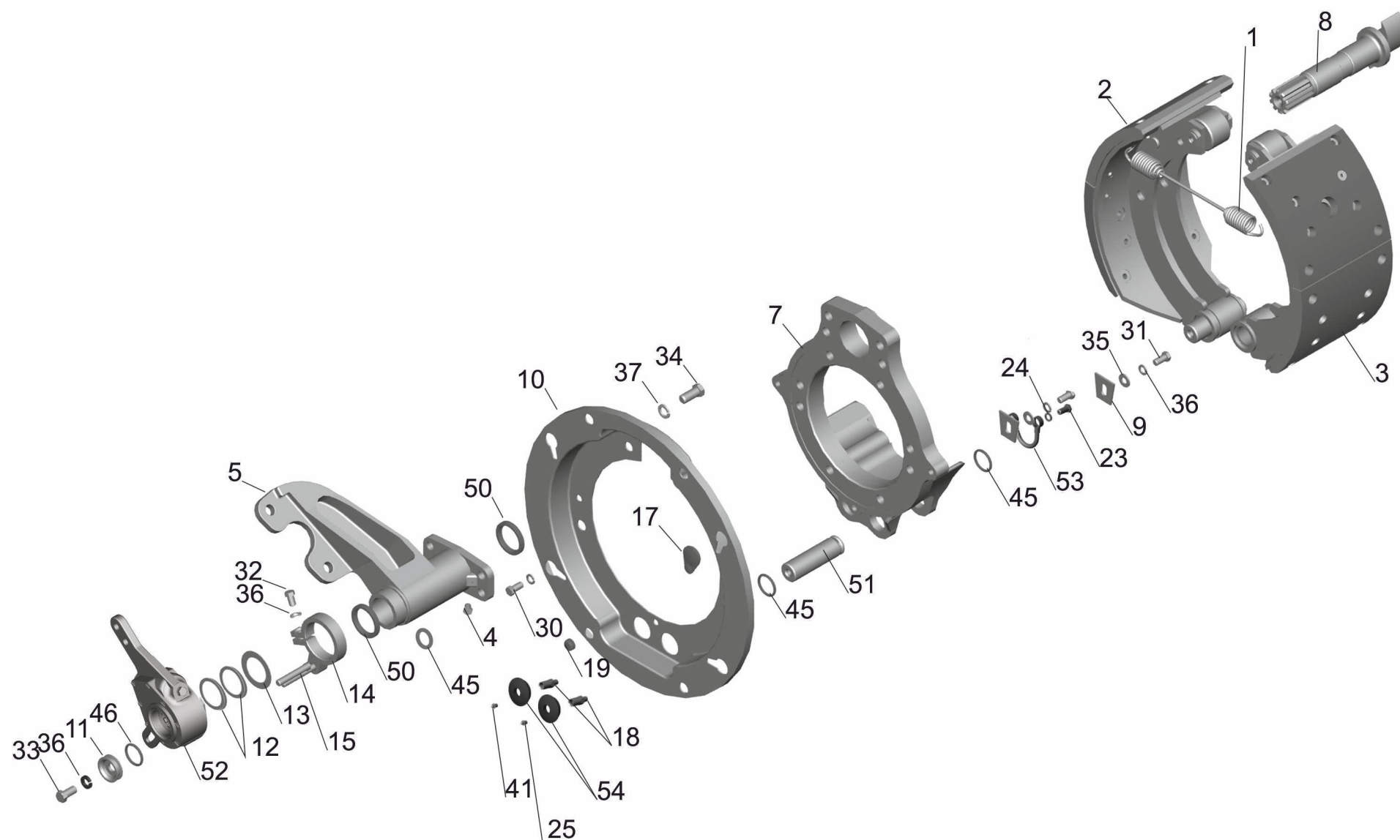
Рис. 133 Тормоз передний 5440-3501004 (5440-3501005) Fig. 133 Front brake 5440-3501004 (5440-3501005)
