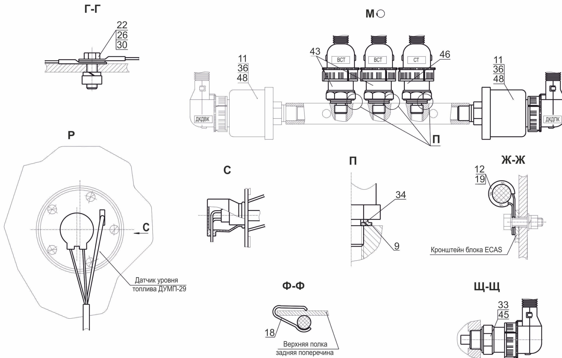
Рис. 186 Установка электрооборудования на шасси 643018-3700010-090, (-790) (лист 2) Fig. 186 Installation of electrical equipment on the chassis 643018-3700010-090, (-790) (page 2)
