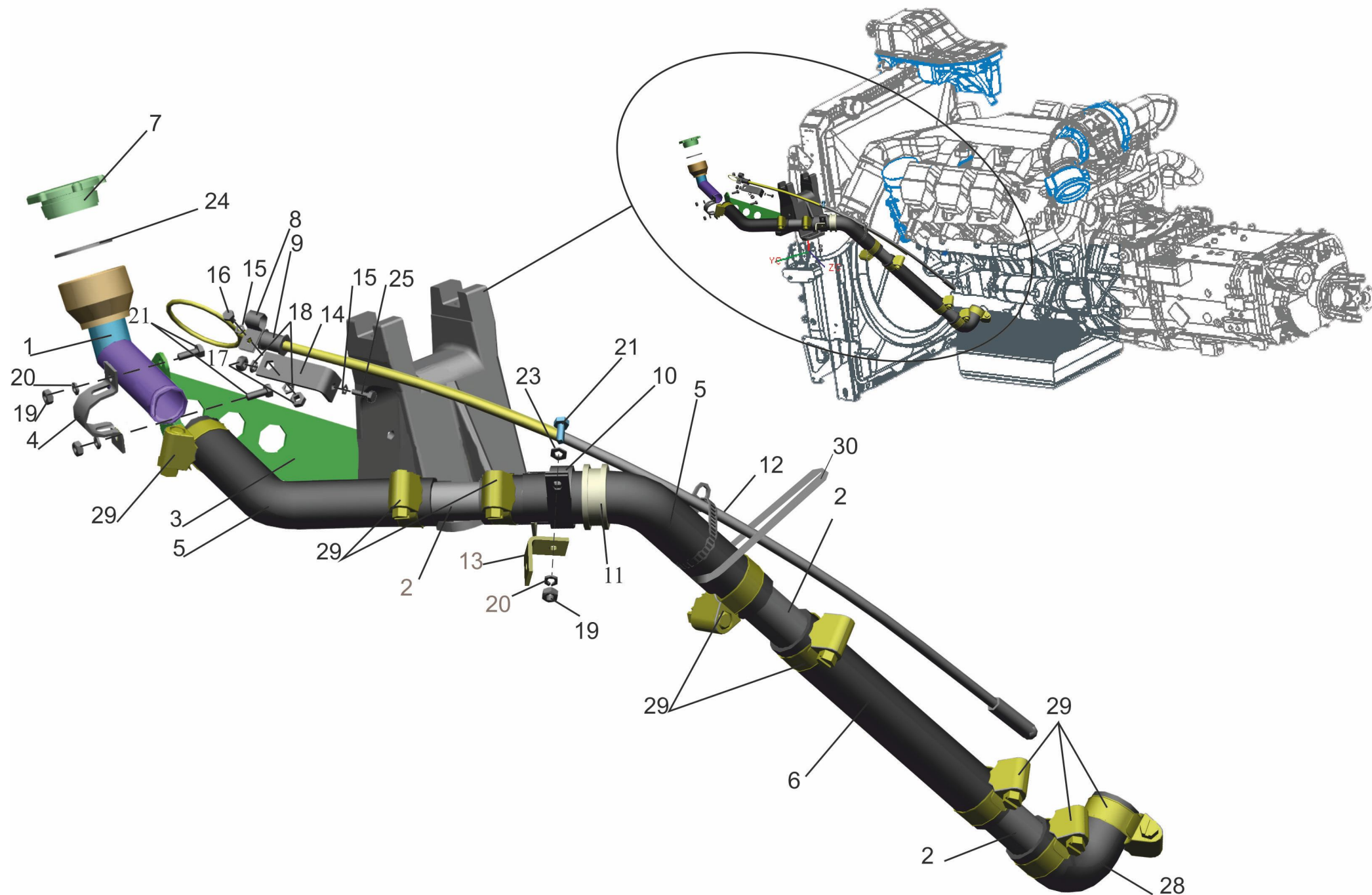
Рис. 4 Установка системы заливки и контроля уровня масла 544019-1018002 Fig. 4 Installation of system of oil priming and its level checking 544019-1018002
