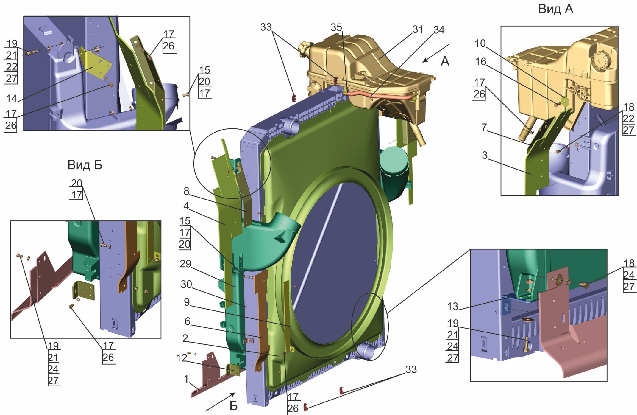
Рис. 30 Радиатор с кожухом 544019-1301009 Fig. 30 Cooler with housing 544019-1301009
