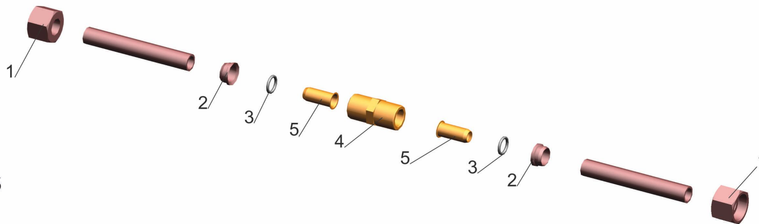
Рис.181 Соединение для ремонта поврежденных трубопроводов Fig.181 Connection for repair of the damaged pipelines
