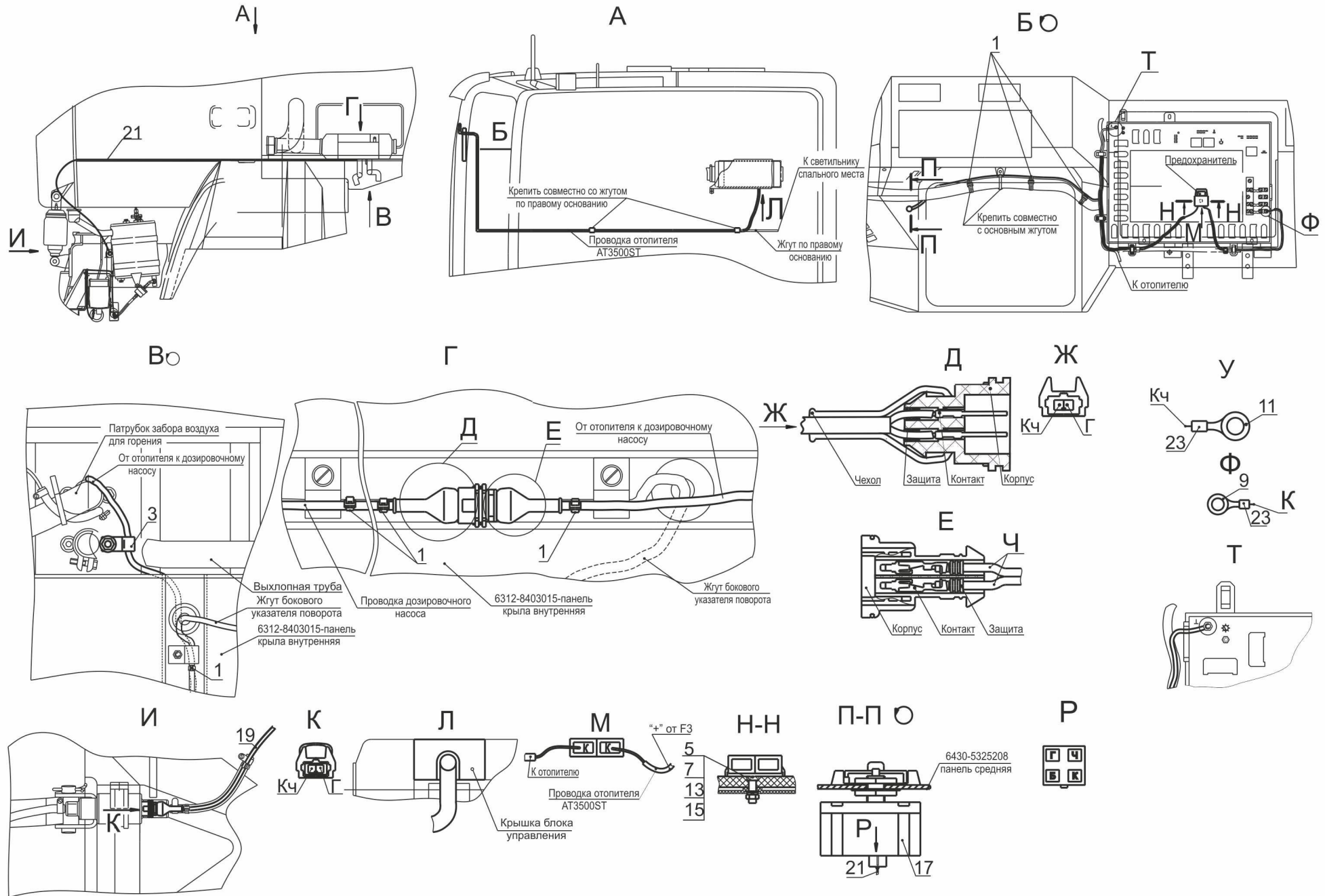
Рис. 295 Установка электрооборудования независимого отопителя 6430-3700088-010 Fig. 295 Setting of an electrical equipment of an independent heater 6430-3700088-010
