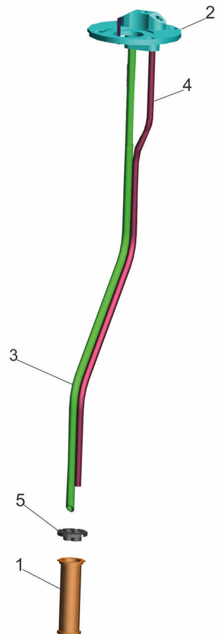
Рис. 18 Топливозаборник 5440В9-1105014 Fig. 18 Fuel intake 5440В9-1105014
