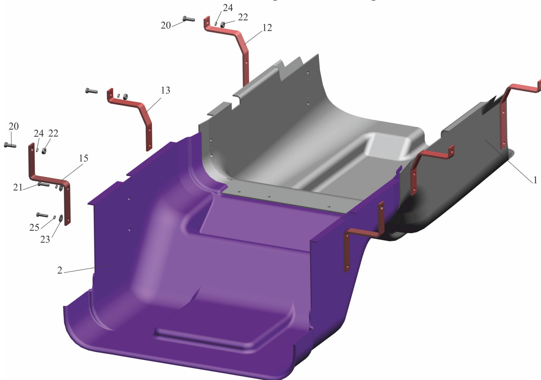
Рис.14 Установка шумоизоляционных экранов Fig.14 Mounting noise isolation screens
