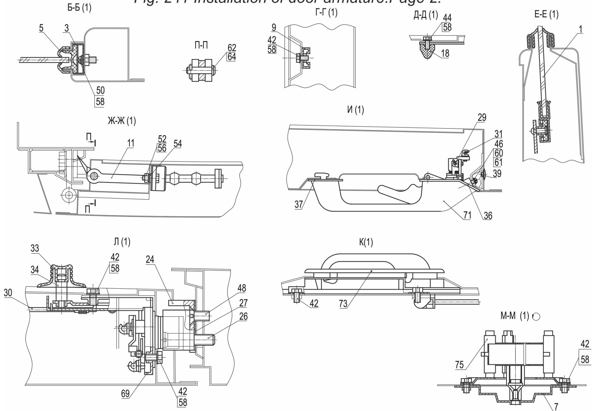
Рис. 241 Установка дверной арматуры Лист 2. Fig. 241 Installation of door armature. Page 2.
