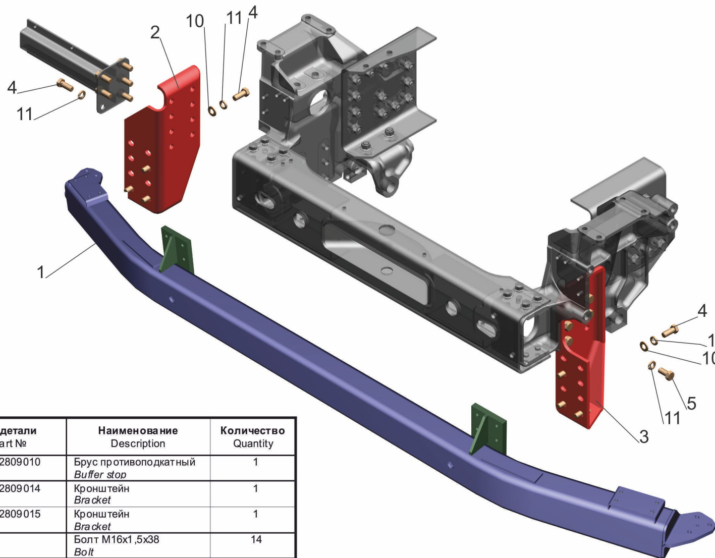
Рис. 106 Установка переднего противоподкатного бруса 643018-2800030-010 Fig. 106 Installation of front buffer stop 643018-2800030-010
