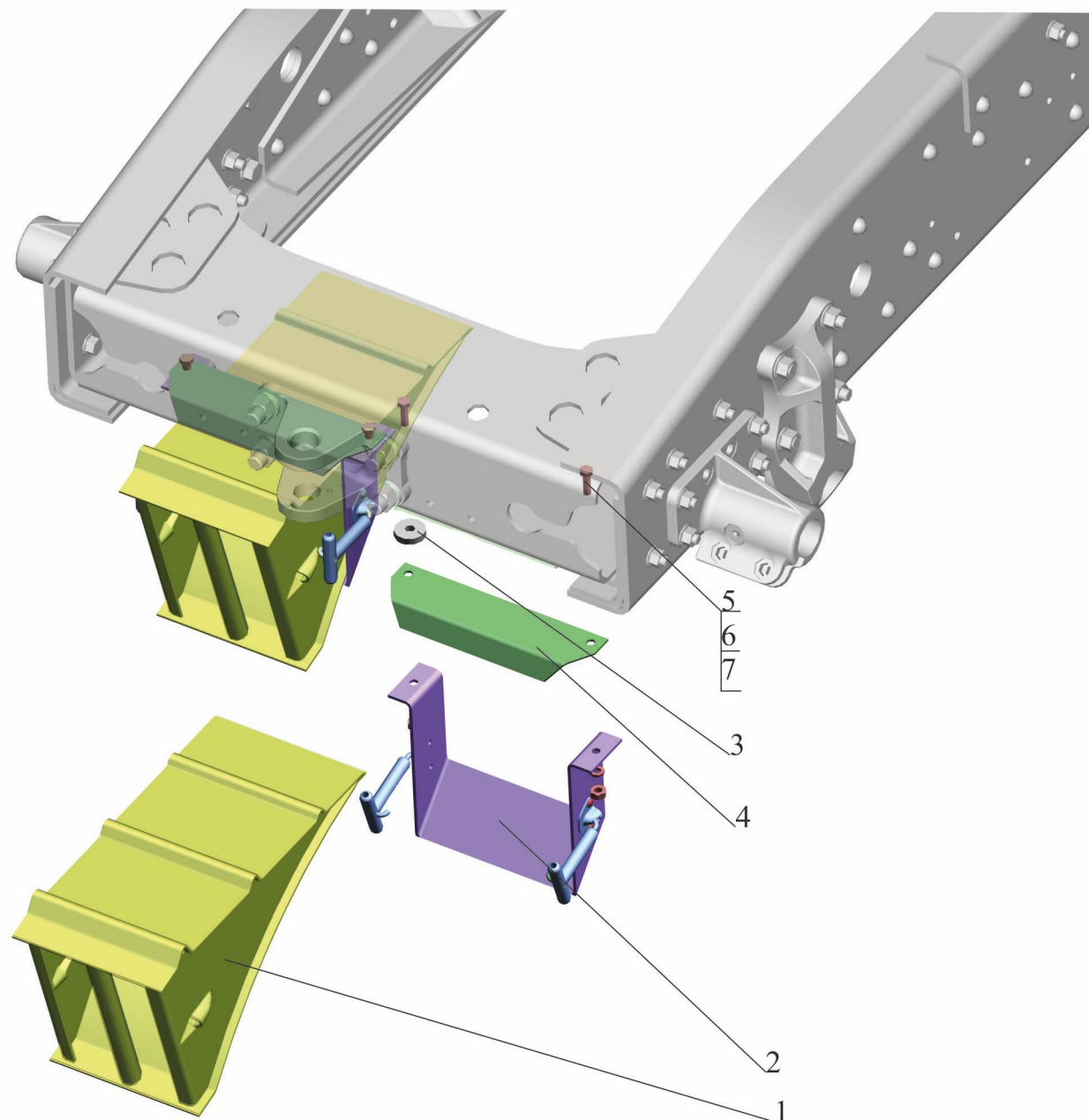
Рис. 217 Установка противооткатных упоров 643018-3900037 Fig. 217 Installation of buffer stops 643018-3900037
