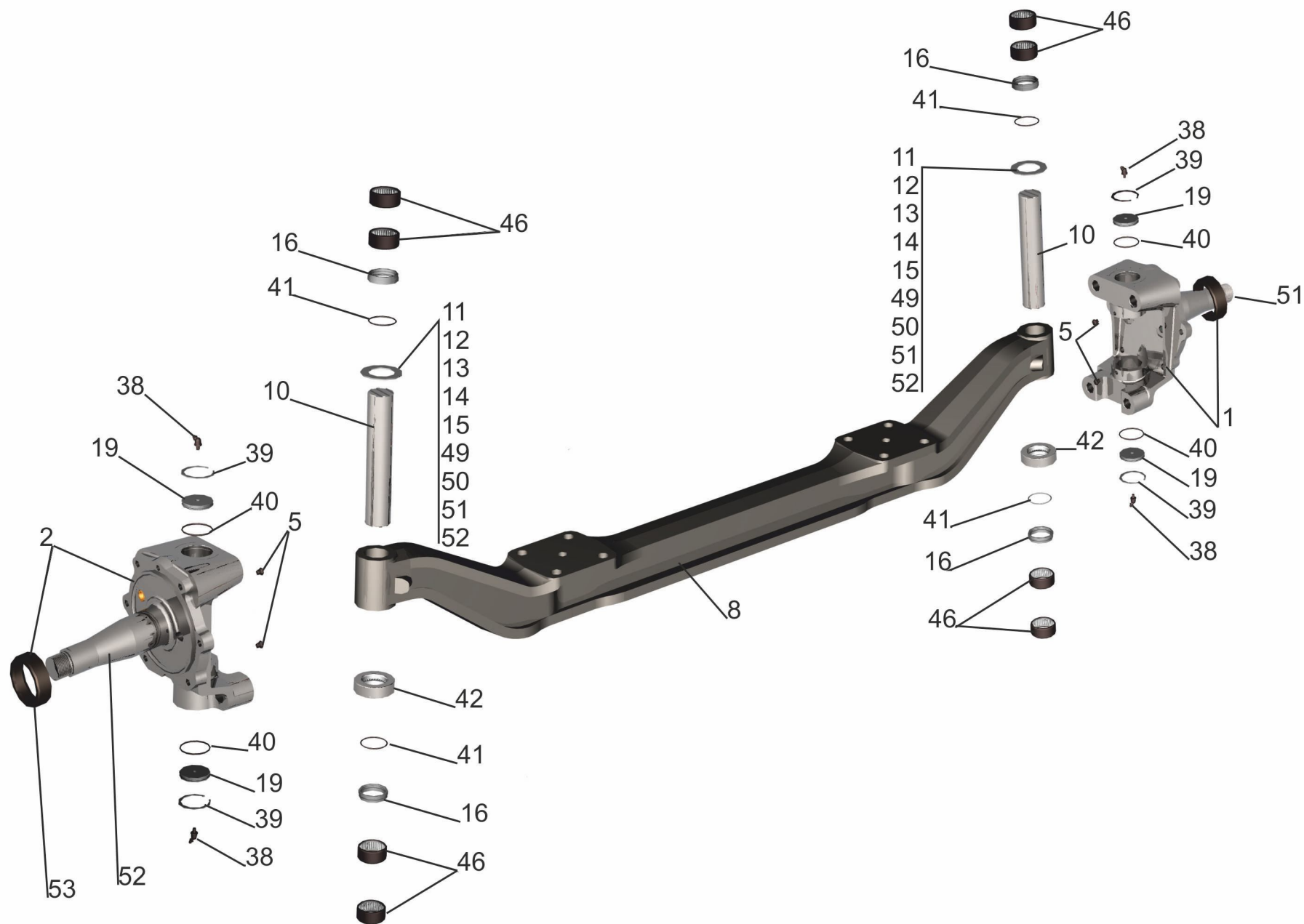
Рис. 124 Передняя ось 544019-3000015 (лист 2) Fig. 124 Front axle 544019-3000015 (page 2)
