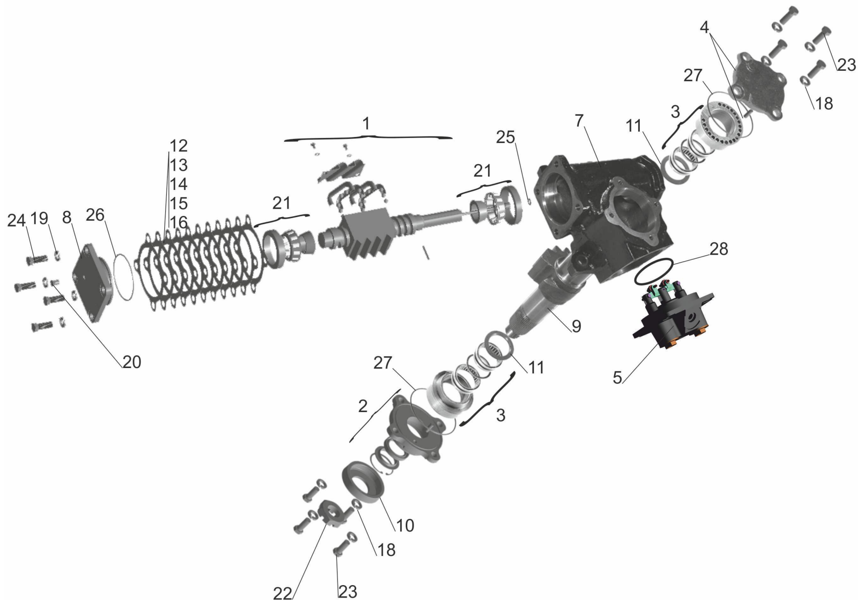
Рис. 145 Механизм рулевой 64221-3401005-10 Fig. 145 Steering mechanism 64221-3401005-10
