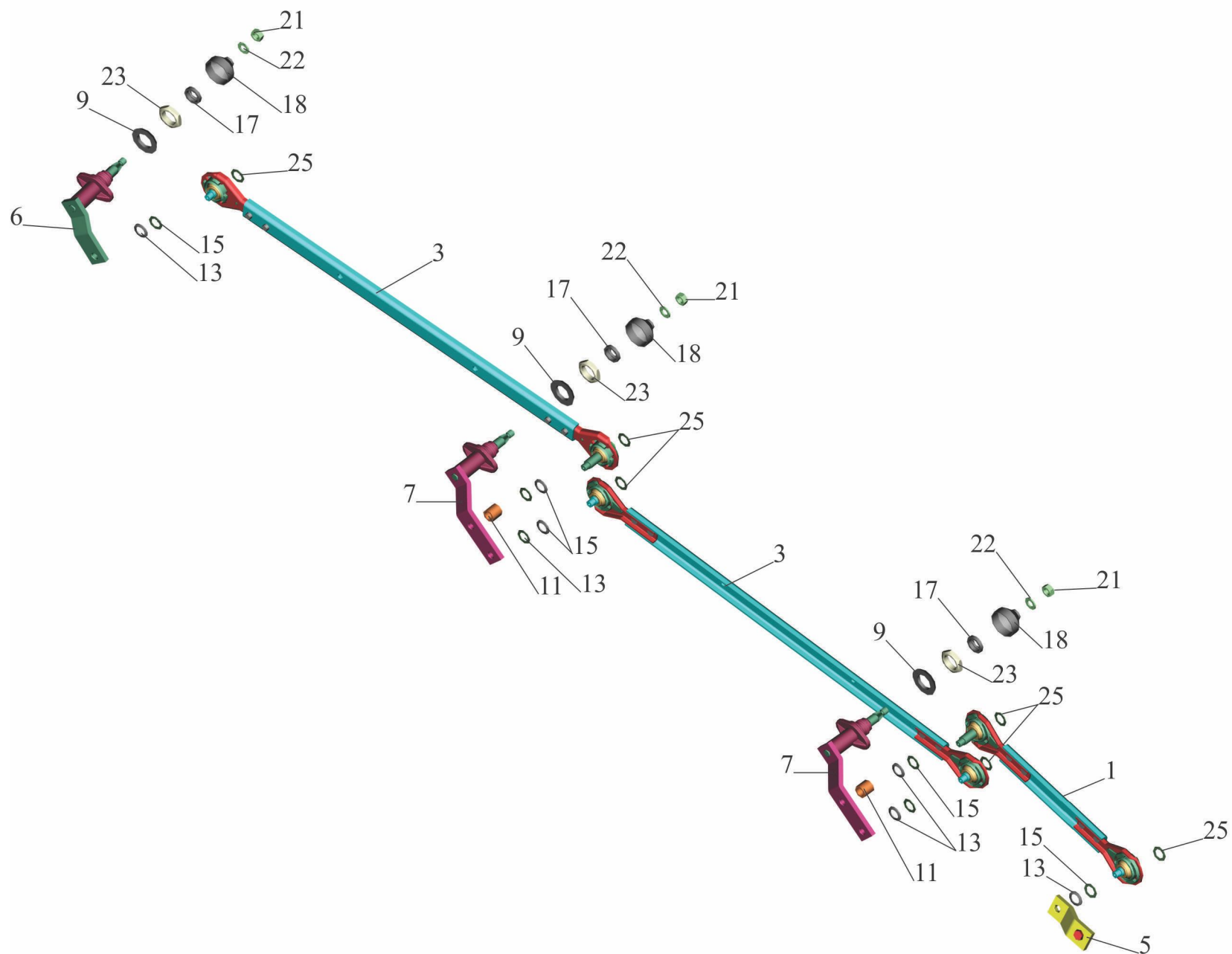
Рис. 230 Привод стеклоочистителя 6430-5205500-010 Fig. 230 Drive of cleaner of glasses 6430-5205500-010
