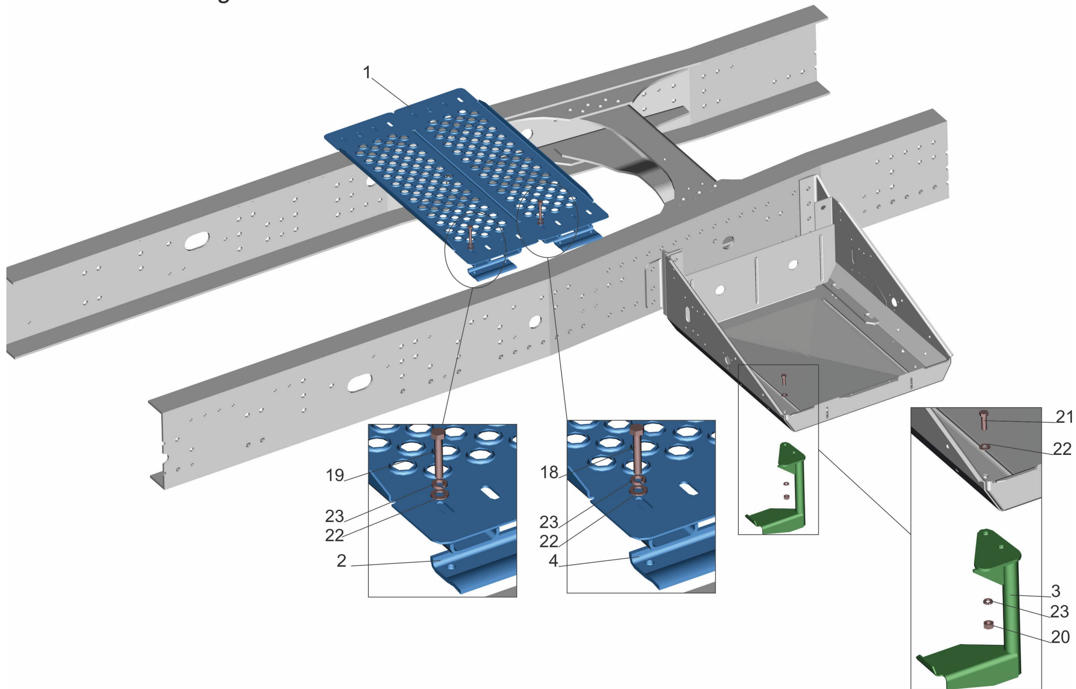
Рис. 105 Установка площадки шасси и подножки 643018-2800026 Fig. 105 Installation Platform the chassis and sideboard 643018-2800026
