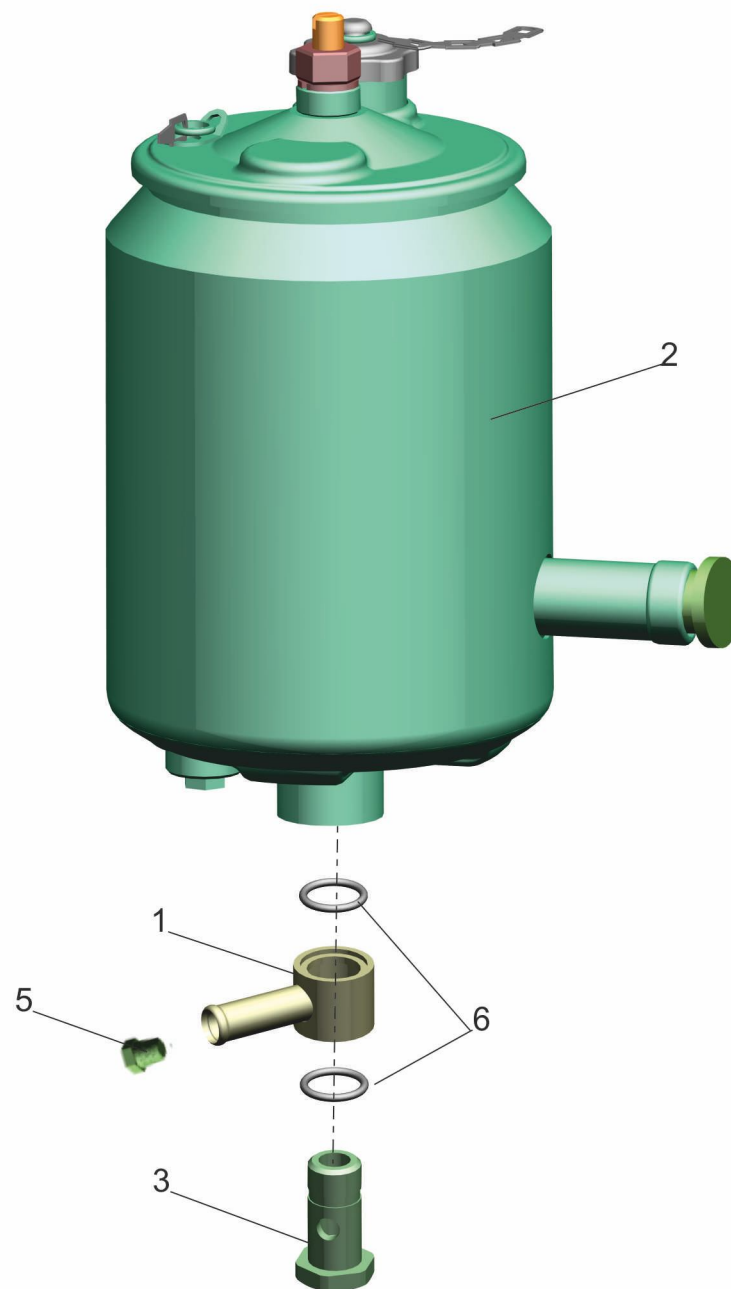
Рис. 156 Бак масляный 64221-3410008 Fig. 156 Oil tank 64221-3410008
