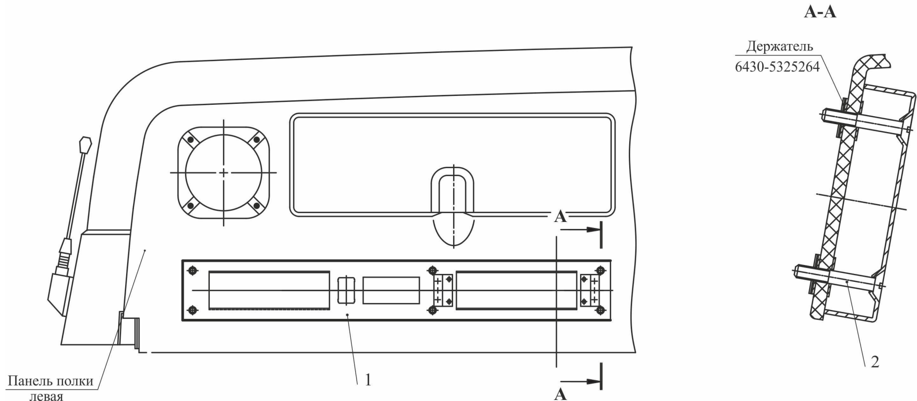
Рис. 211 Установка панели на полке 544019-7901080 Fig. 211 Panel installation on shelf 544019-7901080
