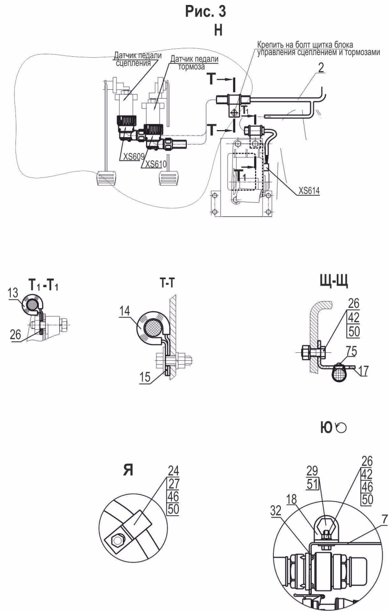
Рис. 216 Установка электрооборудования ЭСУ двигателя 544018-3800060, (-010) (лист 3) Fig. 216 Installation of electronic control system of the engine 544018-3800060, (-010) (page 3)
