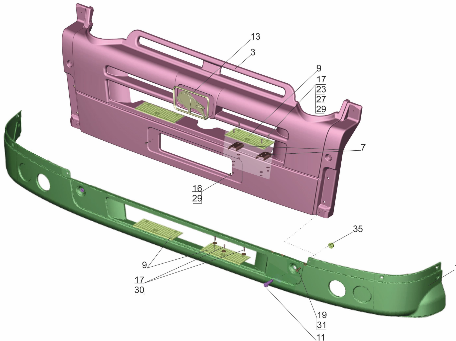
Рис.98 Бампер передний 643019-2803010 Fig. 98 Bumper 643019-2803010
