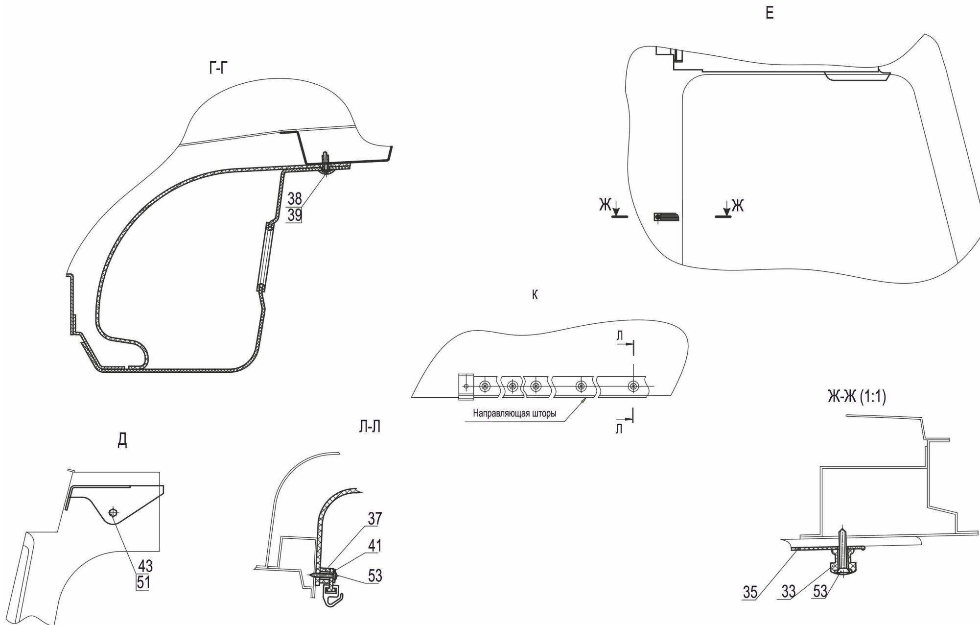
Рис. 257 Установка полки, штор 5440-8200034-010 Лист 2 Fig. 257 Installation Curtains and sun 5440-8200034-010 Page 2
