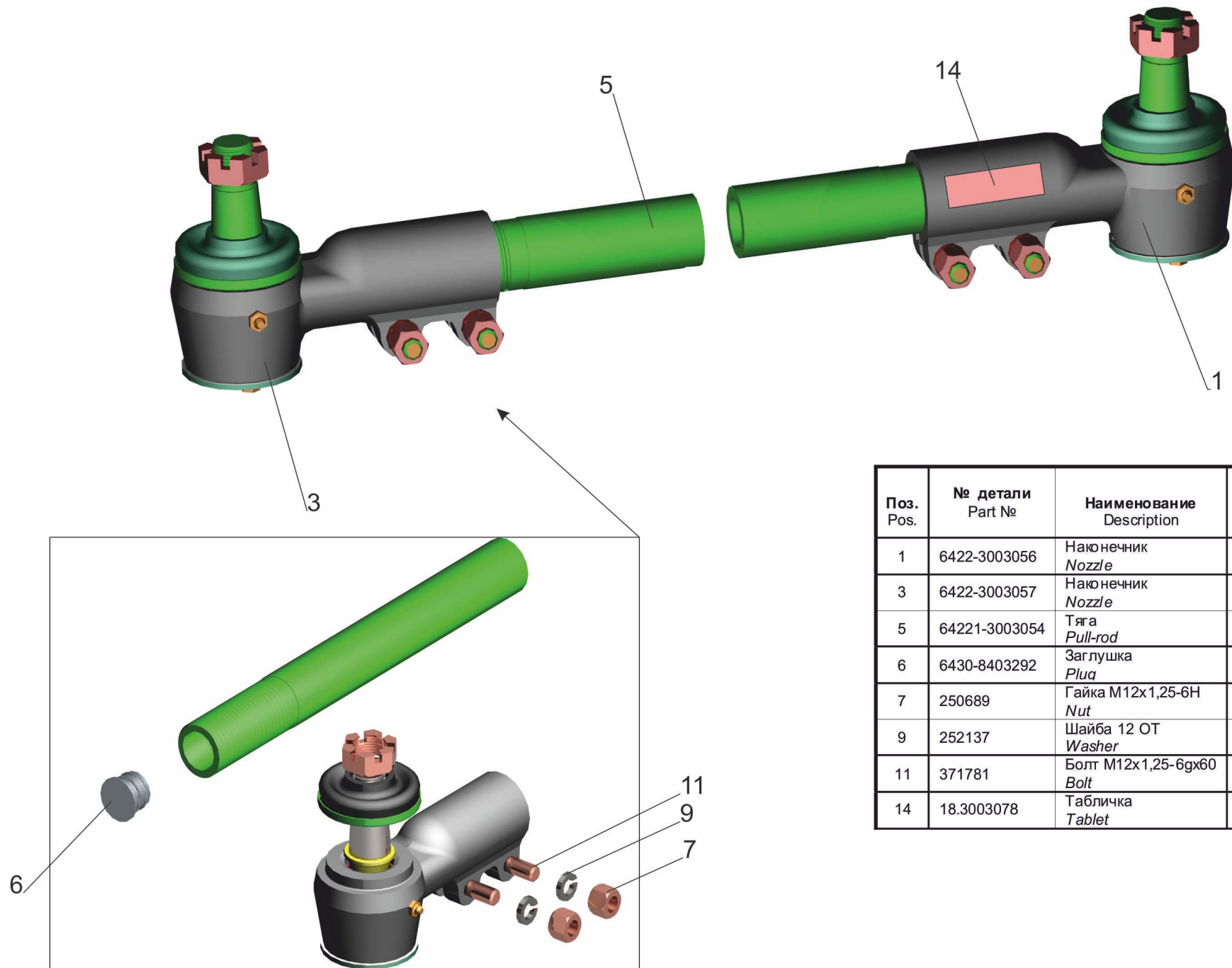
Рис.126 Тяга поперечная 64221-3003052 Fig. 126 Pull-rod cross 64221-3003052
