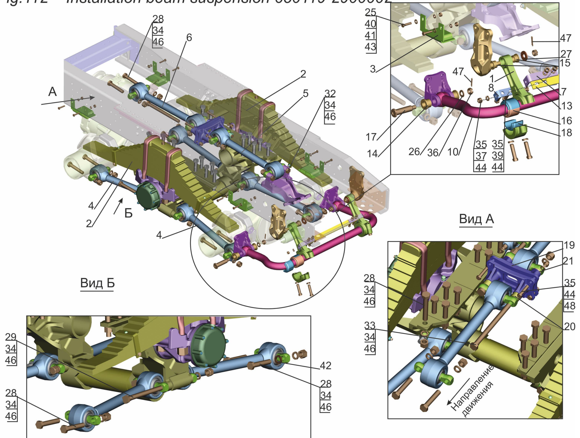
Рис.112 Установка подвески задней 650119-2900002 Fig.112 Installation beam suspension 650119-2900002
