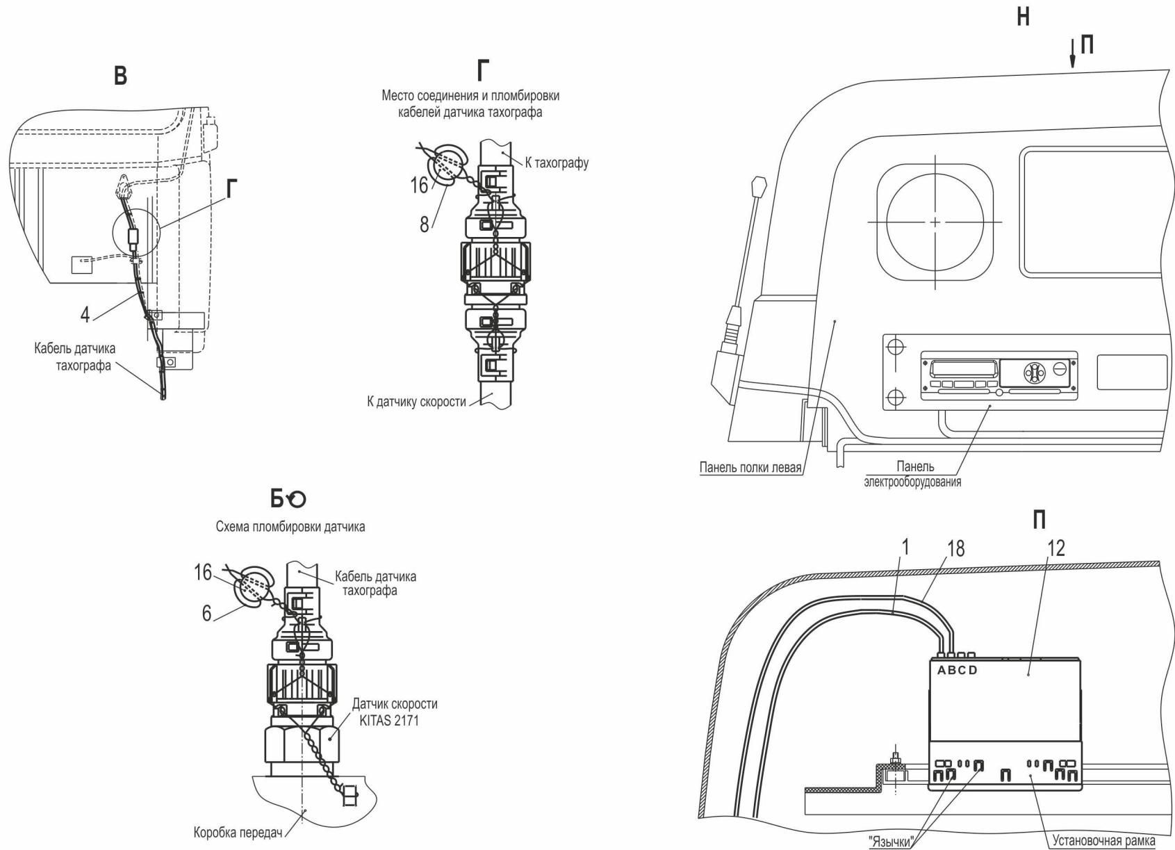
Рис. 209 Установка и пломбировка тахографа 544069-3800005 (лист 2) Fig.209 Installation and identification seal of tachograph 544069-3800005 (page 2)
