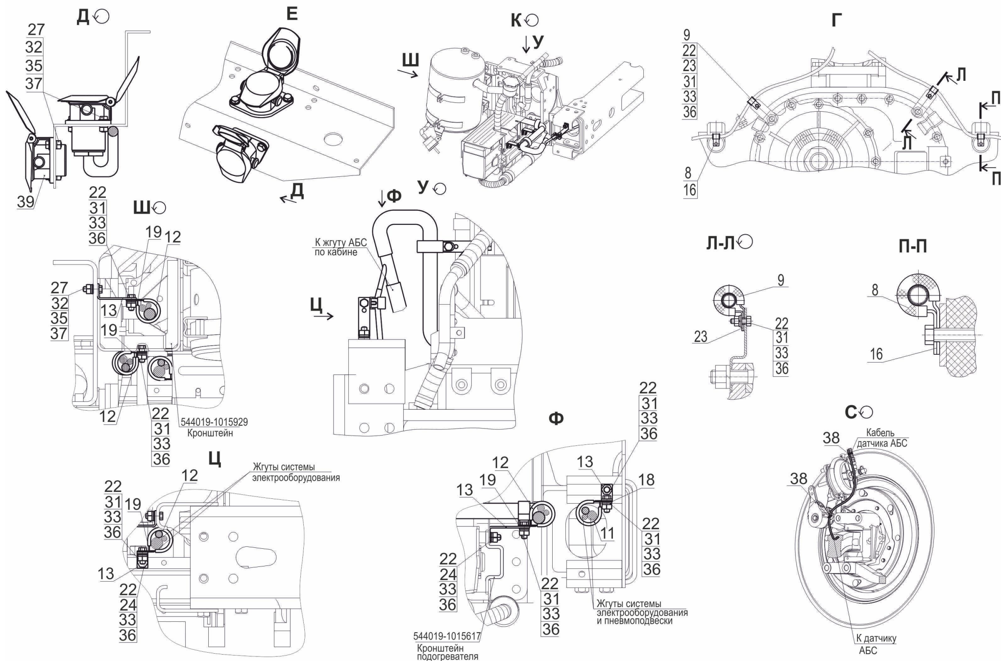
Рис. 213 Установка электрооборудования АБС тормозов 643018-3800040 (лист 2) Fig. 213 Setting of electrical equipment ABS brakes 643018-3800040 (page 2)
