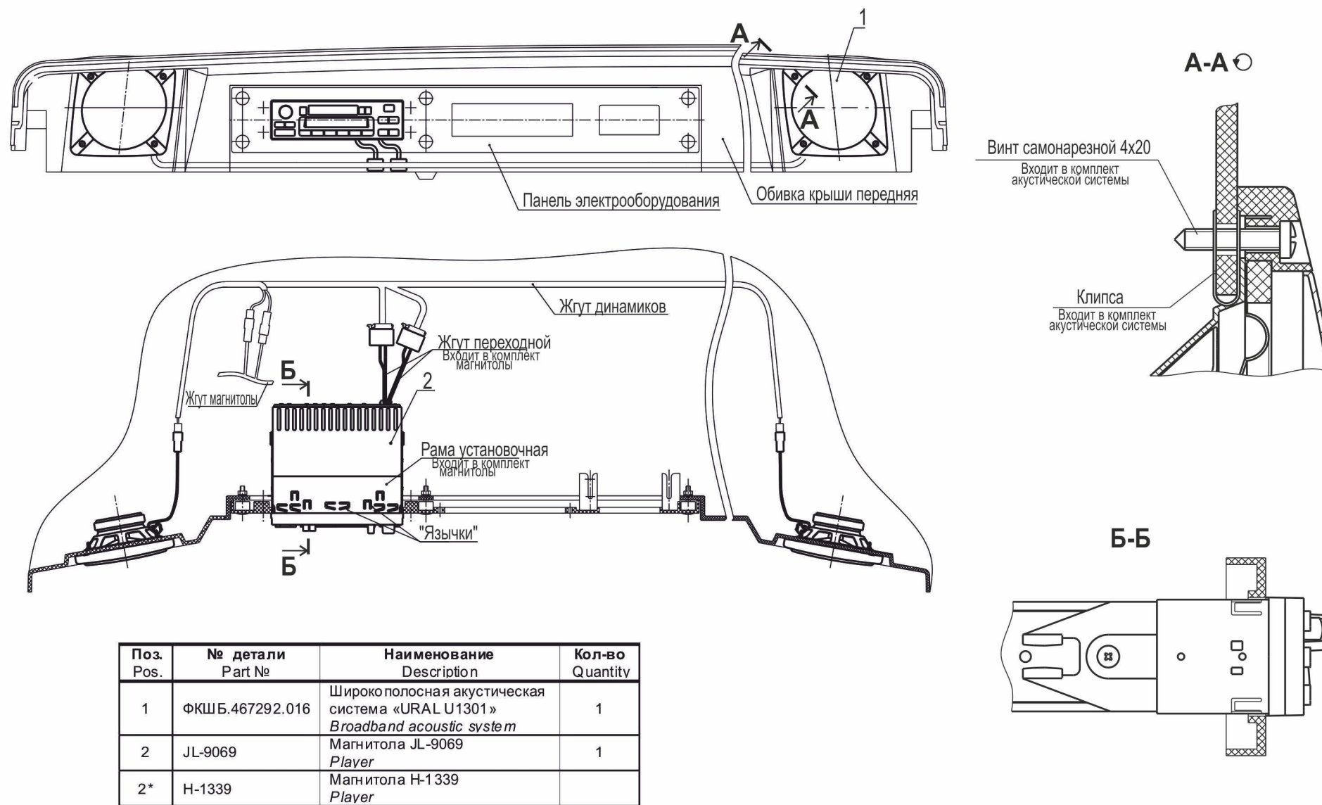
Рис. 210 Установка радиоприемника с CD проигрывателем 6501-7900030 Fig. 210 Installation of receiver with CD player 6501-7900030
