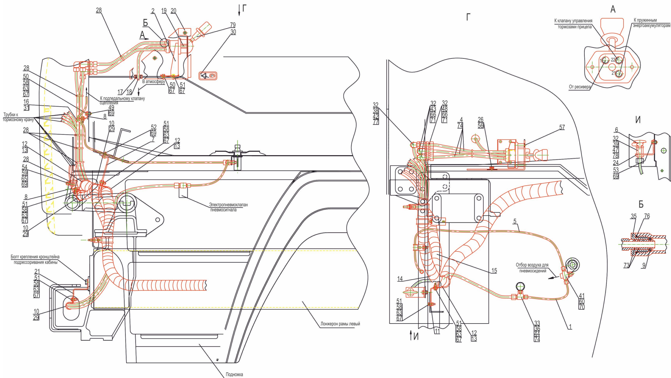
Рис. 179 Привод стояночного тормоза 544019-3537006 Fig. 179 Drive of a parking brake 544019-3537006
