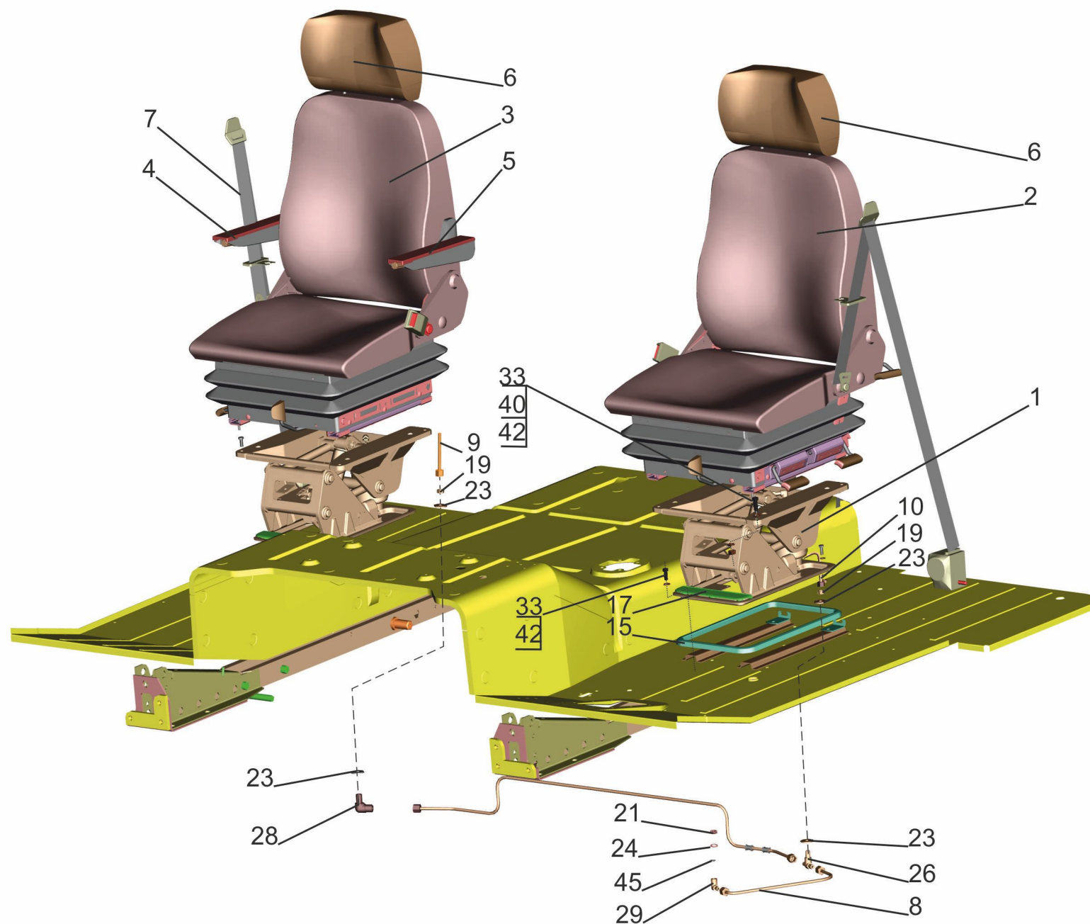
Рис. 243 Установка и пневмопитание сидений 6430-6800006-001 Fig. 243 Installation and pneumatic supply of seat 6430-6800006-001
