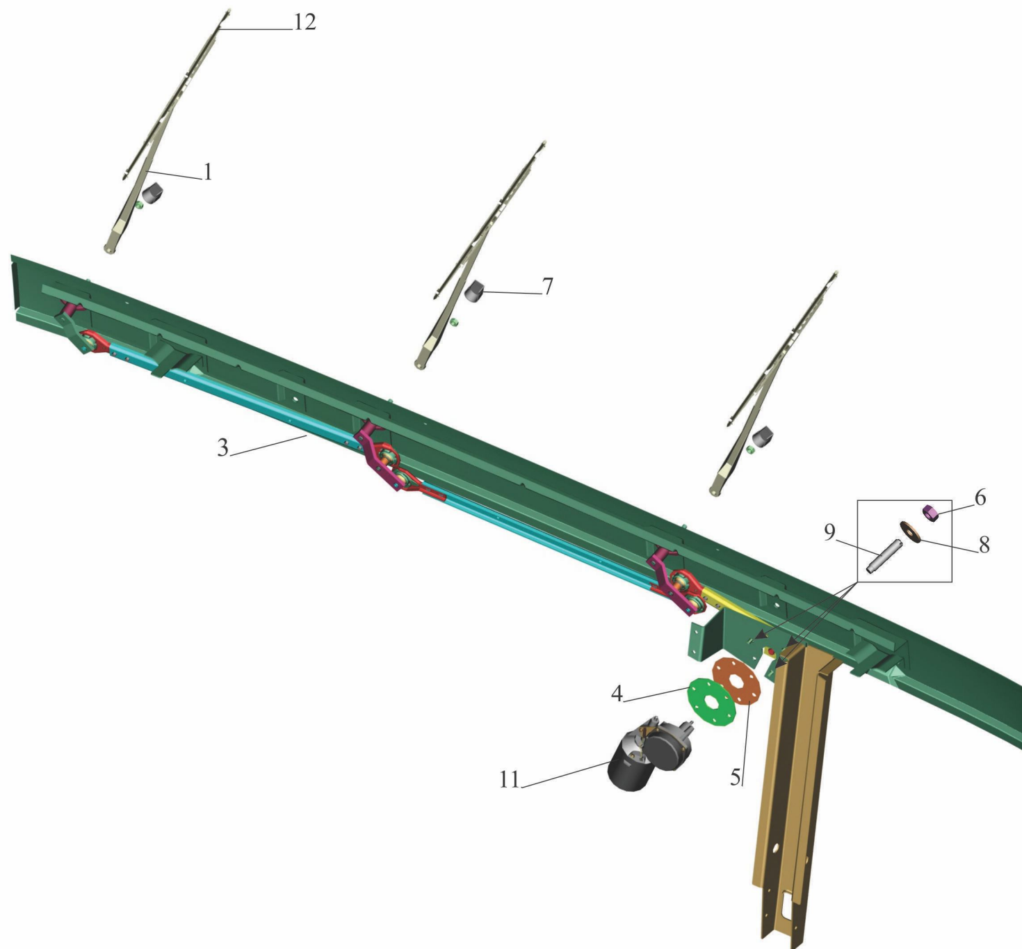
Рис.229 Установка стеклоочистителя 6430-3700041-001 Fig. 229 Installation of cleaner of glasses 6430-3700041-001
