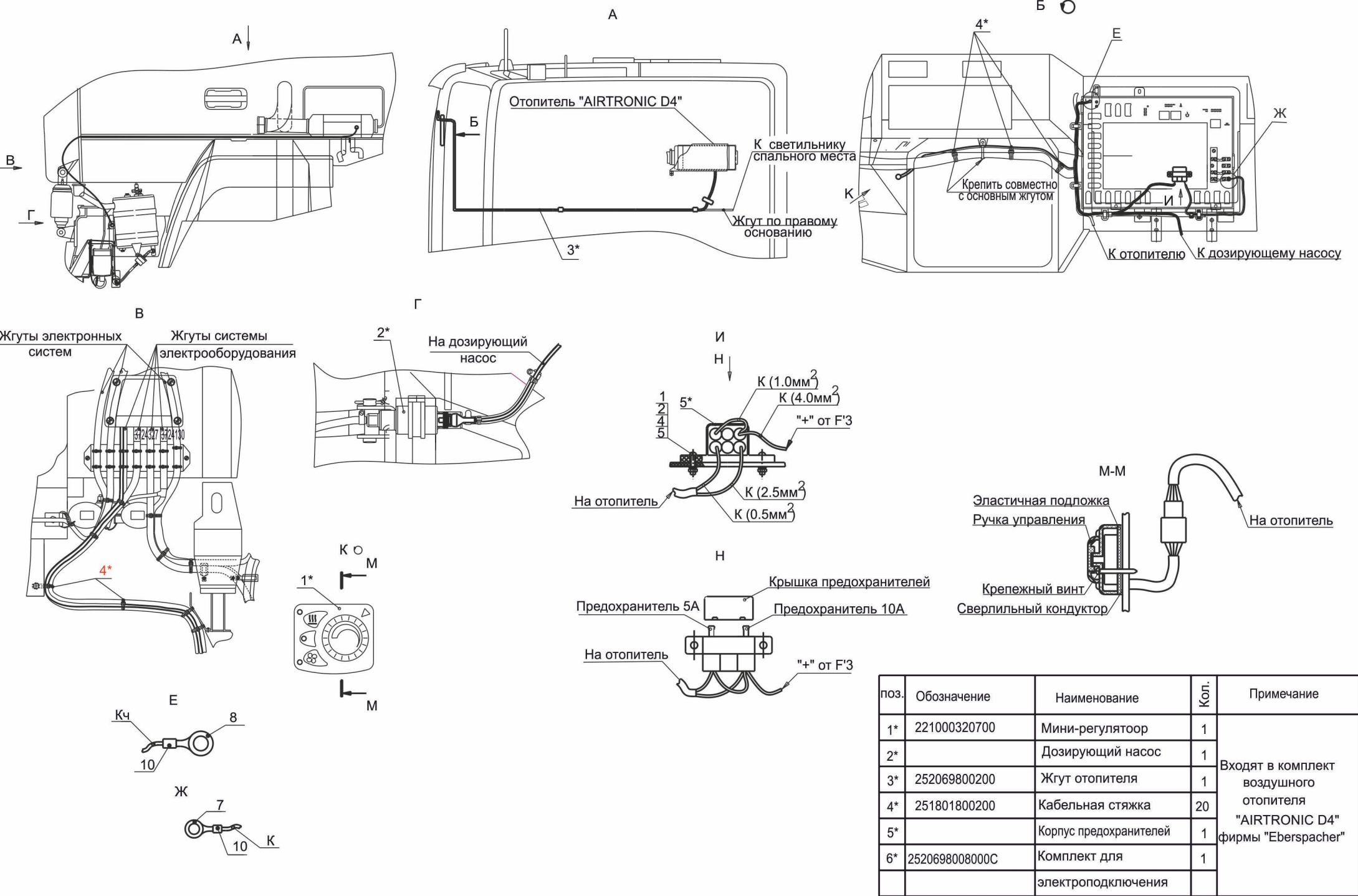
Рис. 294 Установка электрооборудования независимого отопителя 6430-3700088 Fig. 294 Installation of an electrical equipment independent heater 6430-3700088
