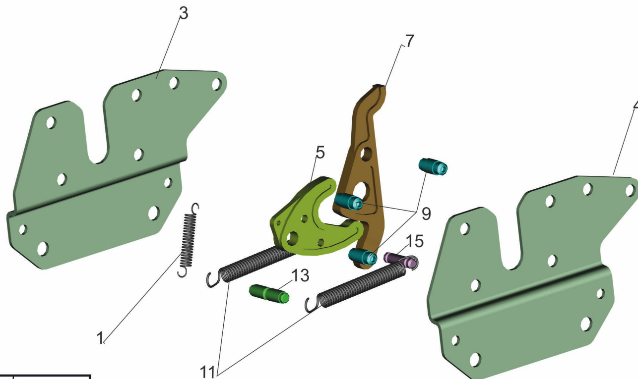
Рис.220 Запорный механизм кабины 6501-5001550 Fig.220 Cab lock mechanism 6501-5001550
