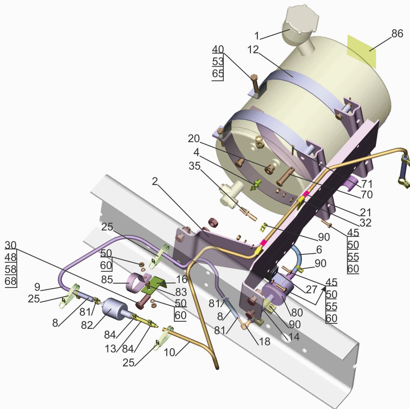
Рис. 8 Крепление топливопроводов подогревателя 4371P2-1015004-000 Fig. 8 Mounting fuel lines of heater 4371P2-1015004-000
