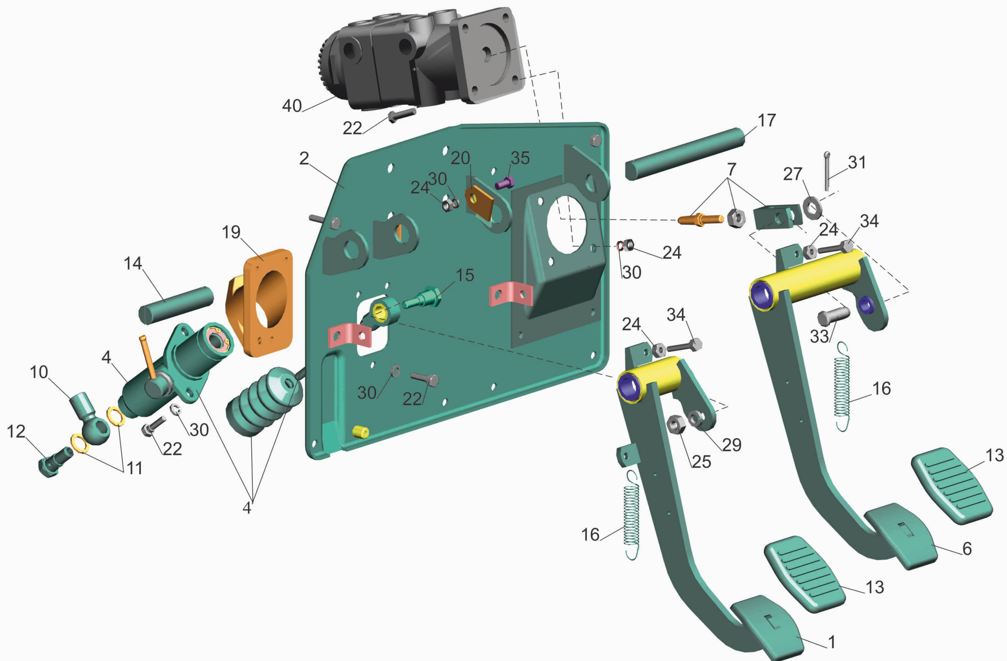
Рис. 32 Блок управления сцеплением 6430-1602004 Fig. 32 Clutch and brake control unit 6430-1602004
