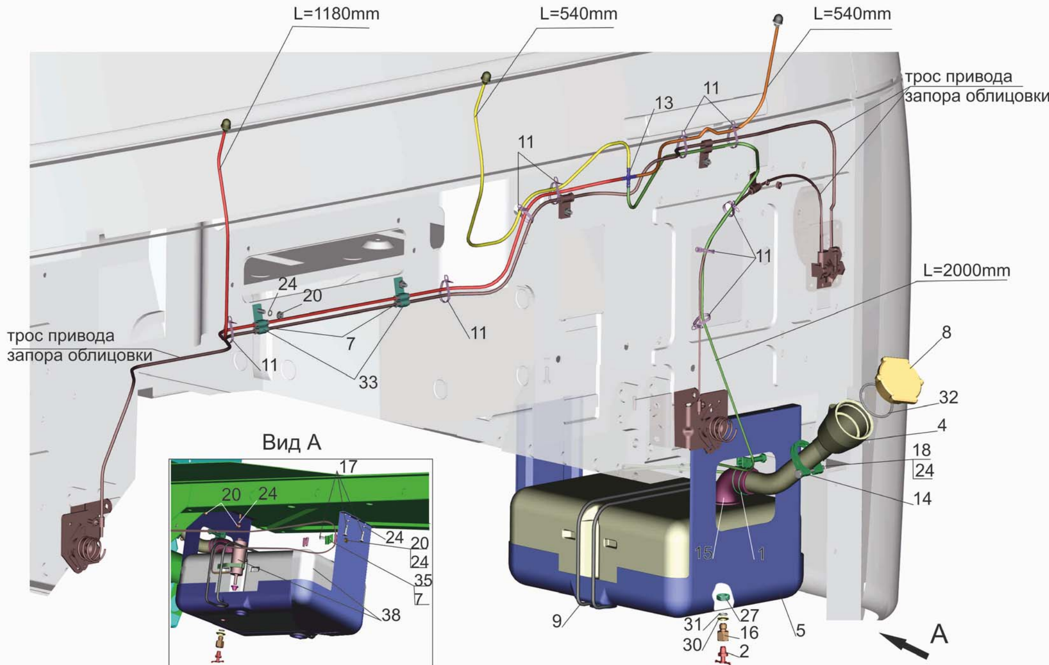
Рис.185 Установка омывателя 6430-5200008 Fig.185 Installation of washer 6430-5200008
