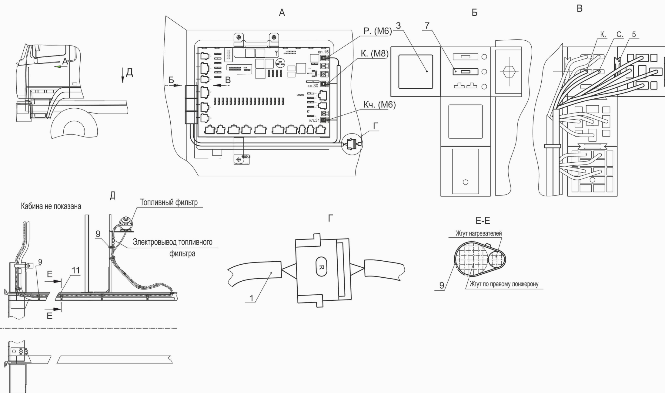
Рис.159 Установка нагревателей на двигателе 4371W1-3700101-000, (-700) Fig. 159 Installation of heating of the fuel filter 4371W1-3700101-000, (-700)
