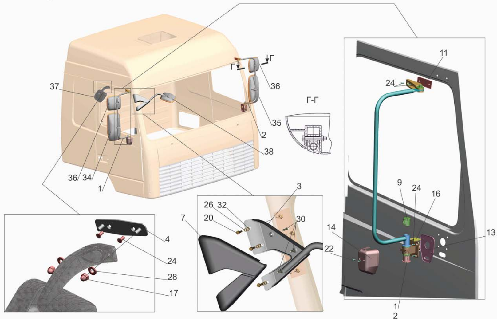
Рис.195 Установка зеркал 6430-82000005-020 Fig.195 Installation mirrors 6430-82000005-020
