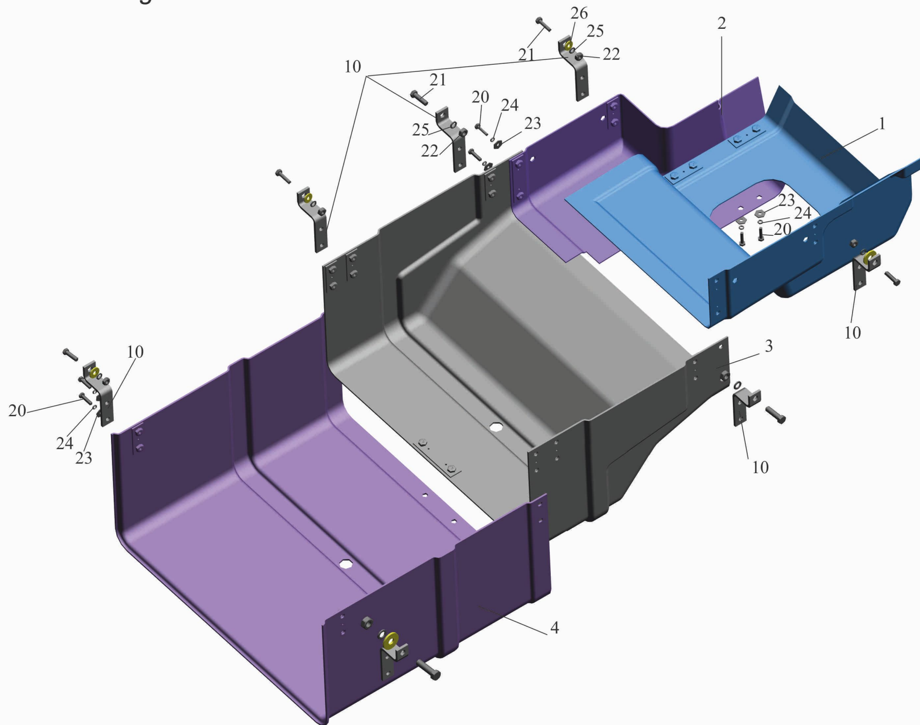
Рис. 11 Установка шумоизоляционных экранов 4571P2-1061004-000 Fig.11 Mounting noise isolation screens 4571P2-1061004-000
