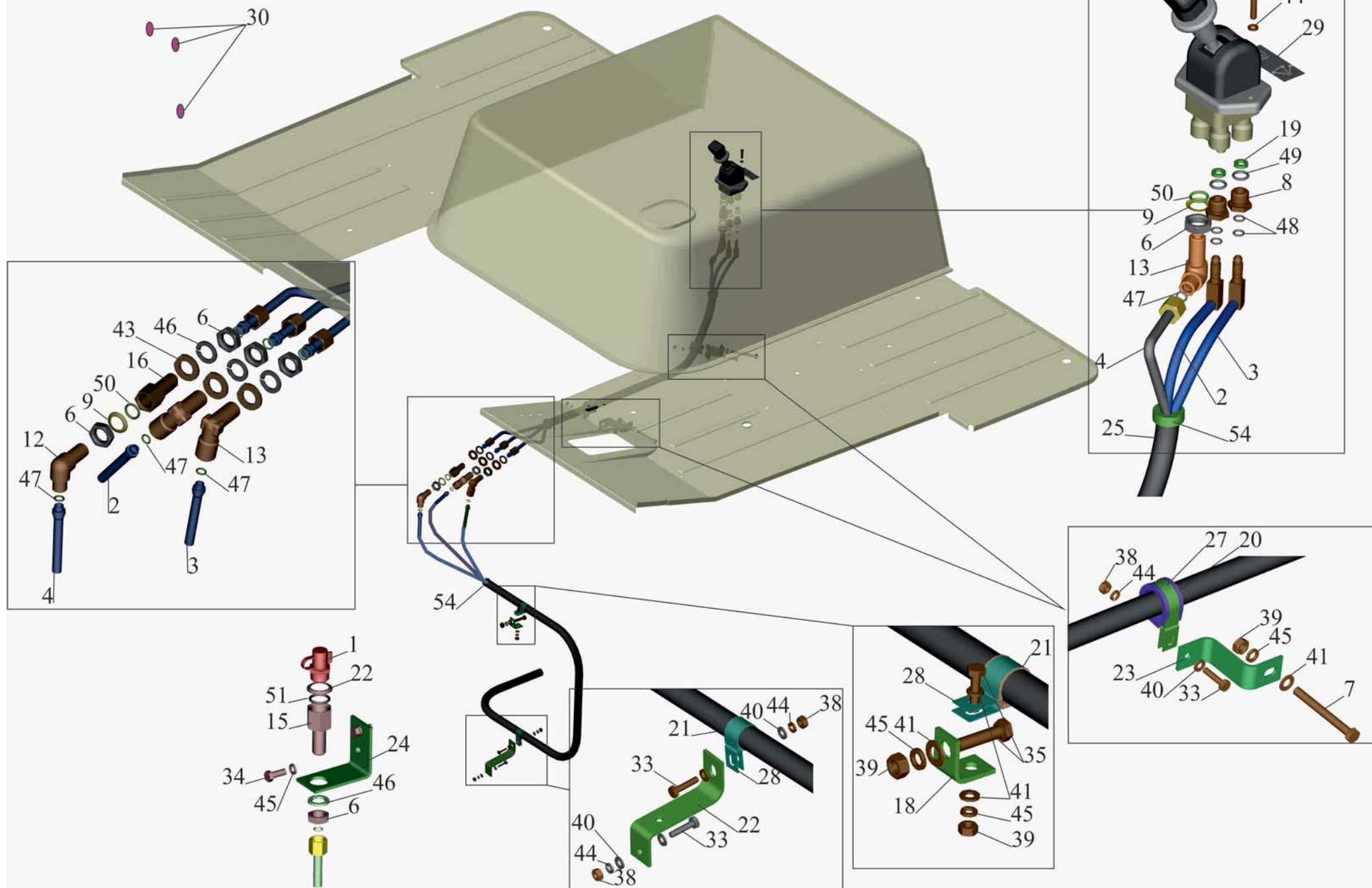
Рис.139 Привод стояночного тормоза 437141-3537006 Fig. 139 Drive gear of parking brake
