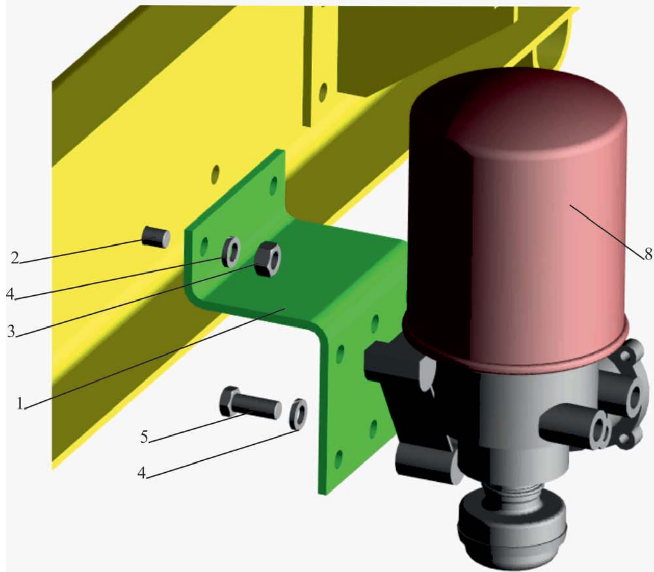
Рис. 137 Крепление осушителя воздуха 4370-3536004 Fig. 137 Installation of air dehumidifier 4370-3536004
