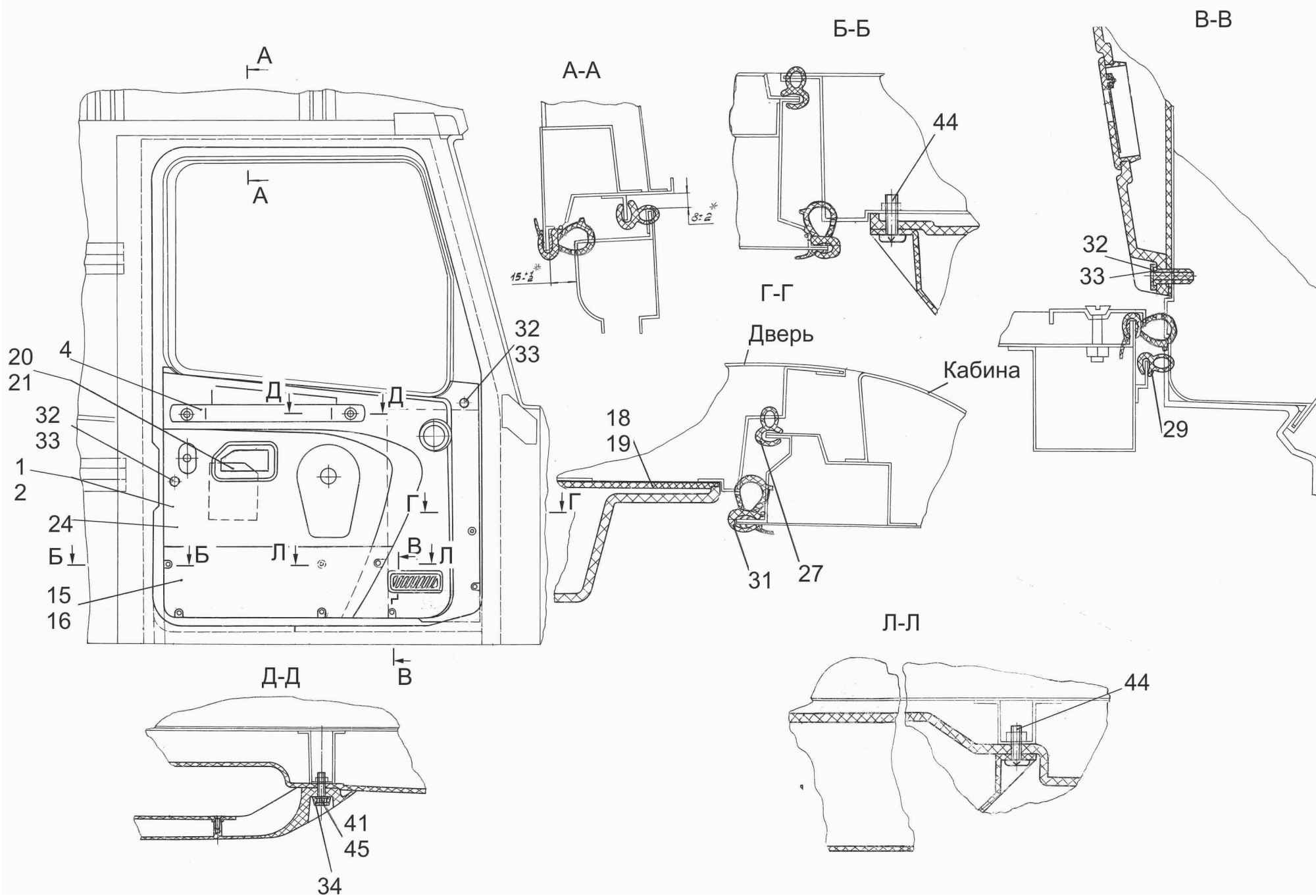
Рис.193 Установка обивок и уплотнителей дверей 6430-6100015-020 Fig.193 Installation of upholsteries and weather strips of doors 6430-6100015-020
