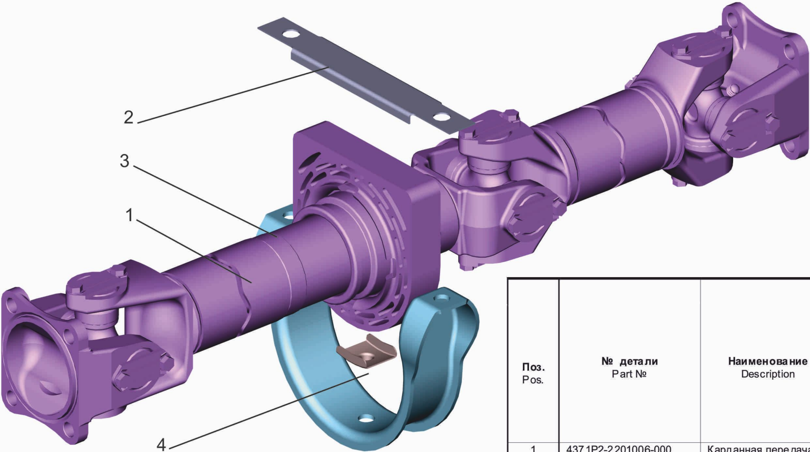
Рис. 48 Комплект карданной передачи 4371P2-2201007-000, 4371P2-2201007-000 Д, 4371P2-2201007-010, 4371P2-2201007-010 Д Fig. 48 Complete set of a cardan drive 4371P2-2201007-000, 4371P2-2201007-000 Д, 4371P2-2201007-010, 4371P2-2201007-010 Д
