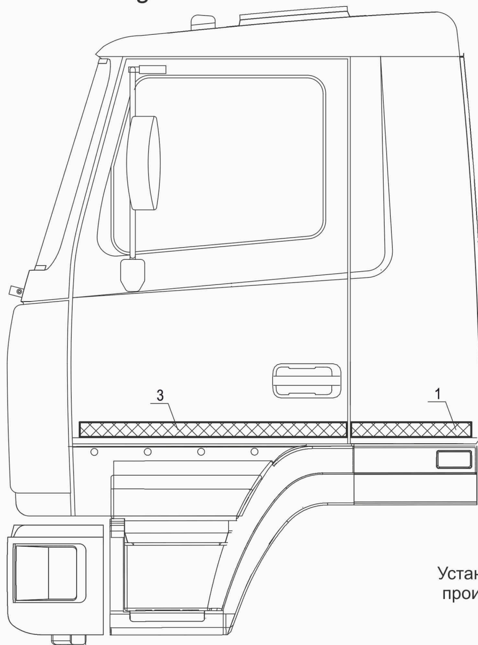
Рис. 169 Установка светоотражающей маркировки 447131-8200001-000 Fig. 169 Installation of switches
