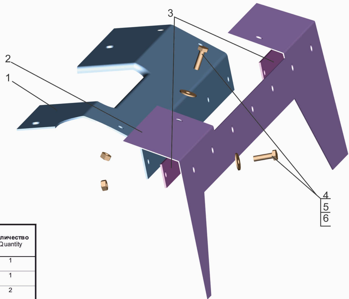
Рис. 27 Уплотнитель с пластиной 447131-1310068 Fig. 27 Seal with plate 447131-1310068
