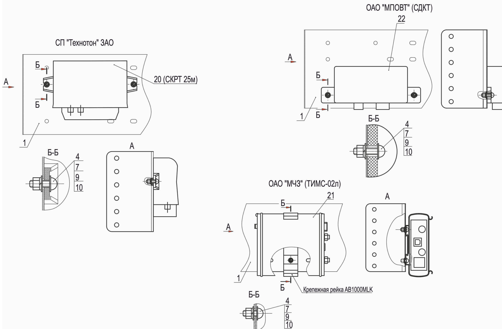
Рис. 171 Установка системы телеметрии Лист 1 Fig. 171 Installation of system of telemetry Page 1
