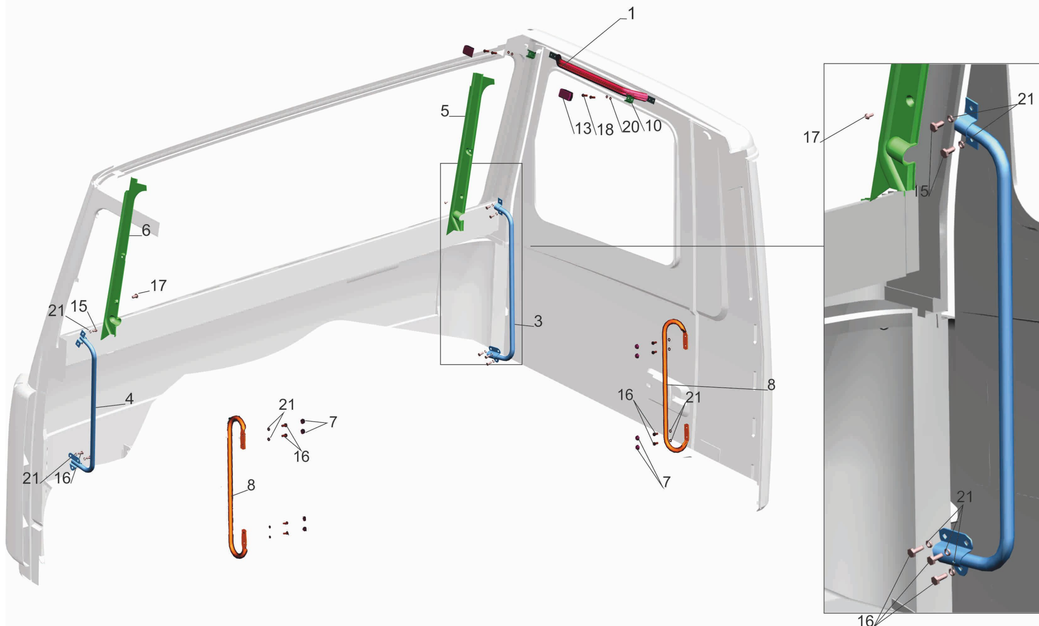
Рис. 197 Установка поручней в кабине 6430-8200030. Fig. 197 Installation of grab handles in cab 6430-8200030.
