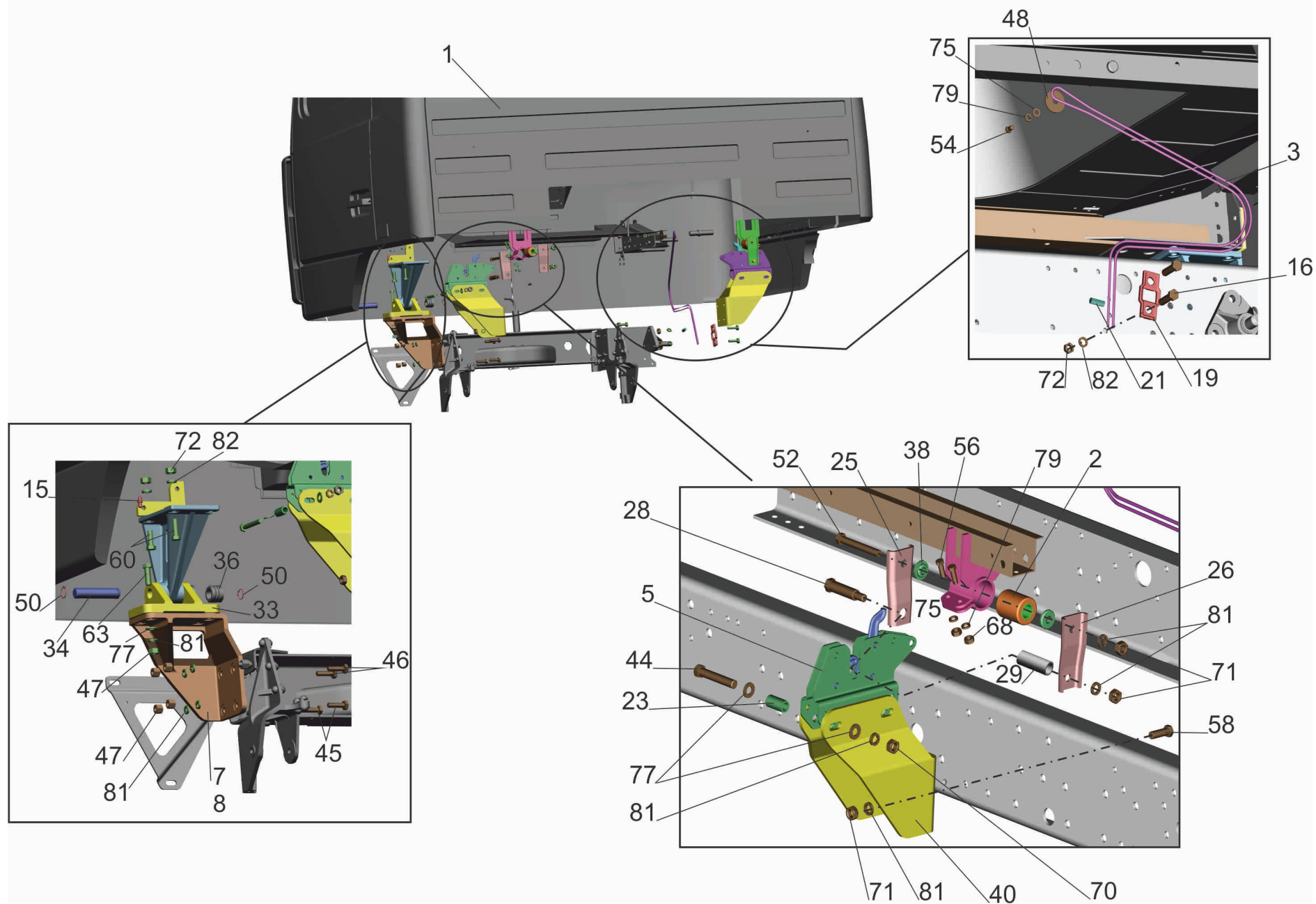
Рис. 179 Крепление кабины к раме Fig. 179 Fastening cabin to frame
