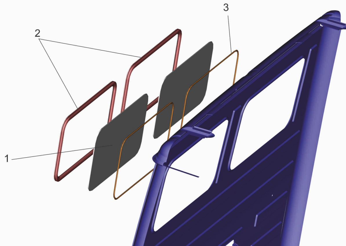
Рис.187 Установки стекла задка 6501-5600015. Fig.187 Installation a back glass 6501-5600015.
