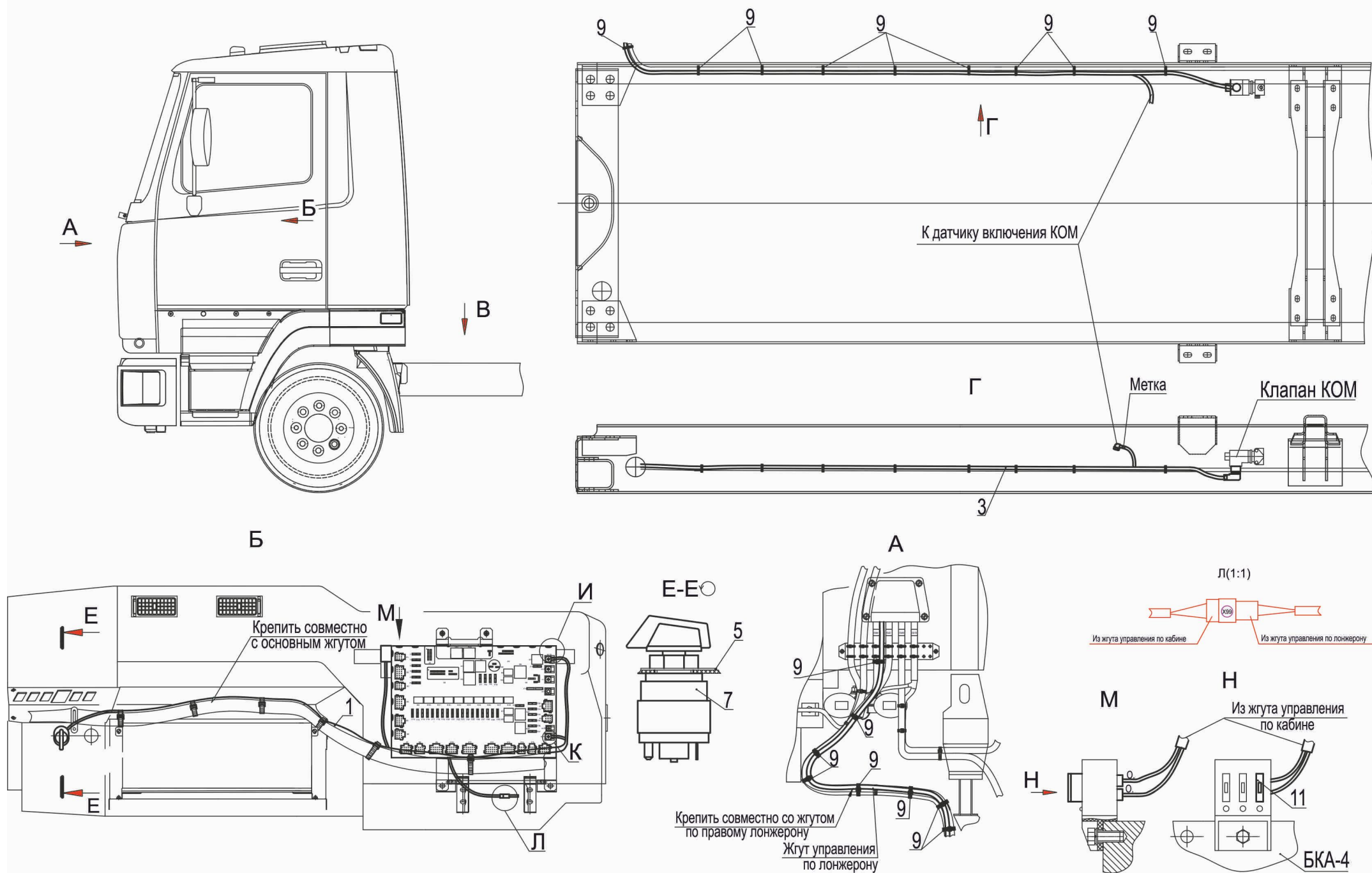
Рис. 161 Установка электрооборудования управления платформой 4381W2-3700112-000 Fig. 161 Installation of an electric equipment of control by a platform 4381W2-3700112-000
