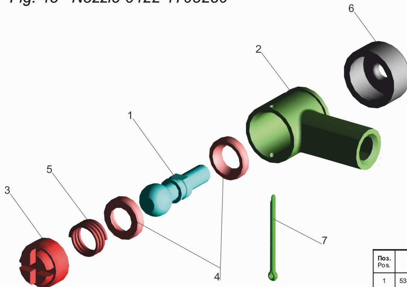
Рис. 45 Наконечник 6422-1703250 Fig. 45 Nozzle 6422-1703250
