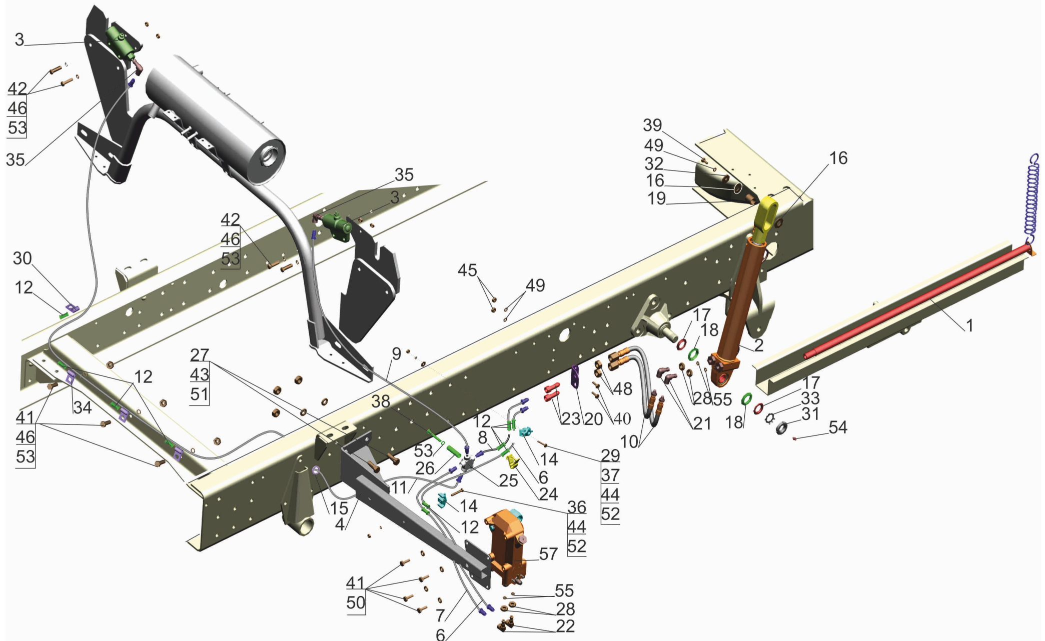
Рис.204 Механизм подъема кабины 4371Р2-5000040-000 Fig. 204 Cab tilting mechanism 4371P2-5000040-000
