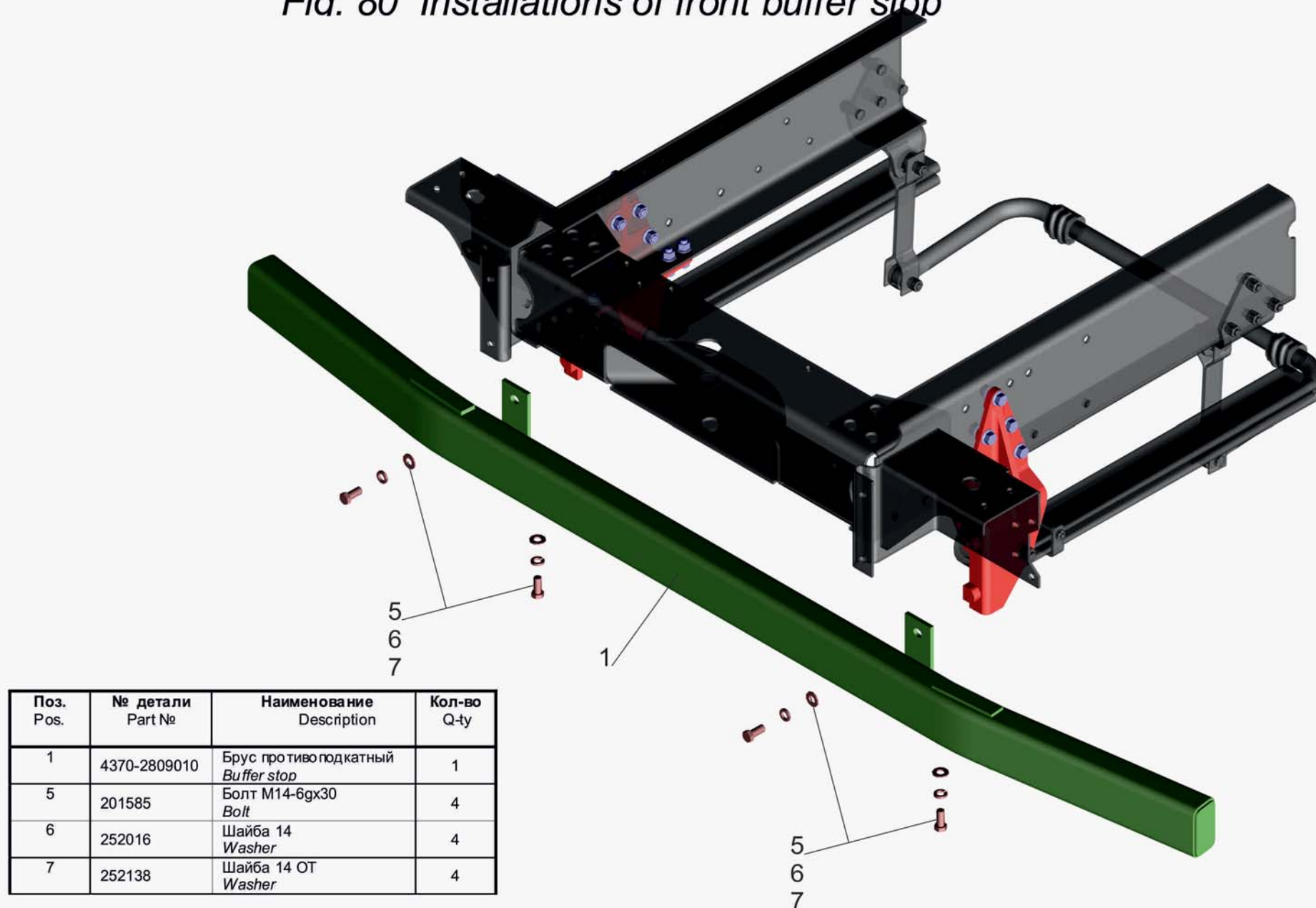
Рис. 80 Установка переднего противоподкатного бруса 4370-2800030. Fig. 80 Installations of front buffer stop
