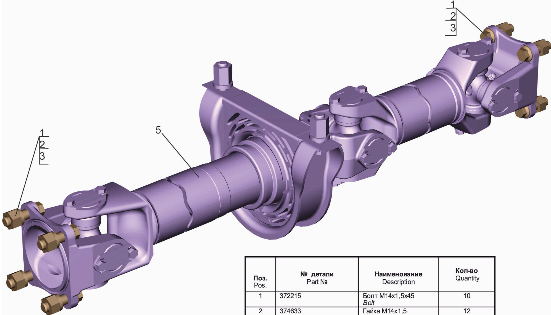
Рис. 47 Установка карданной передачи 4371P2-2200000-010 Fig. 47 Installation of a cardan drive 4371P2-2200000-010
