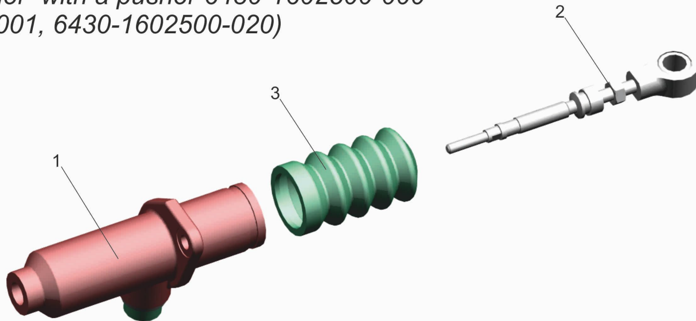
Рис. 34 Цилиндр подпедальный с толкателем 6430-1602500-000 (6430-1602500-001, 6430-1602500-020)
