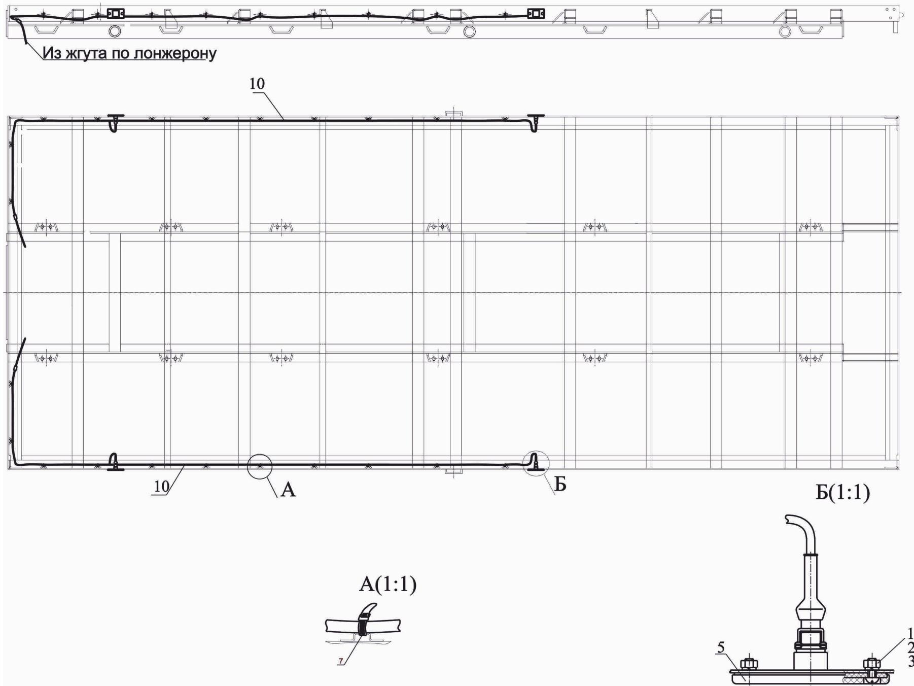
Рис.153 Установка боковых габаритных фонарей Fig.153 Setting of lateral sidelights
