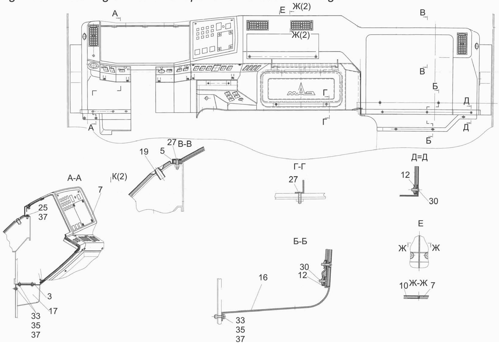
Рис. 188 Установка панели приборов 6418-5300014 Лист 1 Fig. 188 Installing of instrument panel 6418-5300014 Page 1
