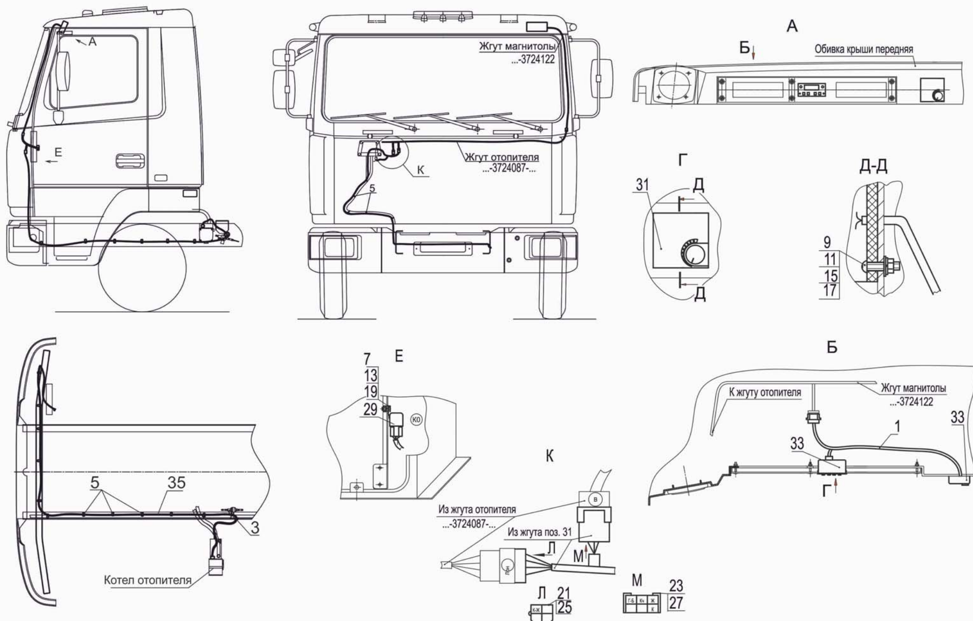
Рис. 154 Установка электрооборудования подогревателя 437141-3700085 Fig.154 Mounting of electrical equipment heater 437141-3700085
