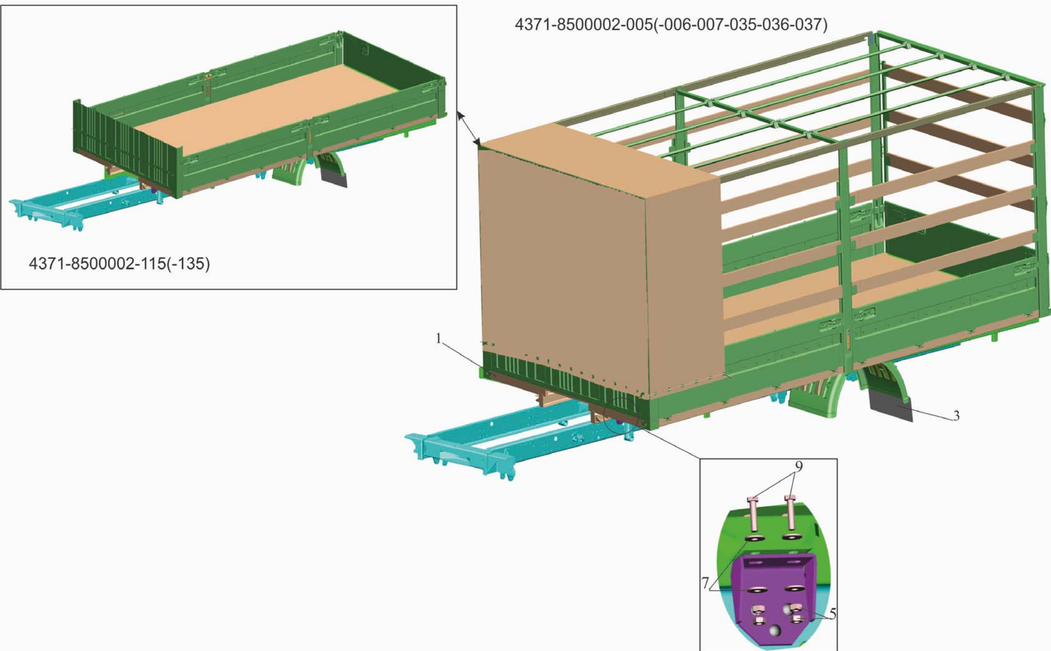
Рис. 242 Установка платформы Fig. 242 Installation platform
