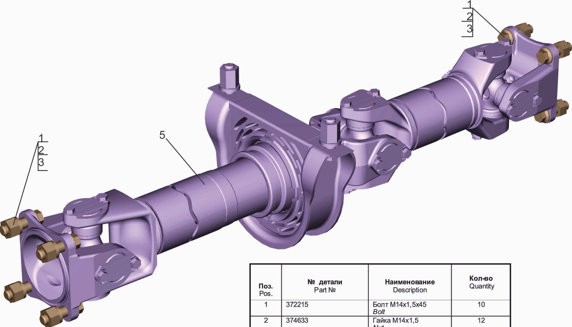
Рис. 46 Установка карданной передачи 4371P2-2200000-000 Fig. 46 Installation of a cardan drive 4371P2-2200000-000
