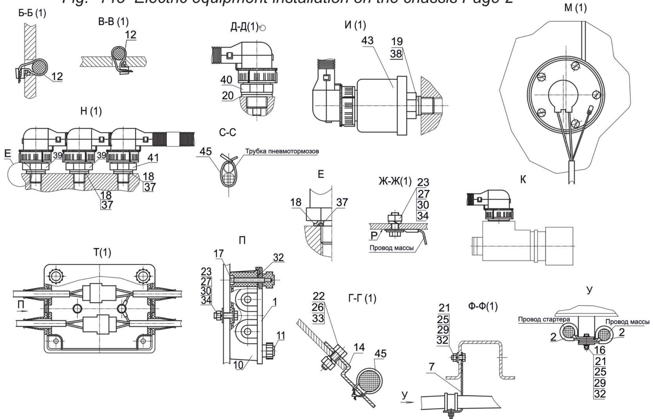
Рис. 145 Установка электрооборудования на шасси Лист 2 Fig. 145 Electric equipment installation on the chassis Page 2
