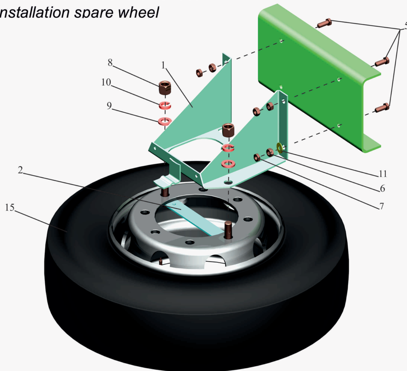
Рис.108 Установка запасного колеса
