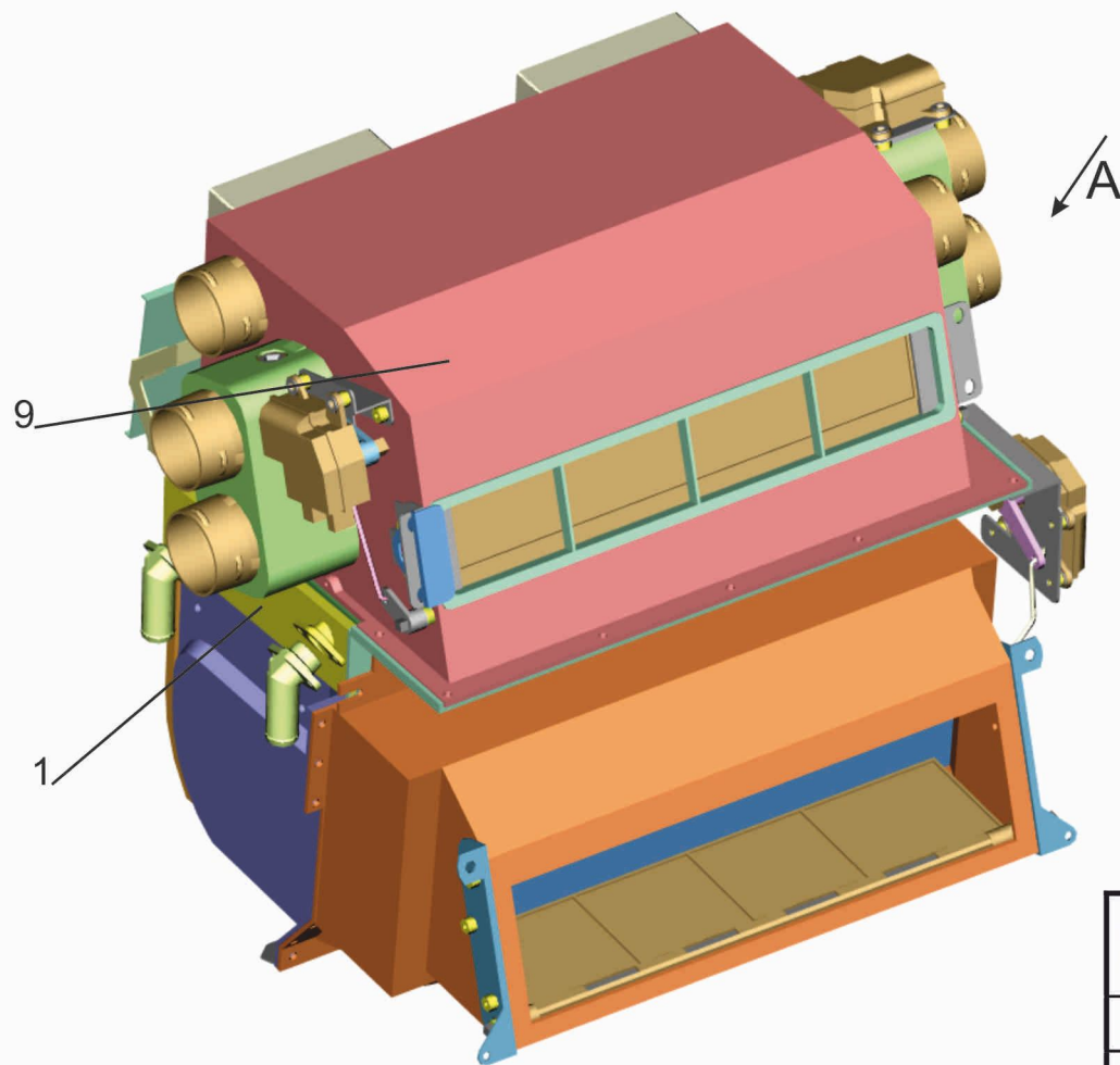
Рис. 227 Отопитель 631019-8101010 Fig. 227 Heater 631019-8101010
