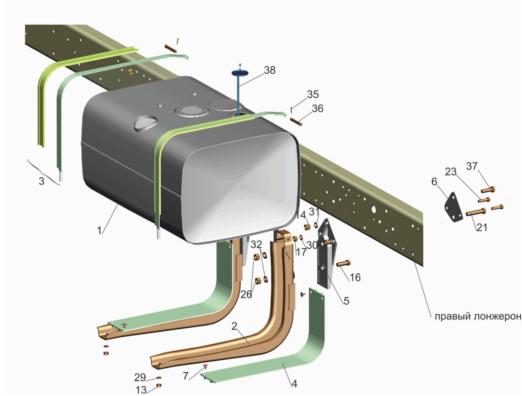
Рис.13 Крепление топливного бака 4371V2-1101002-000 Fig. 13 Mounting of fuel tank 4371V2-1101002-000
