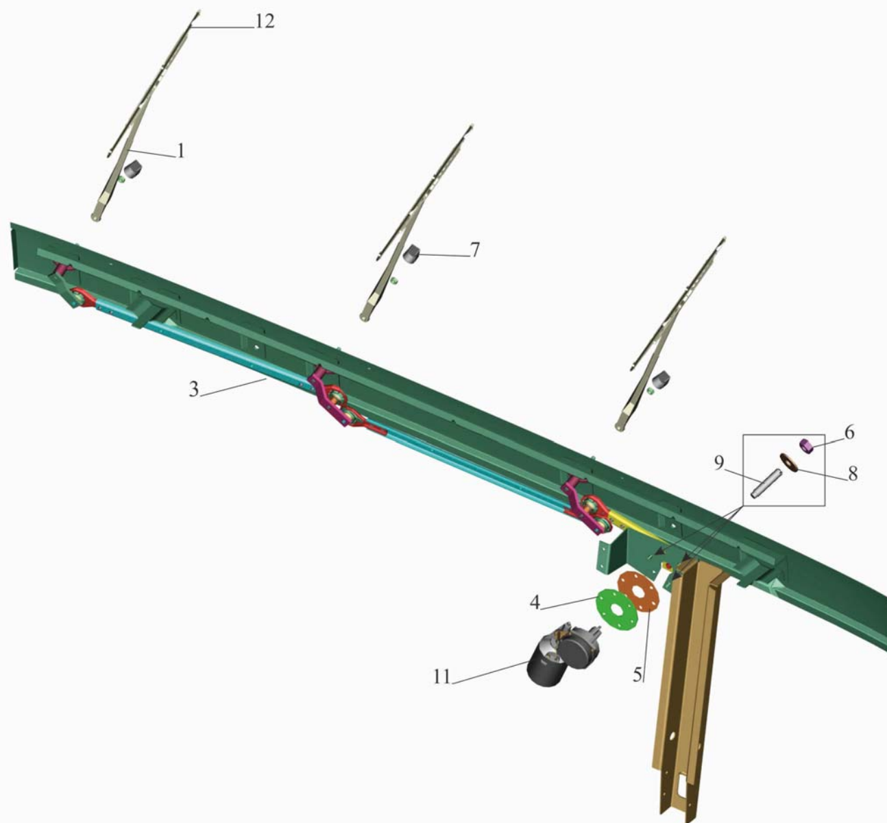
Рис.182 Установка стеклоочистителя 6430-3700041-001 Fig.182 Installation of cleaner of glasses 6430-3700041-001
