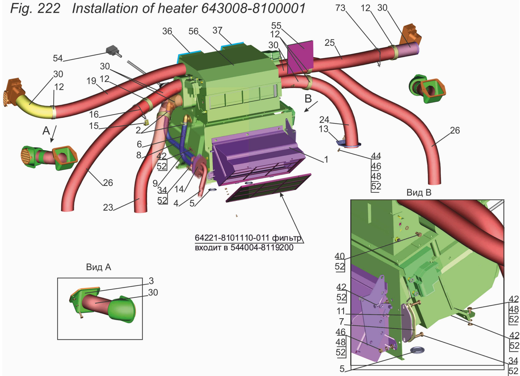
Рис. 222 Установка отопителя 643008-8100001
