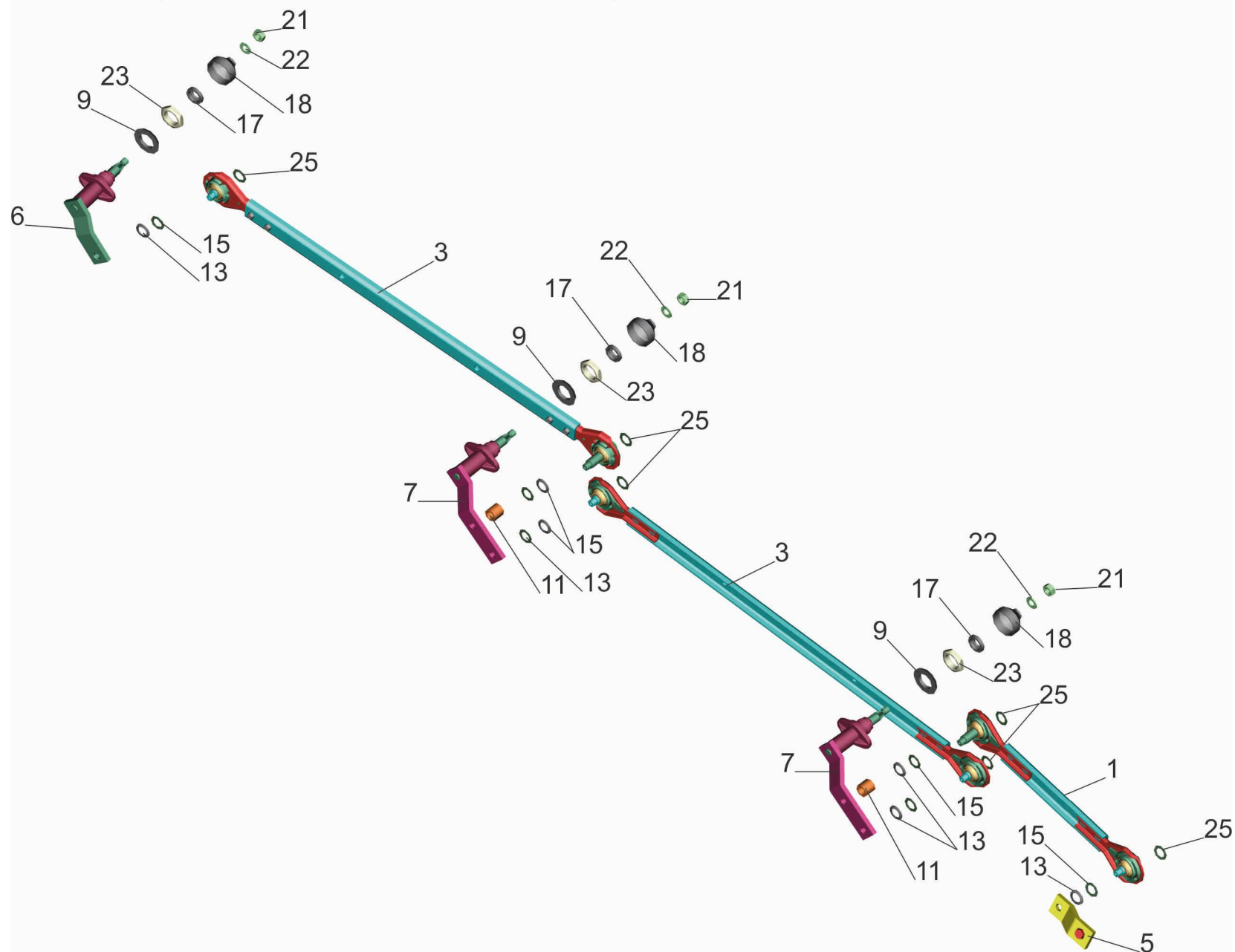
Рис.183 Привод стеклоочистителя 6430-5205500-010 Fig.183 Drive of cleaner of glasses 6430-5205500-010
