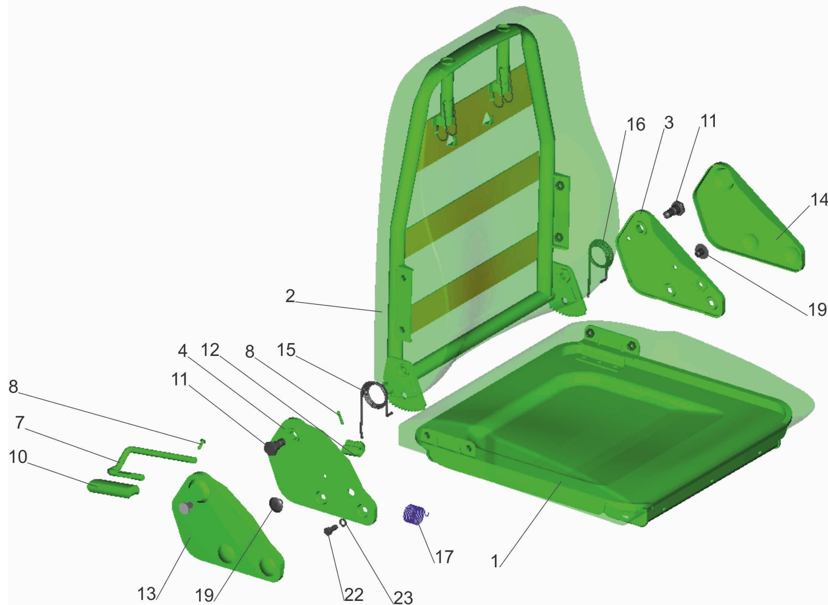
Рис. 218 Подушка и спинка сидения 6430-6810012 Fig. 218 Pad and back seat 6430-6810012
