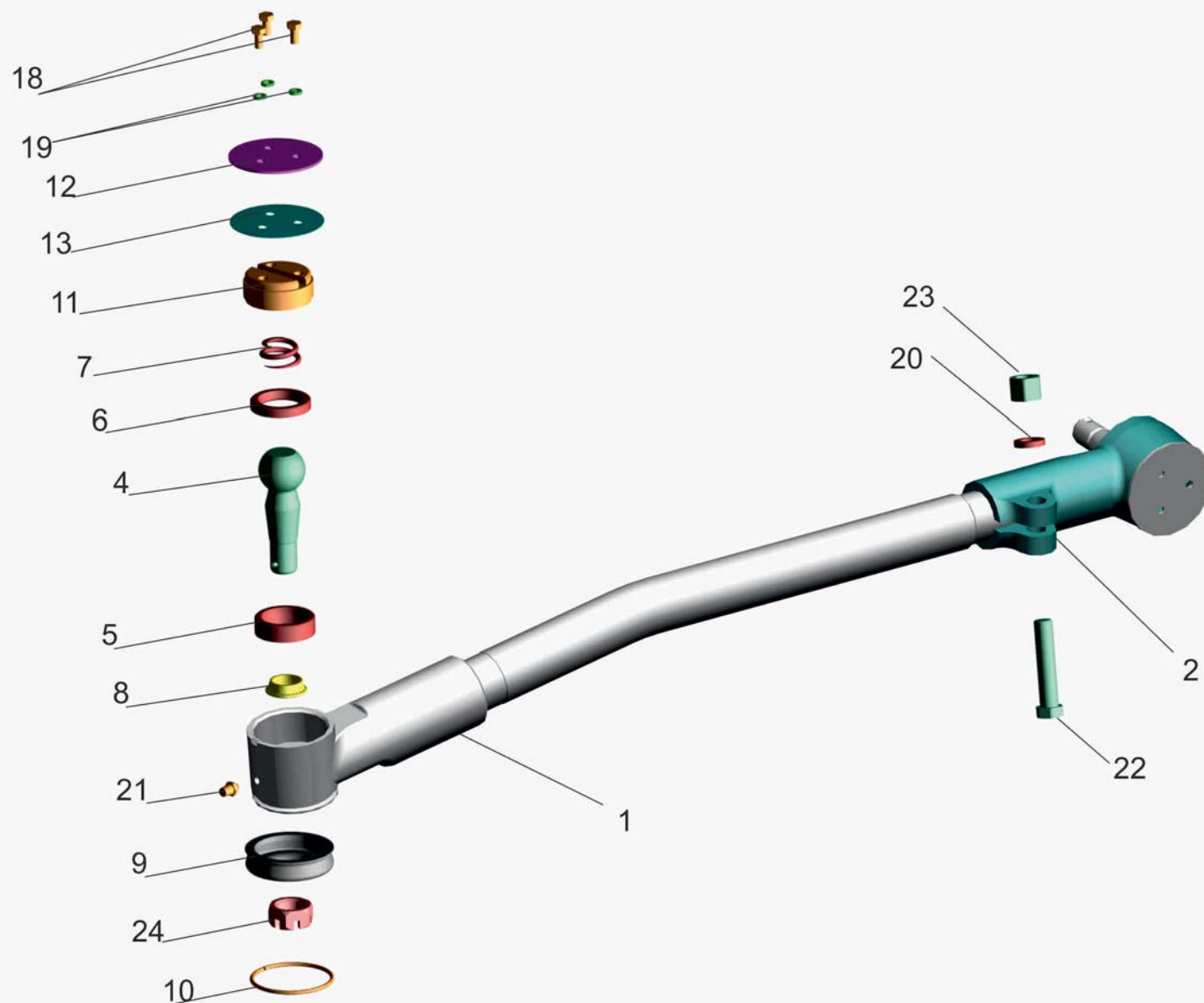
Рис. 106 Тяга продольная 437040-3003010 Fig. 106 Drag rod 437040-3003010
