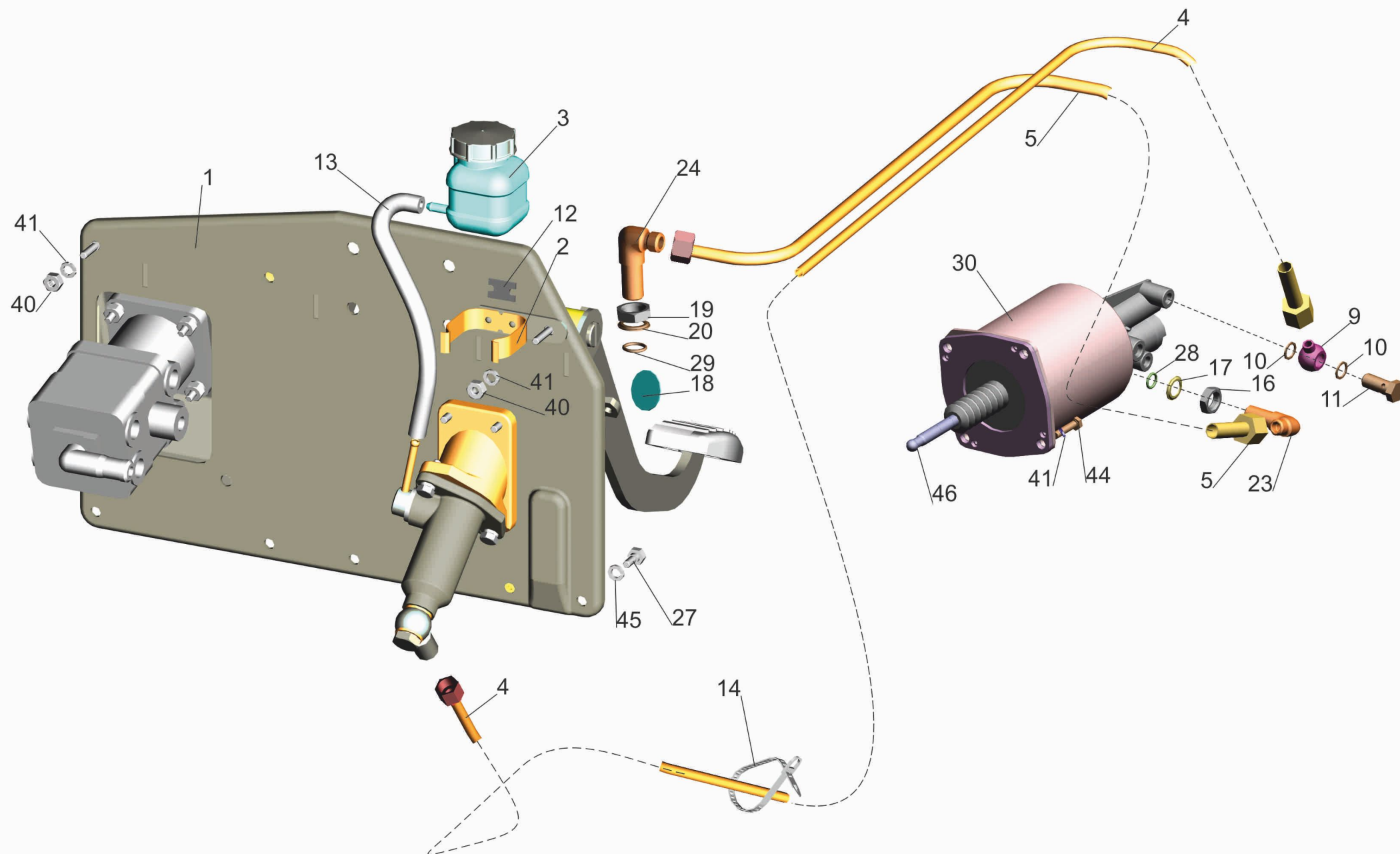
Рис. 30 Установка механизма управления сцеплением 437141-1600005-010 Fig. 30 Installation of a clutch-operating device 437141-1600005-010
