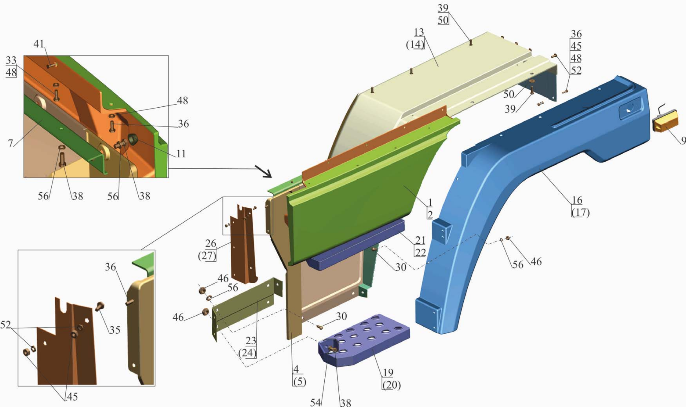
Рис. 239а Установка оперения 4371W2-8400020-000 Fig. 239a Installation of plumage
