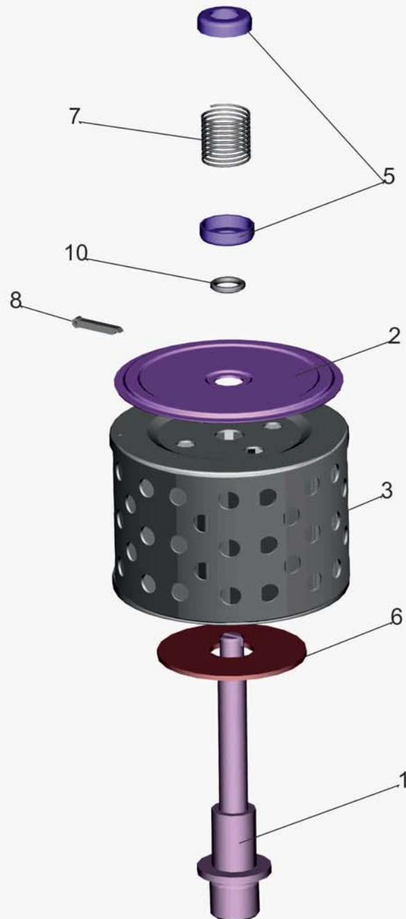
Рис. 122 Фильтр с клапаном 5336-3410051 Fig. 122 Filter with the valve 5336-3410051
