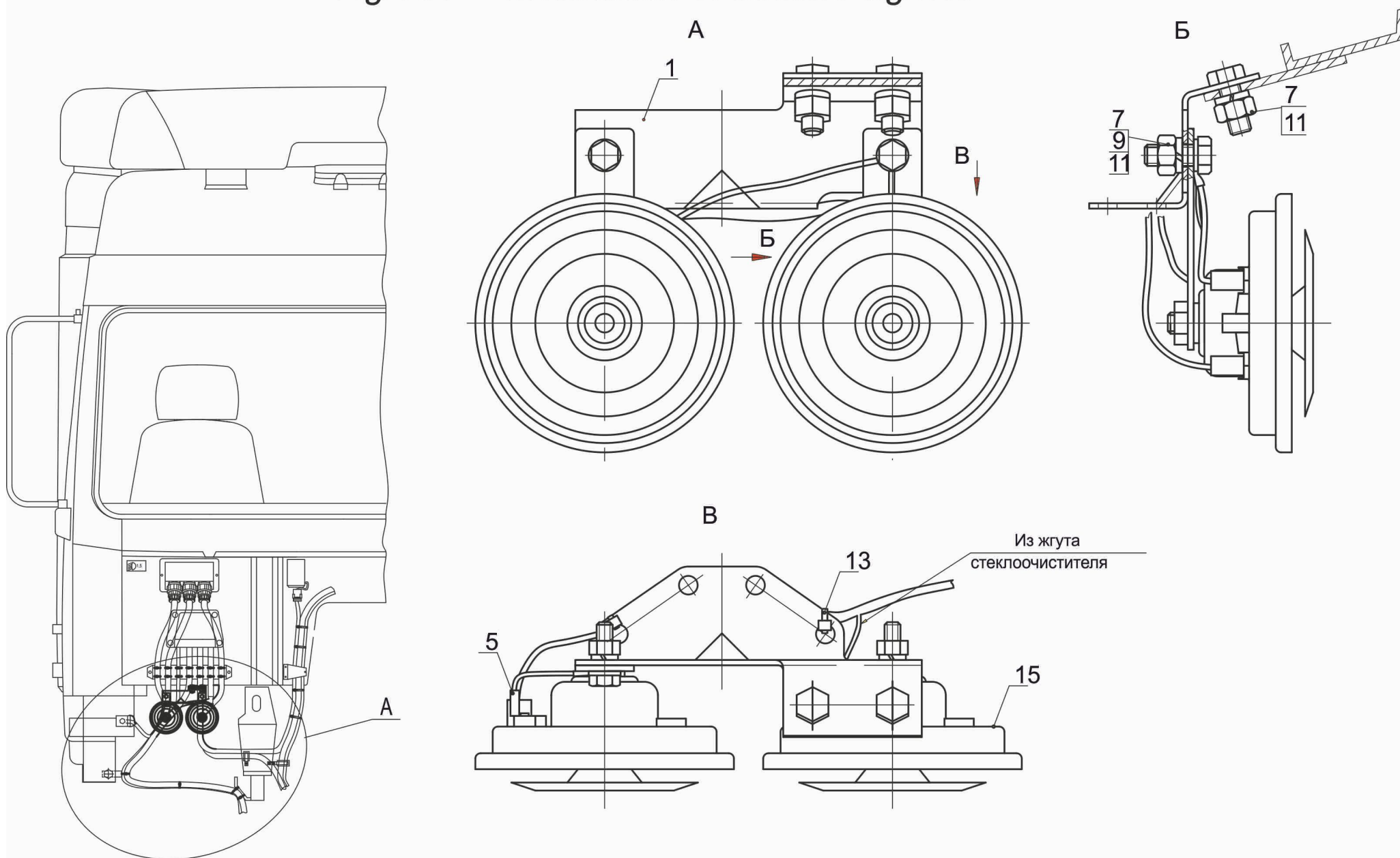
Рис.151 Установка звуковых сигналов Fig.151 Installation of audible signals
