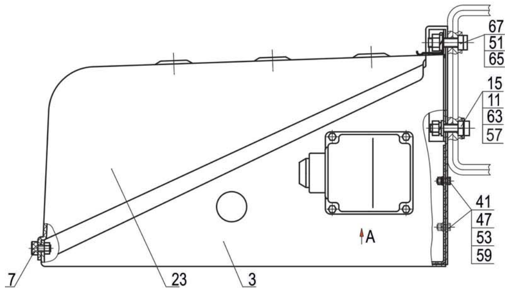
Рис. 143 Установка аккумуляторных батарей Fig. 143 Installation of storage batteries
