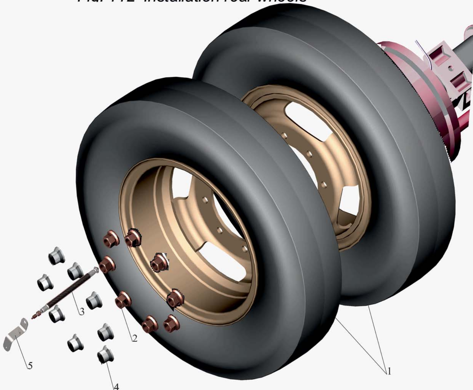
Рис. 112 Установка задних колес Fig. 112 Installation rear wheels
