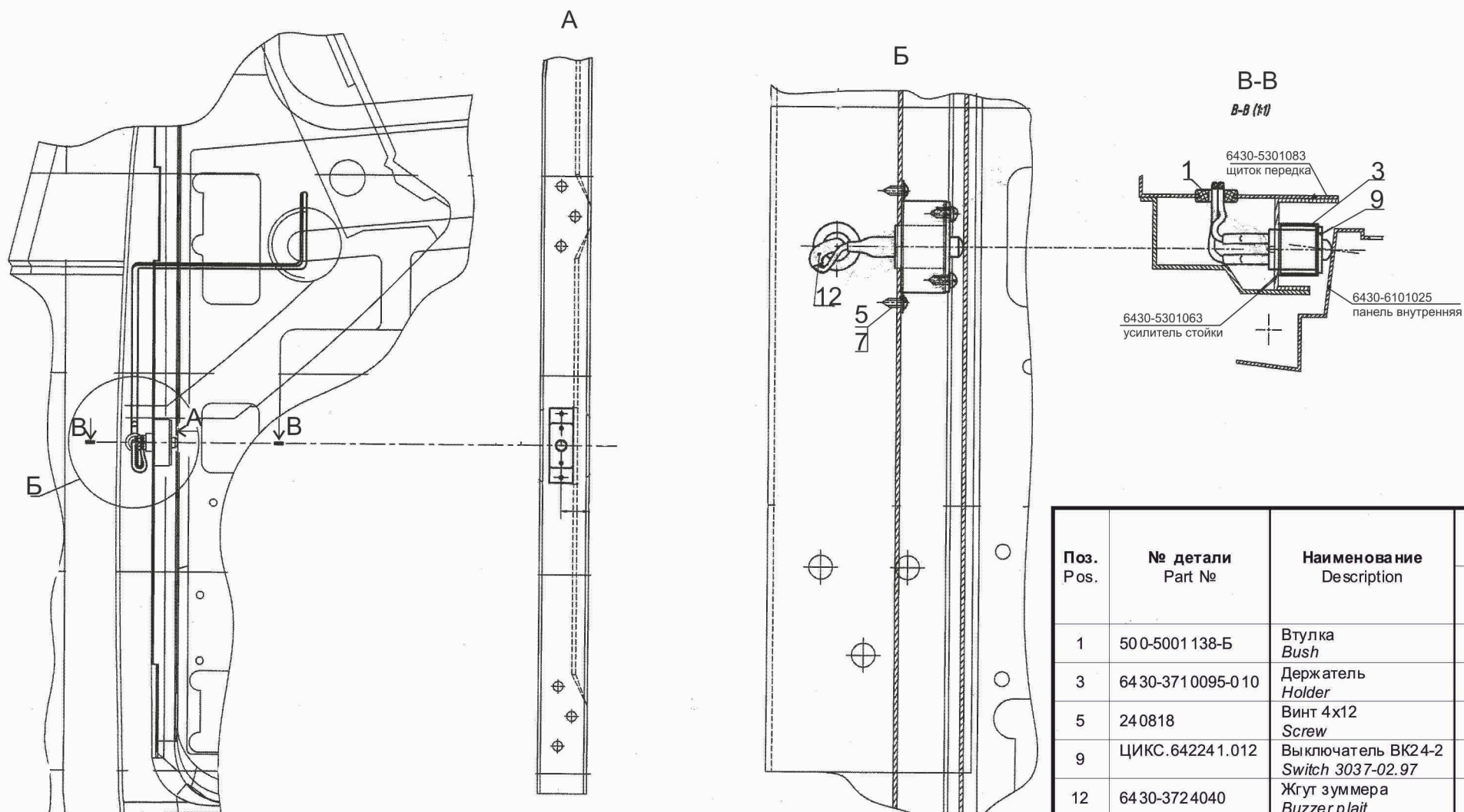
Рис. 152 Установка датчика открытой двери Fig.152 Installation of the gauge of an open door
