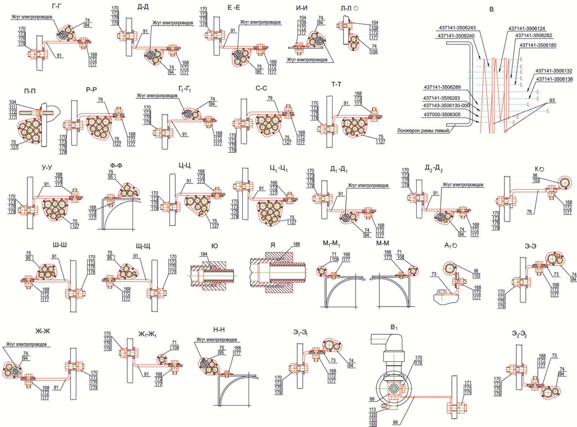
Рис.128 Установка пневмотормозов 4371Р2-3500003-060 (лист 2) Fig.128 Installation pneumobrakes
