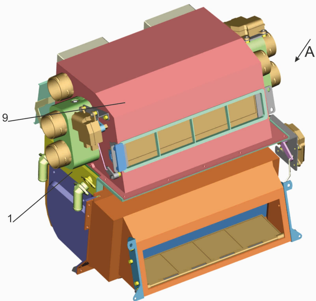
Рис. 226 Отопитель 643008-8101010 Fig. 226 Heater 643008-8101010
