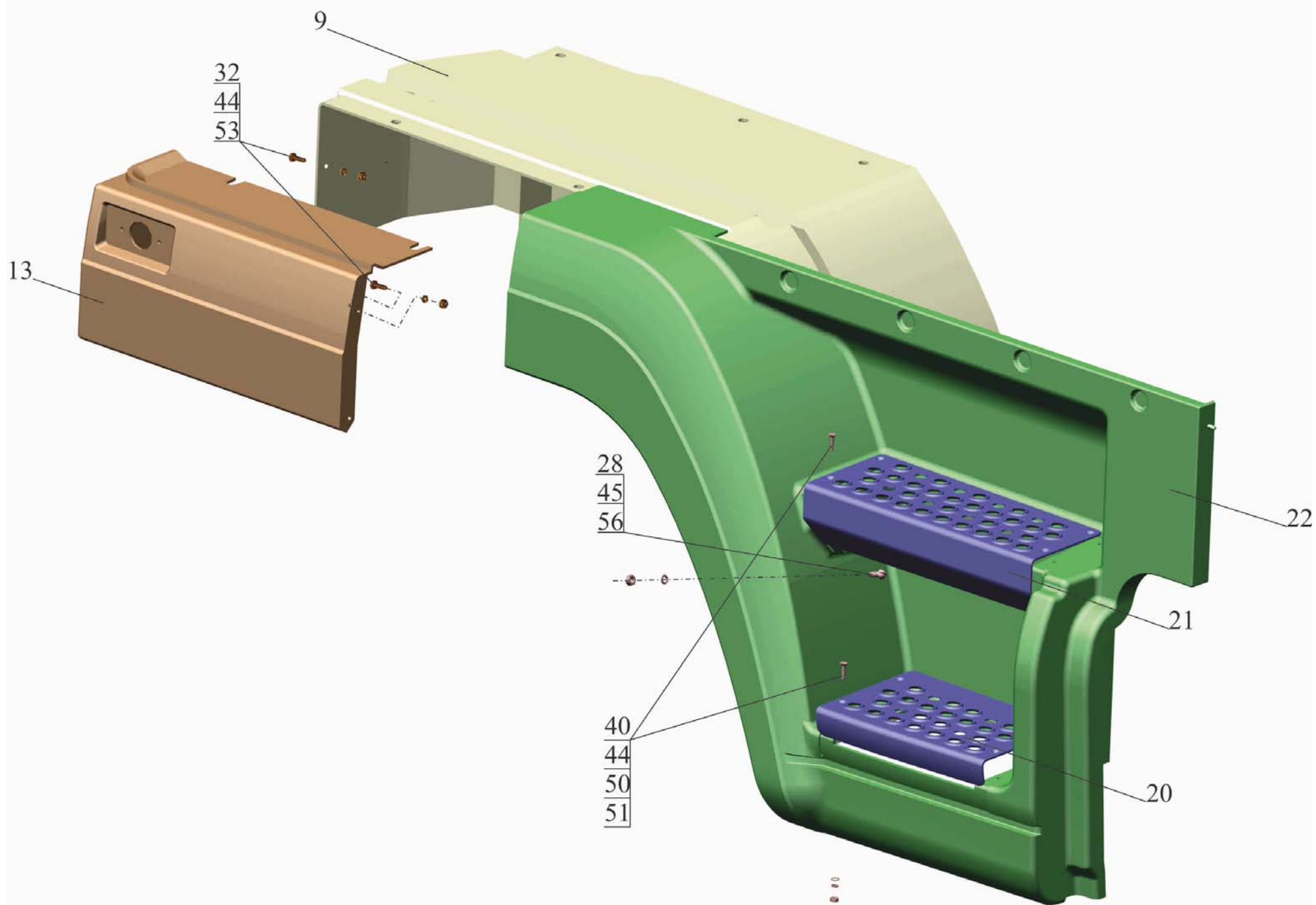
Рис.2396 Оперение 4371-8400010-010 Fig.2396 Plumage 4371-8400010-010
