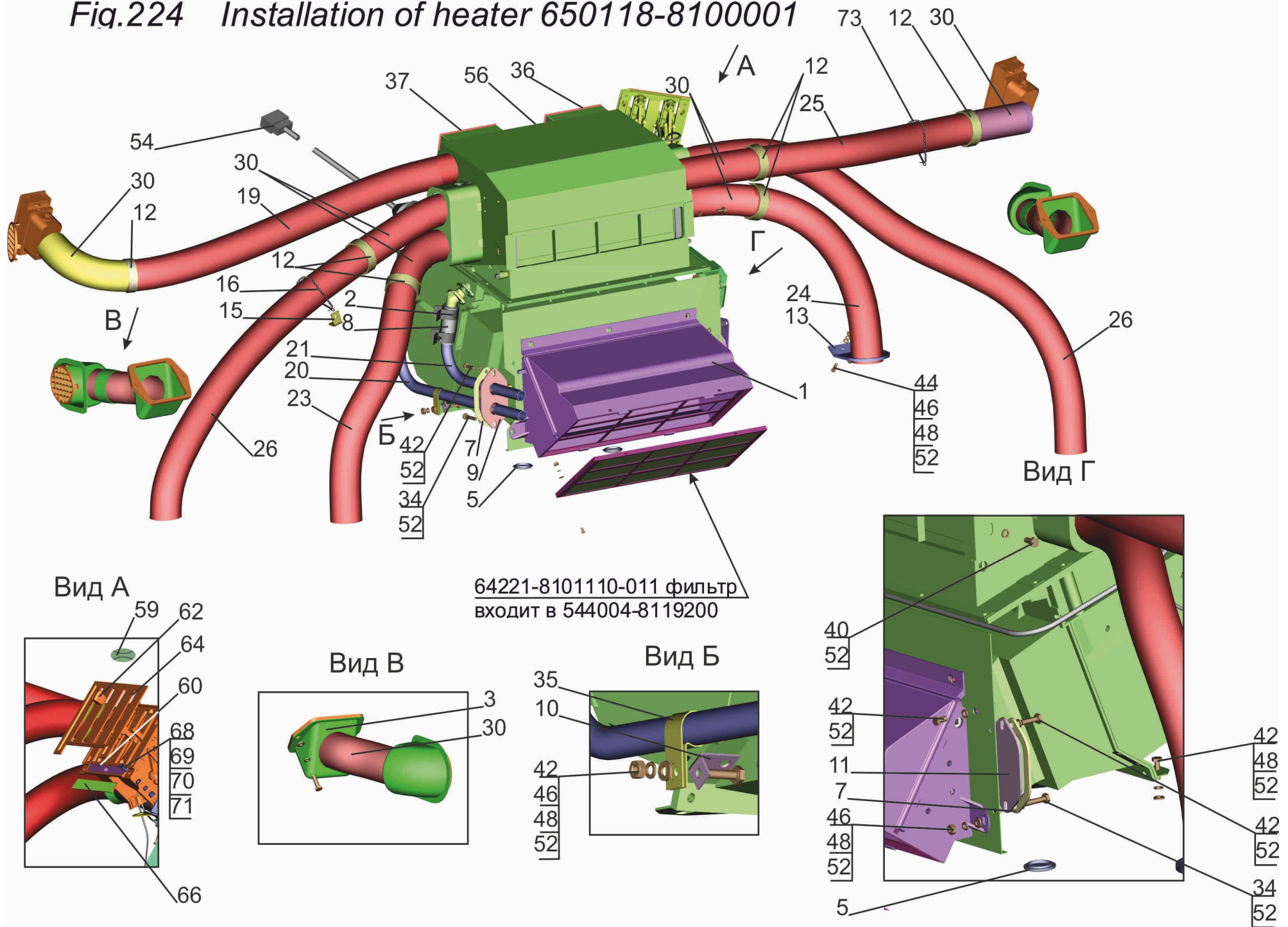
Рис.224 Установка отопителя 650118-8100001
