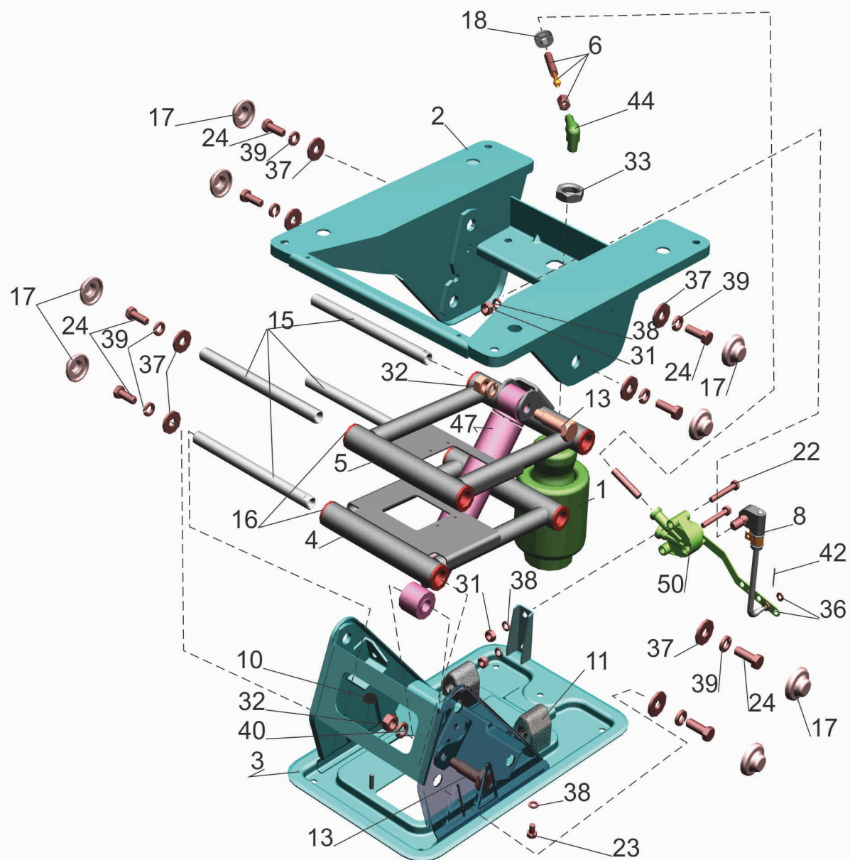
Рис. 216 Подставка сиденья с пневмооборудованием 6430-6807006-010 Fig. 216 Seat support with pneumatic equipment 6430-6807006-010
