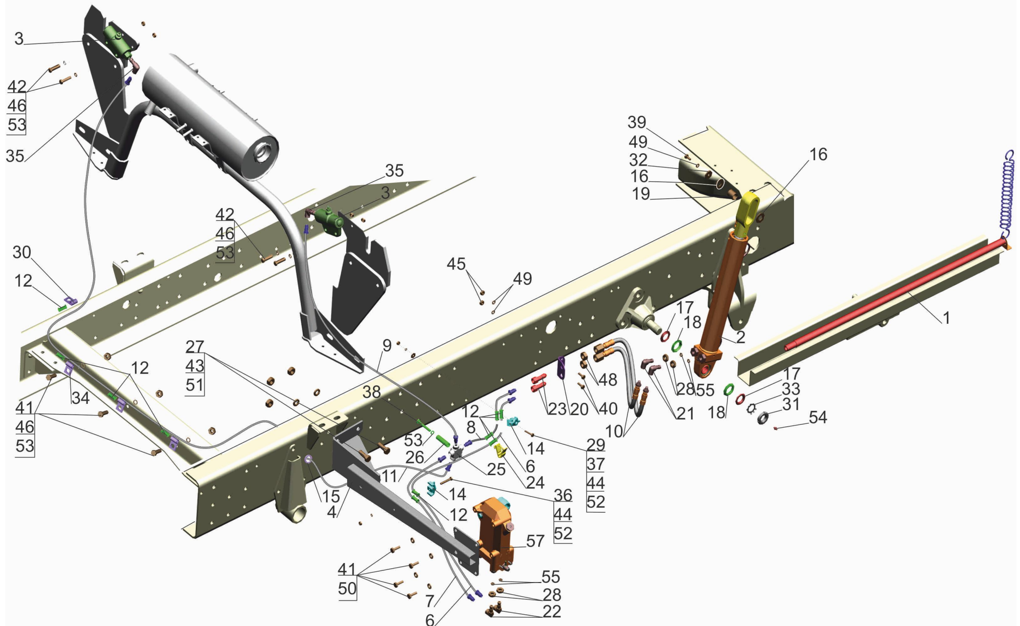
Рис.205 Механизм подъема кабины 4371Р2-5000040-010 Fig. 205 Cab tilting mechanism 4371P2-5000040-010
