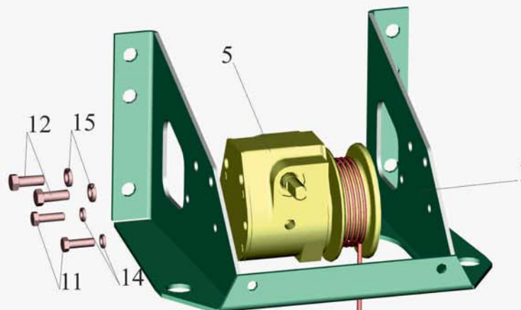
Рис. 110 Кронштейн 437041-3105050 Fig. 110 Bracket 437041-3105050
