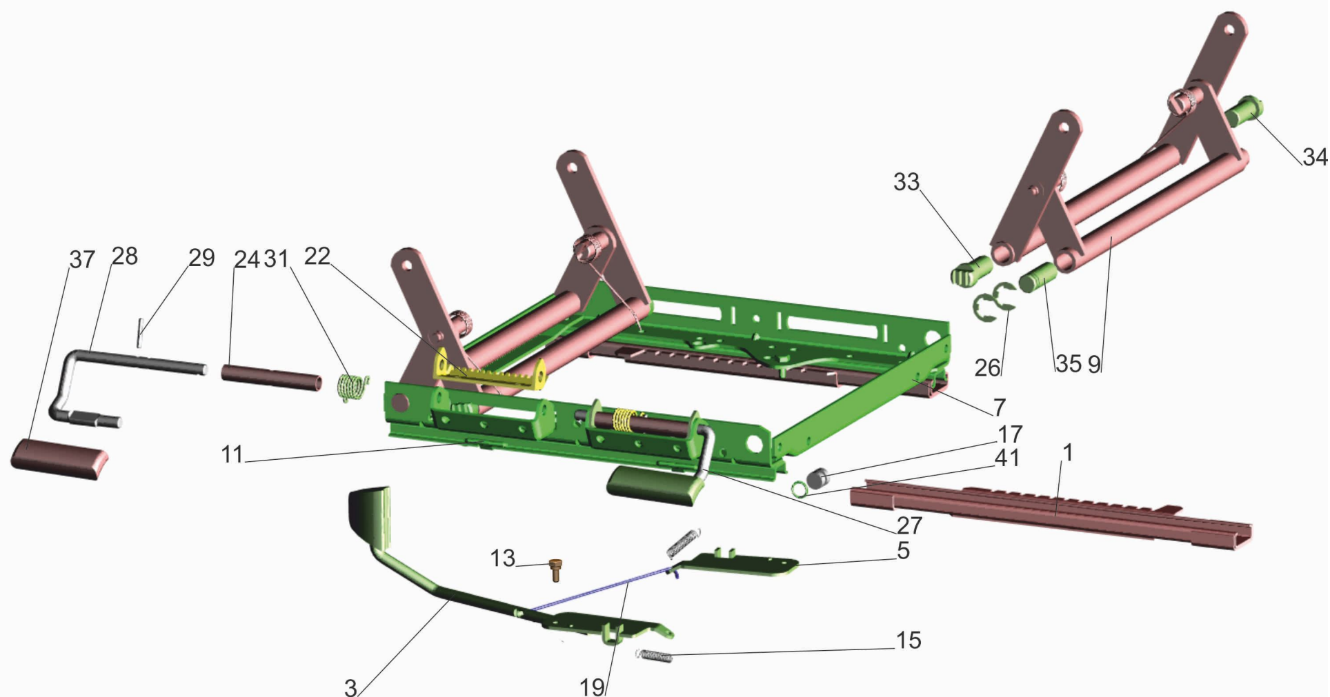
Рис.215 Механизм регулирования высоты 6430-6804100-010 Fig.215 Adjusting mechanisms of seat height 6430-6804100-010
