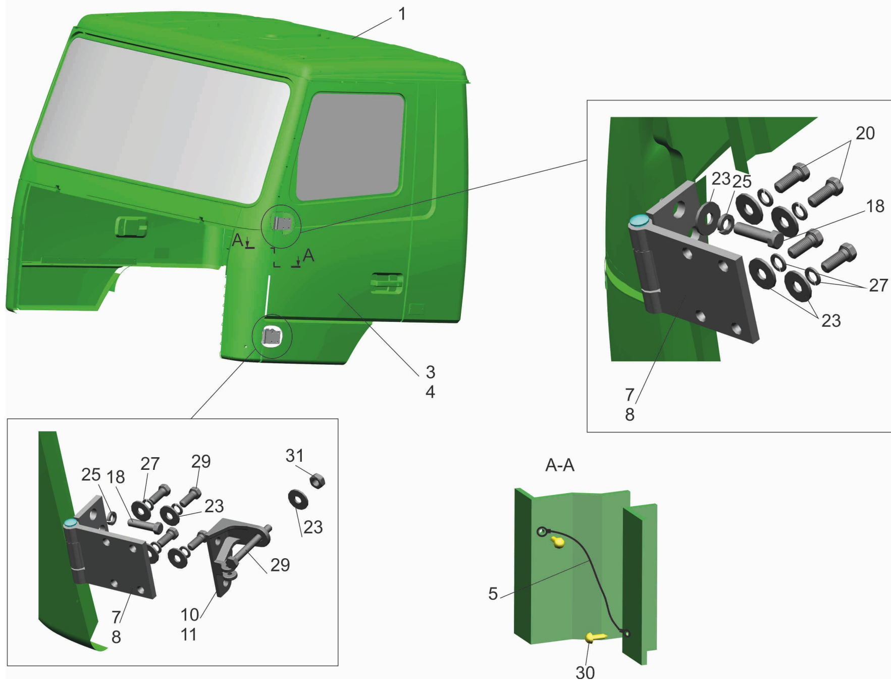
Рис.201 Кабина 4371-5000022-050, 4371-5000022-060 Fig.201 Cabin 4371-5000022-050, 4371-5000022-060
