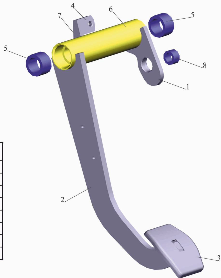
Рис.38 Педаль 6430-3504032, 64302-3504032 Fig.38 Pedal 6430-3504032, 64302-3504032
