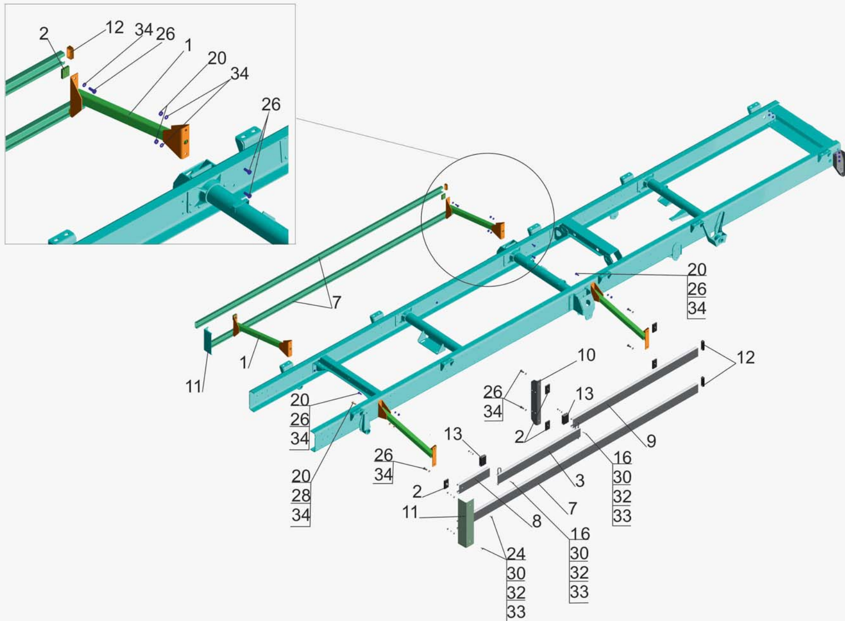
Рис.82 Установка бокового ограждения 4371W1-2800040-010 Fig.82 Installation of cross guard 4371W1-2800040-010
