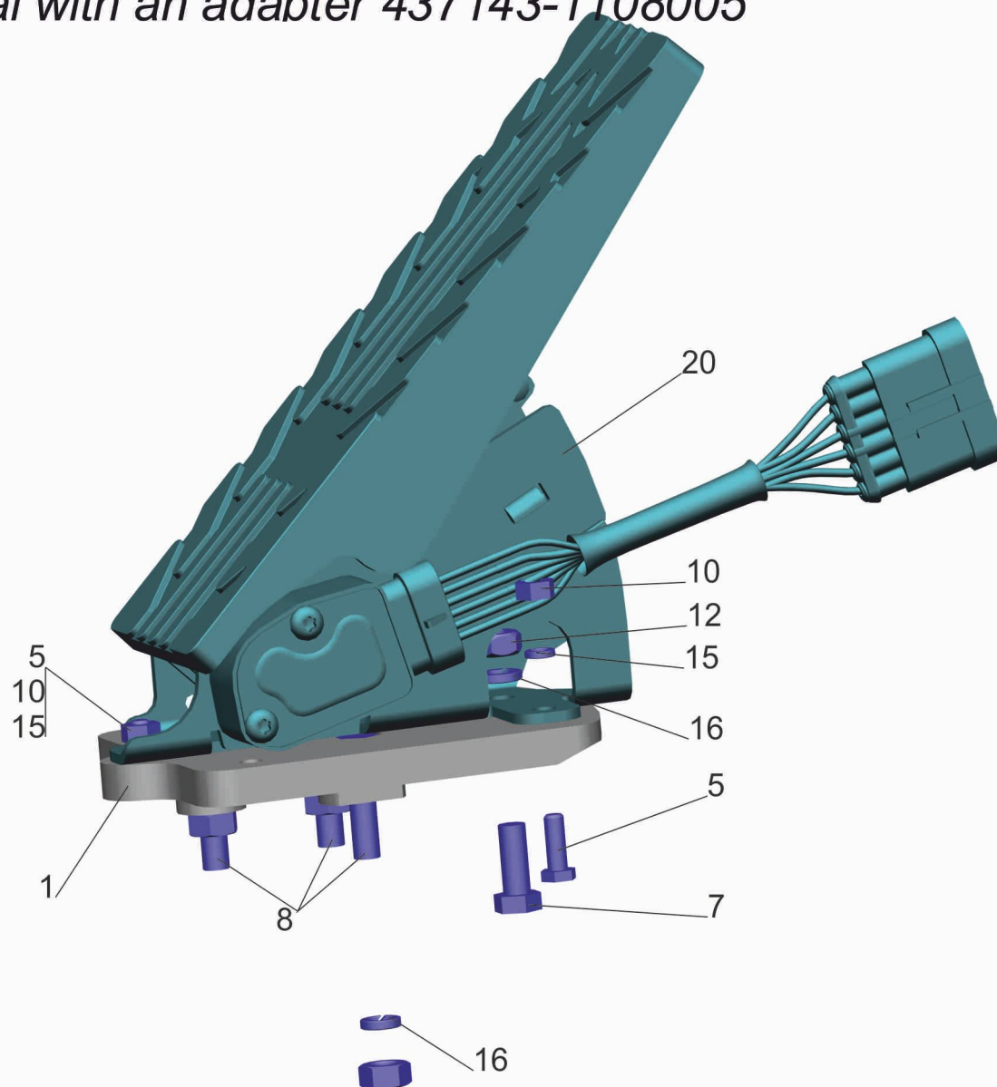
Рис. 21 Педаль с переходником 437143-1108005 Fig. 21 Pedal with an adapter 437143-1108005
