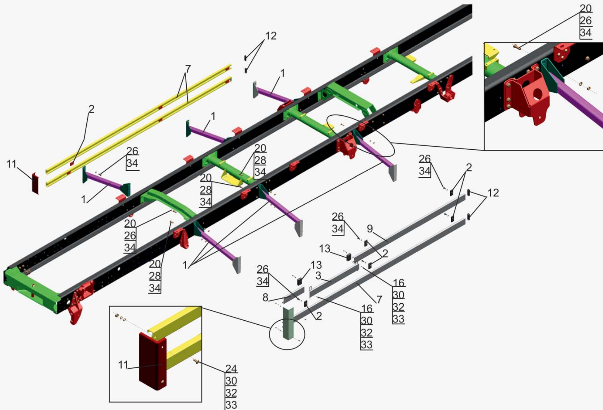
Рис.81 Установка бокового ограждения 4371W1-2800040-000 Fig.81 Installation of cross guard 4371W1-2800040-000
