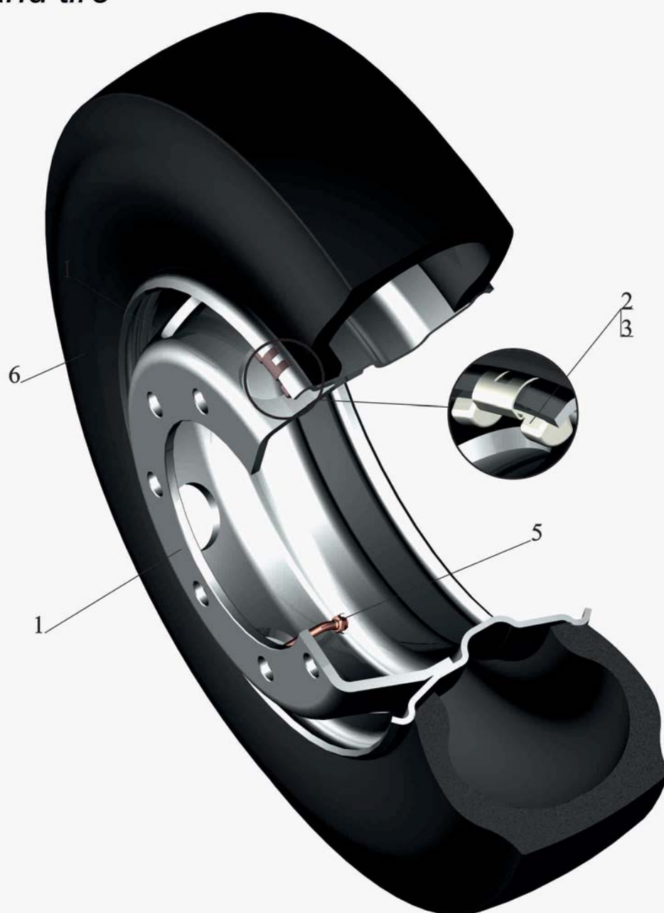
Рис.115 Колесо и шина Fig.115 Wheel and tire
