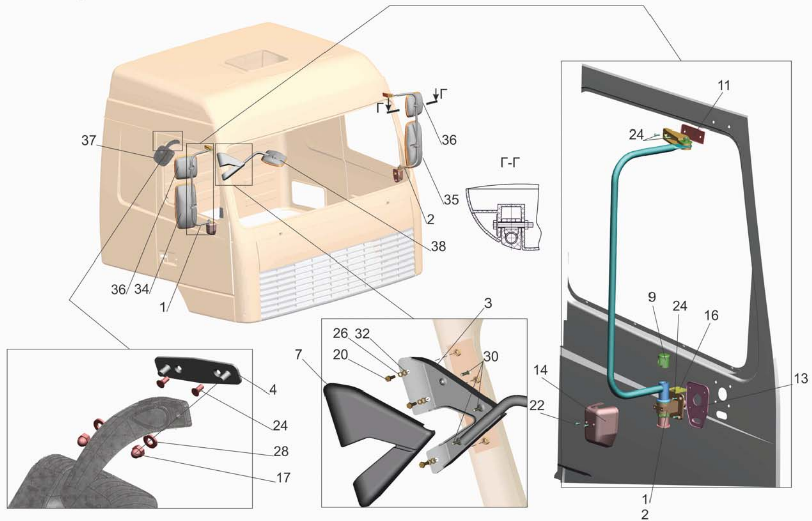
Рис.196 Установка зеркал 6430-8200005-010 Fig.196 Installation mirrors 6430-8200005-010
