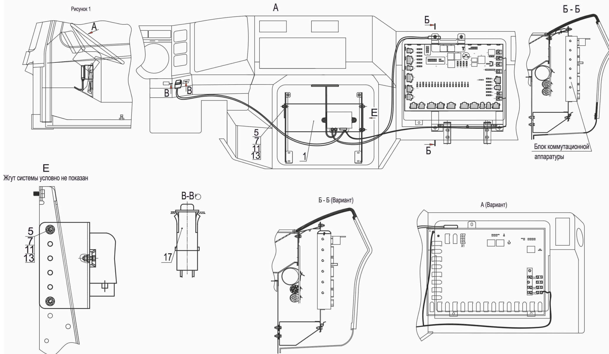
Рис. 170 Установка навигационного оборудования 643008-7937001-000 Fig. 170 Installation navigation equipment 643008-7937001-000
