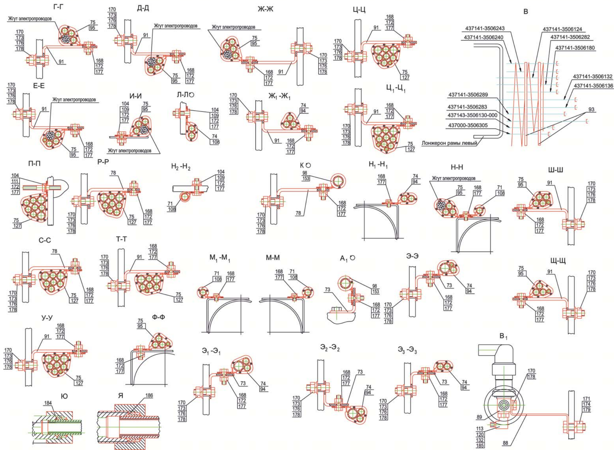
Рис.127 Установка пневмотормозов 4371Р2-3500003-040 (лист 2) Fig.127 Installation pneumobrakes
