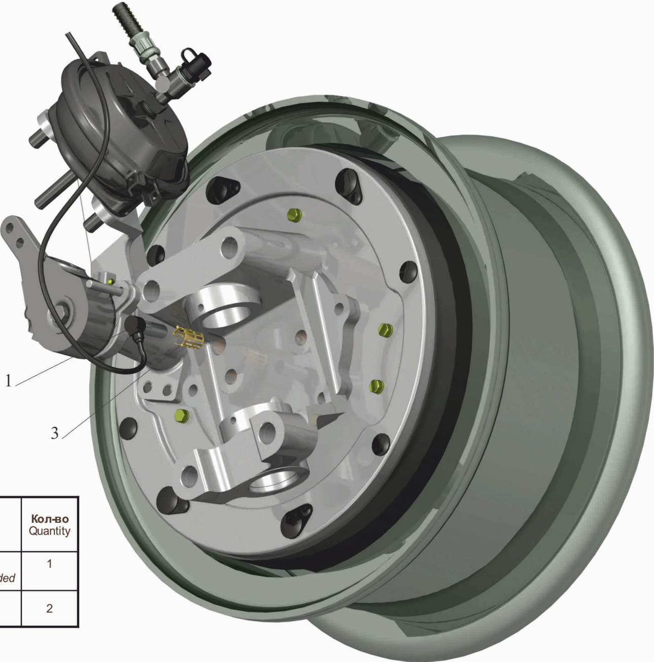
Рис. 173 Установка датчика АБС с кабелем на переднем колесе 437137-3538101 Fig. 173 Mounting of ABS sensor with the cable on the front wheel 437137-3538101
