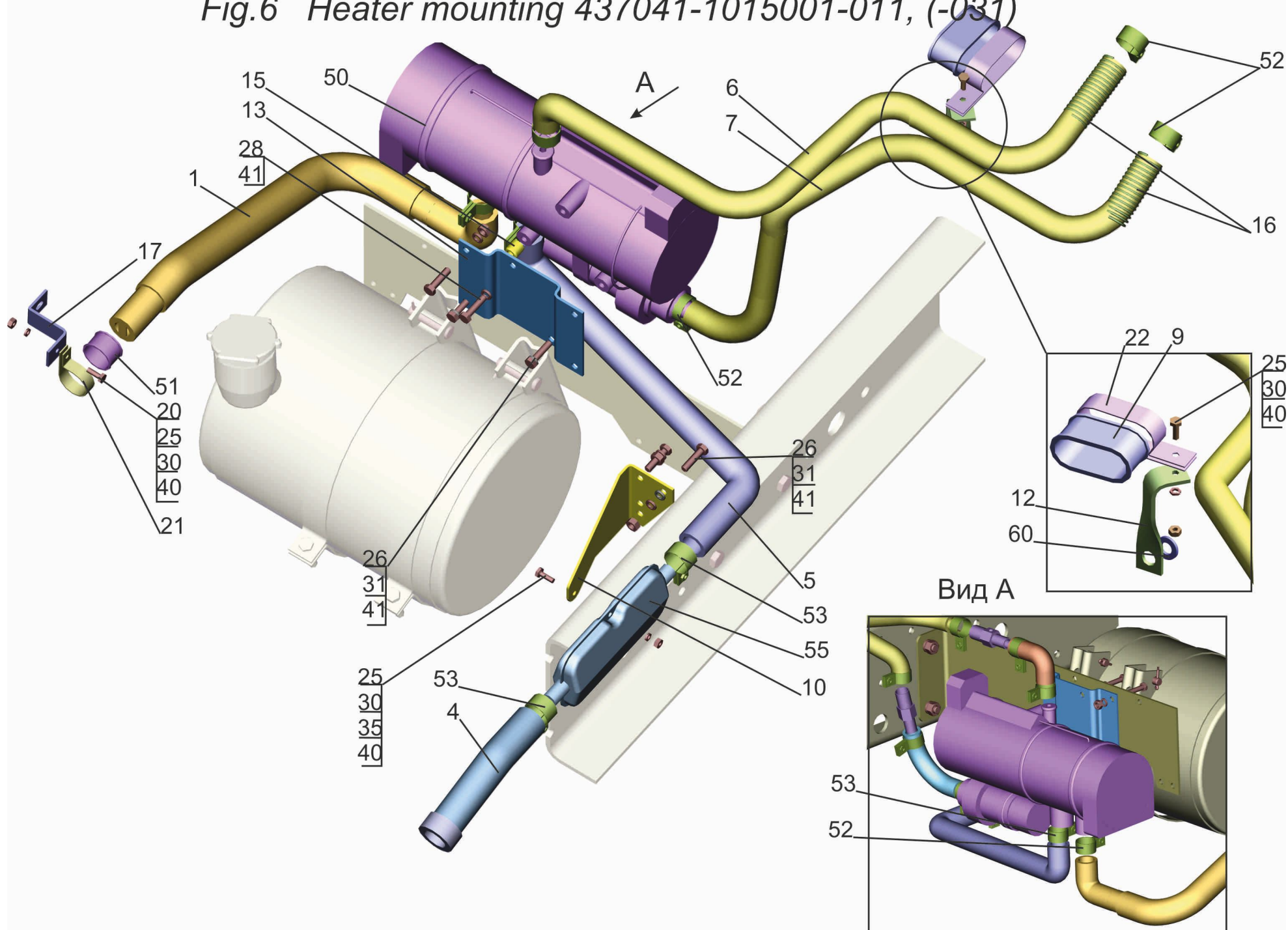
Рис.6 Установка подогревателя 437041-1015001-011, (-031)
