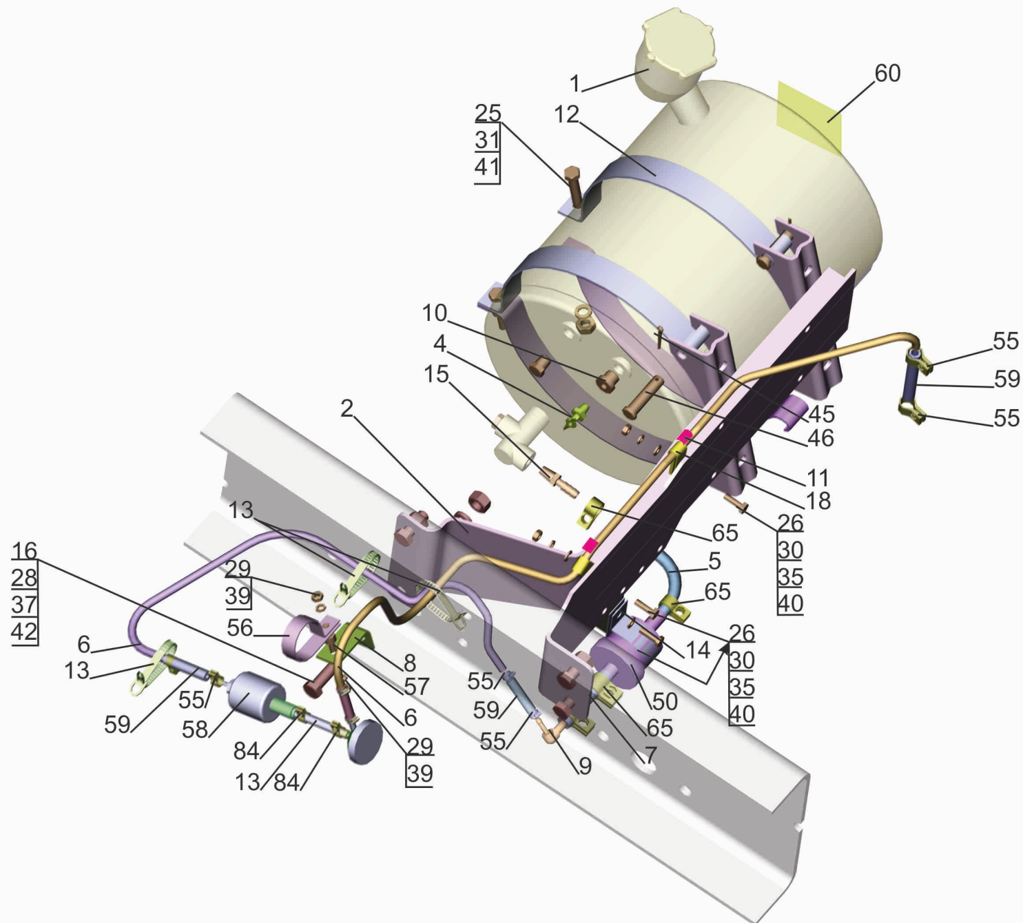
Рис. 9 Крепление топливопроводов подогревателя 4371P2-1015004-010 Fig. 9 Mounting fuel lines of heater 4371P2-1015004-010
