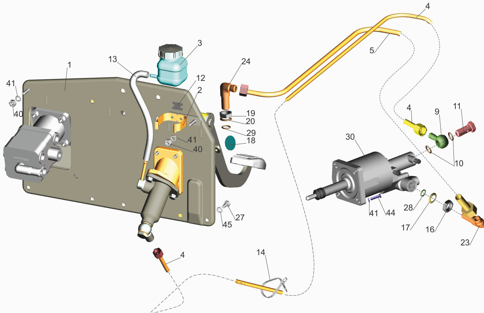
Рис. 31 Установка механизма управления сцеплением 437141-1600005-011 Fig. 31 Installation of a clutch-operating device 437141-1600005-011
