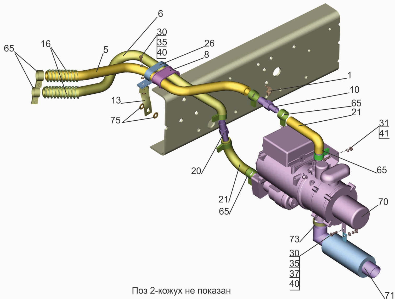
Рис. 4 Крепление подогревателя 437143-1015001-000, (-010) Fig. 4 Heater mounting 437143-1015001-000. (-010)
