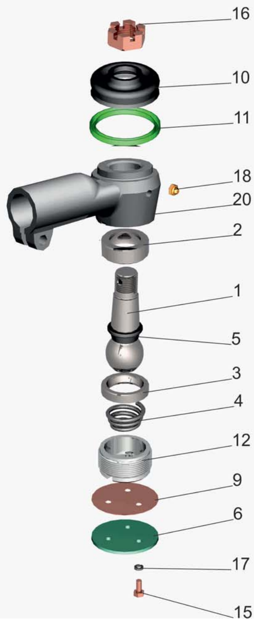
Рис.98 Наконечник 4370-3003056 Fig.98 Nozzle 4370-3003056
