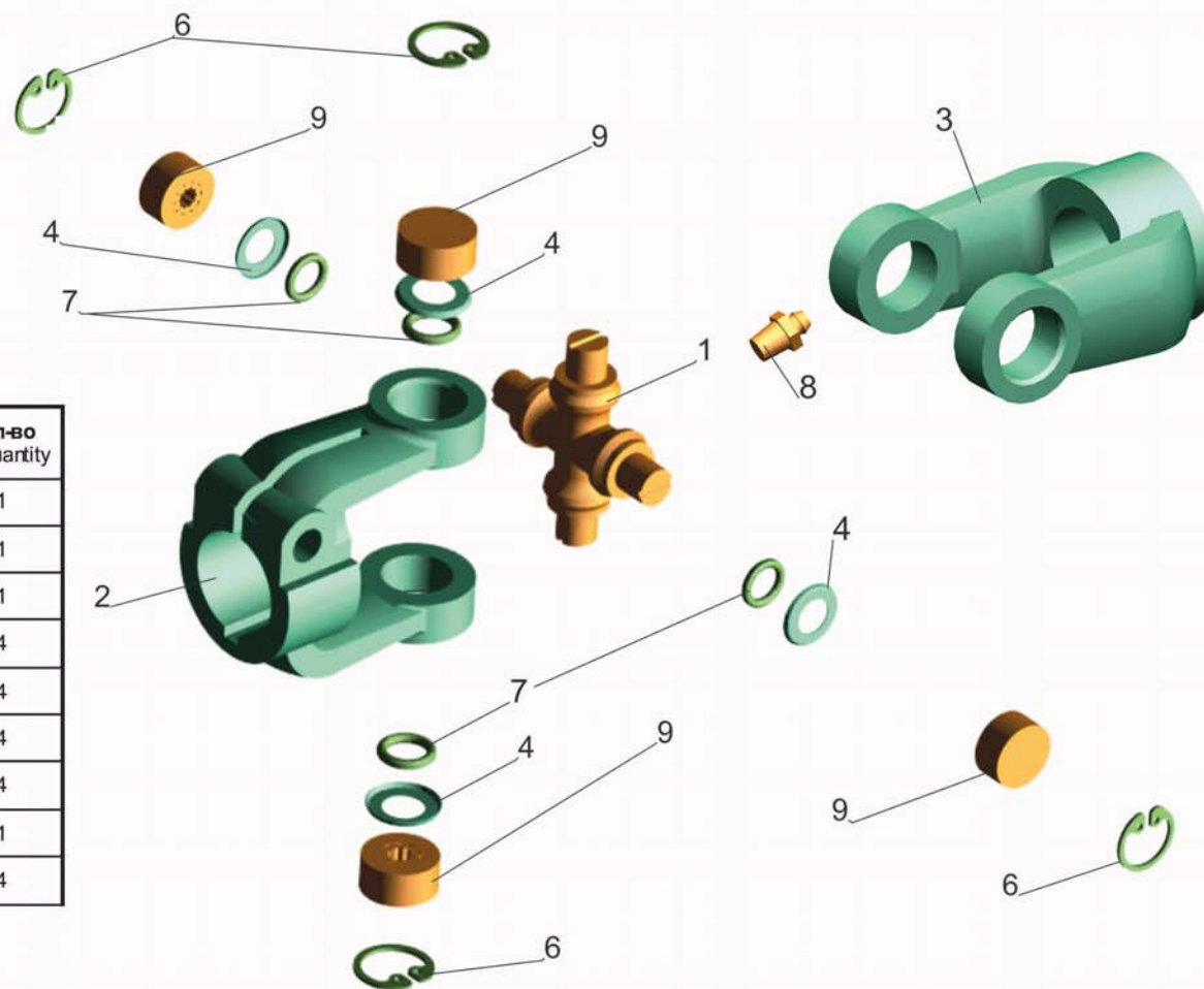
Fig. 124 Hinge cardan 6430-3444052-010
