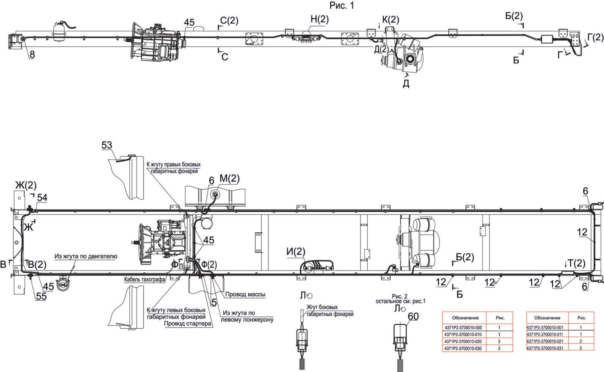
Рис. 145 Установка электрооборудования на шасси Лист 1 Fig. 145 Electric equipment installation on the chassis Page 1
