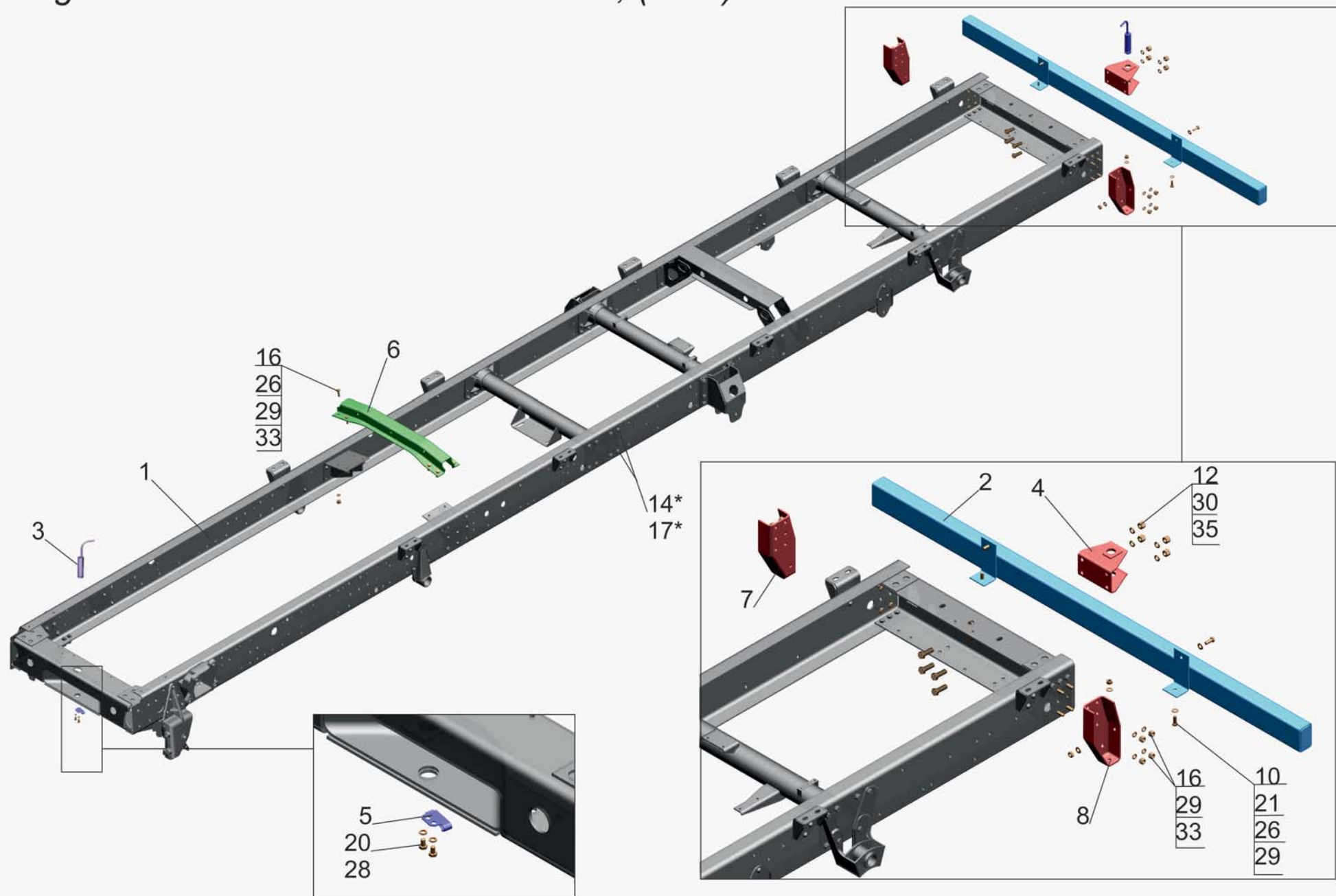
Рис. 76 Рама 4371P2-2800010-005, (-015) Fig.76 Frame 4371P2-2800010-005, (-015)
