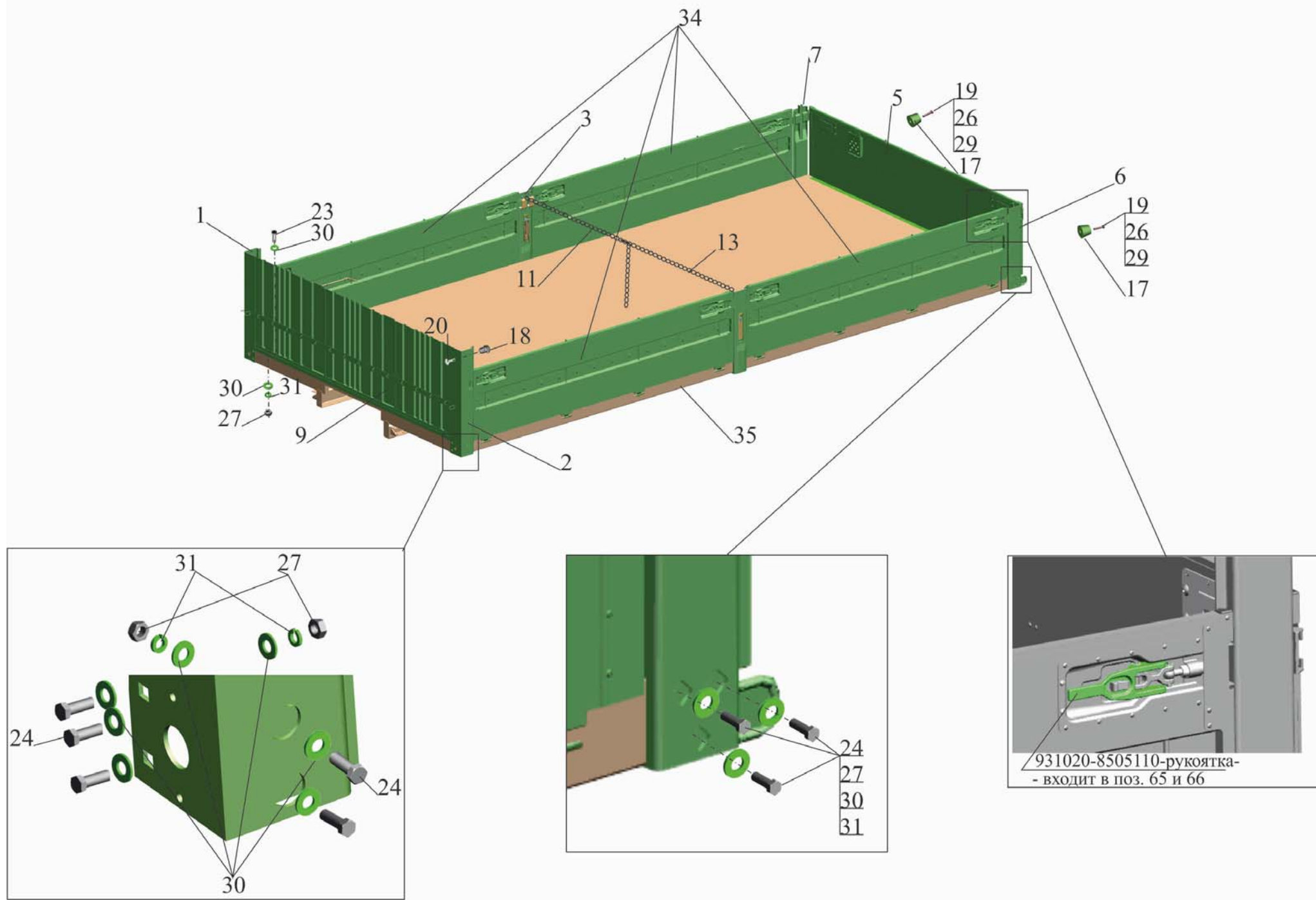
Рис. 249 Платформа 4371-8500020-110(-130) Fig. 249 Platform 4371-8500020-110(-130)
