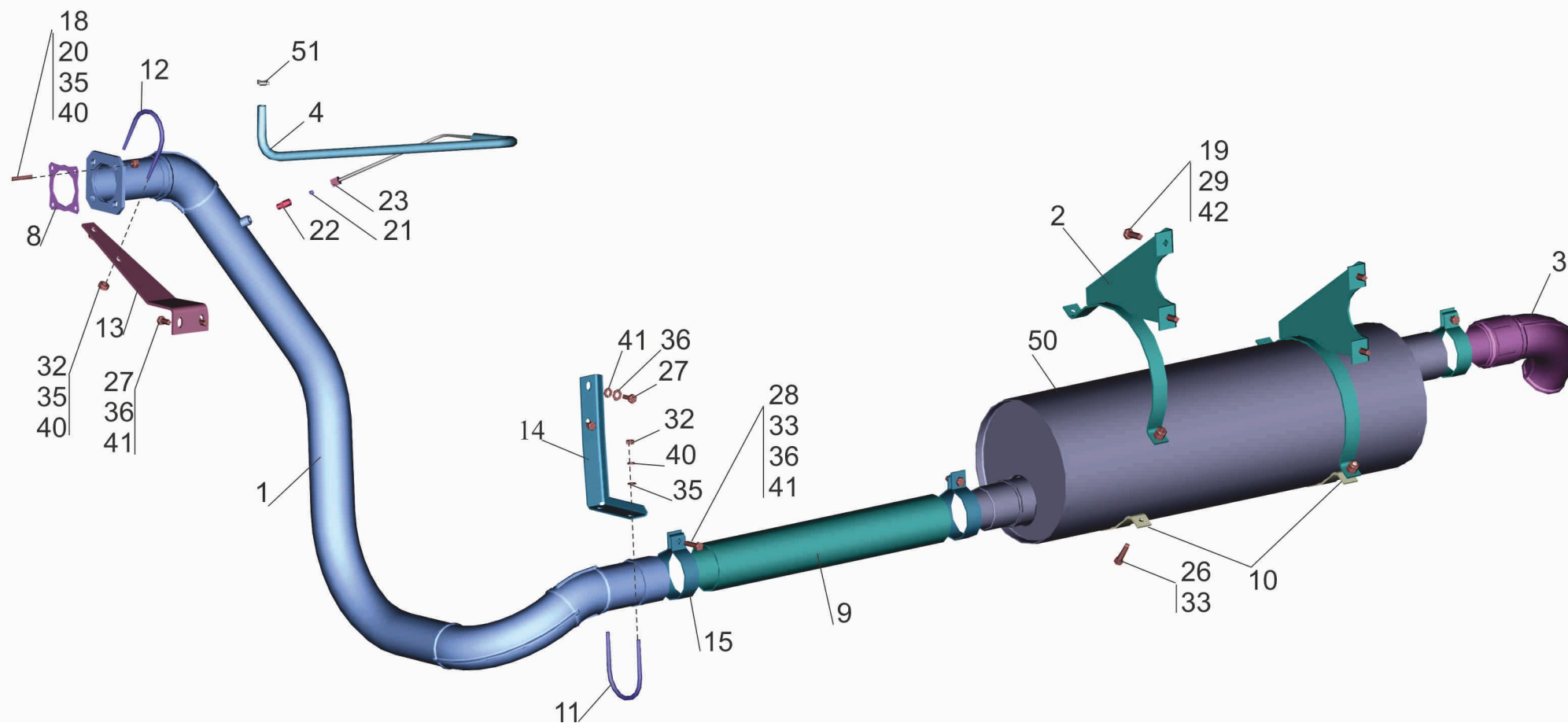
Рис.24 Установка системы выпуска газов 4371P2-1200001-010 Fig.24 Mounting of gas release system 4371P2-1200001-010
