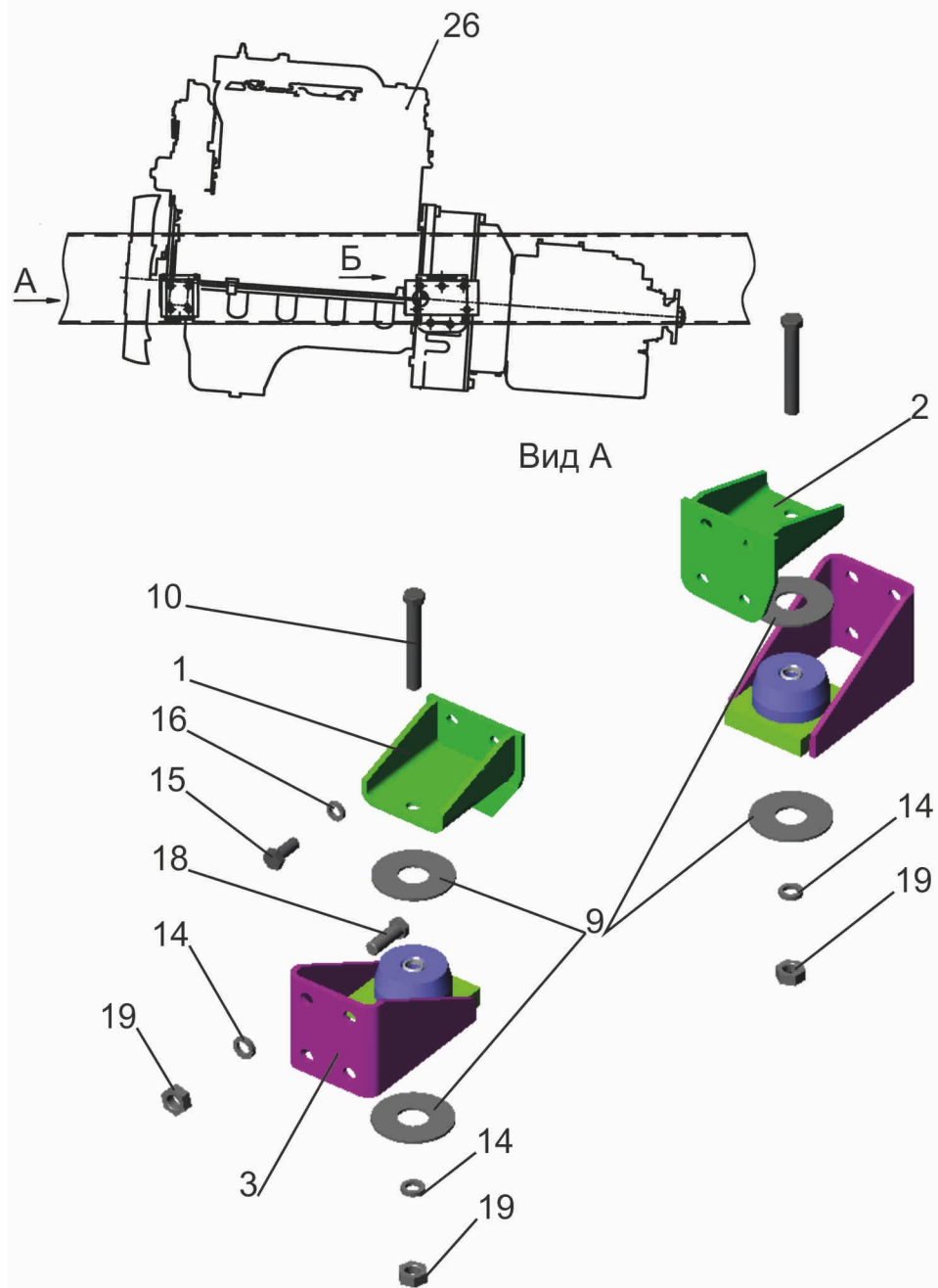
Рис.3 Крепление двигателя Fig.3 Engine mounting
