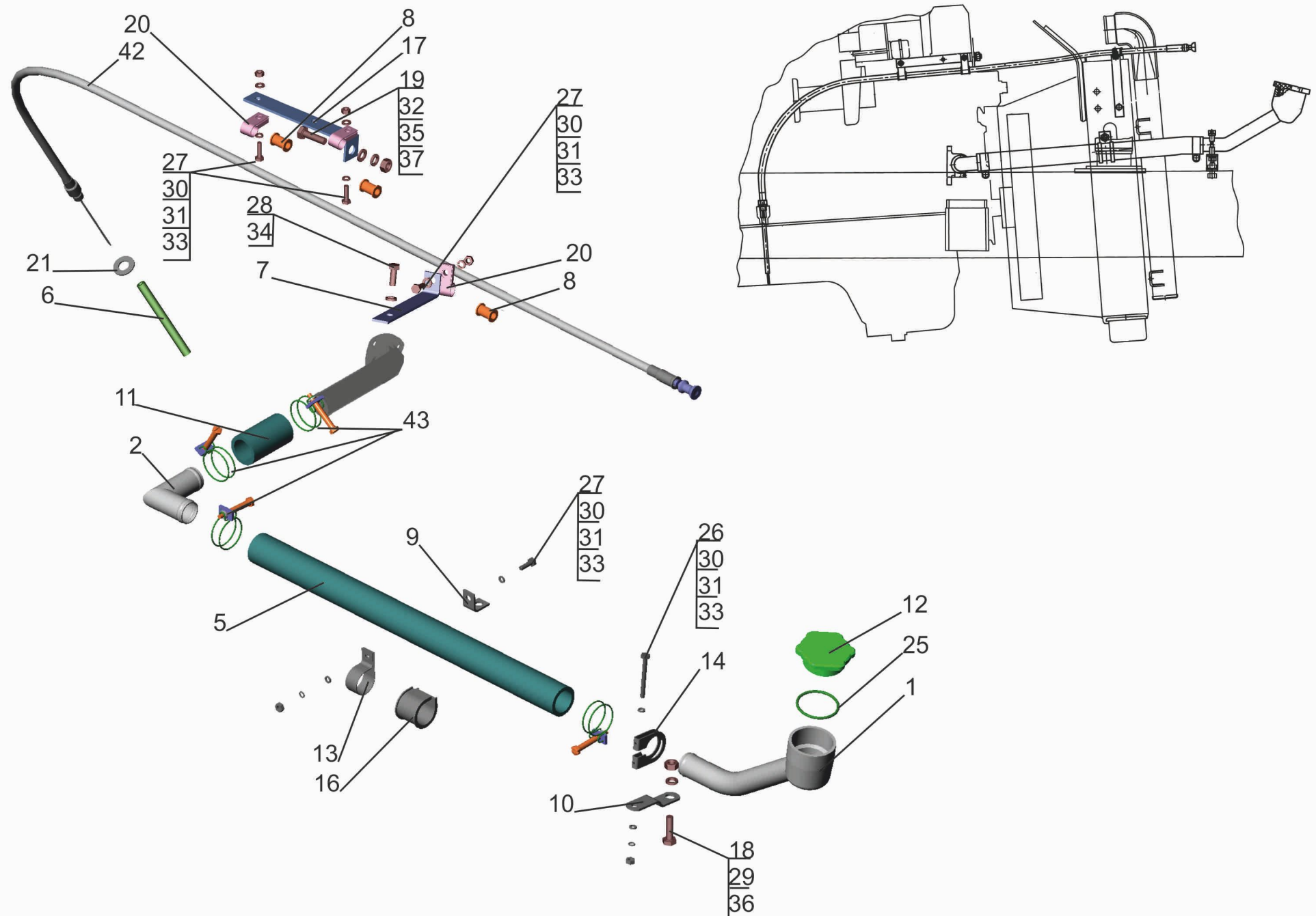
Рис.2 Крепление системы заливки и контроля уровня масла 4381P2-1018002-000 Fig.2 System of oil priming and its level checking 4381P2-1018002-000.
