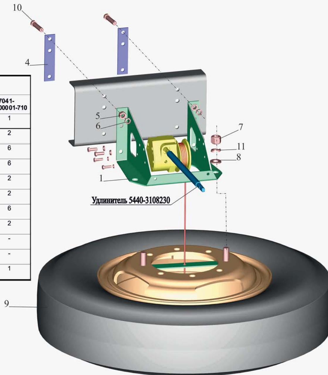
Рис. 109 Установка запасного колеса Fig. 109 Installation spare wheel
