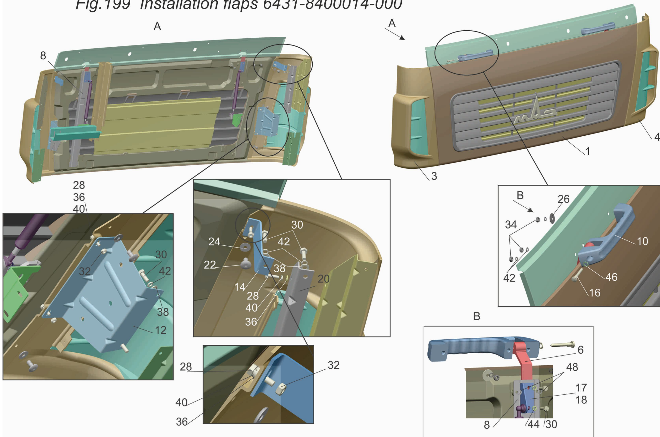
Рис. 199 Установка щитков 6431-8400014-000
