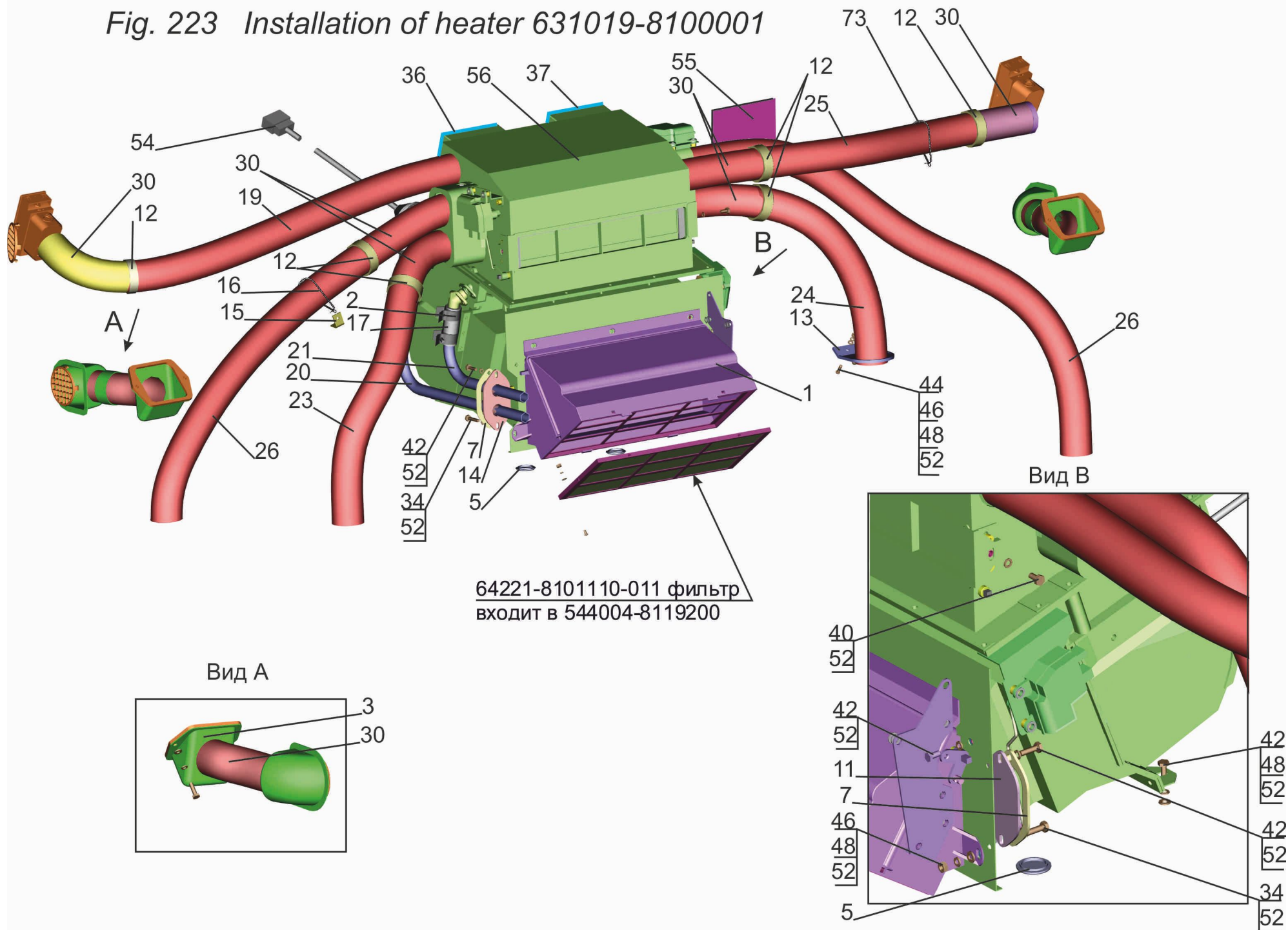
Рис. 223 Установка отопителя 631019-8100001
