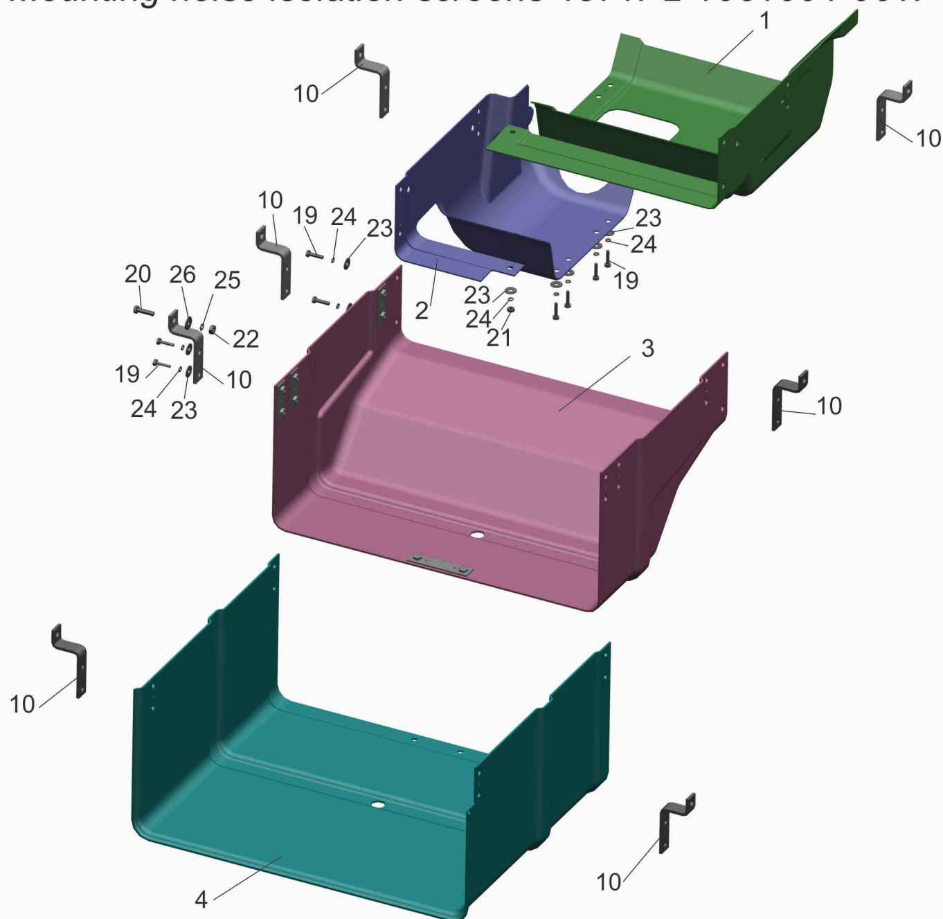
Рис. 12 Установка шумоизоляционных экранов 4371P2-1061004-061. Fig. 12 Mounting noise isolation screens 4371P2-1061004-061.
