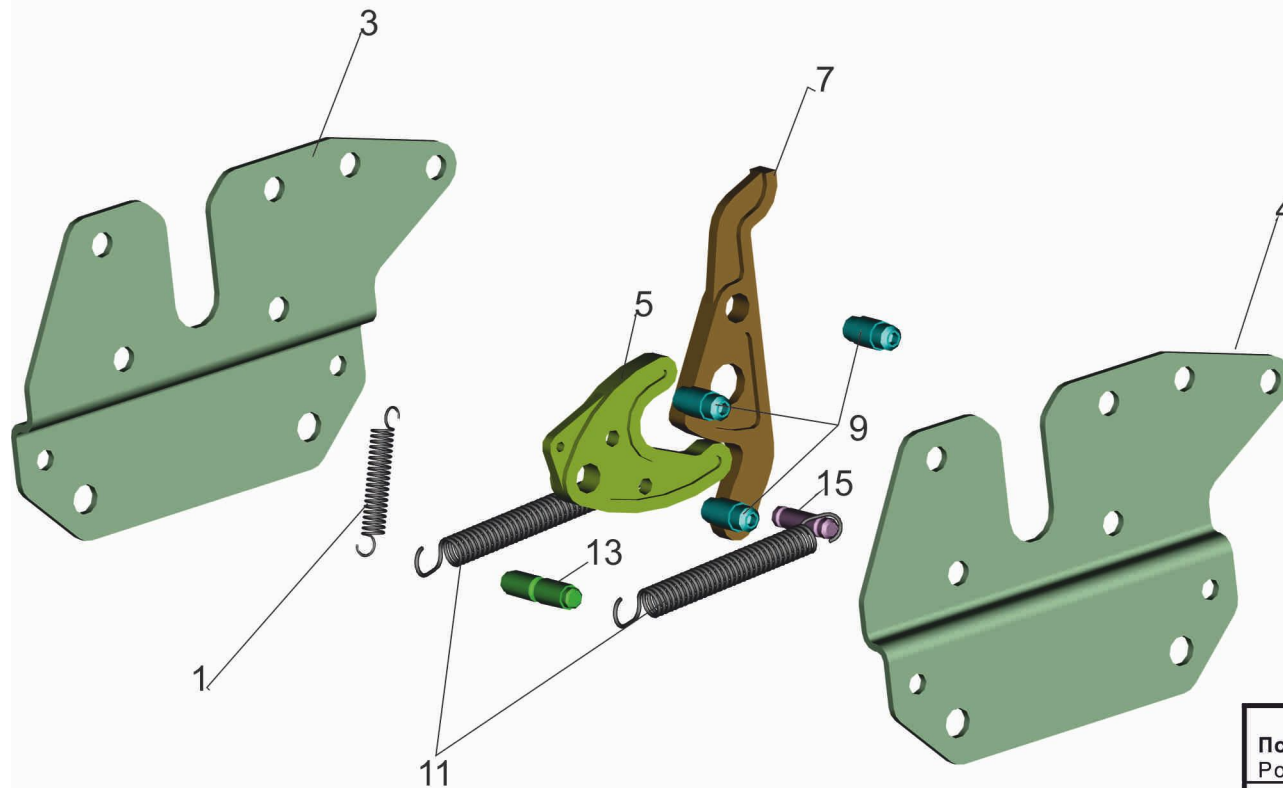
Рис.180 Запорный механизм кабины 6501-5001550 Fig.180 Cab lock mechanism 6501-5001550
