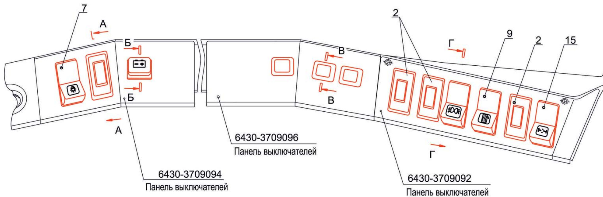
Рис.147 Установка выключателей 4371W1-3700018-000 Fig.147 Installation of switches 4371W1-3700018-000
