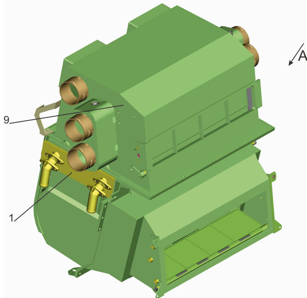
Рис 228 Отопитель 650118-8101010 Fig 228 Heater 650118-8101010
