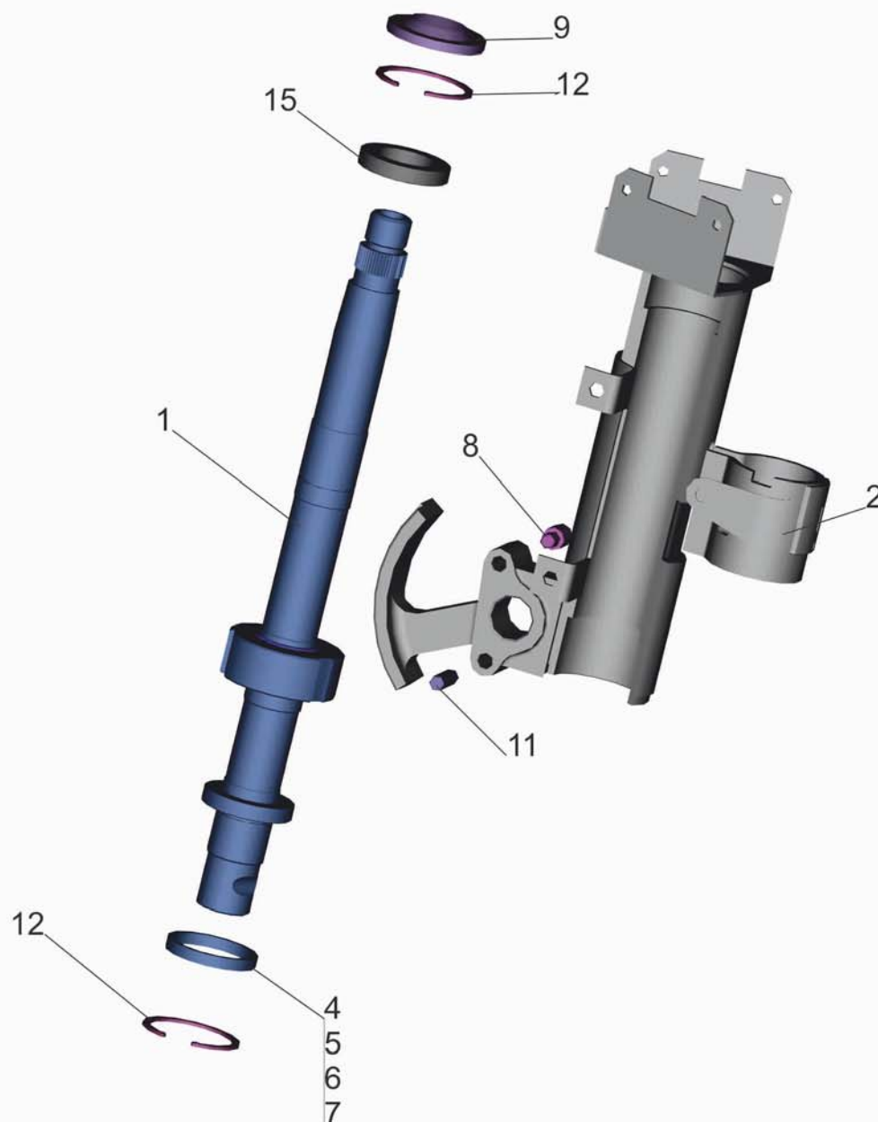
Рис. 119 Колонка 5440-3444010 Fig. 119 Column 5440-3444010
