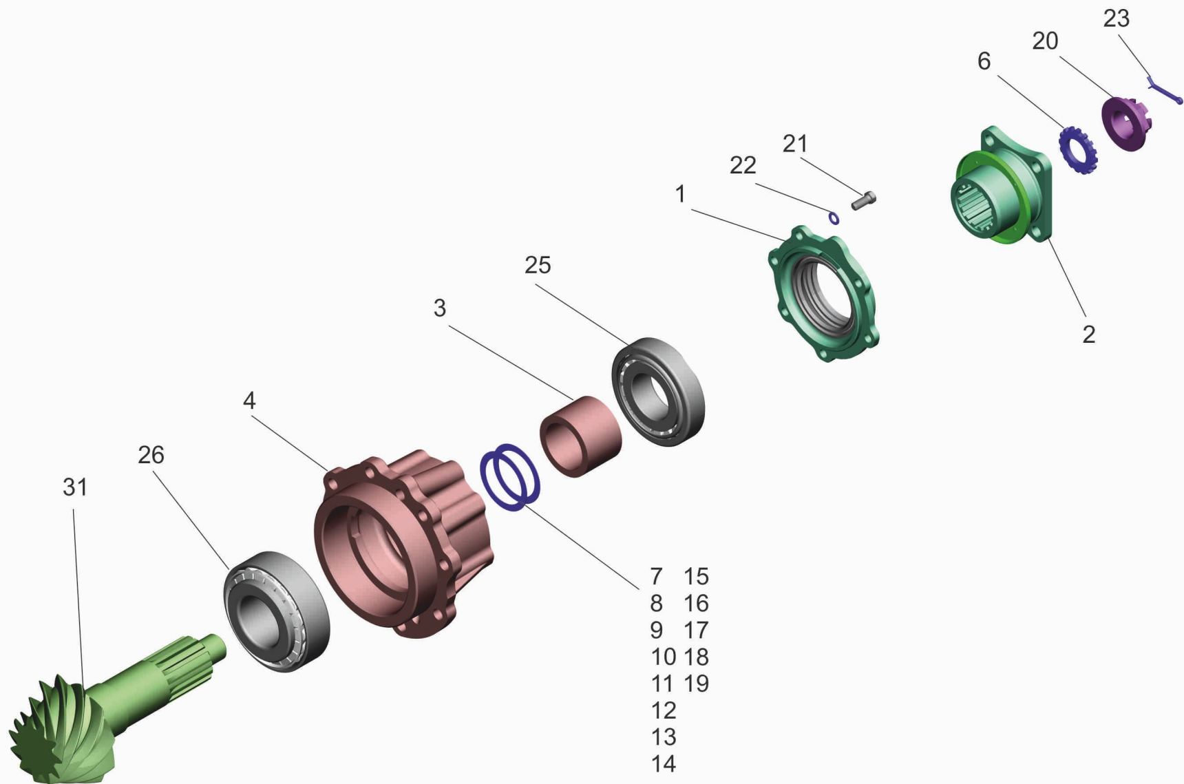
Рис.68 Шестерня ведущая Fig.68 Drive pinion
