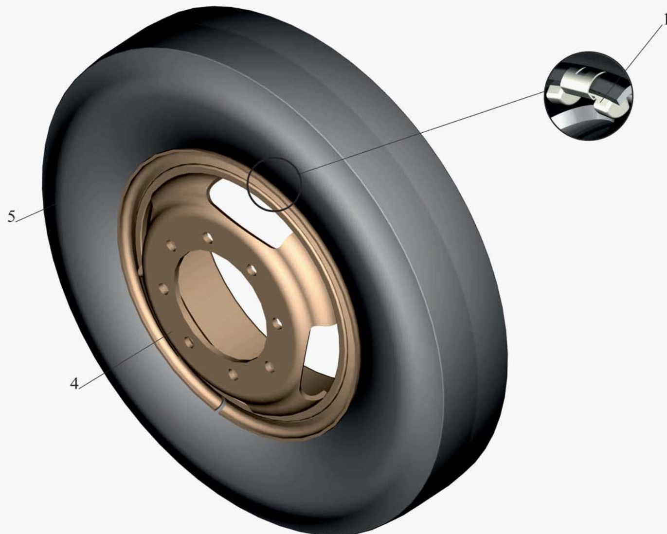
Рис. 116 Колесо и шина 457041-3101011(-010) Fig. 116 Wheel and tire 457041-3101011(-010)
