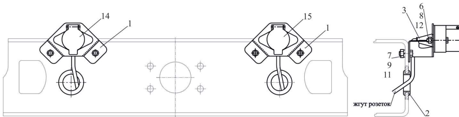
Рис.146 Установка штепсельных розеток Fig.146 Installation of outlet sockets
