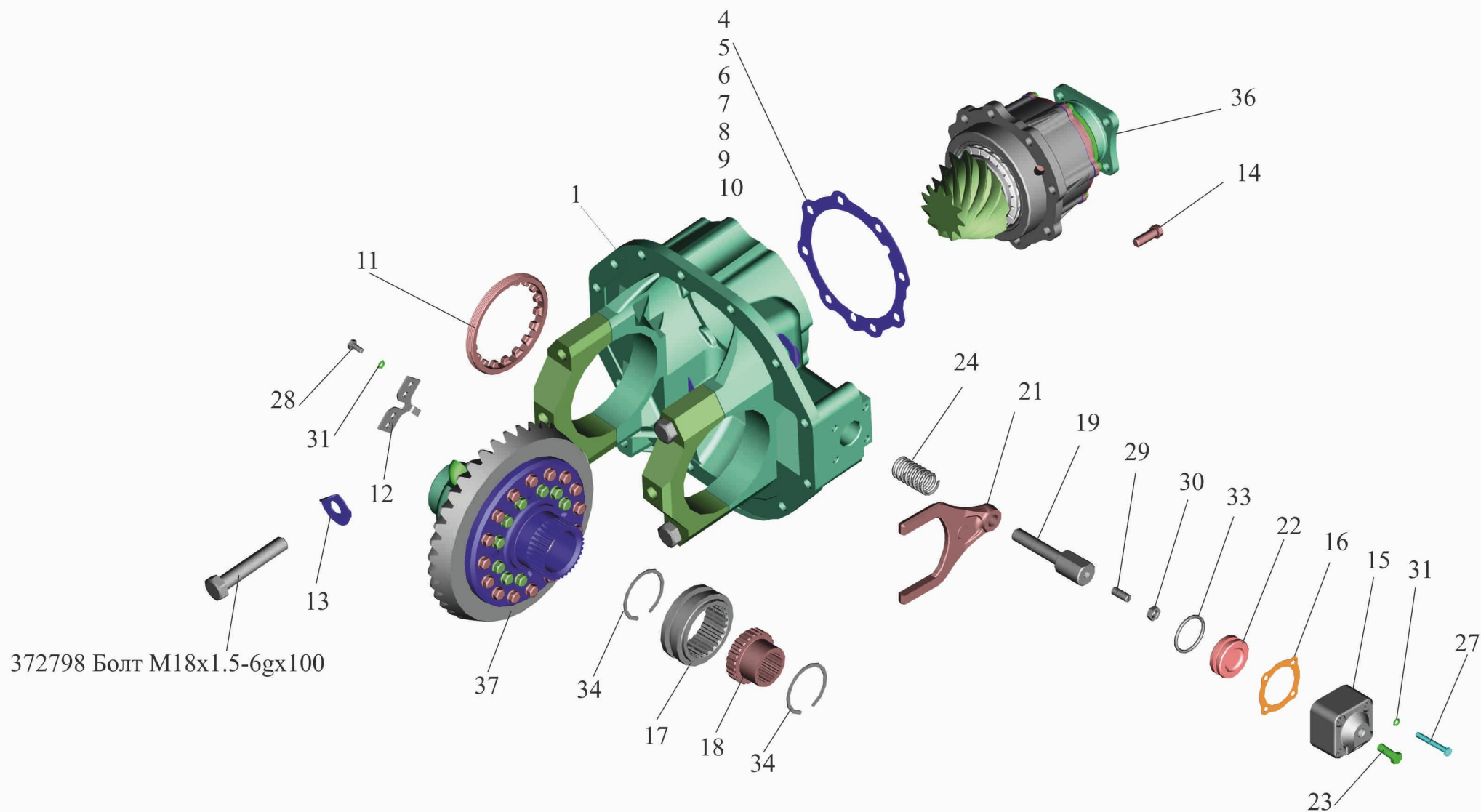
Рис. 66 Редуктор заднего моста. Fig. 66 Rear Axle Reduction Gear.
