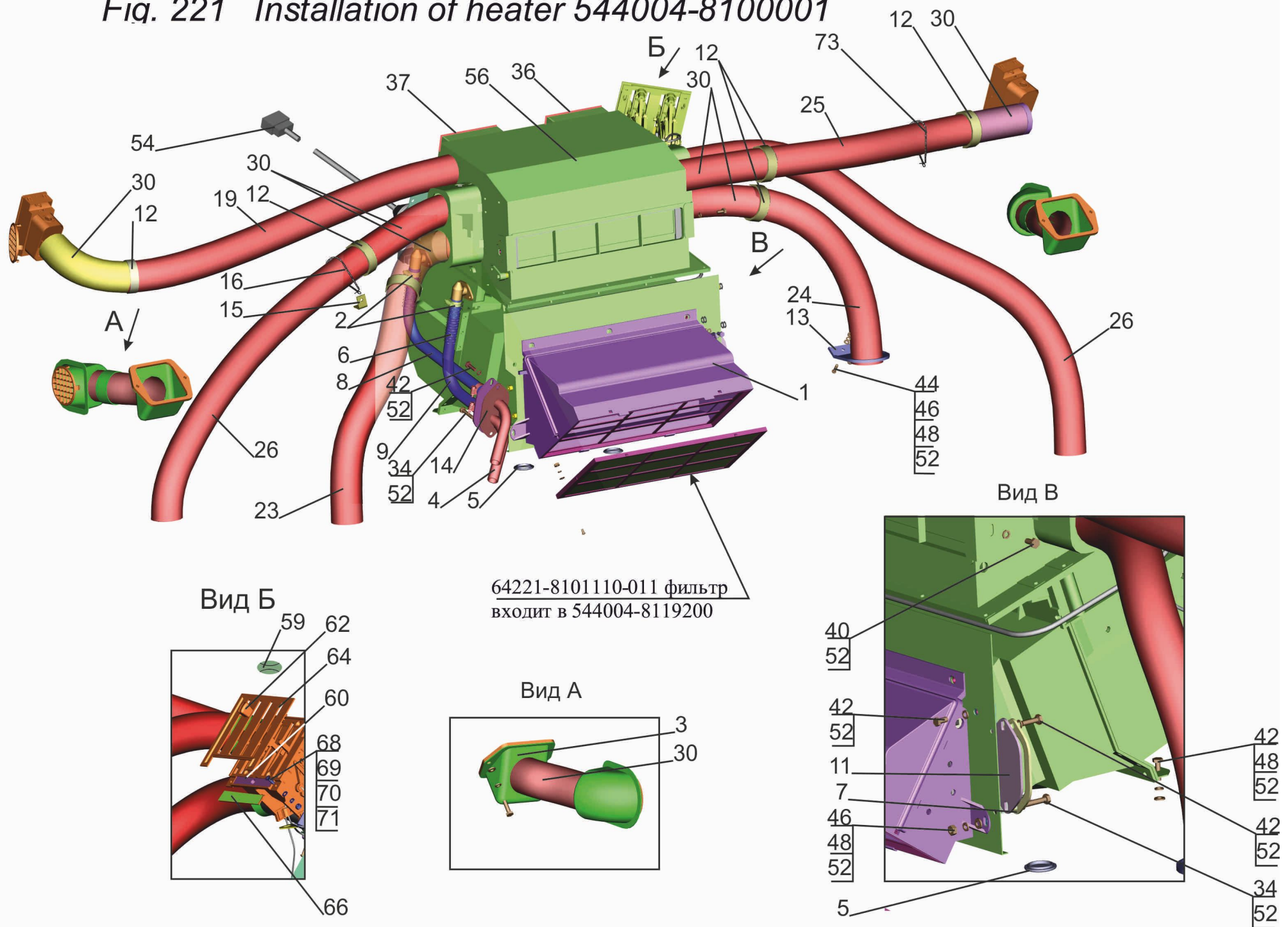
Рис. 221 Установка отопителя 544004-8100001
