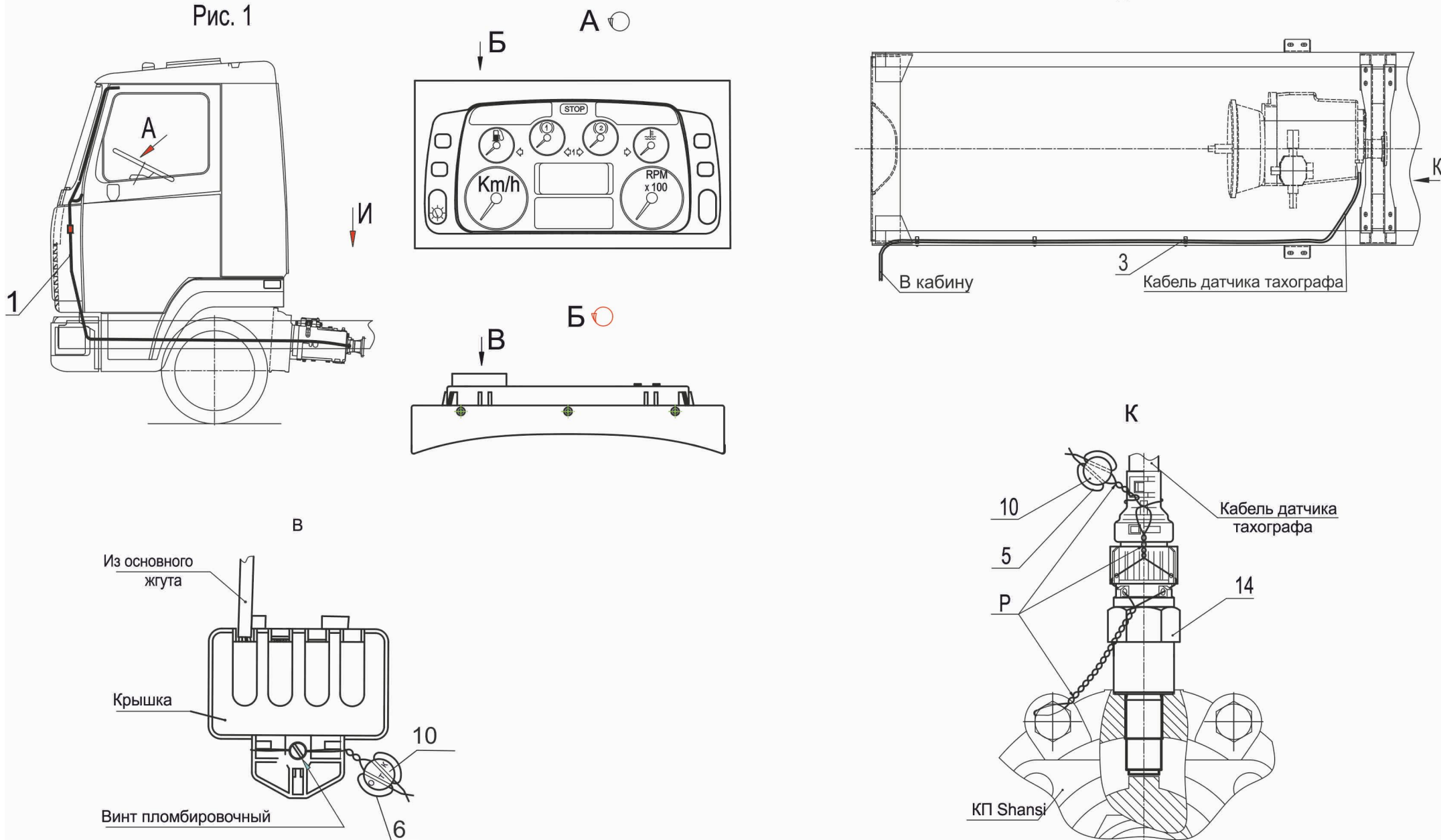
Рис.163 Установка и пломбировка спидометра 4371P2-3800004-030 Fig.163 Installation and identification seal of speedometer 4371P2-3800004-030
