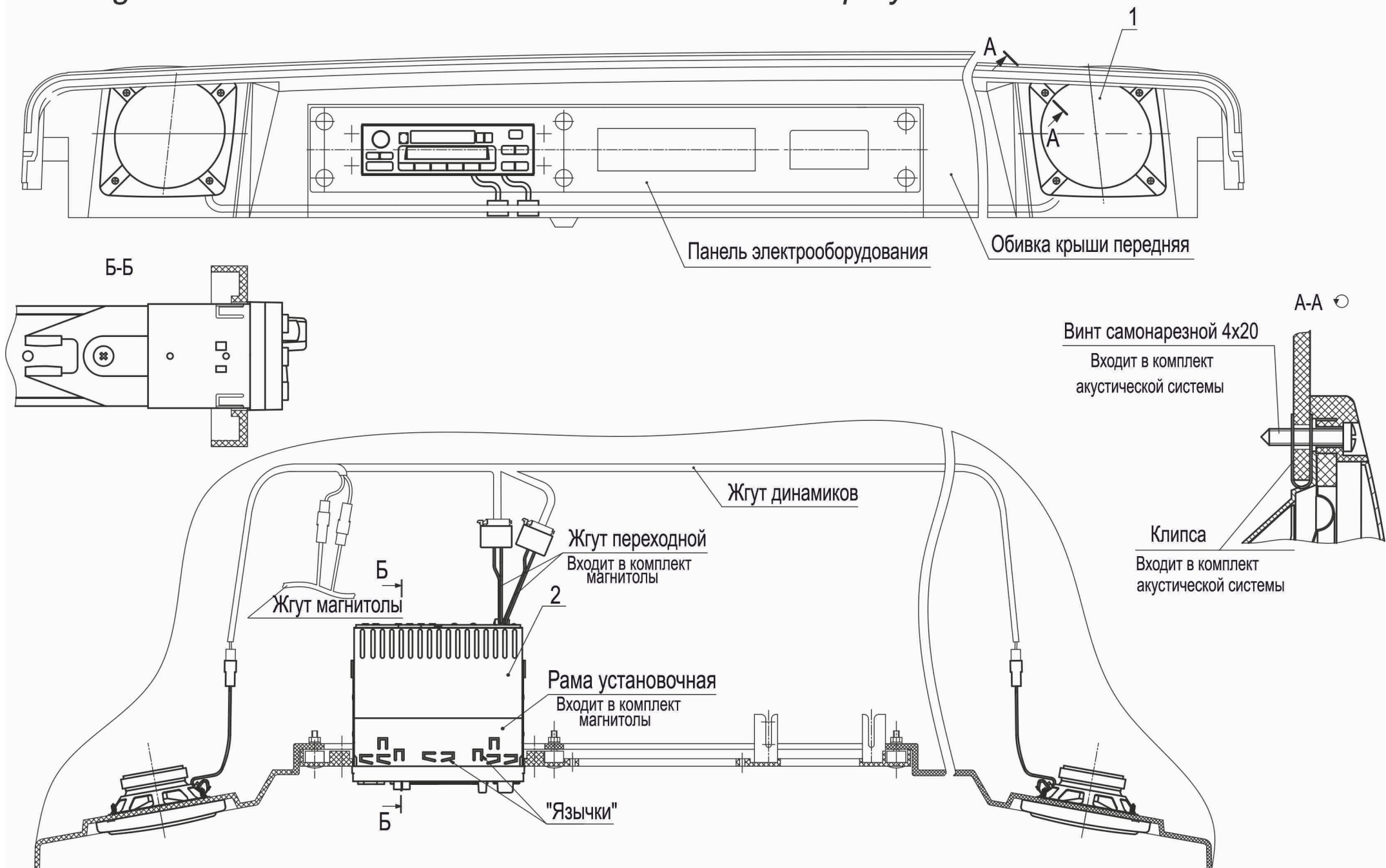
Рис.165 Установка радиоприемника с CD проигрывателем 6501-7900030 Fig.165 Installation of a radio receiver from CD a player 6501-7900030
