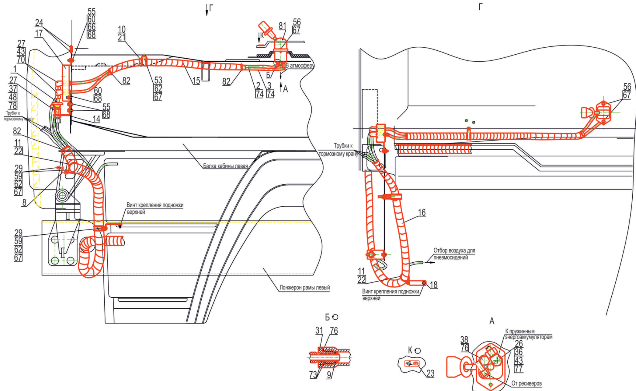
Рис. 140 Привод стояночного тормоза 4371Р2-3537006-010 Fig. 140 Drive gear of parking brake
