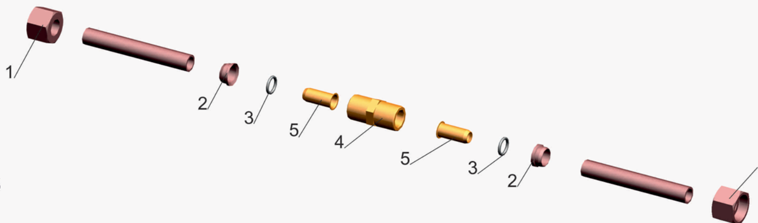
Рис. 142 Соединение для ремонта поврежденных трубопроводов Fig. 142 Connection for repair of the damaged pipelines
