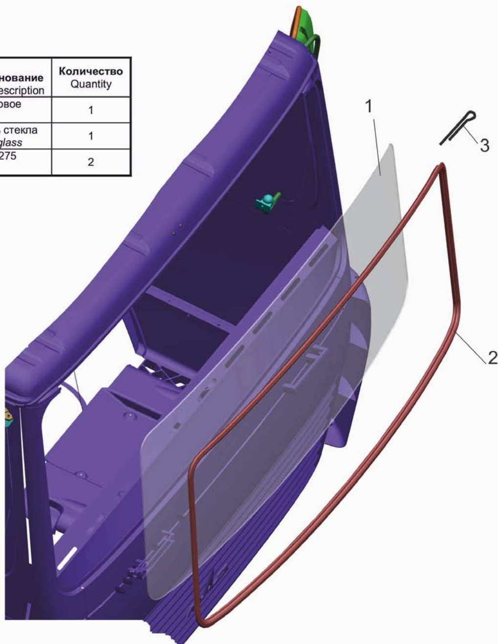
Рис. 186 Установки стекла 6430-5200010 Fig. 186 Installation of a glass 6430-5200010
