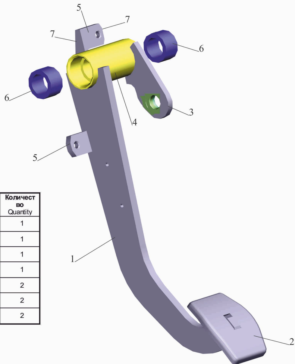
Рис. 33 Педаль 6430-1602112, 64302-1602112 Fig. 33 Pedal 6430-1602112, 64302-1602112
