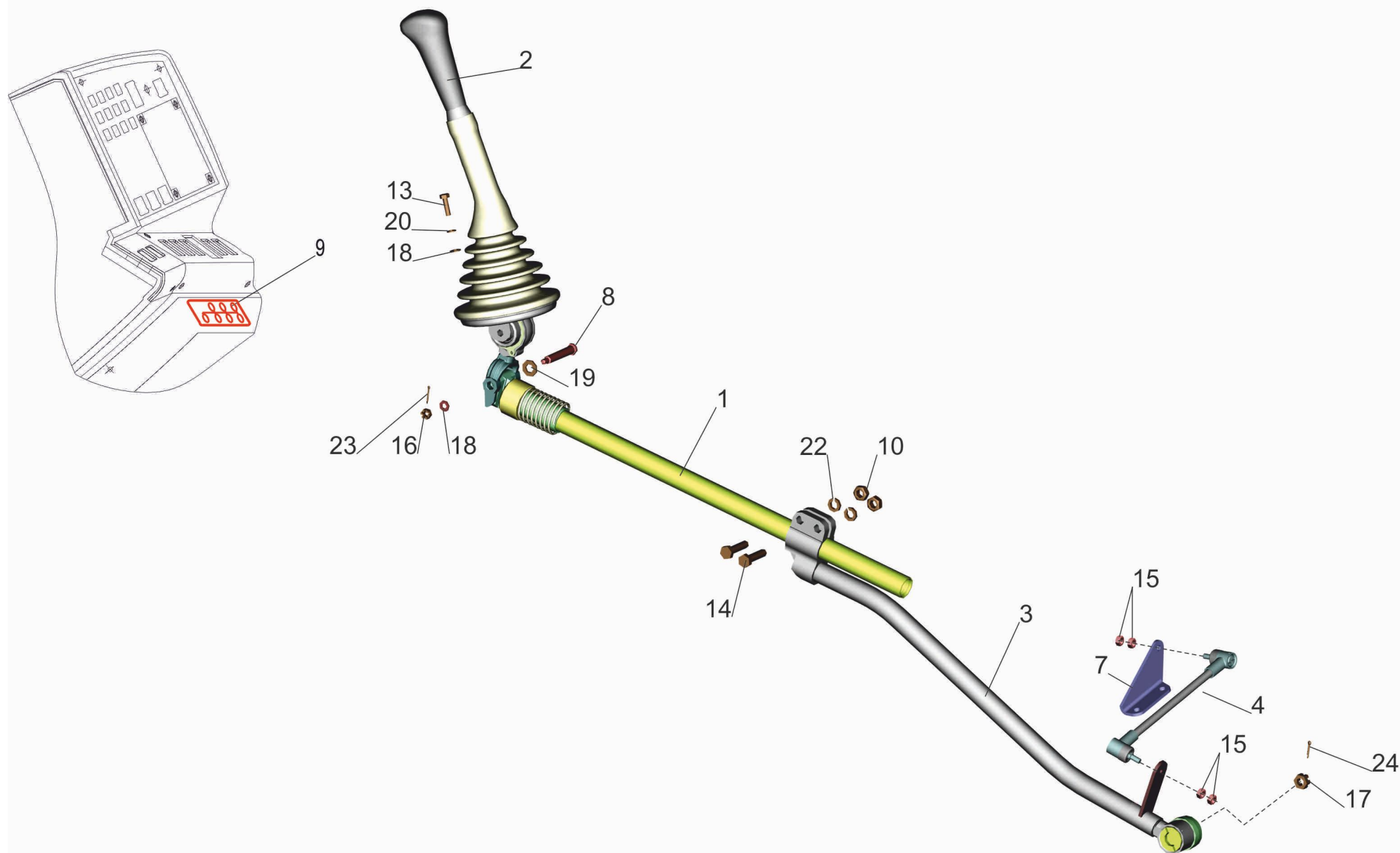
Рис. 40 Установка привода управления коробкой передач 4571P2-1700002-000 Fig. 40 Installation drive of control of gear box 4571P2-1700002-000
