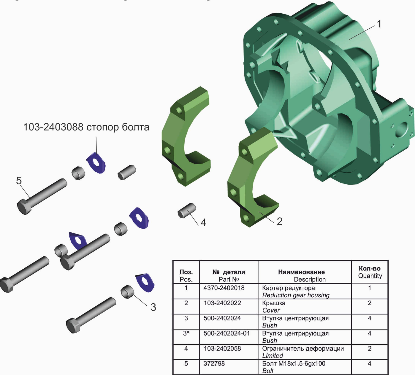
Рис.67 Картер редуктора 4370-2402015 Fig.67 Reductor gear housing 4370-2402015
