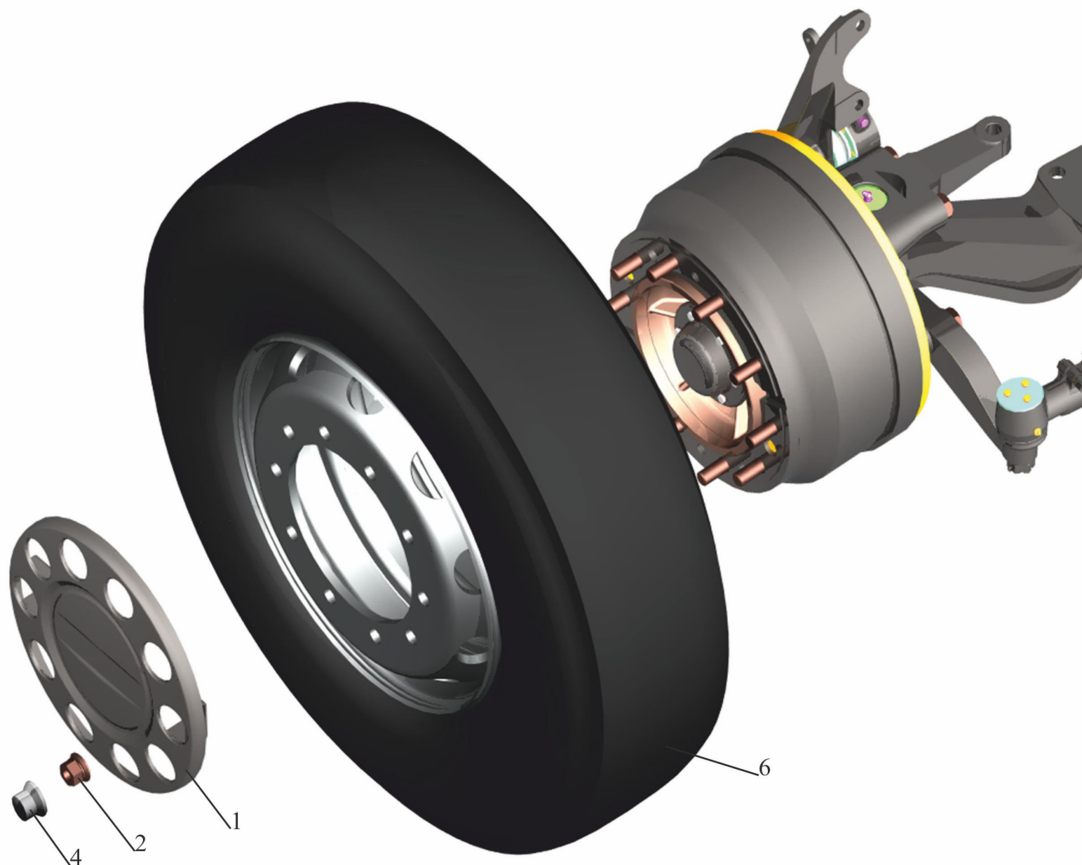
Рис. 143 Установка передних колес Fig. 143 Installation of front wheels
