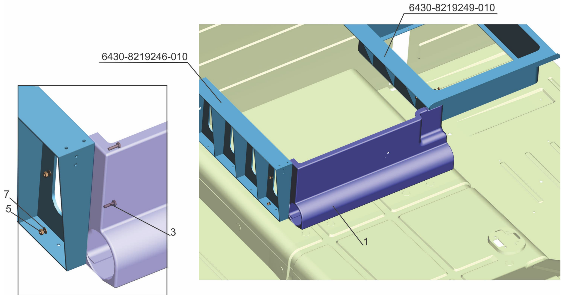
Рис. 253 Установка стенки 6430-8200041 Fig. 253 Installation wall 6430-8200041
