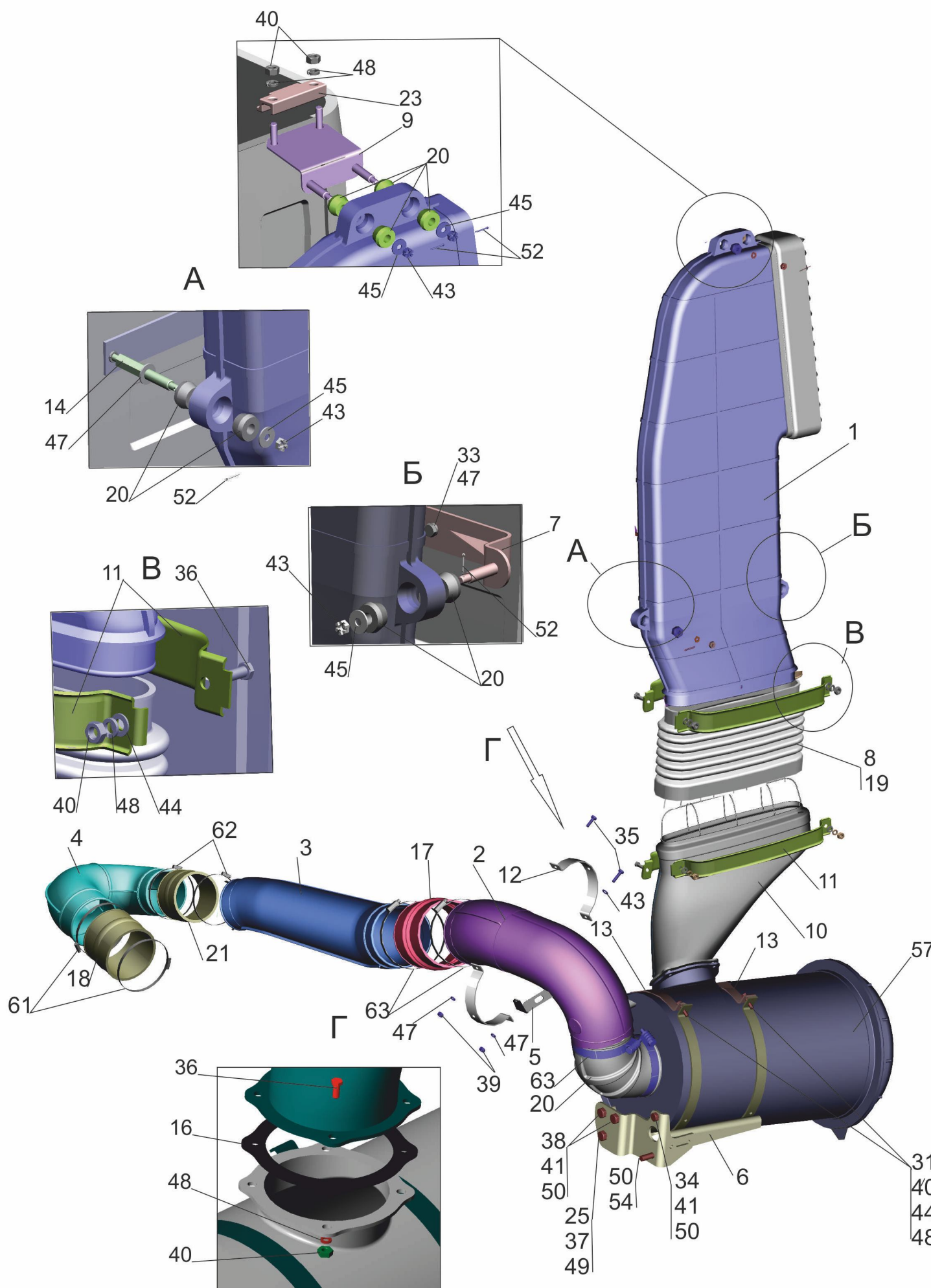
Рис. 26 Крепление воздушного фильтра 6501B9-1109002-05 Fig. 26 Air filter mounting 6501B9-1109002-050
