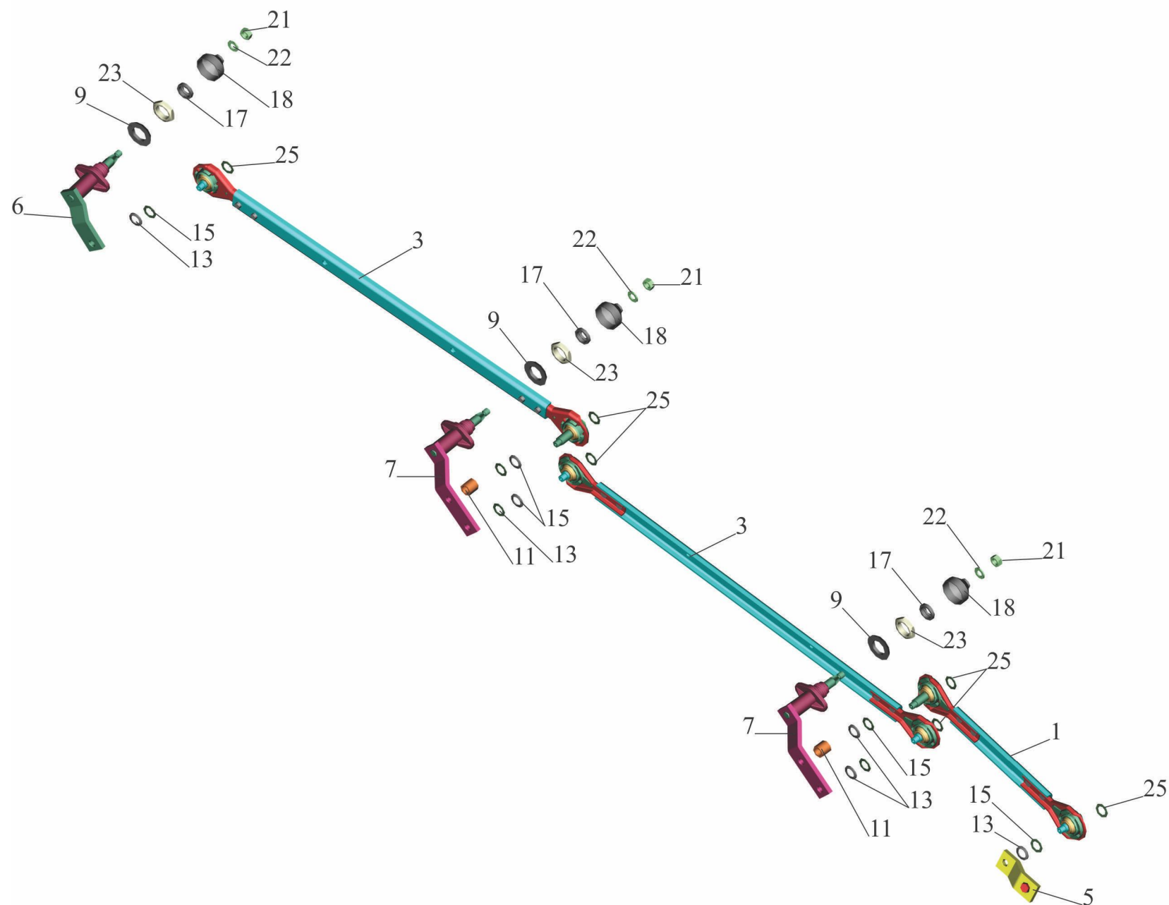
Рис. 218 Привод стеклоочистителя 6430-5205500-010 Fig. 218 Drive of cleaner of glasses 6430-5205500-010
