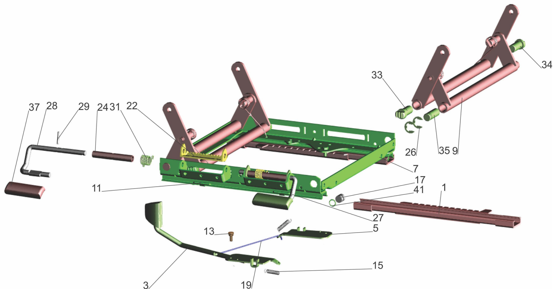
Рис.268 Механизм регулирования высоты 6430-6804100-010 Fig.268 Adjusting mechanisms of seat height 6430-6804100-010
