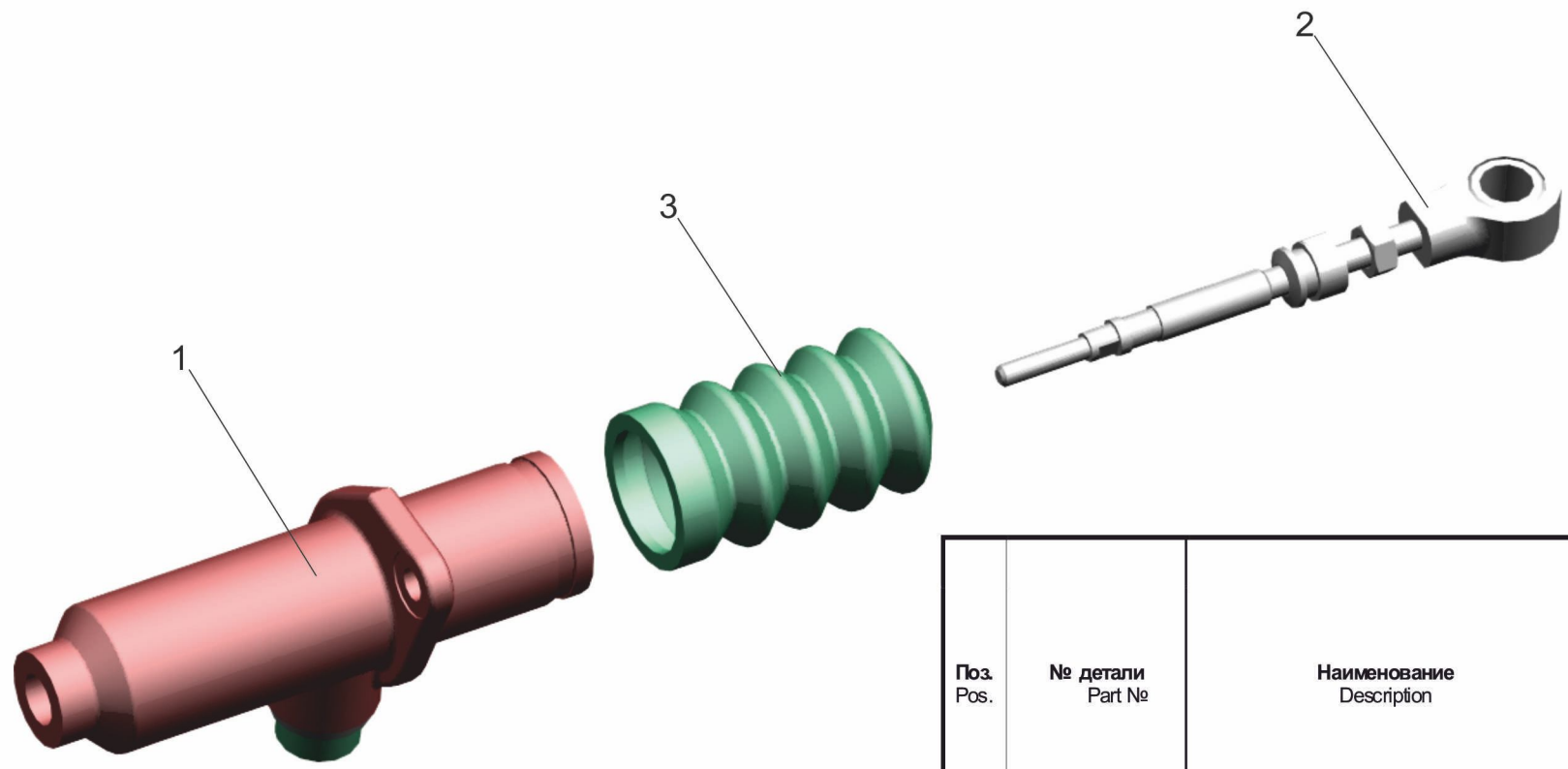
Рис. 42 Цилиндр подпедальный с толкателем 6430-1602500-000 (6430-1602500-001, 6430-1602500-020, 6430-1602500-002) Fig. 42 Under pedal cylinder with a pusher 6430-1602500-000 (6430-1602500-001, 6430-1602500-020, 6430-1602500-002)
