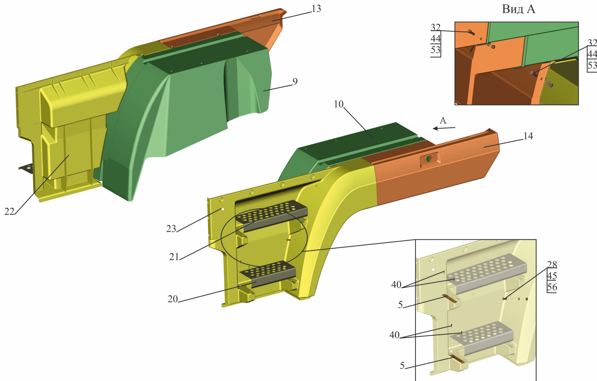
Fig. 257 Plumage
