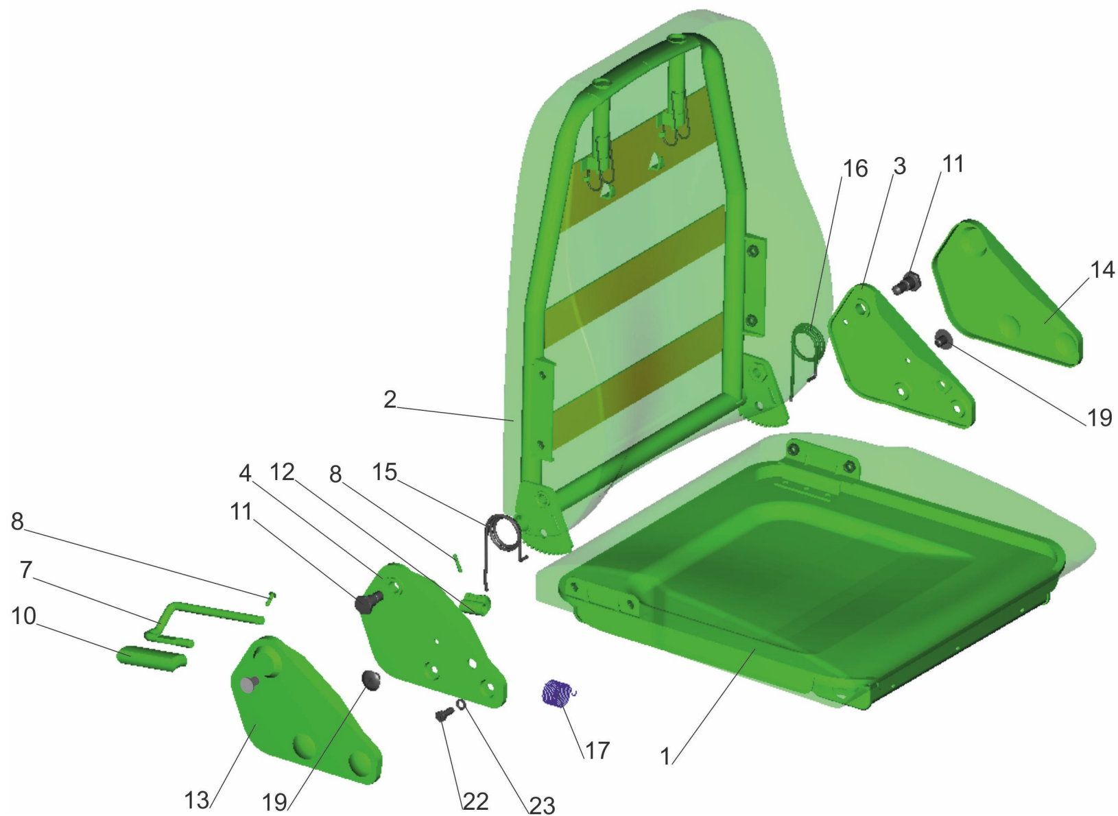
Рис.267Подушка и спинка сидения 6430-6810012 Fig.267 Pad and back seat 6430-6810012
