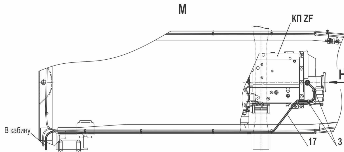
Рис. 210 Установка и пломбировка тахографа 5440-3800005 (лист 2 ) Fig. 210 Installation and identification seal of tachograph 5440-3800005 (page 2)
