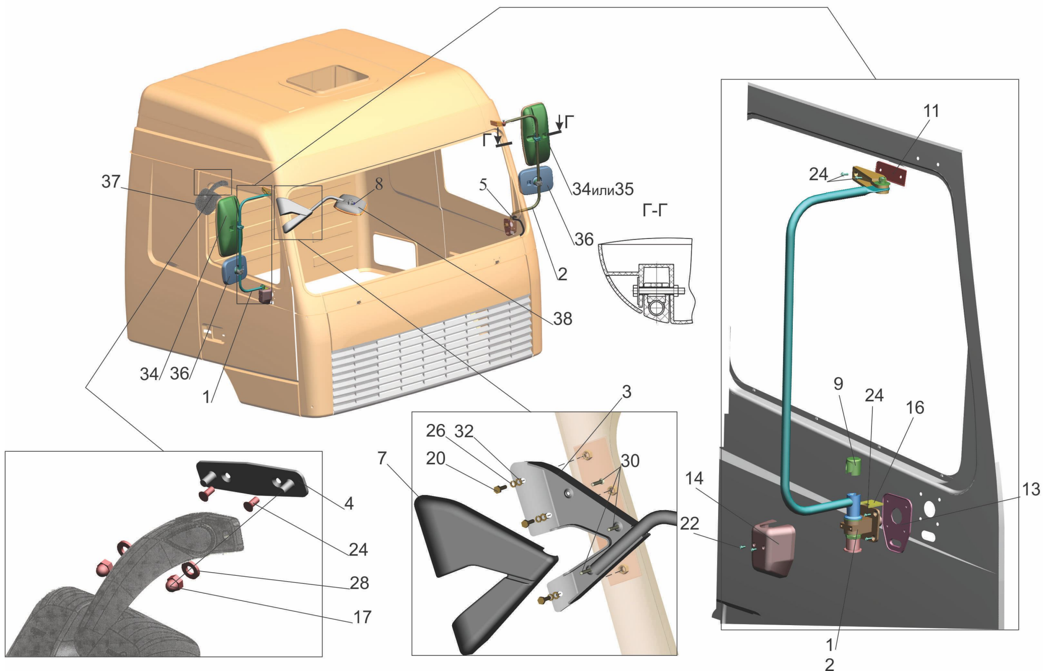
Рис. 260 Установка зеркал 6430-8200005-010,(-012,-020) Fig. 260 Installation mirrors 6430-8200005-010,(-012,-020)
