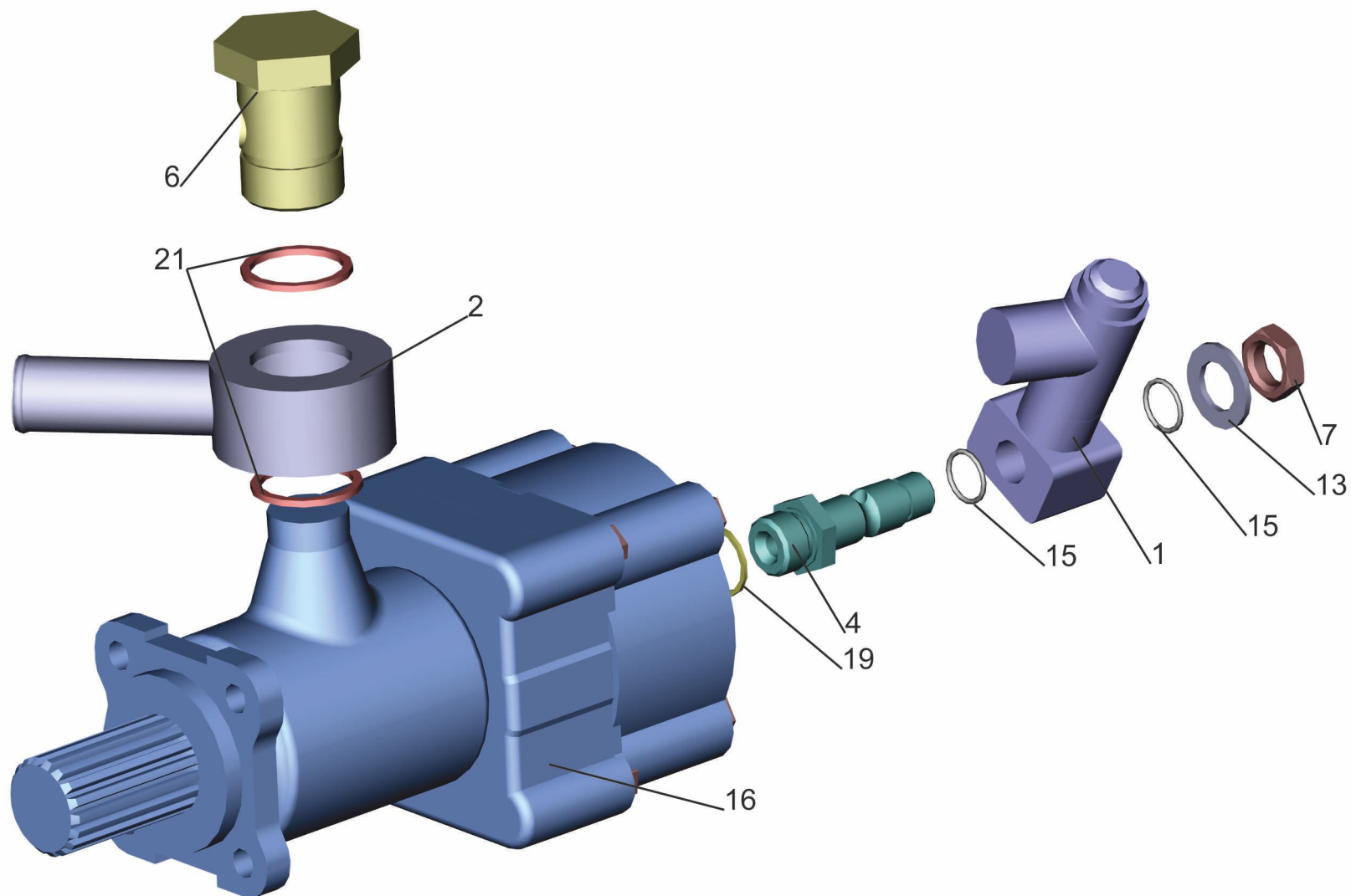
Рис. 338 Насос с арматурой 6501B9-8604010-069 Fig. 338 Pump with accessories 6501B9-8604010-069
