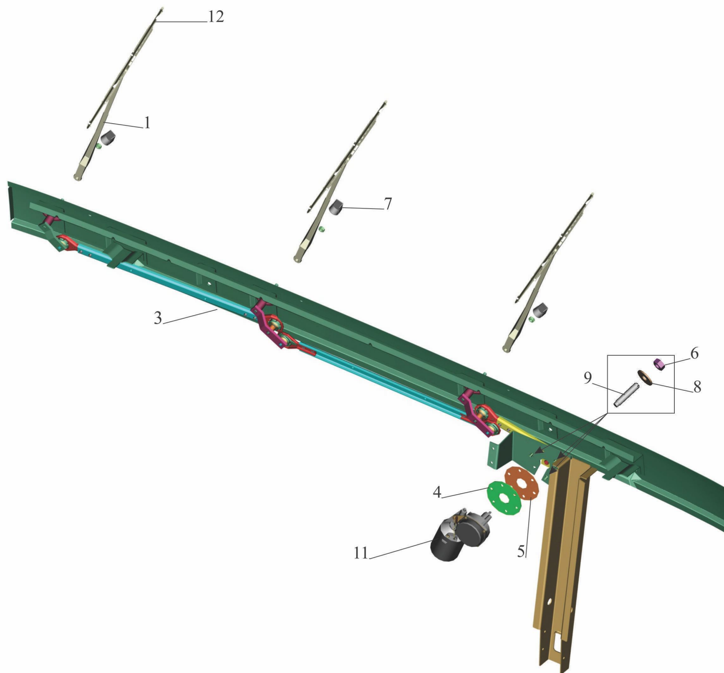
Рис.217 Установка стеклоочистителя 6430-3700041-001 Fig. 217 Installation of cleaner of glasses 6430-3700041-001
