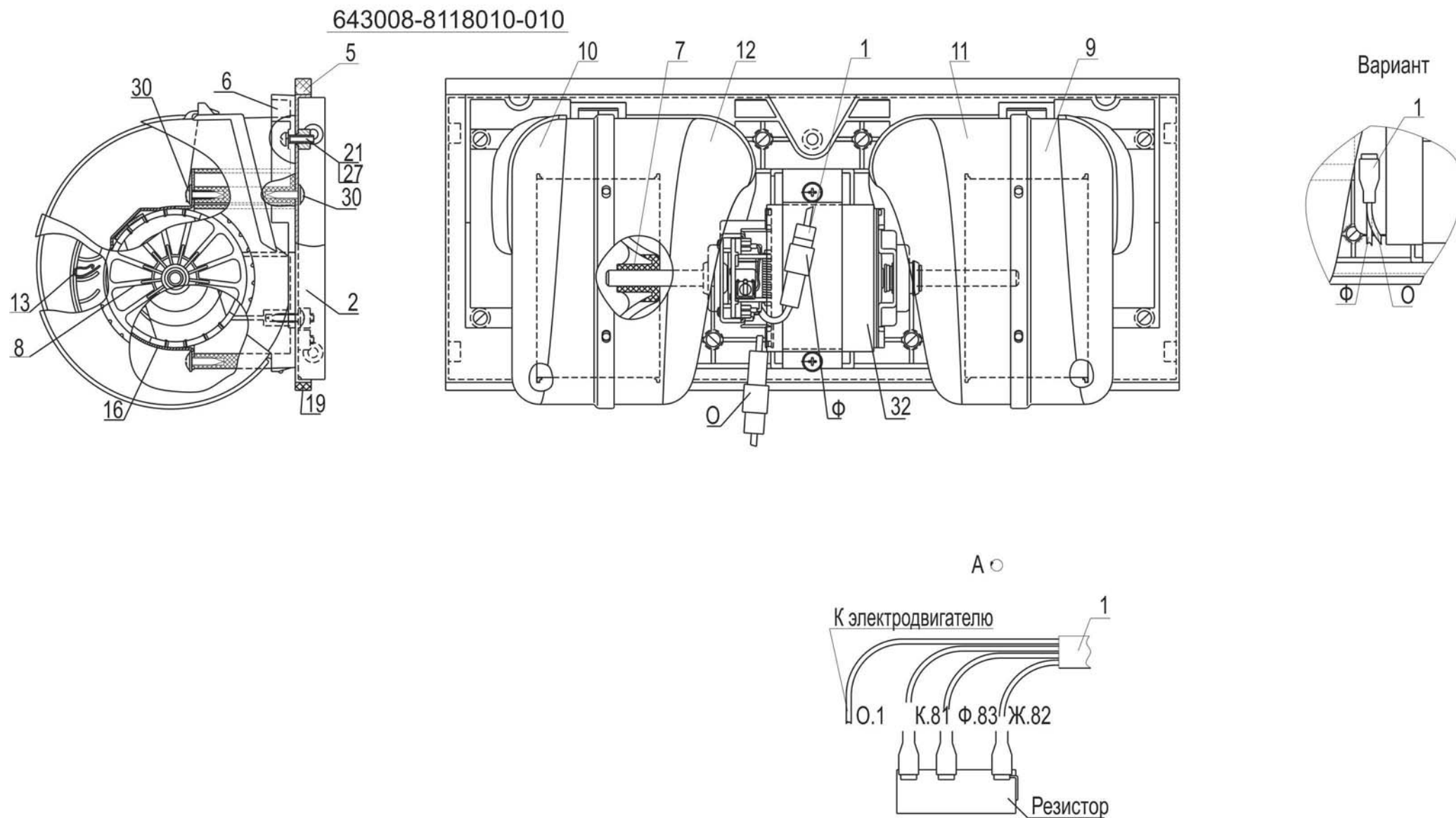
Рис. 290 Блок вентиляторный 643008-8118010-010, (-030) Fig. 290 Fan unit 643008-8118010-010, (-030)
