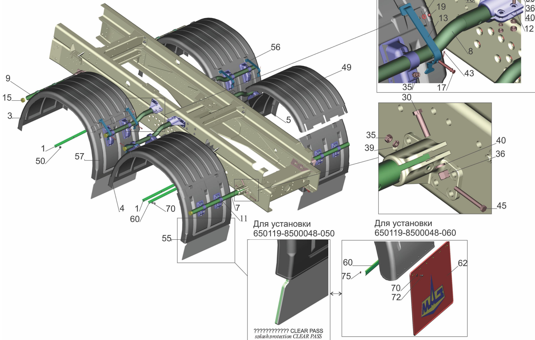
Рис. 327 650119-8500048-050/060 Fig. 327 The fenders installation
