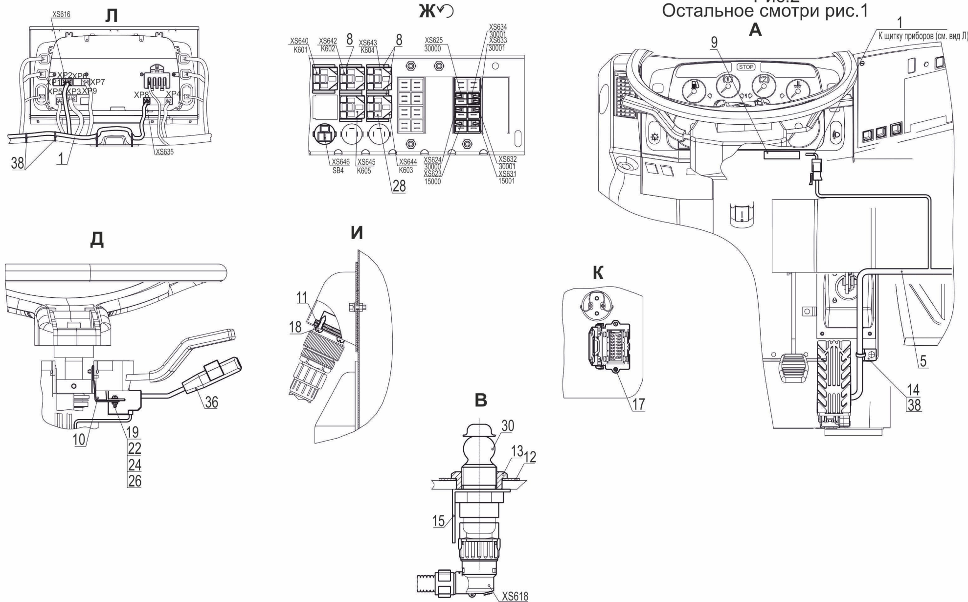
Рис. 222 Установка электрооборудования ЭСУ двигателя 6516В9-3800060-000 (лист 2) Fig. 222 Installation of electric equipment of electronic control sistem of the engine (page 2)
