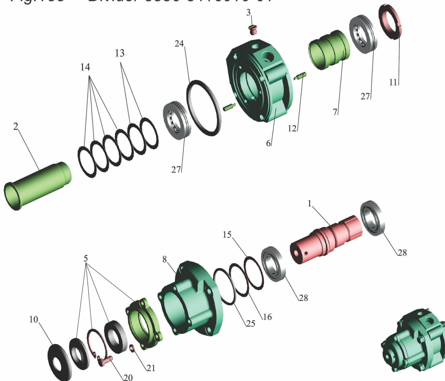
Рис.155 Распределитель 5336-3416010-01 Fig.155 Divider 5336-3416010-01
