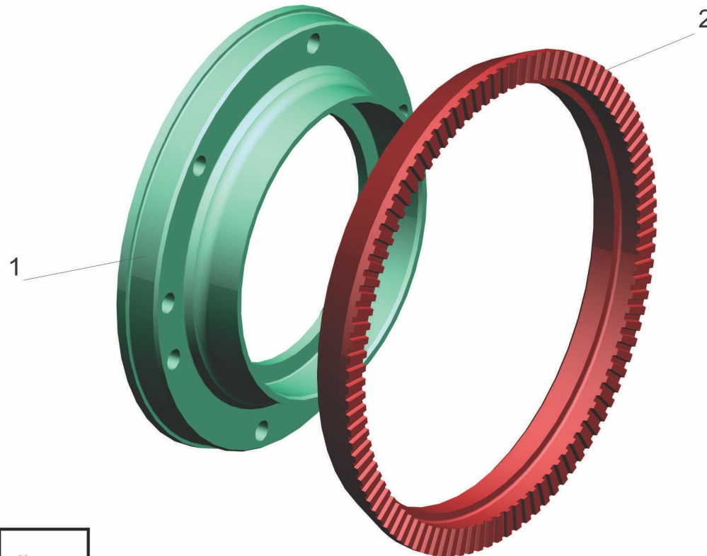
Рис. 68 Крышка 543266-3104035-000 Fig. 68 Cover 543266-3104035-000
