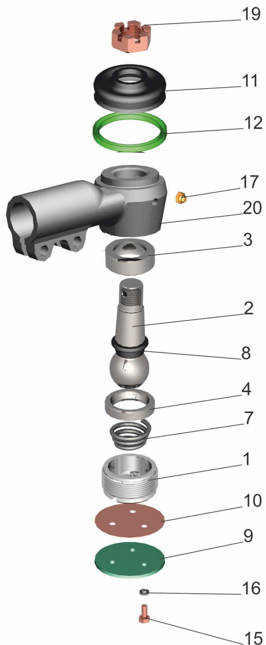
Рис.127 Наконечник 6422-3003056 Fig.127 Nozzle 6422-3003056
