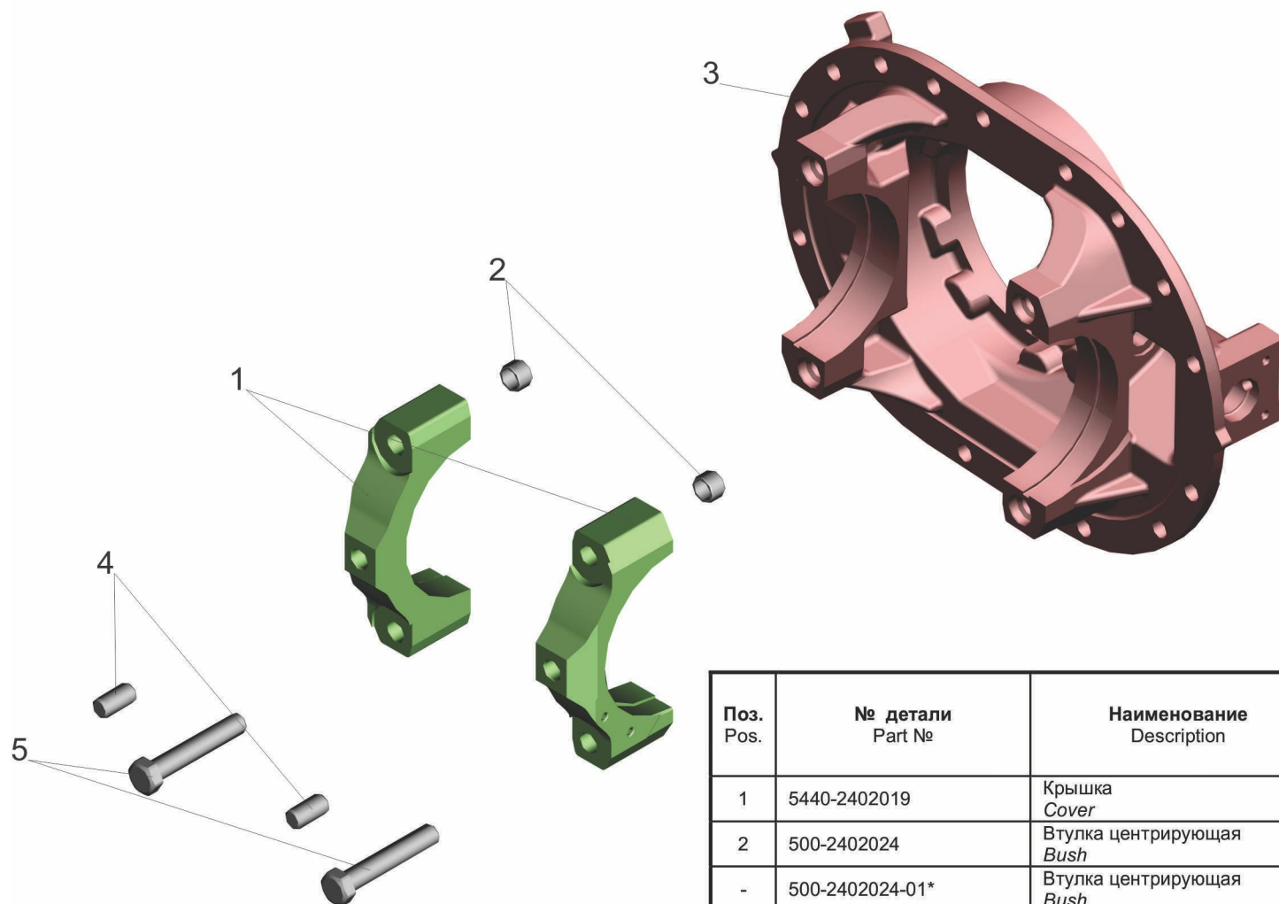
Рис. 72 Картер редуктора 5440-2402015-010 Fig. 72 Reducer gear housing 5440-2402015-010
