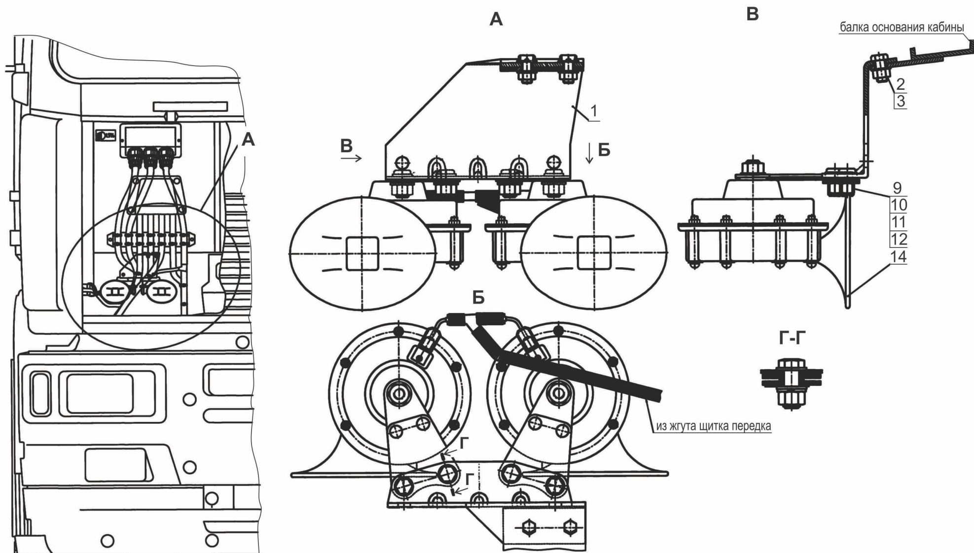
Рис. 194 Установка звуковых сигналов 544008-3700024, (-700) Fig. 194 Installation of audible signals 544008-3700024, (-700)
