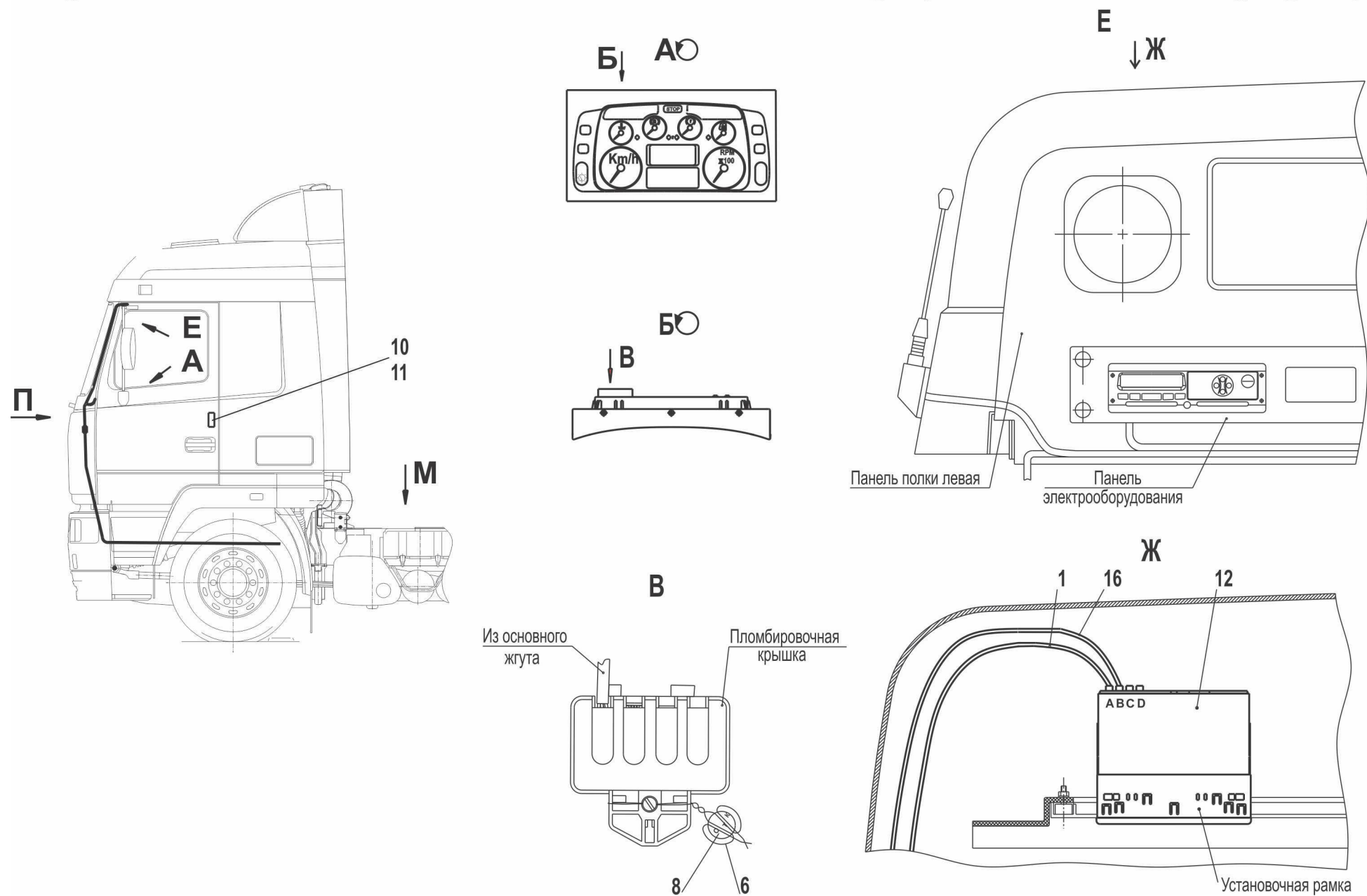
Рис. 210 Установка и пломбировка тахографа 5440-3800005 (лист 1) Fig.210 Installation and identification seal of tachograph 5440-3800005 (page 1)
