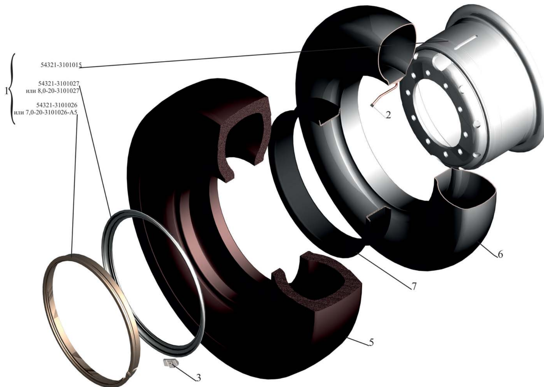
Рис. 144 Колесо и шина Fig. 144 Wheel and tyre
