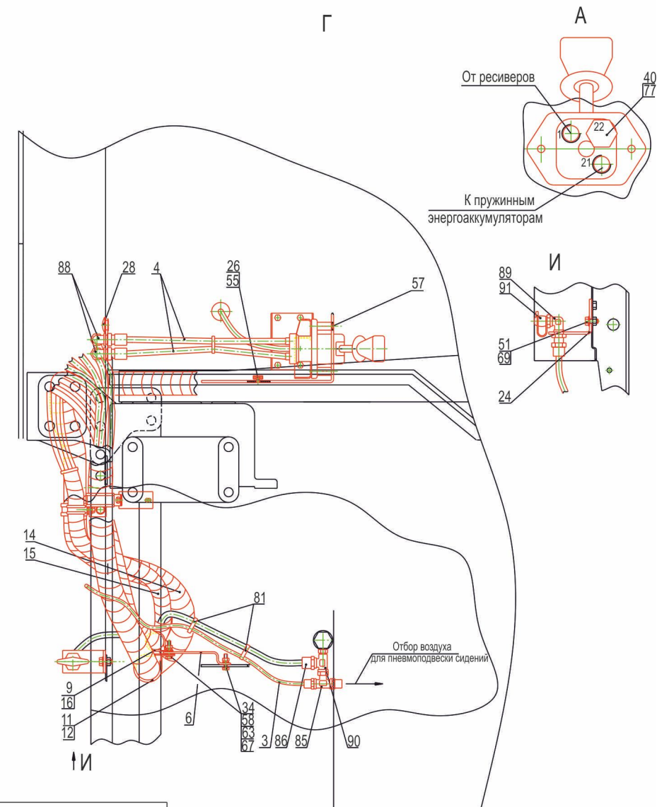
Рис. 180 Привод стояночного и моторного тормозов (лист 1) Fig. 180 Drive parking and motor brake.(page 1)
