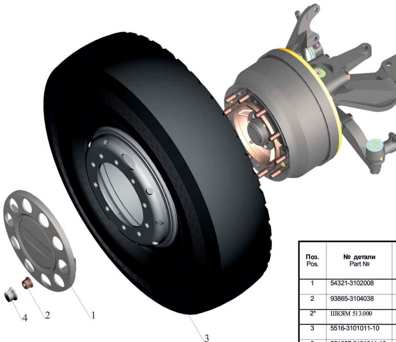
Рис. 142 Установка передних колес Fig. 142 Installation of forward wheels
