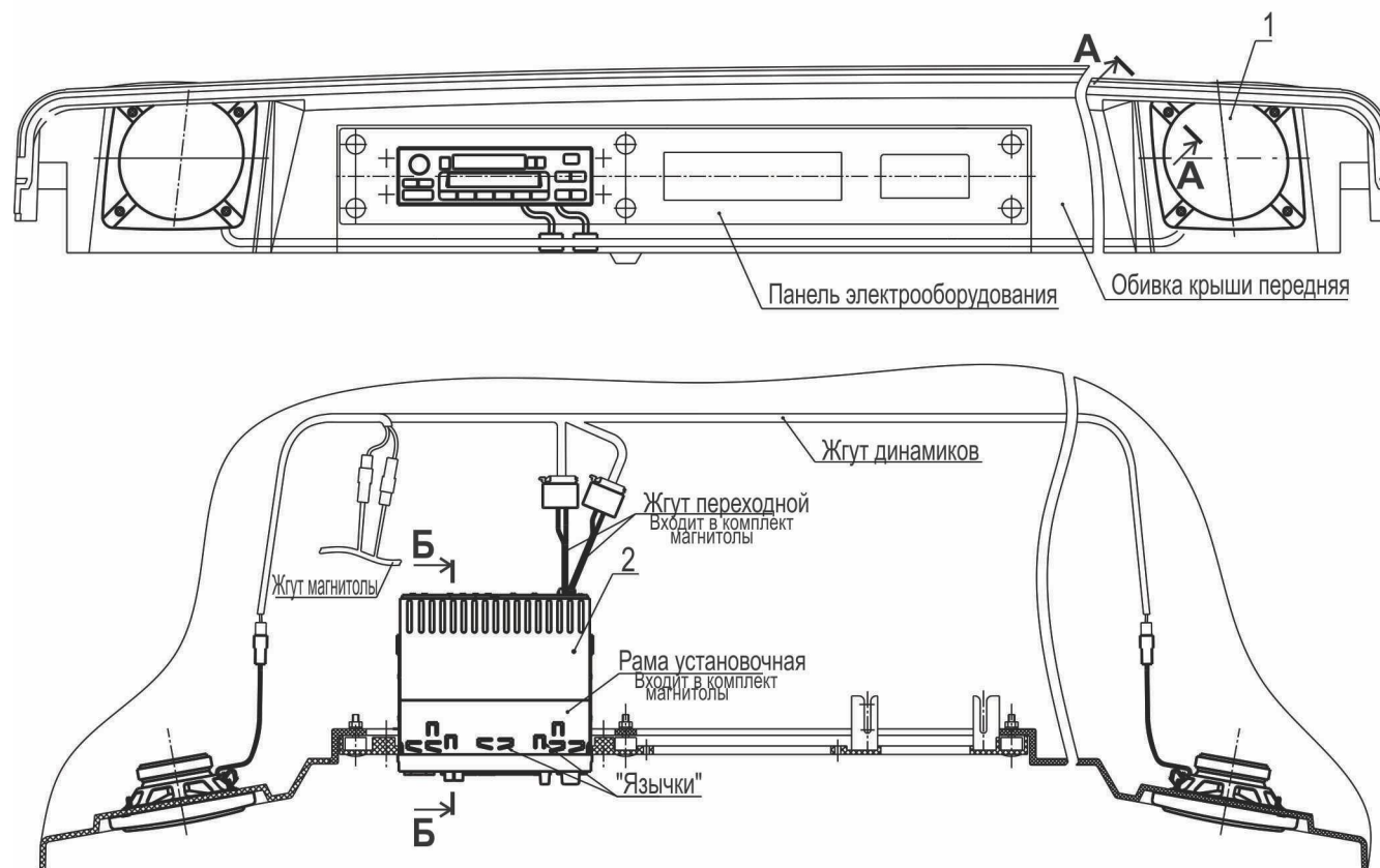
Рис.211 Установка магнитолы 6501-7900010 Fig.211 Installation of player 6501-7900010
