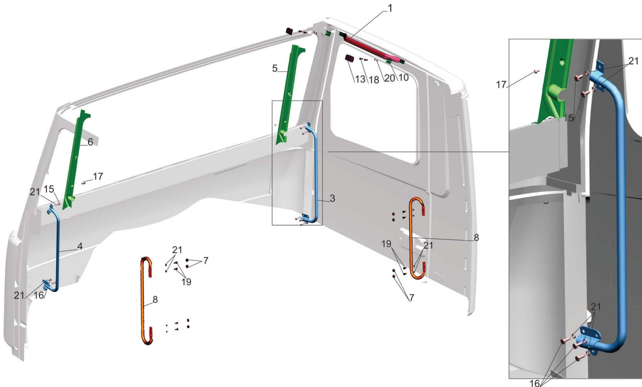
Рис. 250 Установка поручней в кабине 6430-8200030. Fig. 250 Installation of grab handles in cab 6430-8200030.
