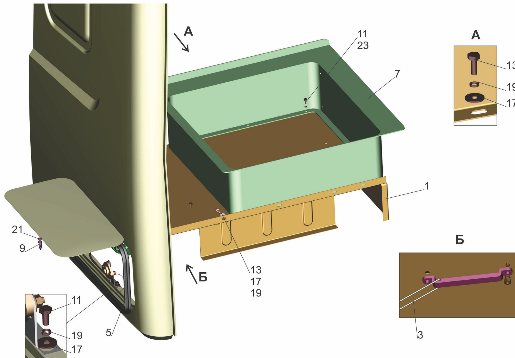
Рис. 240 Установка инструментального ящика 6430-5000115-020 Fig. 240 Installation of a tool box 6430-5000115-020
