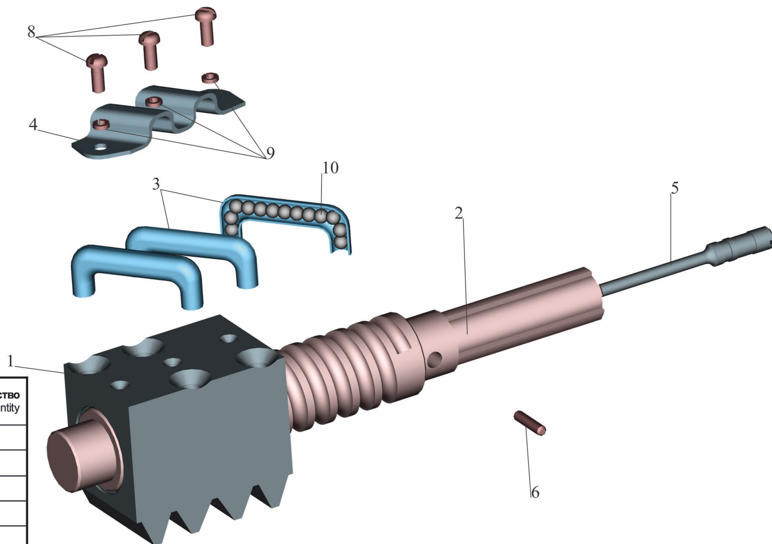
Fig. 152 Screw 64229-3401030
