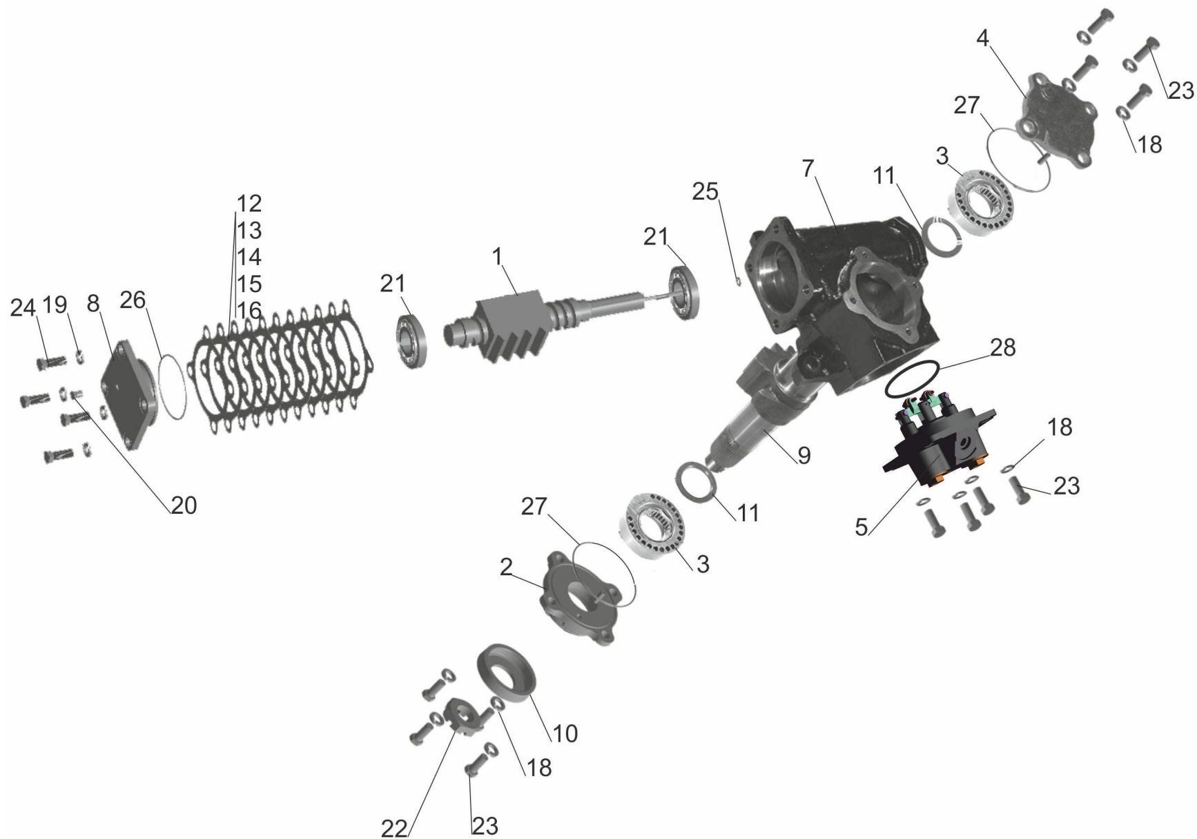
Рис. 150 Механизм рулевой 64221-3401005-10 Fig. 150 Steering mechanism 64221-3401005-10
