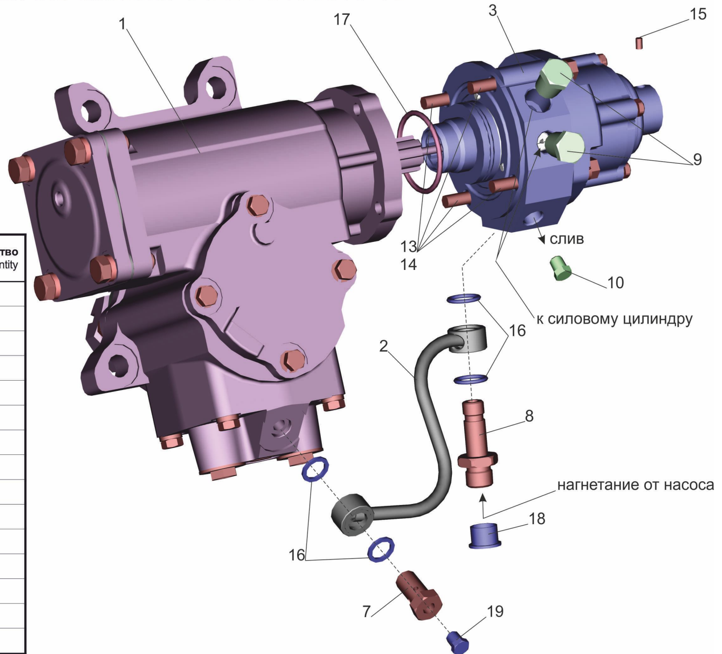
Рис.149 Рулевой механизм с распределителем 64221-3400010-10 Fig. 149 Steer with the allocator 64221-3400010-10
