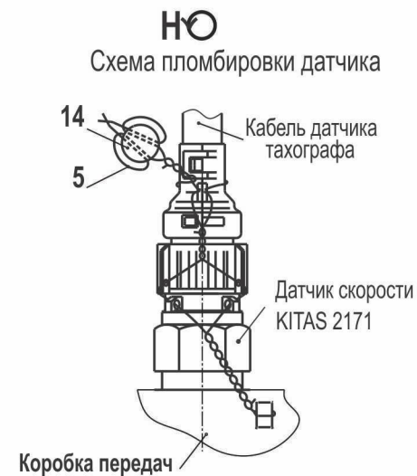
Рис. 210 Установка и пломбировка тахографа 5440-3800005 (лист 2 ) Fig. 210 Installation and identification seal of tachograph 5440-3800005 (page 2)
