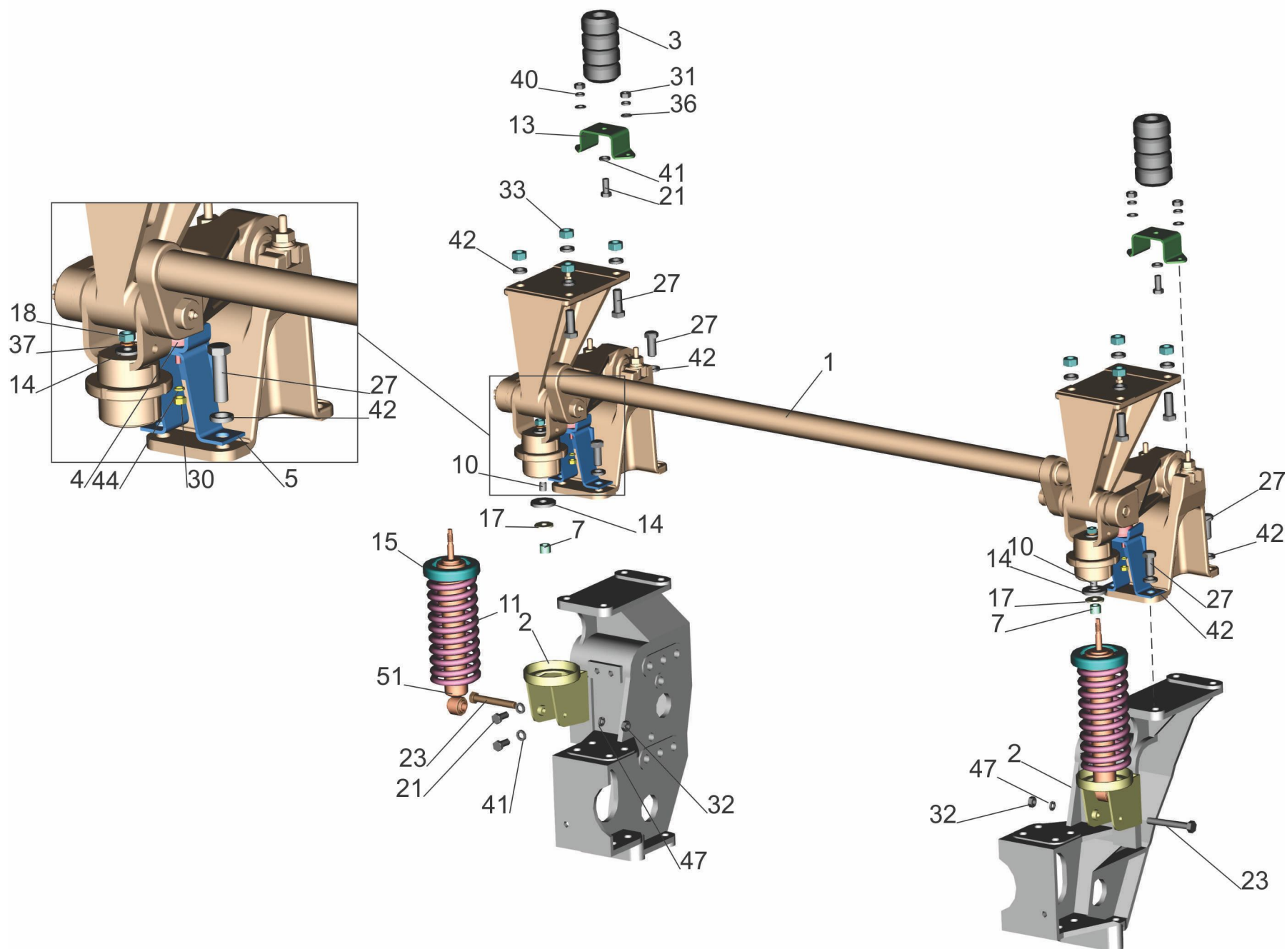
Рис. 229 Переднее подрессоривание 6430-5001700-10 Fig. 229 Front sprigging 6430-5001700-10
