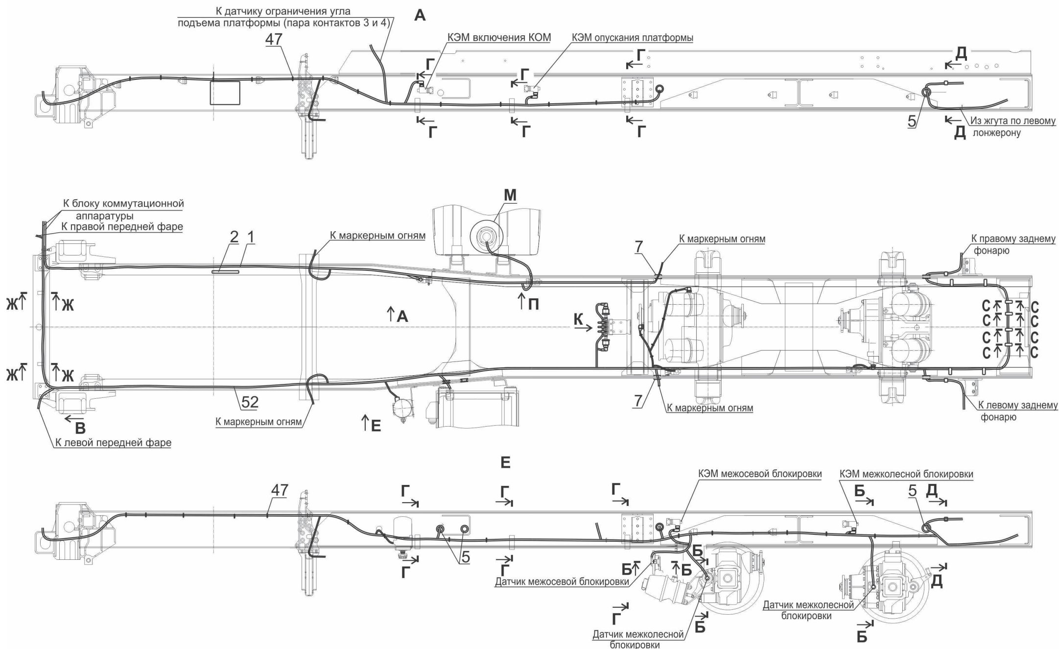
Рис.186 Установка электрооборудования на шасси 6501В9-3700010-040, (-740) (лист 1) Fig.186 Installation of electrical equipment on the chassis 6501В9-3700010-040, (-740) (page 1)
