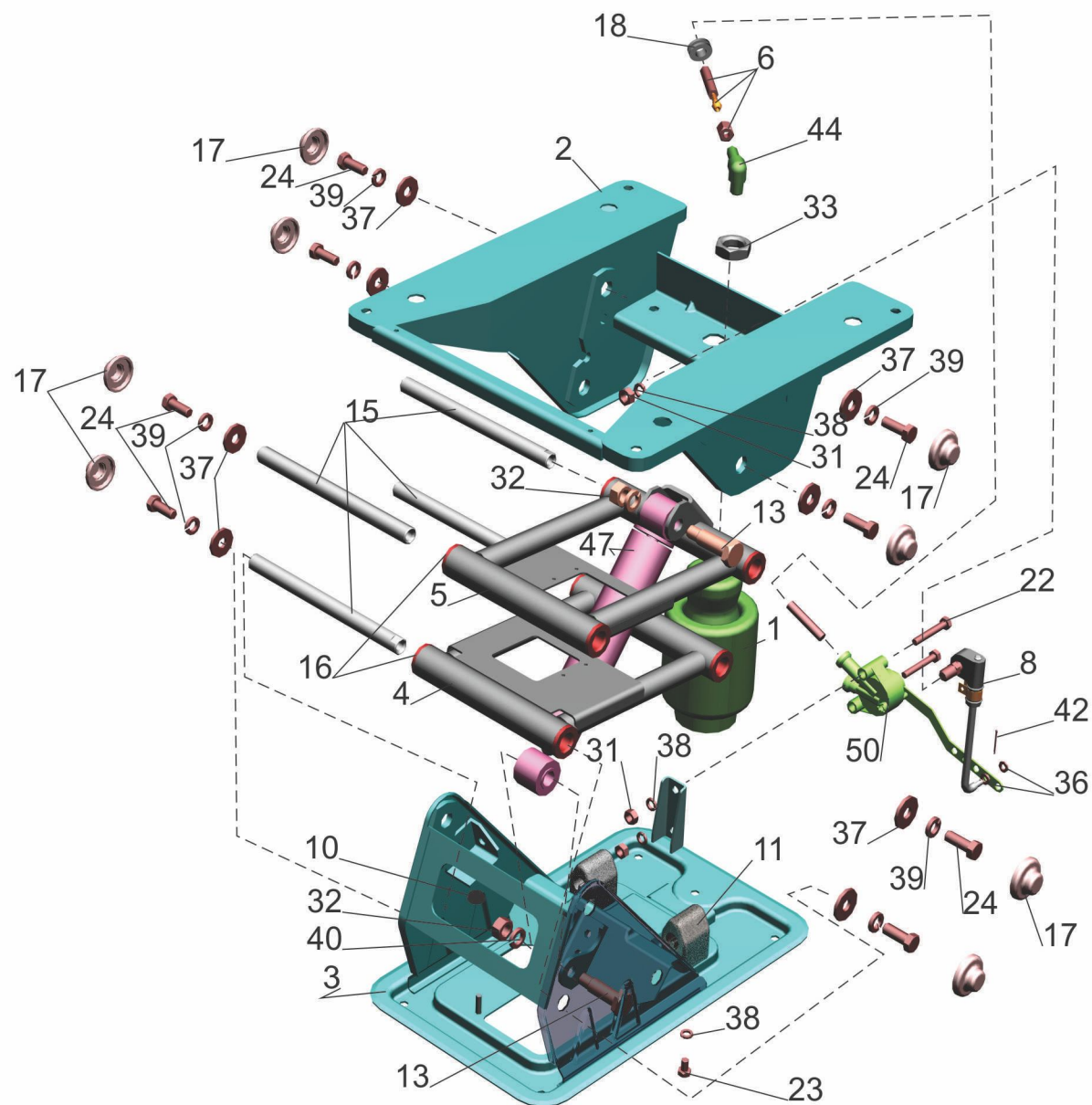
Рис. 273 Подставка сиденья с пневмооборудованием 6430-6807006-010 Fig. 273 Seat support with pneumatic equipment 6430-6807006-010
