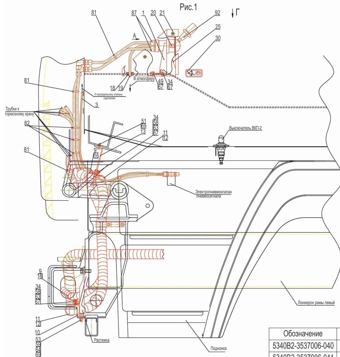
Рис. 180 Привод стояночного и моторного тормозов (лист 1) Fig. 180 Drive parking and motor brake.(page 1)
