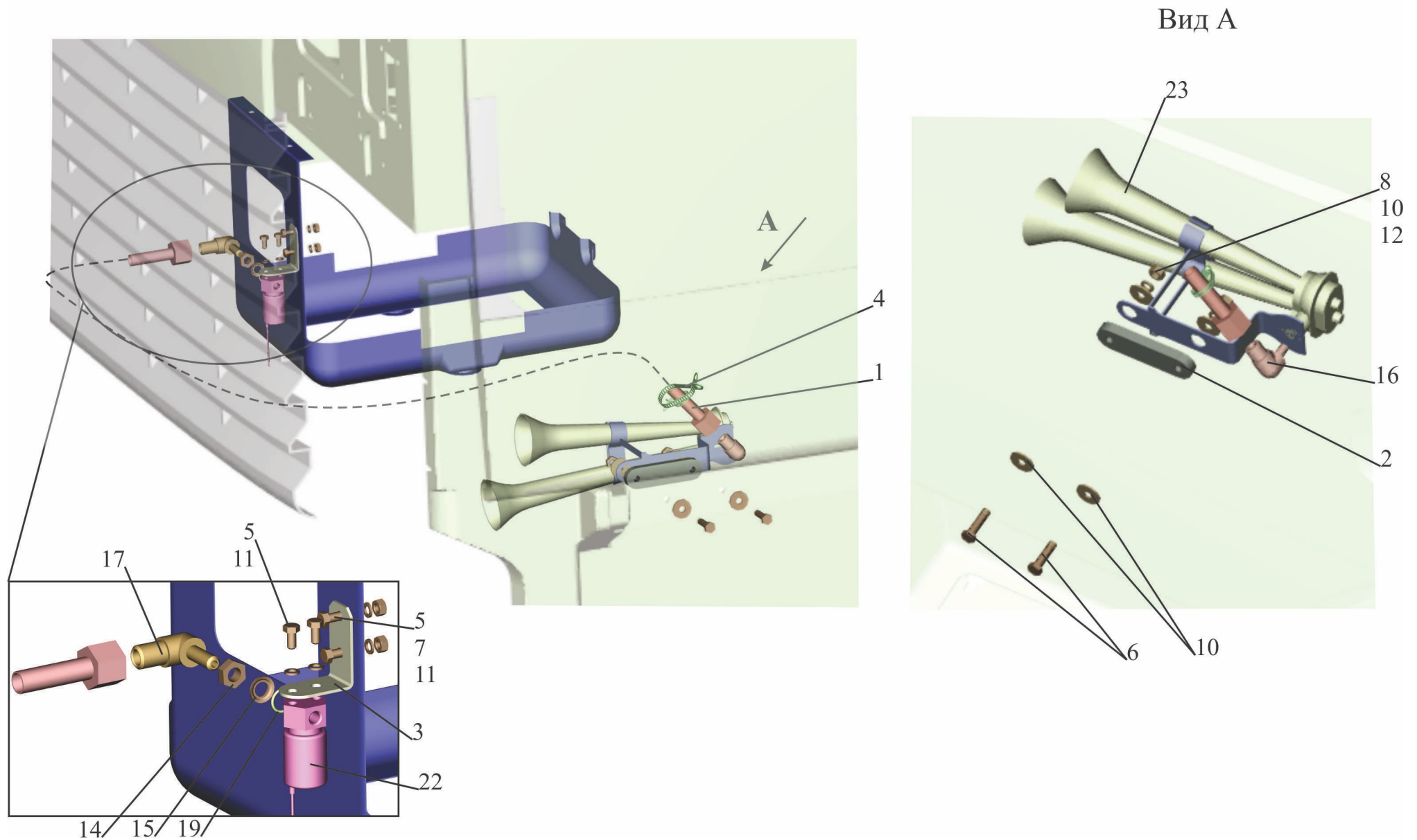
Рис. 198 Установка пневмосигнала 6430-3700096, 6430-3700096-700 Fig. 198 Mounting of air horn 6430-3700096, 6430-3700096-700
