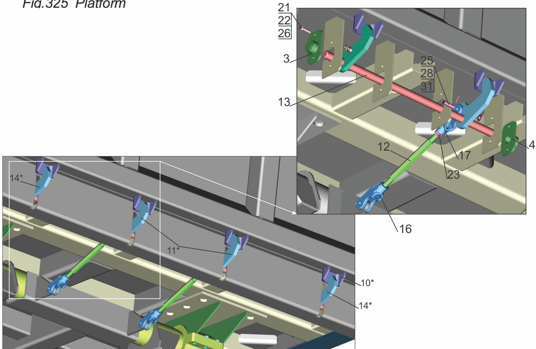
Рис.325 Платформа 6501В9-8500020-000 (лист 2)
