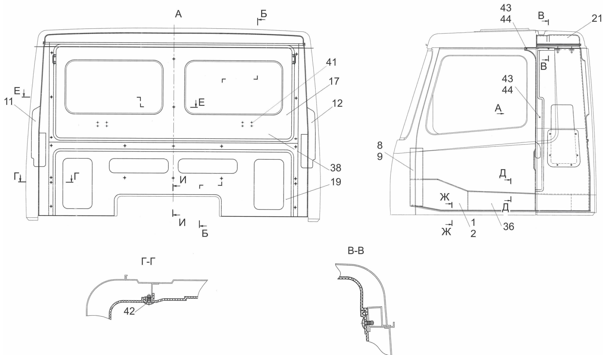
Рис.238 Установка обивок и коврик 6501-5000100 Лист 1 Fig.238 Installation of upholsteries and carpets 6501-5000100 Page 1
