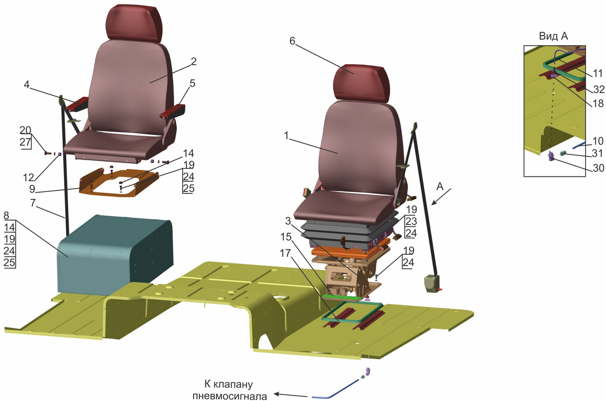
Рис. 263 Установка и пневмопитание сидений 5340V4-6800006-000 Fig. 263 Installation and pneumatic supply of seat 5340V4-6800006-000
