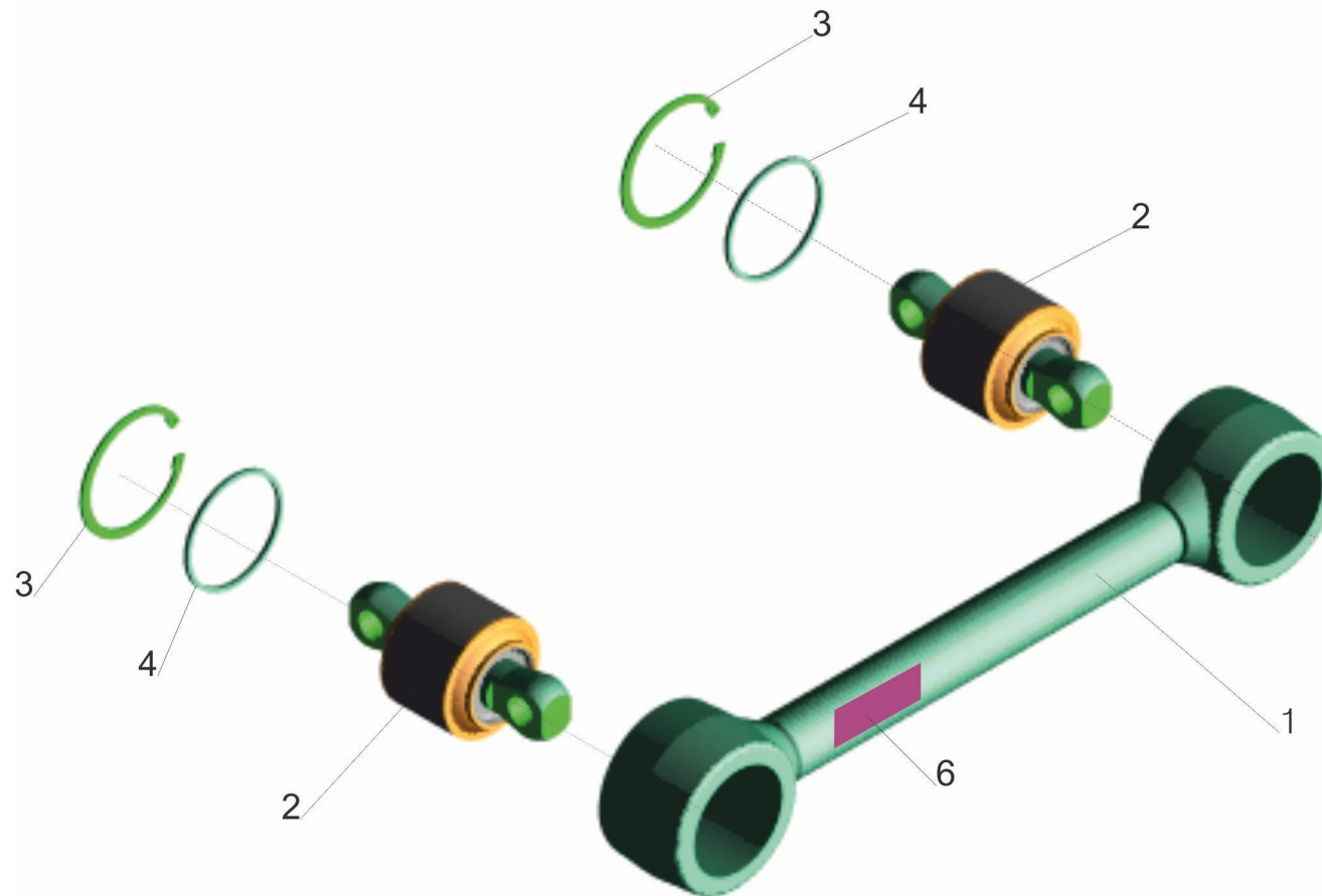
Fia.120 Torque rod 6430-2919014
