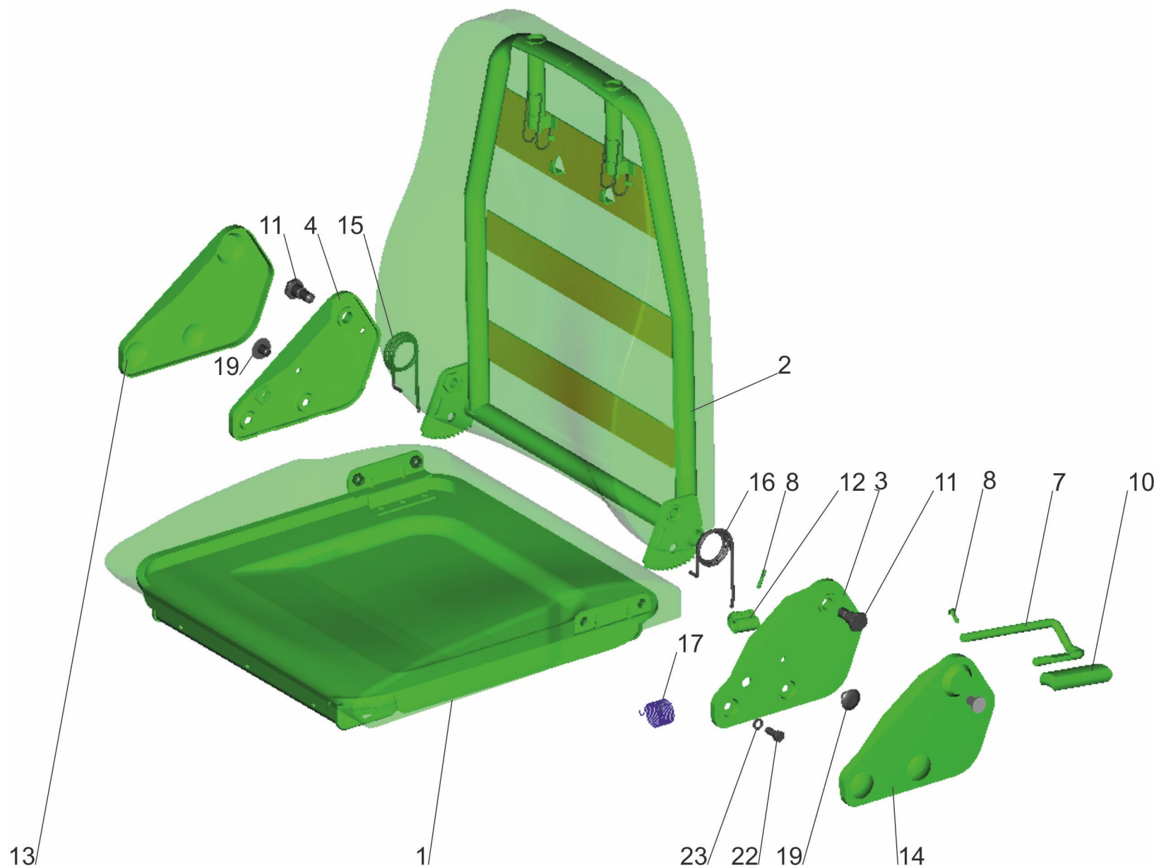
Рис.266 Подушка и спинка сидения 6430-6800012 Fig. 266 Pad and back seat 6430-6800012
