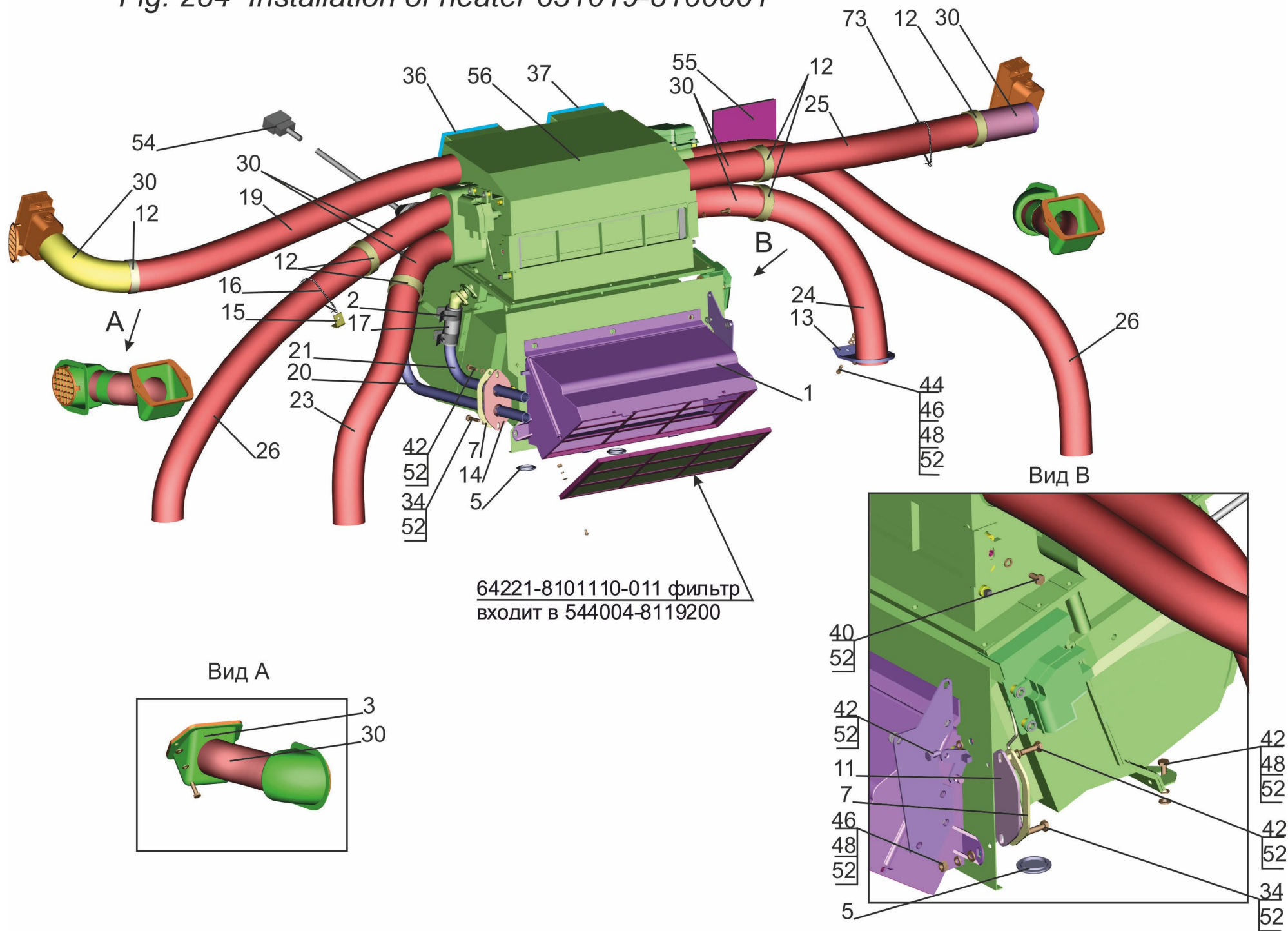
Fig. 284 Installation of heater 631019-8100001
