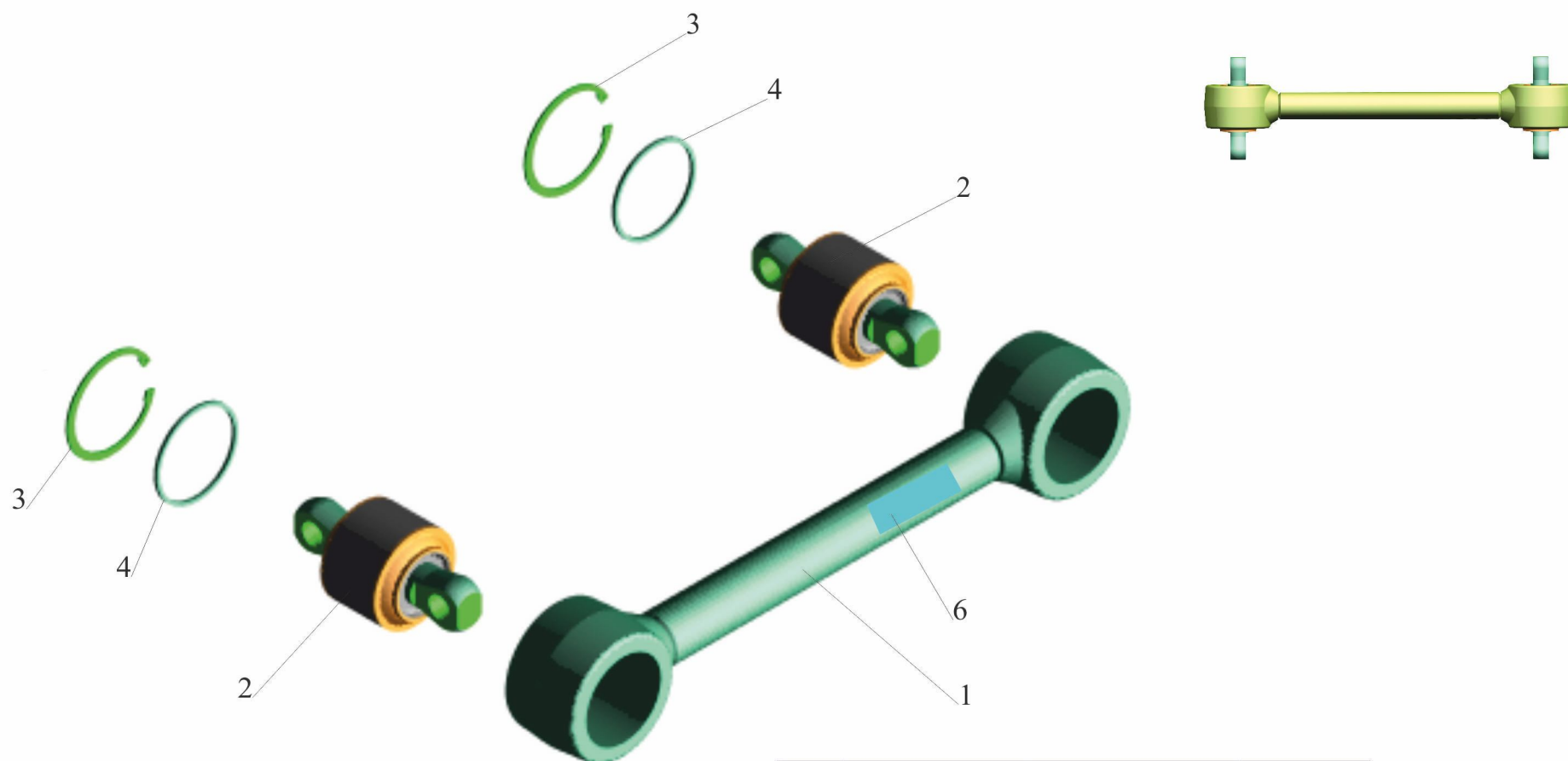
Fig.121 Torque rod 64221-2919015
