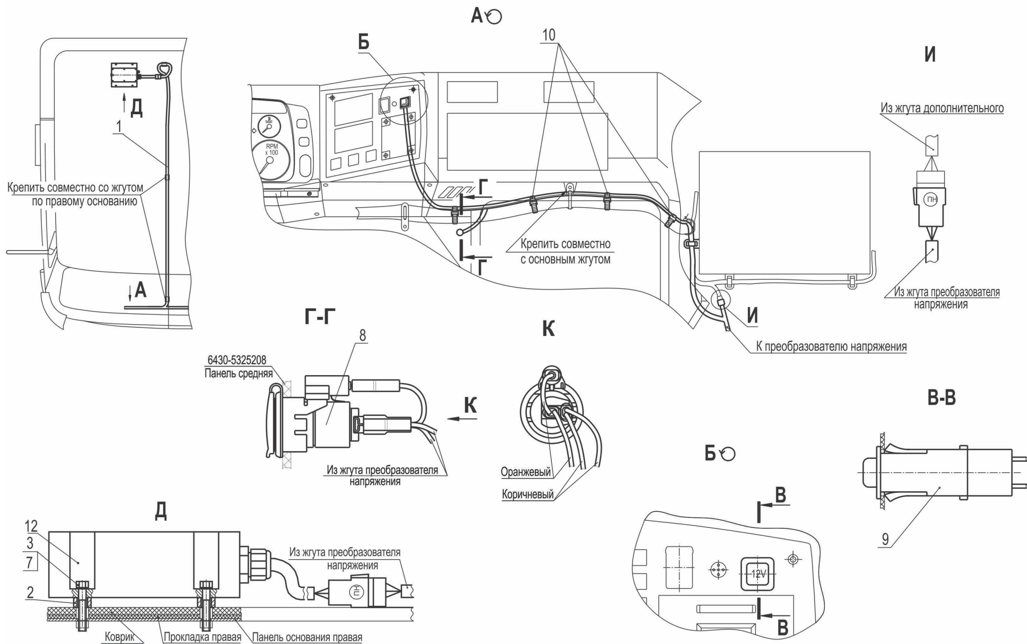
Рис. 201 Установка преобразователя напряжения 6501A8-3700109-000 Fig.201 Installation of a voltage changer 6501A8-3700109-000
