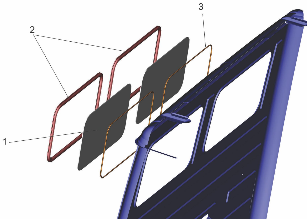
Рис. 246 Установки стекла задка 6501-5600015 Fig. 246 Installation a back glass 6501-5600015
