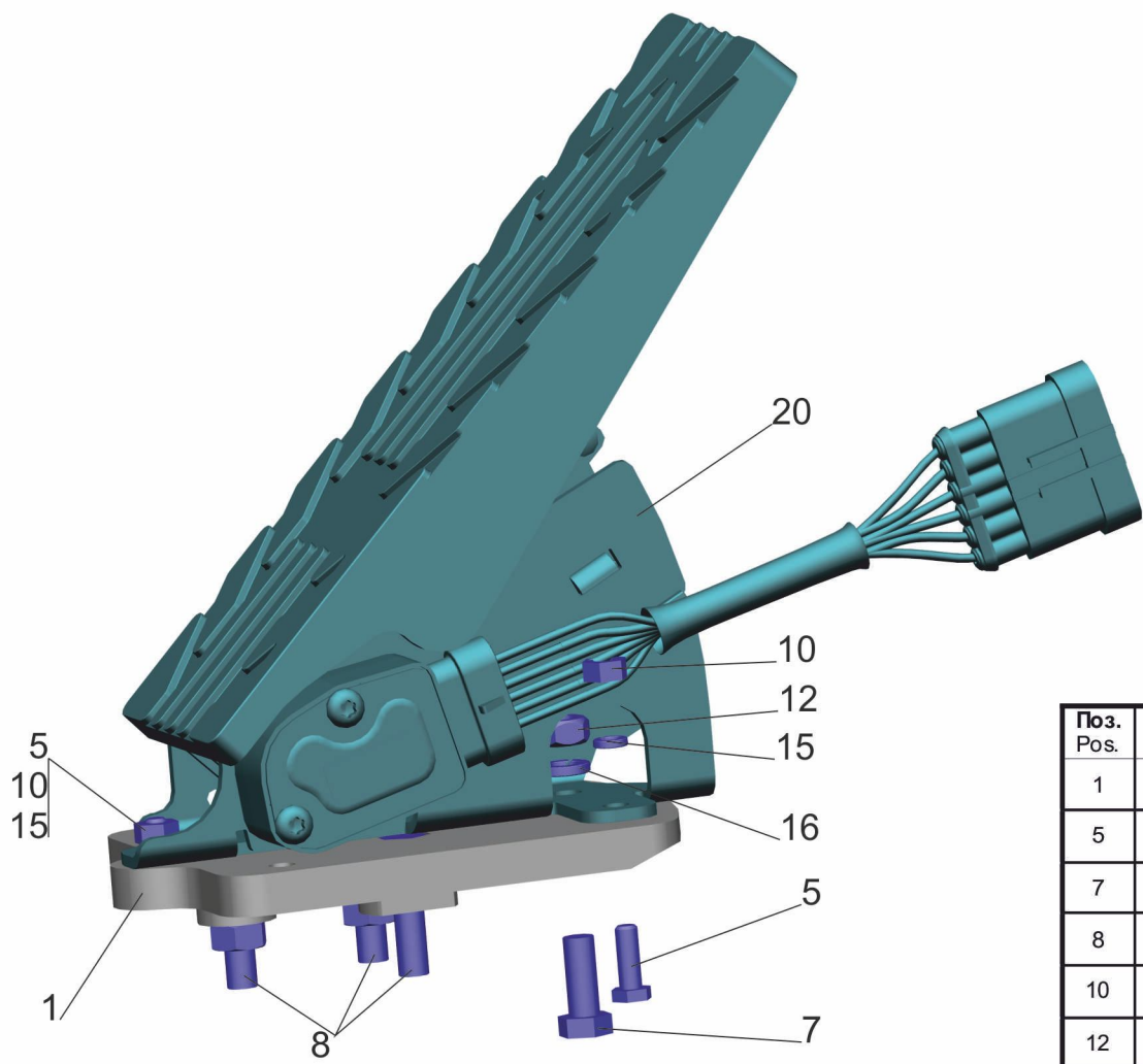
Рис. 30 Педаль с переходником 437143-1108005 Fig. 30 Pedal with an adapter 437143-1108005
