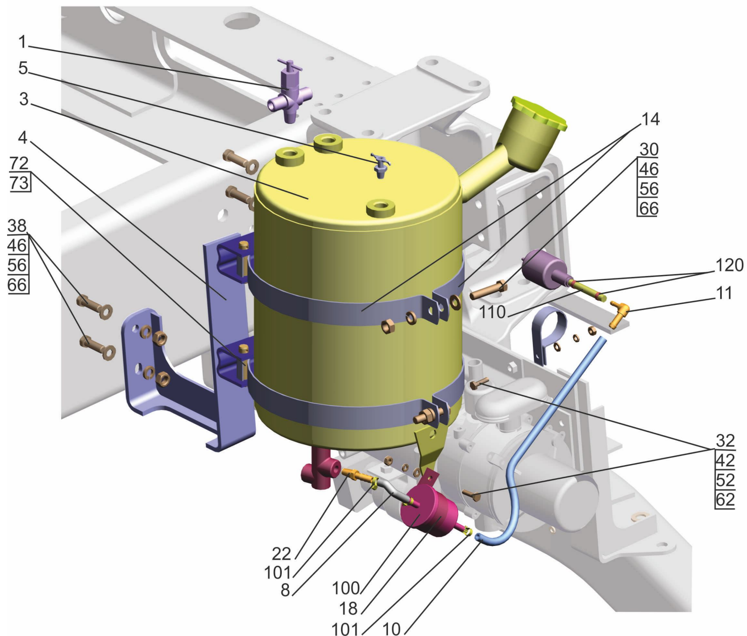
Рис.11 Крепление топливопроводов подогревателя 6501B5-1015004-010 Fig.11 Mounting fuel lines of heater 6501B5-1015004-010
