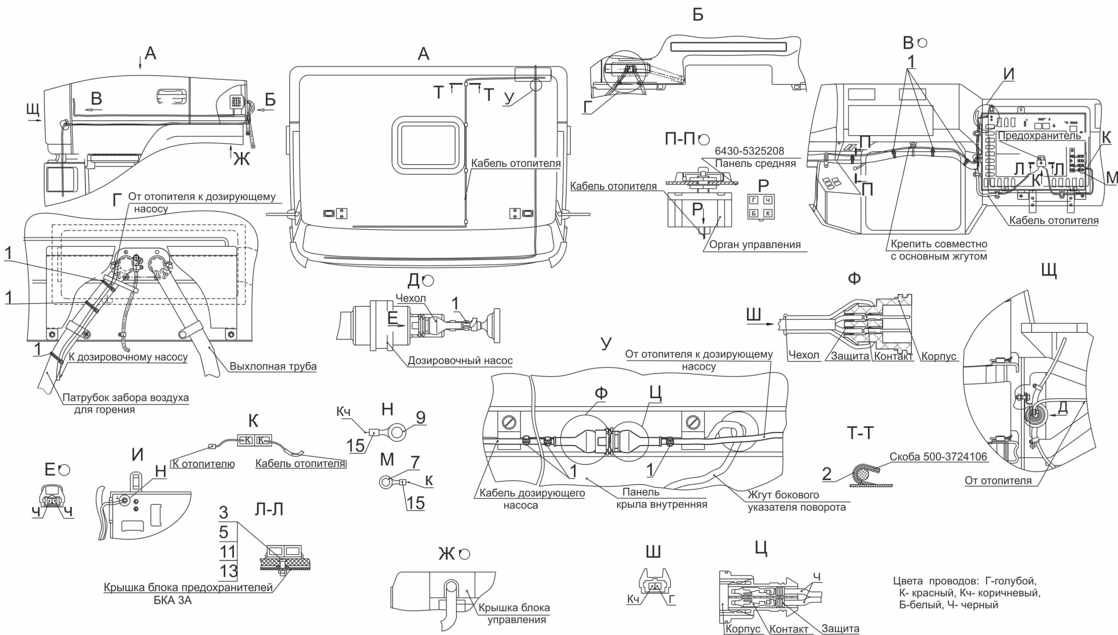
Рис. 301 Установка электрооборудования независимого воздушного отопителя 6501-3700088-010 Fig. 301 Installation of an electrical equipment independent air Heater 6501-3700088-010
