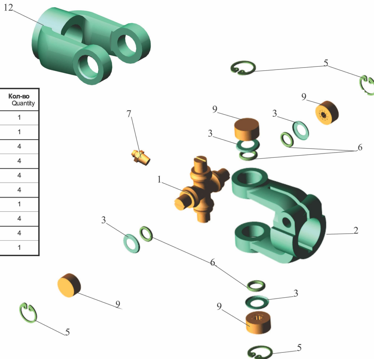
Рис. 166 Шарнир карданный 6430-3444054-001 Fig. 166 Hinge cardan 6430-3444054-001
