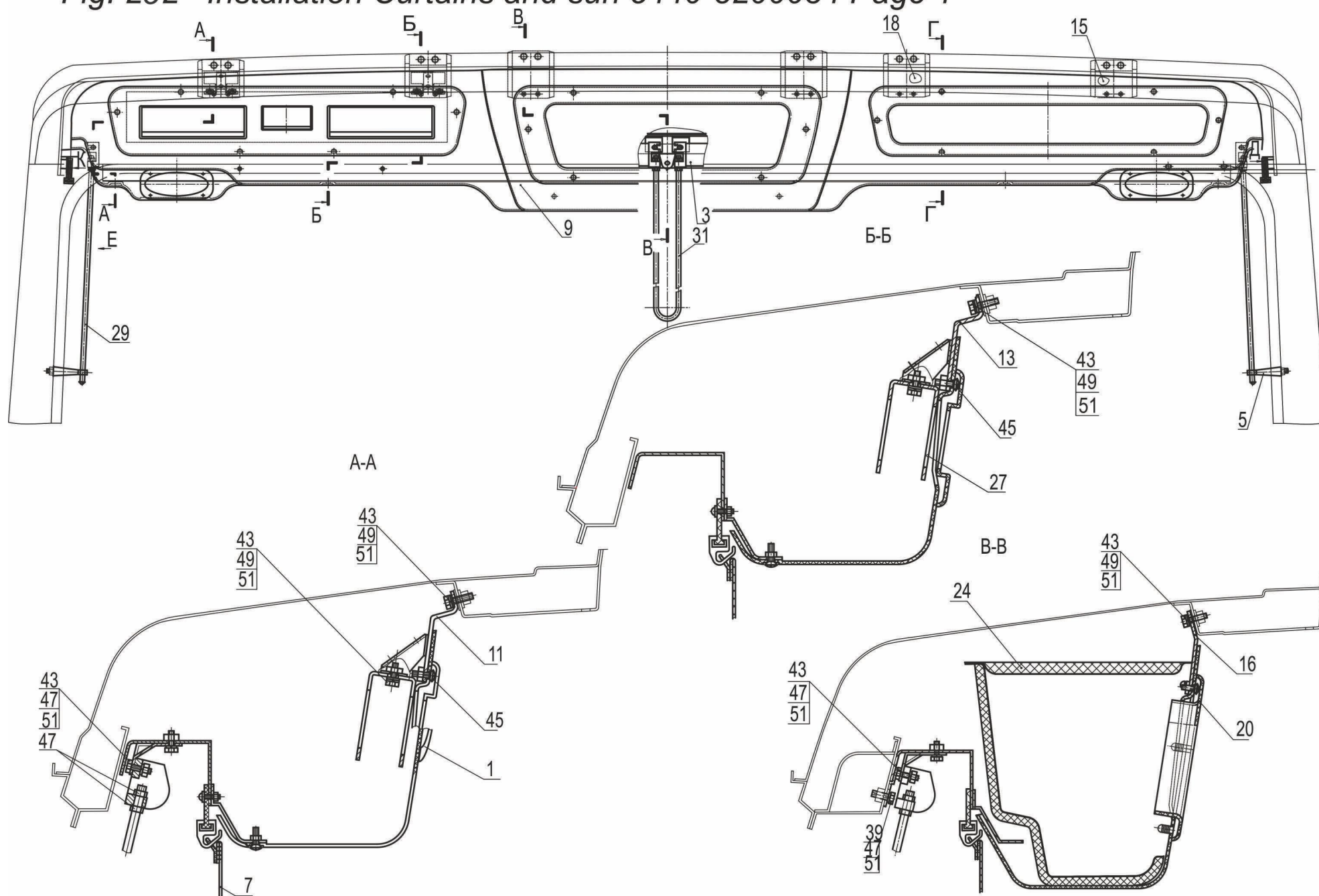
Рис. 252 Установка полки, штор 5440-8200034 Лист 1 Fig. 252 Installation Curtains and sun 5440-8200034 Page 1
