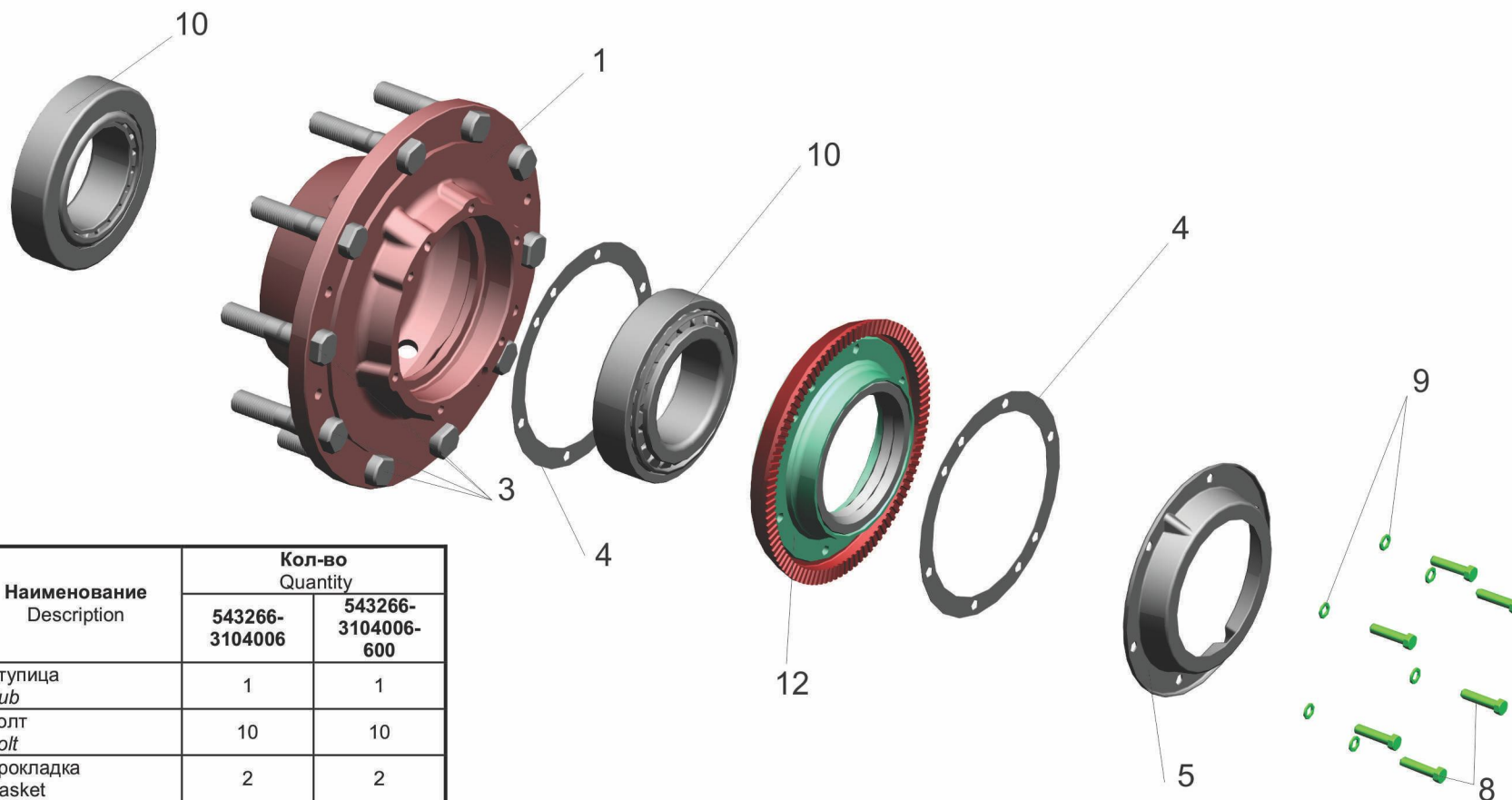
Рис.65 Ступица с крышкой Fig. 65 Rear axle hub
