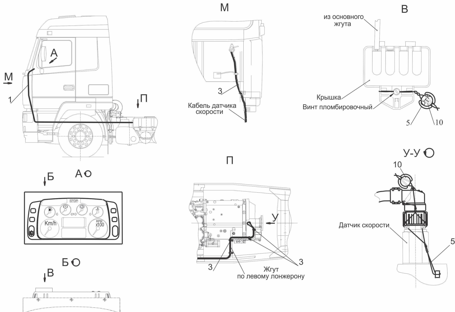
Рис.209 Установка и пломбировка спидометра 6516V8-3800004-030 Fig.209 Installation and identification seal of a speedometer 6516V8-3800004-030
