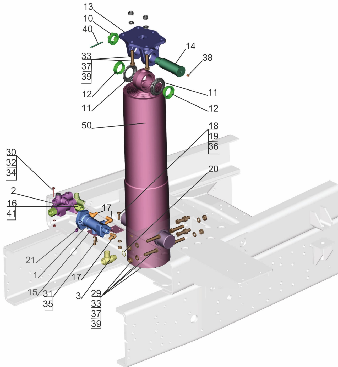
Рис. 333 Установка цилиндра и клапанов 6514H9-8603500-000 Fig. 333 Installation cylinder and valves 6514H9-8603500-000
