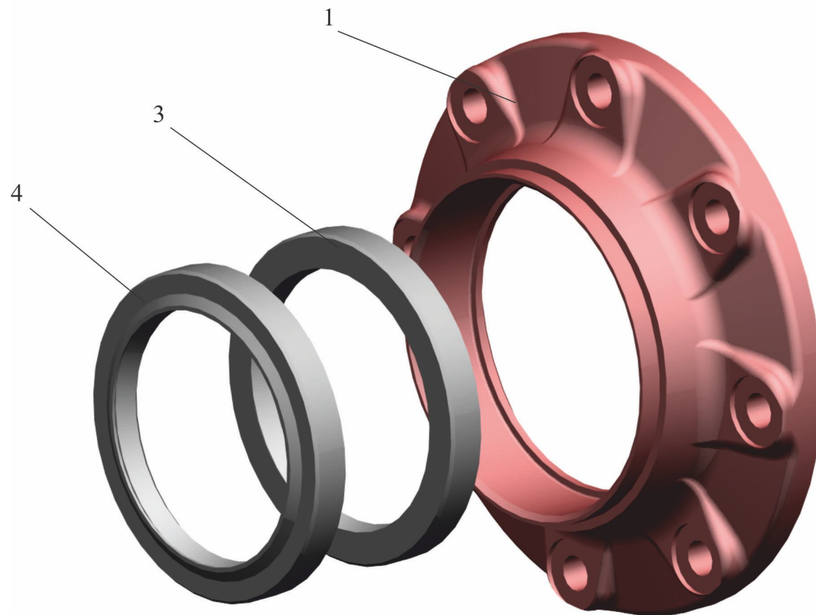
Рис. 91 Крышка 6430-2502140 Fig. 91 Cover 6430-2502140
