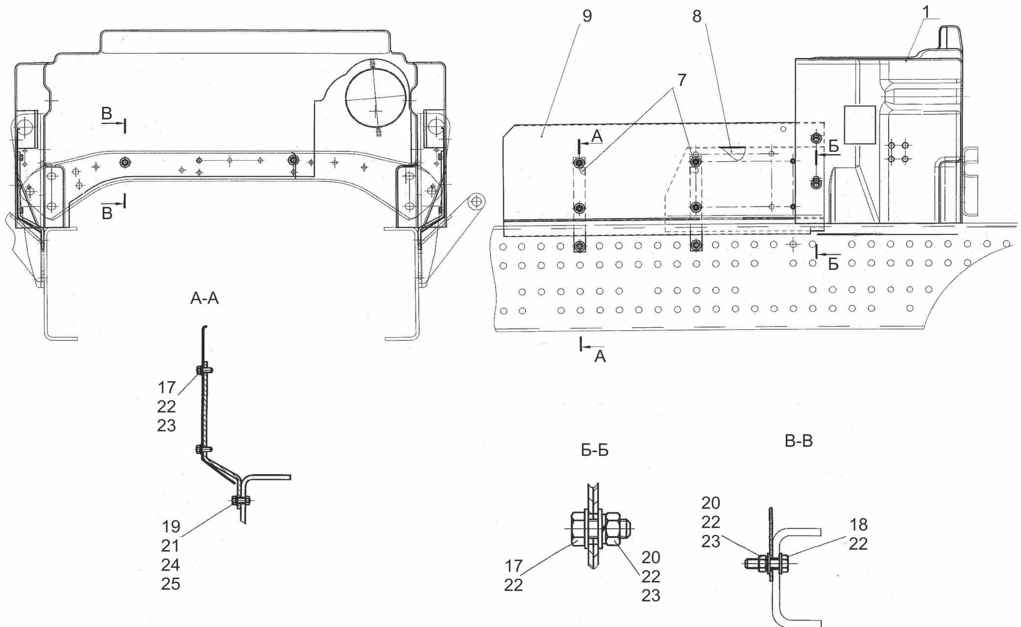
Рис. 16 Установка шумоизоляционных экранов 5340B9-1061003-001 Fig. 16 Mounting noise isolation screens 5340B9-1061003-001
