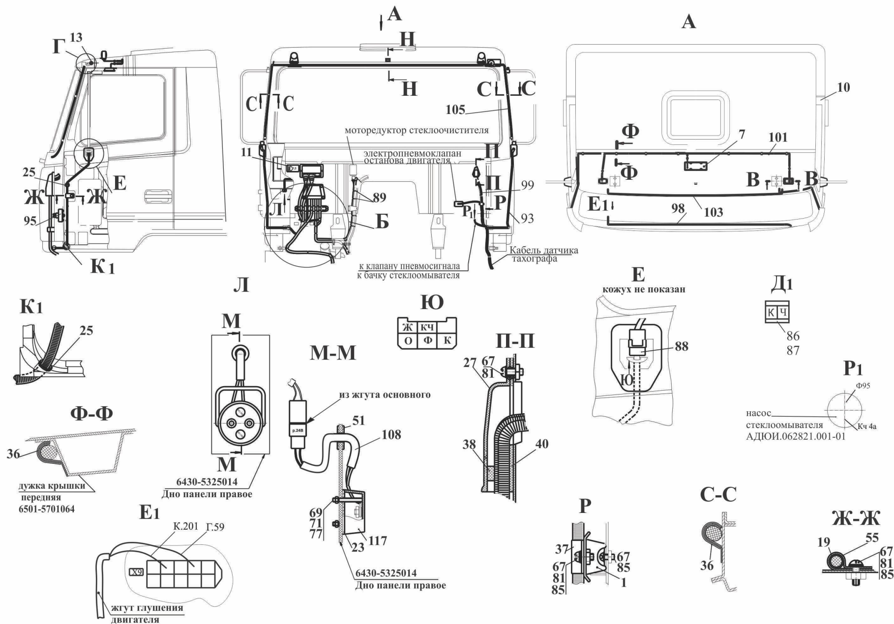
Рис.188 Установка электрооборудования на кабине 6501А9-3700076 (-700) (лист 1) Fig.188 Installation of an electrical equipment in cabin 6501А9-3700076 (-700)(page 1)
