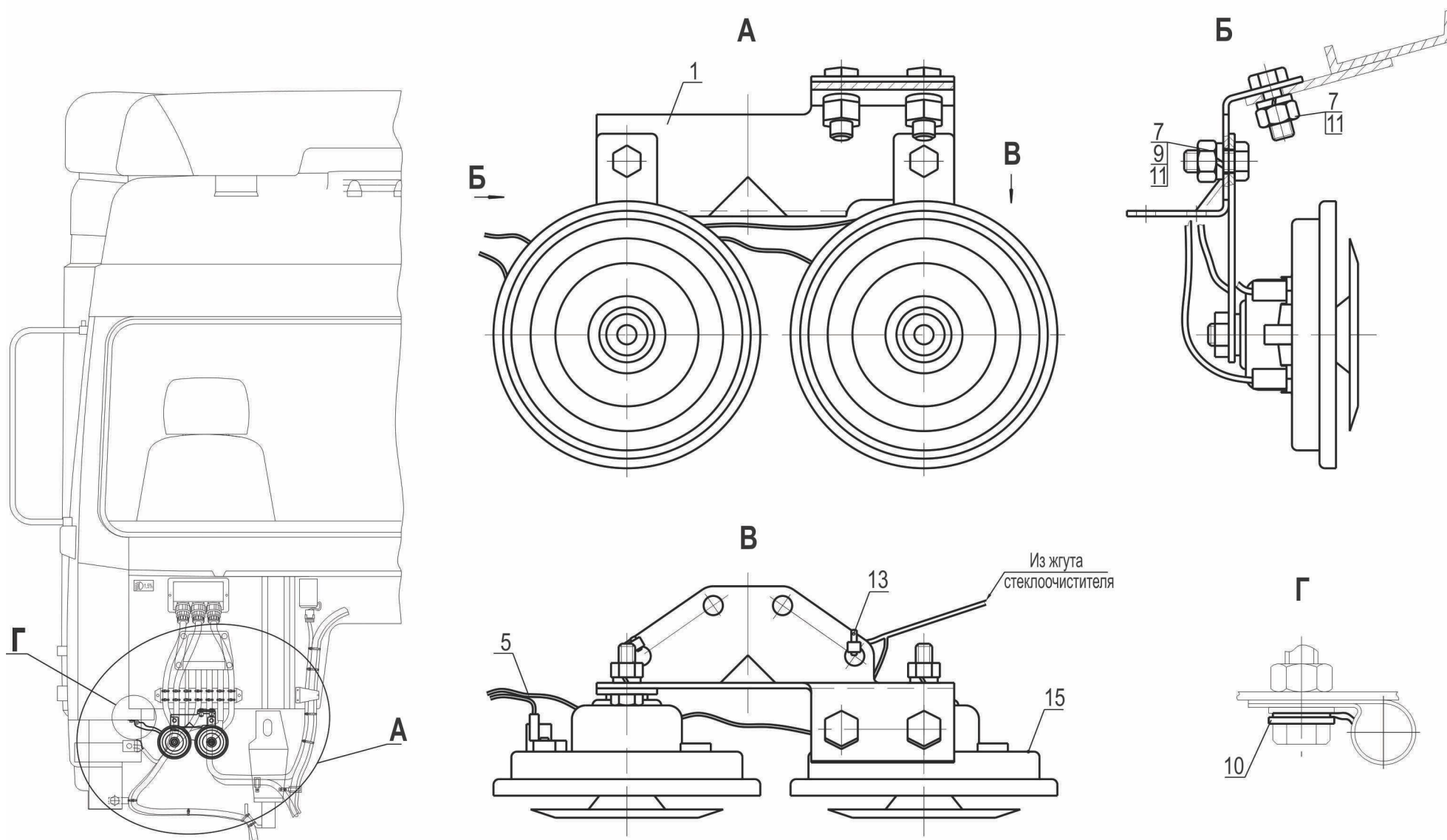
Рис. 195 Установка звуковых сигналов 643008-3700024-000 Fig. 195 Installation of audible signals 643008-3700024-000
