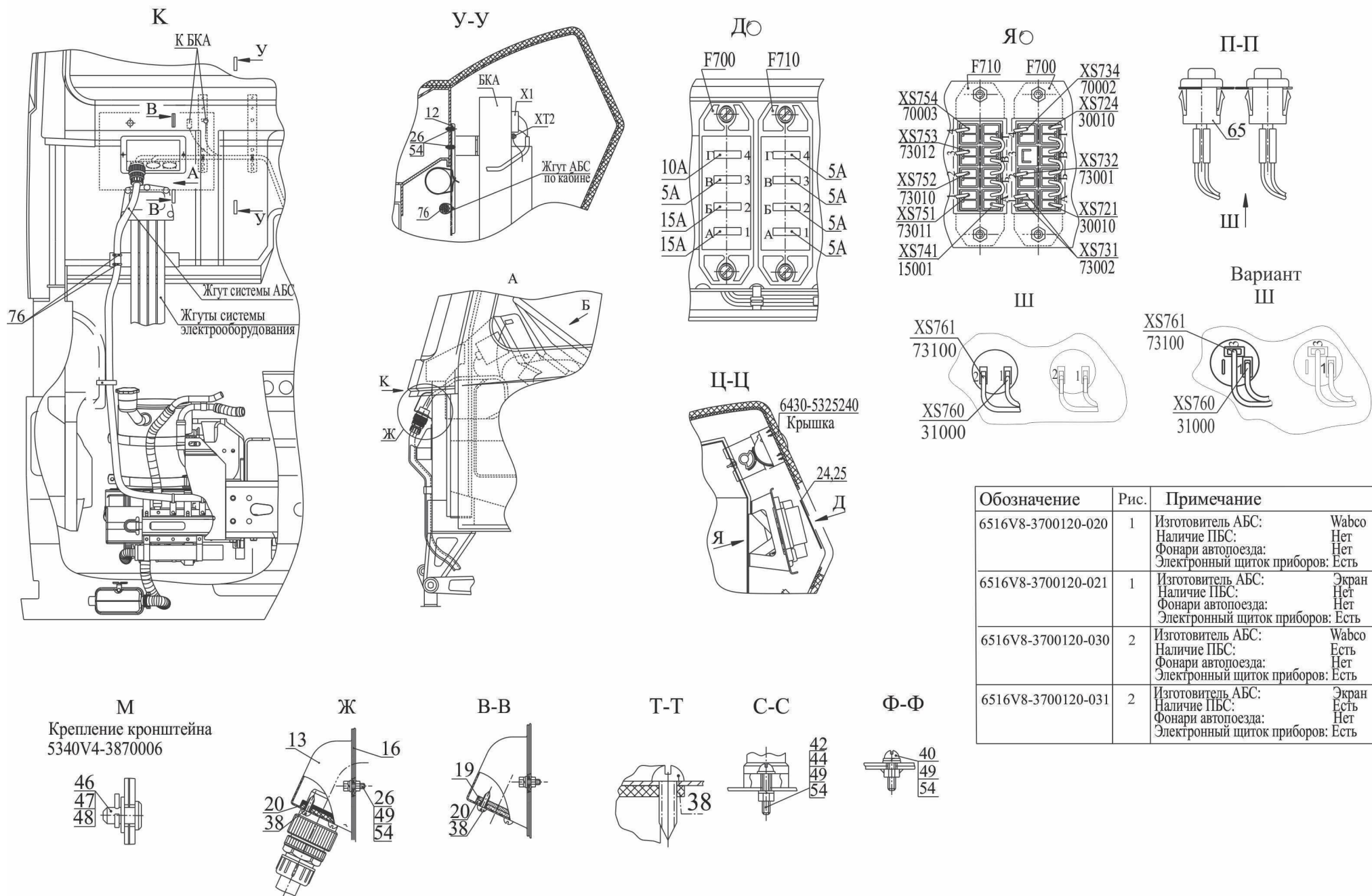
Рис.221 Установка электрооборудования АБС по кабине (лист 1) Fig. 221 Setting electrical equipment ABS on a cabin (page 1)
