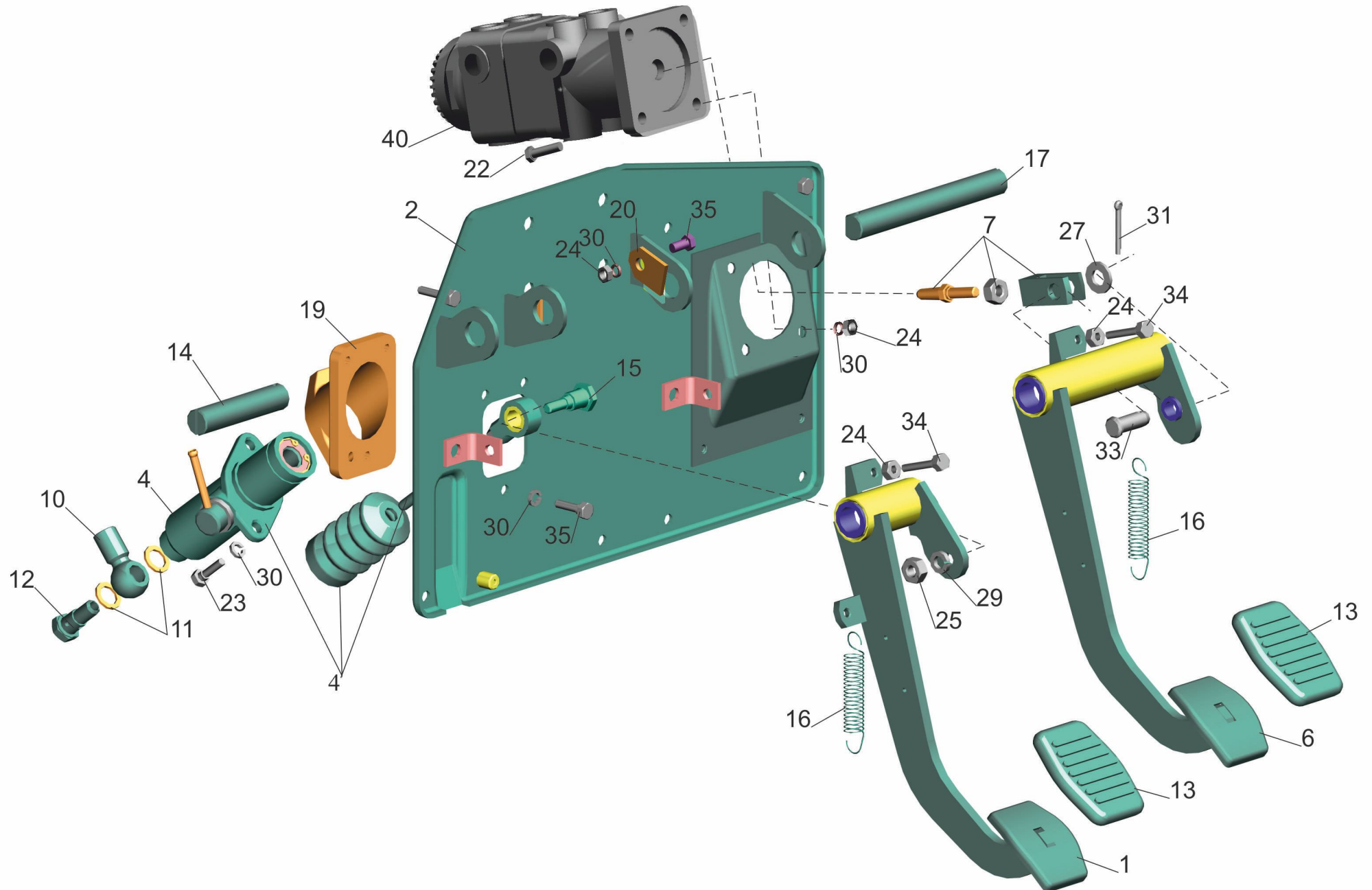
Рис. 41 Блок управления сцеплением 6430-1602004 Fig. 41 Clutch and brake control unit 6430-1602004
