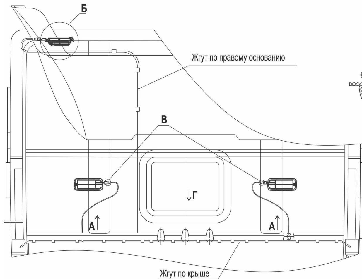
Рис. 191 Установка светильников в кабине 544008-3700136 Fig. 191 Installation of fixtures in a cabin 544008-3700136
