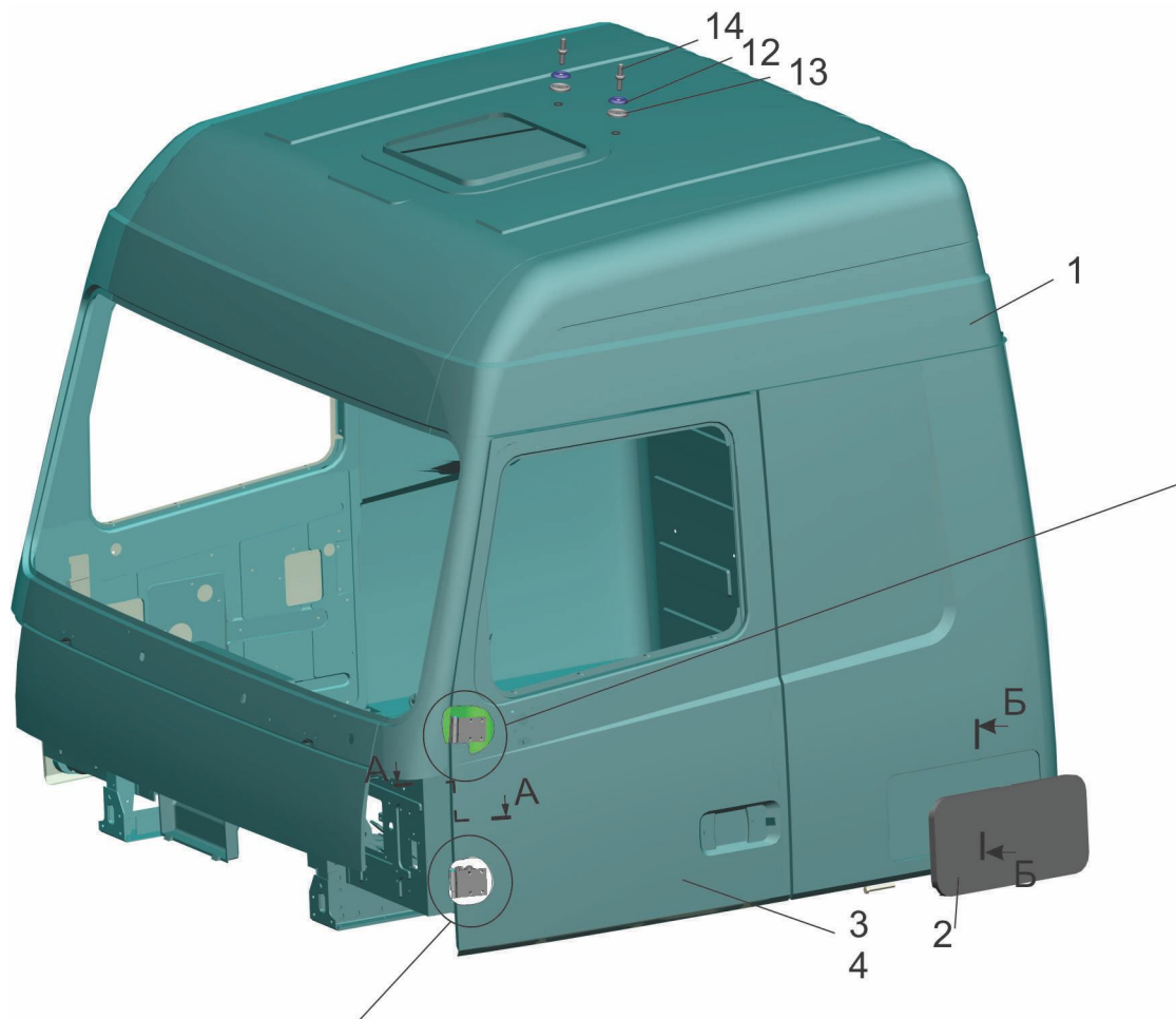
Рис.233 Кабина 5440-5000022-050 Fig. 233 Cabin 5440-5000022-050
