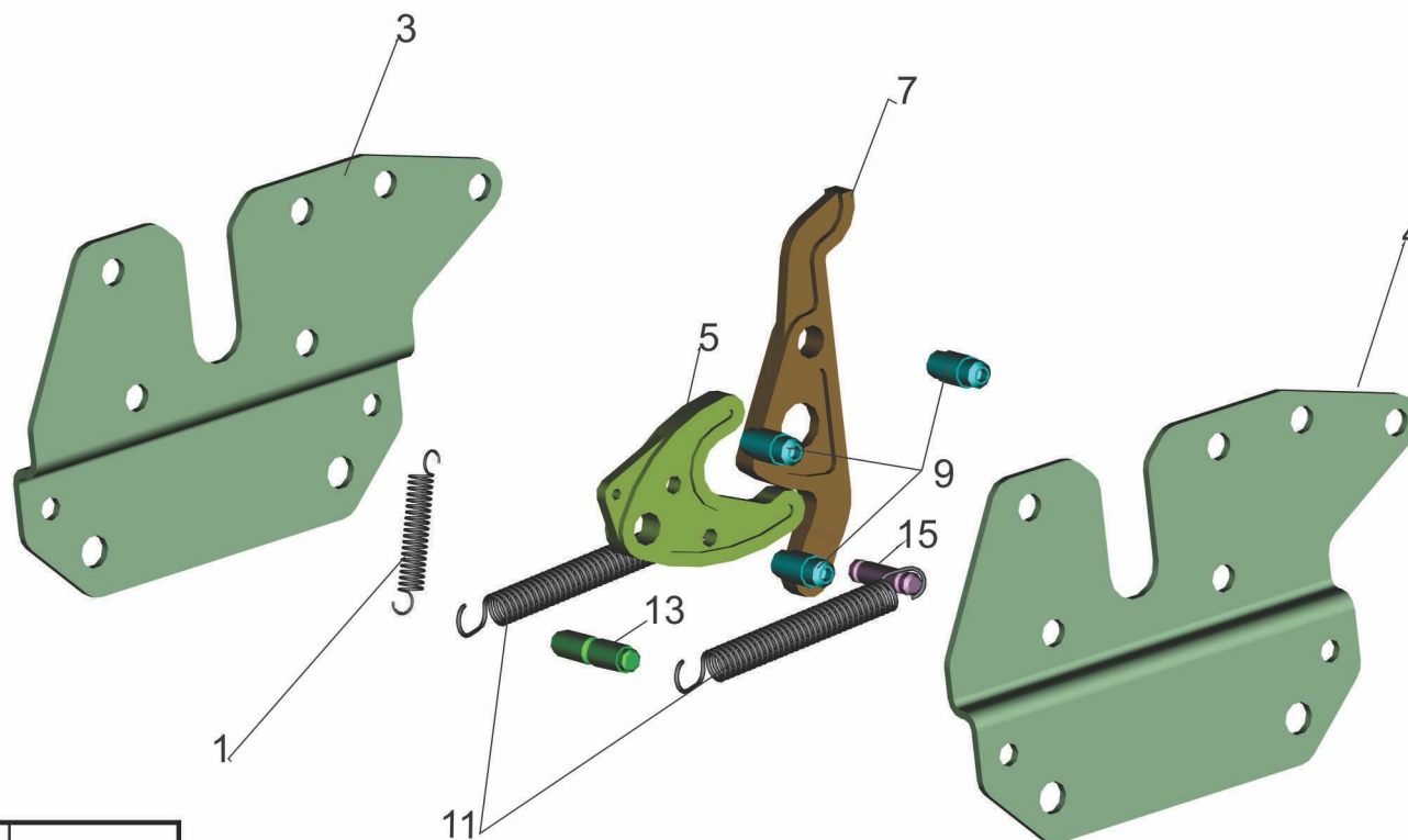
Рис. 227 Запорный механизм кабины 6501-5001550 Fig. 227 Cab lock mechanism 6501-5001550
