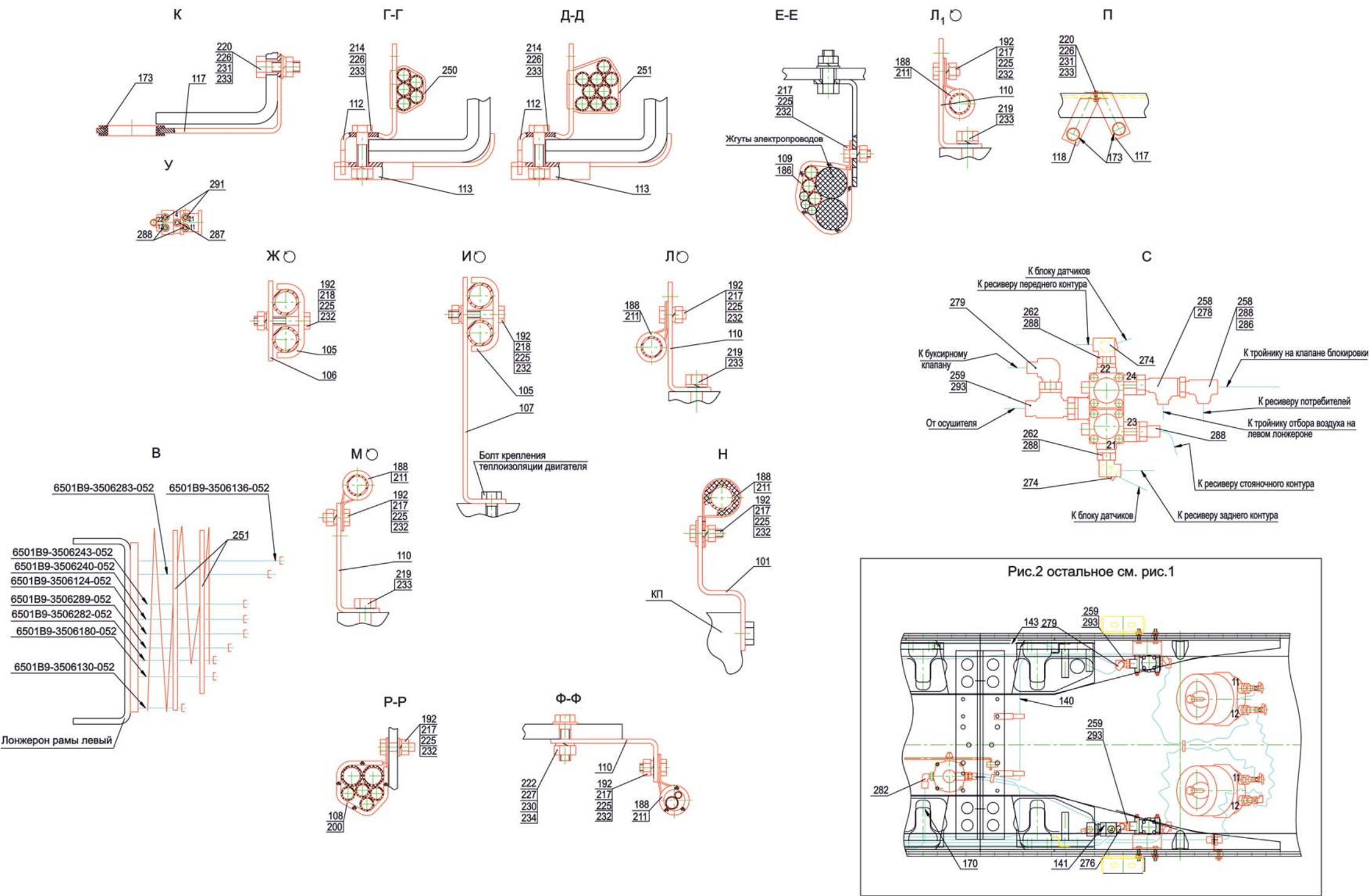
Рис.168 Установка пневмотормозов 6501В9-3500003-052(-053) (лист 2) Fig. 168 Installation pneumobrakes
