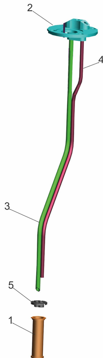
Рис. 21 Топливозаборник 650108-1105014 Fig. 21 Fuel intake 650108-1105014
