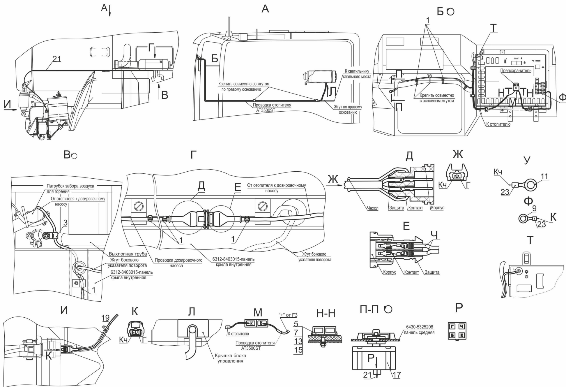
Рис. 303 Установка электрооборудования независимого отопителя 6430-3700088-010 Fig. 303 Setting of an electrical equipment of an independent heater 6430-3700088-010
