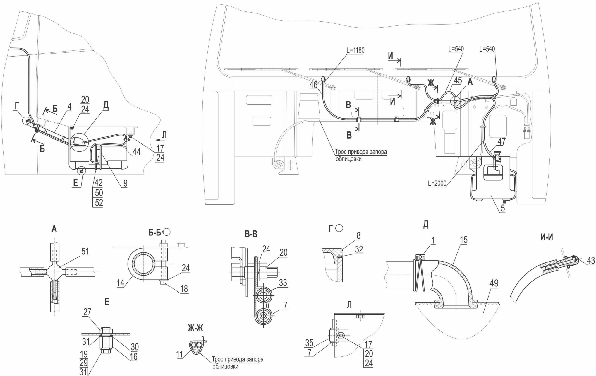
Рис. 243 Установка омывателя 6430-5200008 Fig. 243 Installation of washer 6430-5200008
