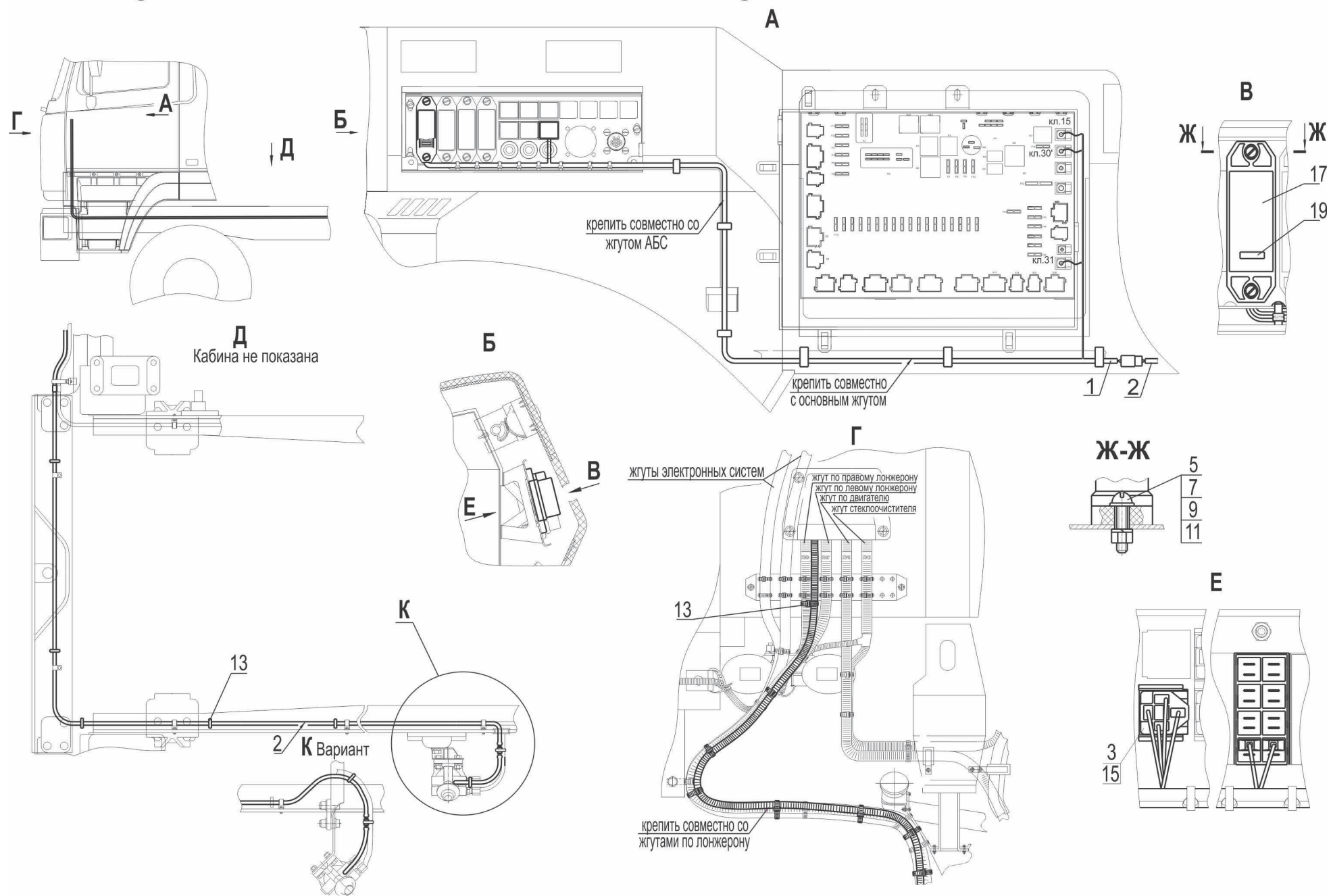
Рис. 200 Установка нагревателей на двигателе 6501P6-3700101-000 Fig.200 Installation of heaters on the engine 6501P6-3700101-000
