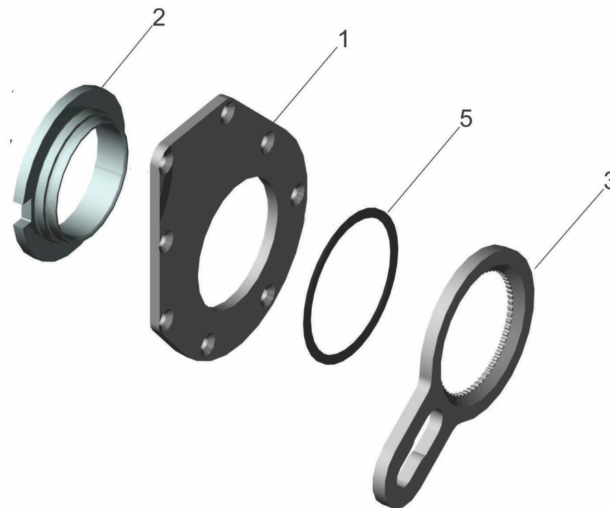
Рис. 78 Привод управляющий 64226-3501166 Fig. 78 Control drive 64226-3501166
