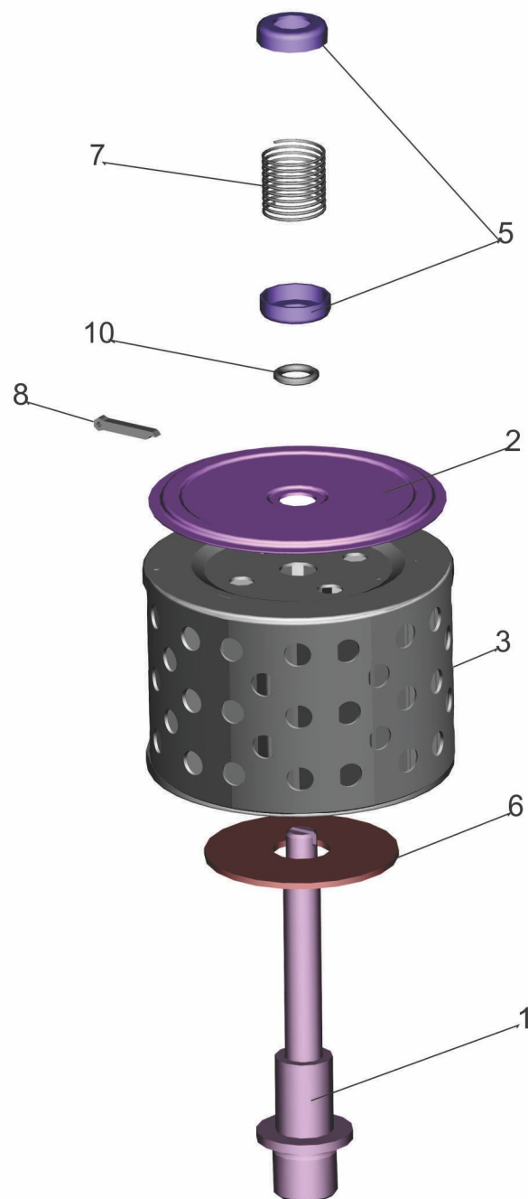
Рис. 163 Фильтр с клапаном 5336-3410051 Fig. 163 Filter with the valve 5336-3410051
