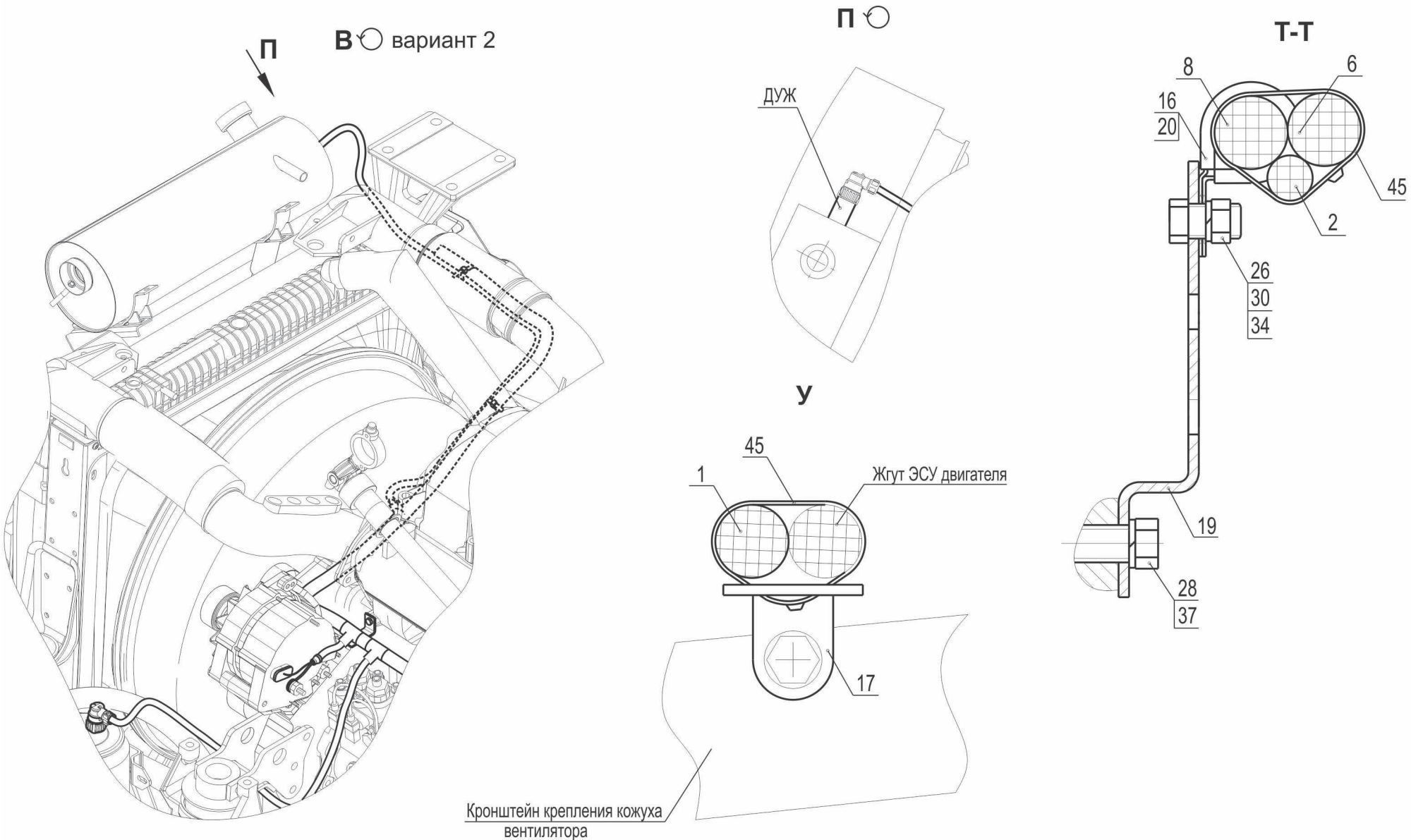
Рис.199 Установка электрооборудования на двигателе 5440A9-3700098, (-700) (лист 3) Fig. 199 Electric equipment installation on the engine 5440A9-3700098, (-700) (page 3)
