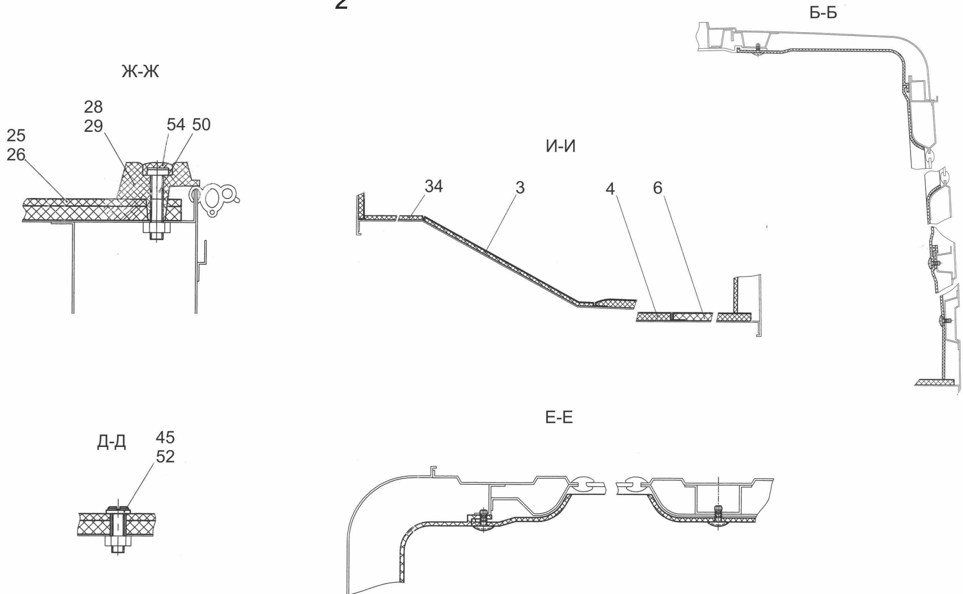
Рис. 238 Установка обивок и ковриков 6501-5000100 Лист 2 Fig.238 Installation of upholsteries and carpets 6501-5000100 Page 2
