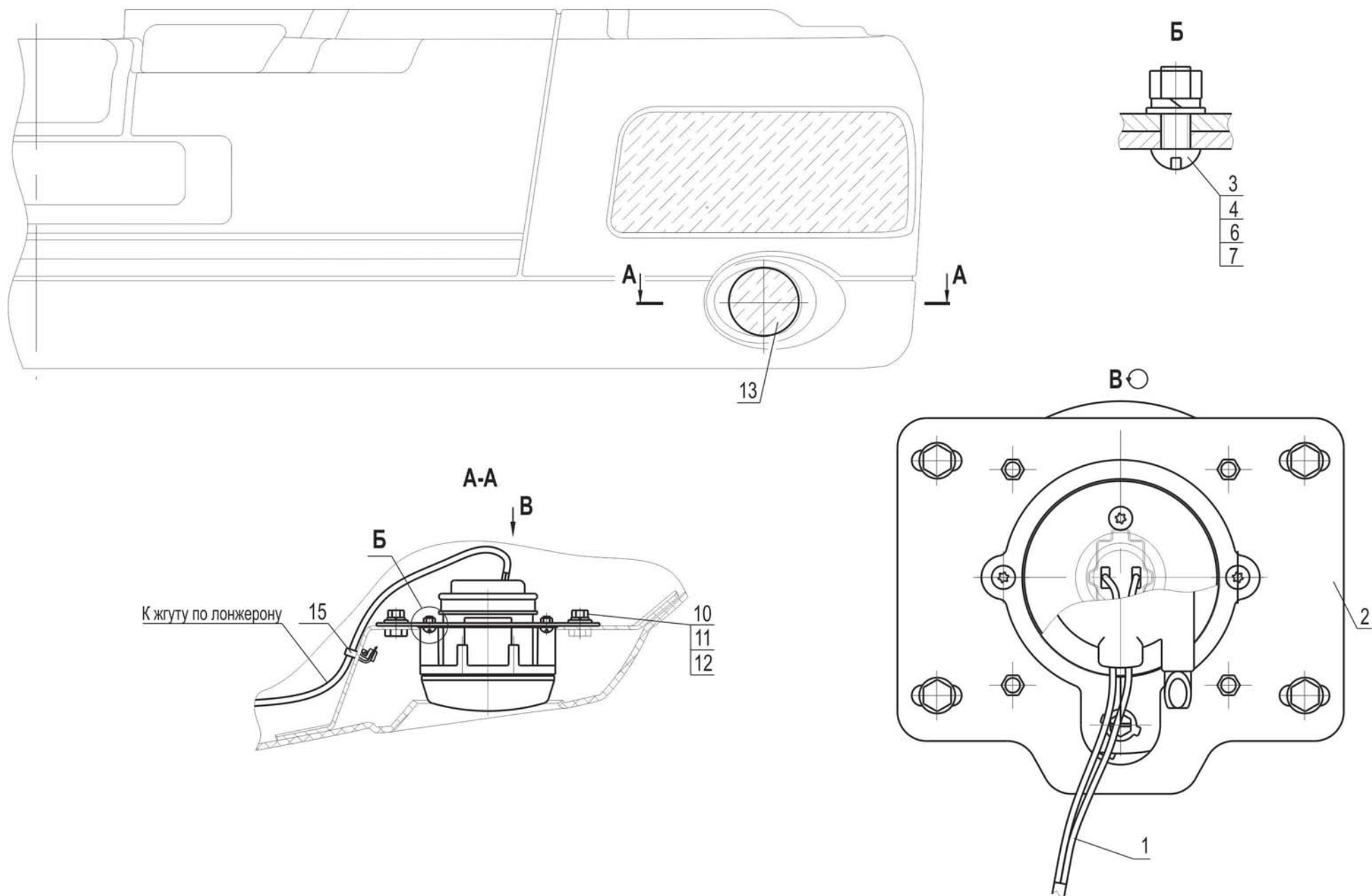
Рис.183 Установка противотуманных фар 447131-3700007-020 Fig. 183 Installation of fog lights 447131-3700007-020
