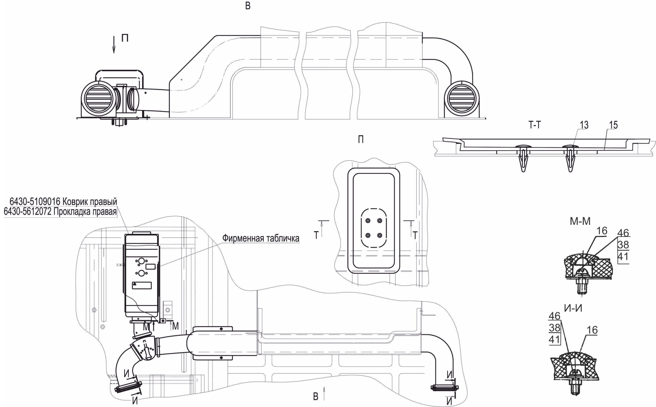
Рис. 299 Установка независимого воздушного отопителя 6430-8100002-021 Fig.299 Installation of the independent air heater 6430-8100002-021
