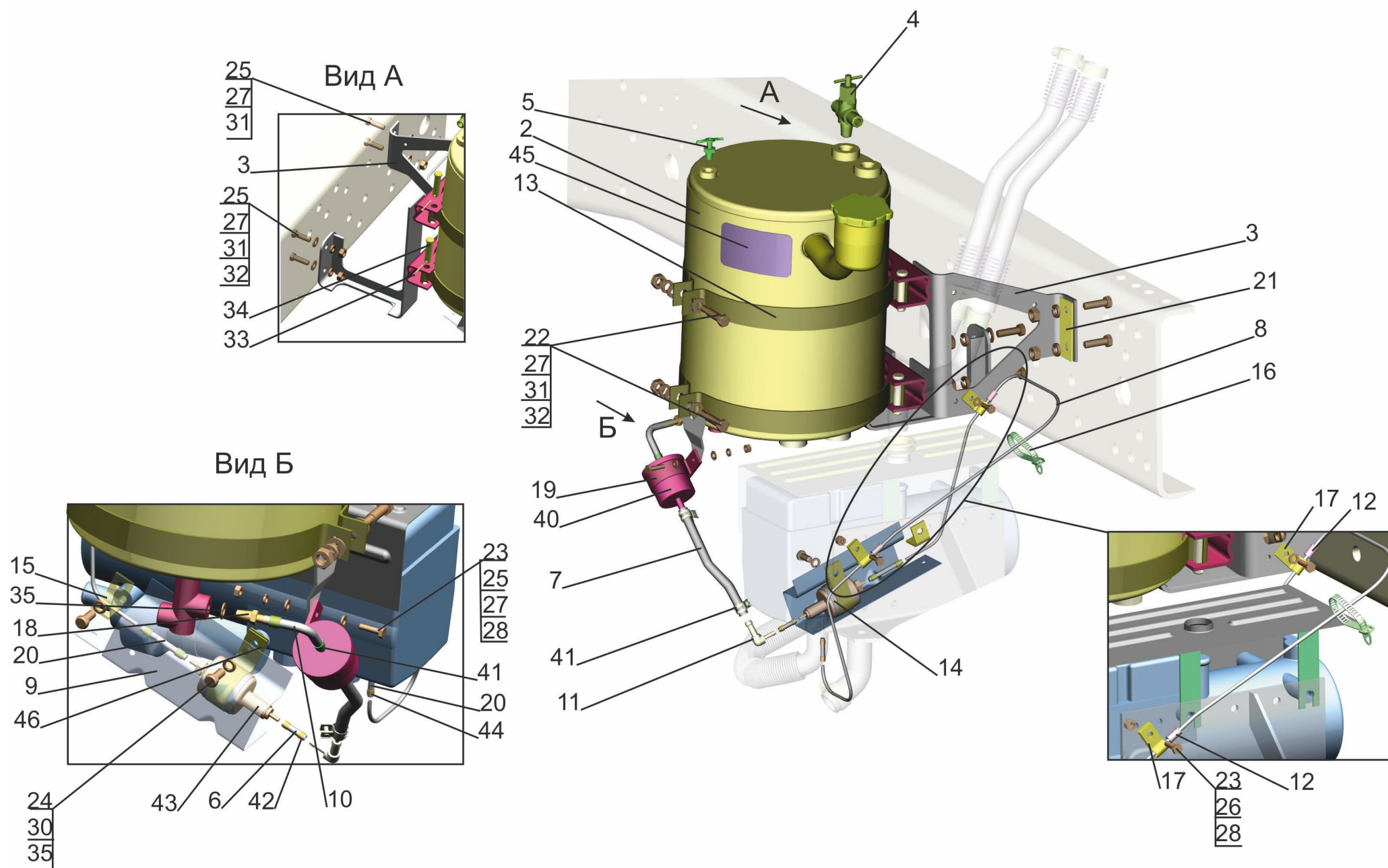
Рис.10 Установка топливопроводов подогревателя 6501B5-1015004 Fig.10 Mounting fuel lines of heater 6501B5-1015004
