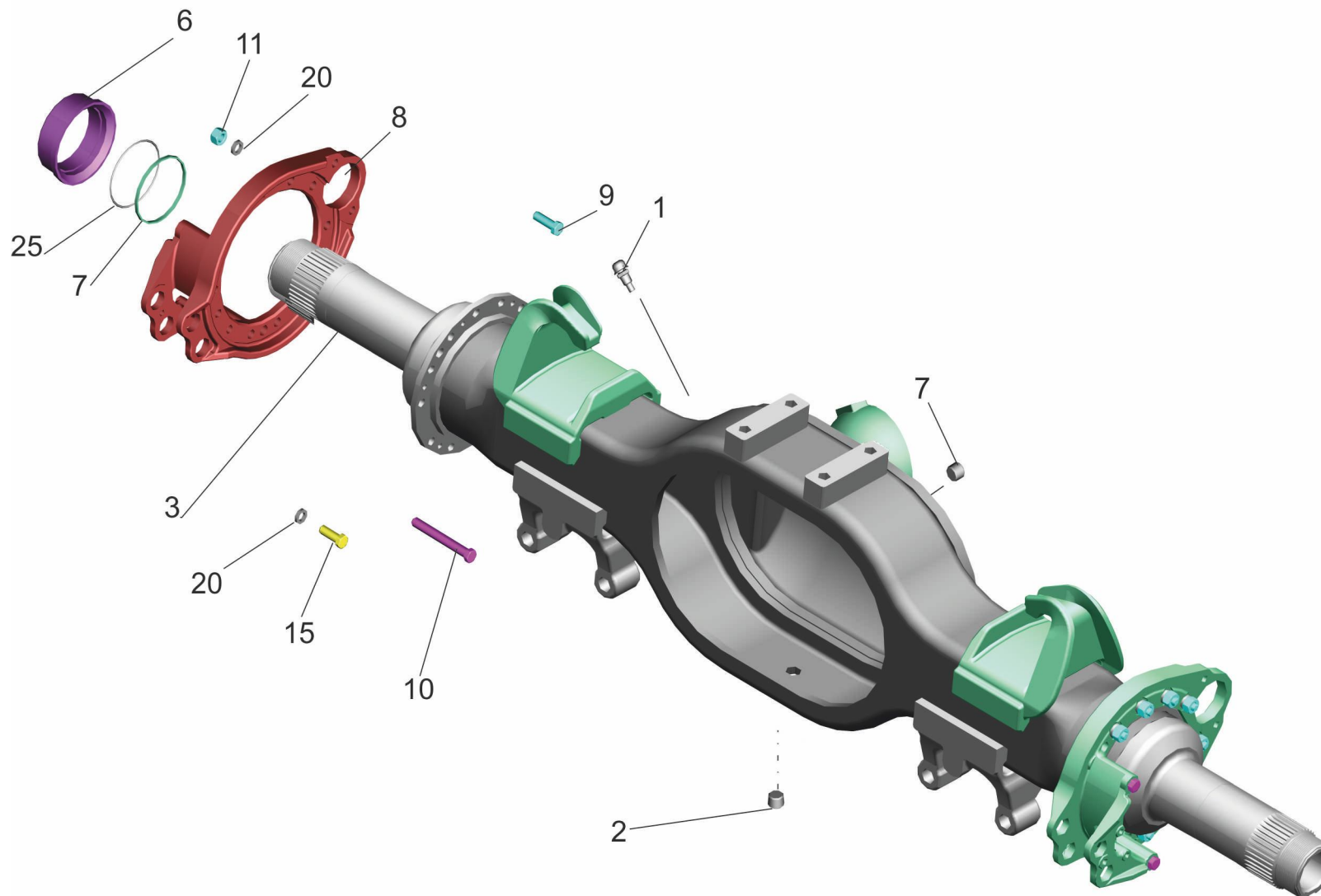
Рис. 87 Картер моста 6501W6-2501010-000 Fig. 87 Axle housing
