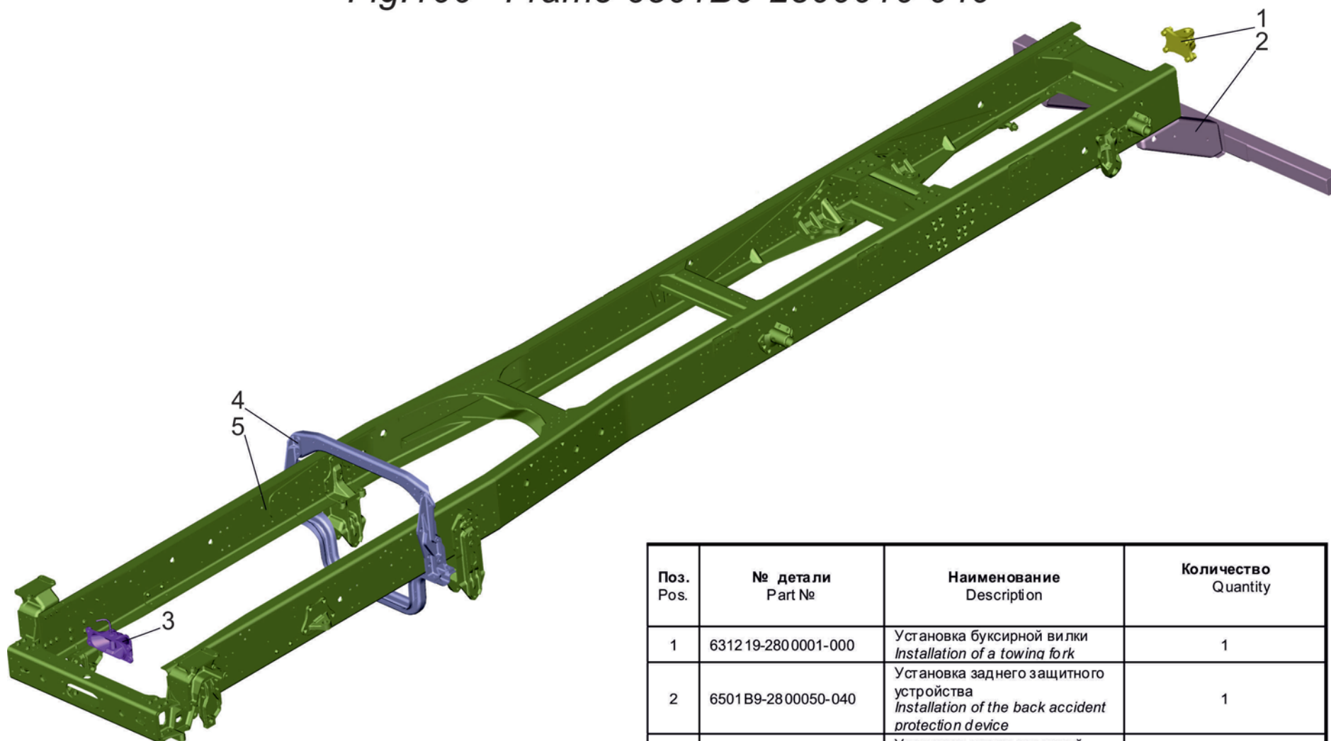
Рис.100 Рама 6501B9-2800010-040 Fig.100 Frame 6501B9-2800010-040
