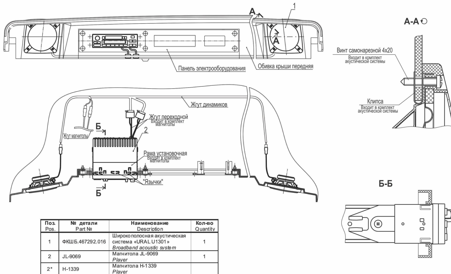
Рис.212 Установка радиоприемника с CD проигрывателем 6501-7900030 Fig.212 Installation of receiver with CD player 6501-7900030
