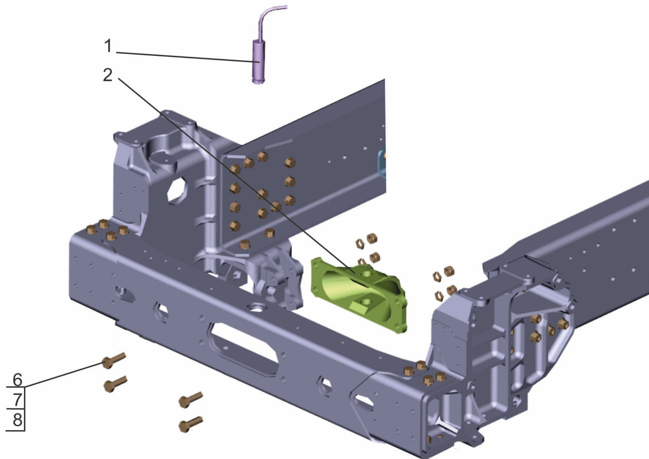
Рис.104 Установка вилки передней 631219-2800070-000 Fig.104 Installation of a fork of a lobby 631219-2800070-000
