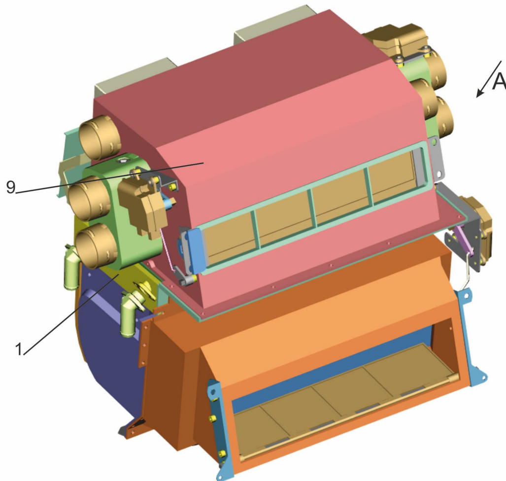
Fig. 286 Heater 643008-8101010
