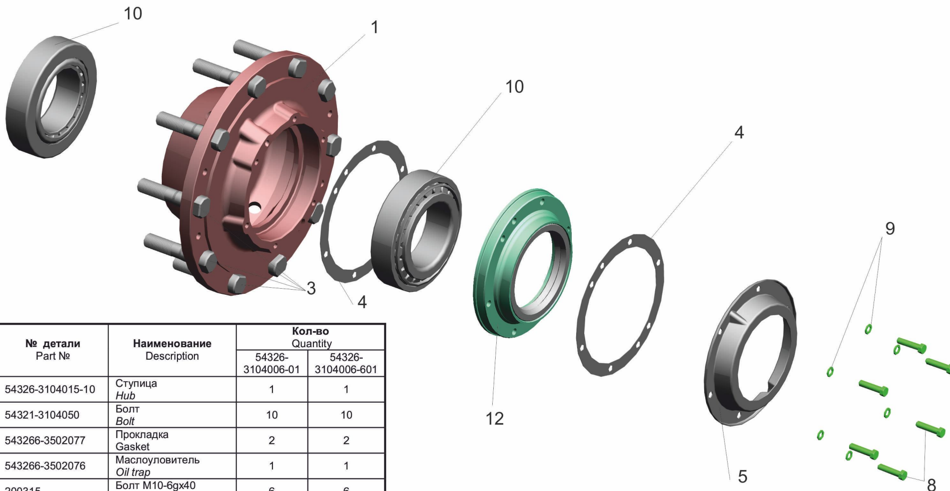
Рис. 82 Ступица с крышкой Fig. 82 Rear axle hub
