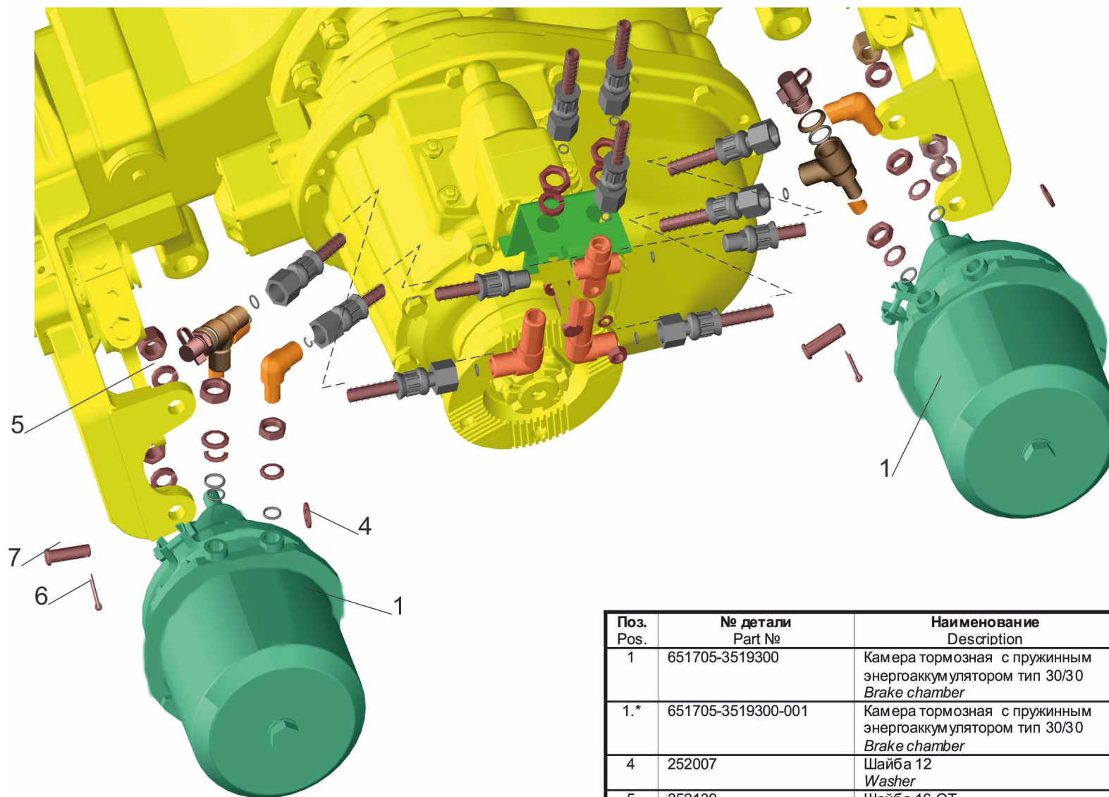
Рис. 176 Крепление тормозных камер 650105-3519003-000 Fig. 176 Installation of brake chambers 650105-3519003-000
