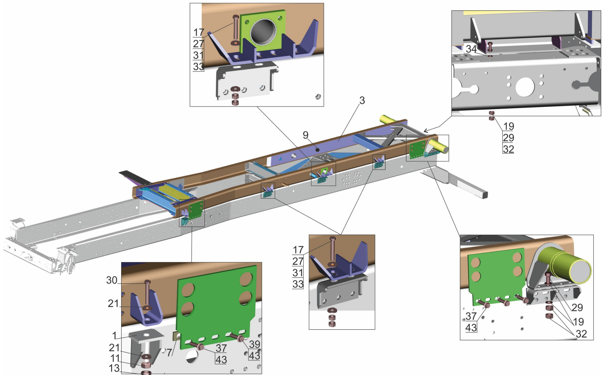
Рис.328 Установка надрамника 6501B9-8600002-020 Fig.328 Installation above frame 6501B9-8600002-020
