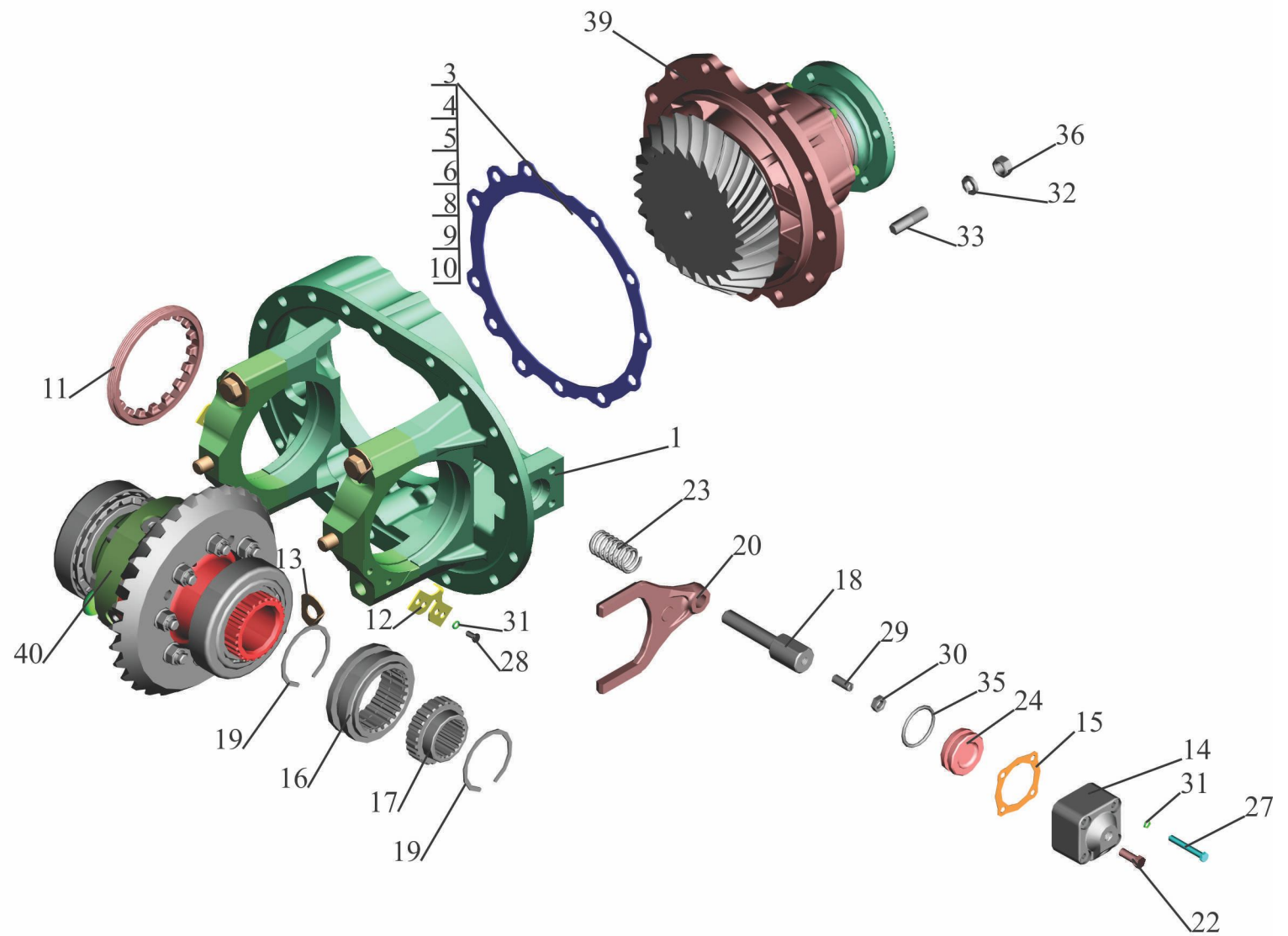
Рис. 71 Редуктор Fig. 71 Reducer gear
