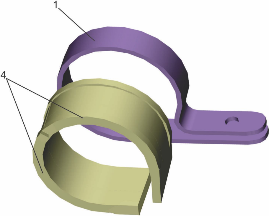
Рис.309 Кляммер 544020-8117052 Fig.309 Clamp 544020-8117052
