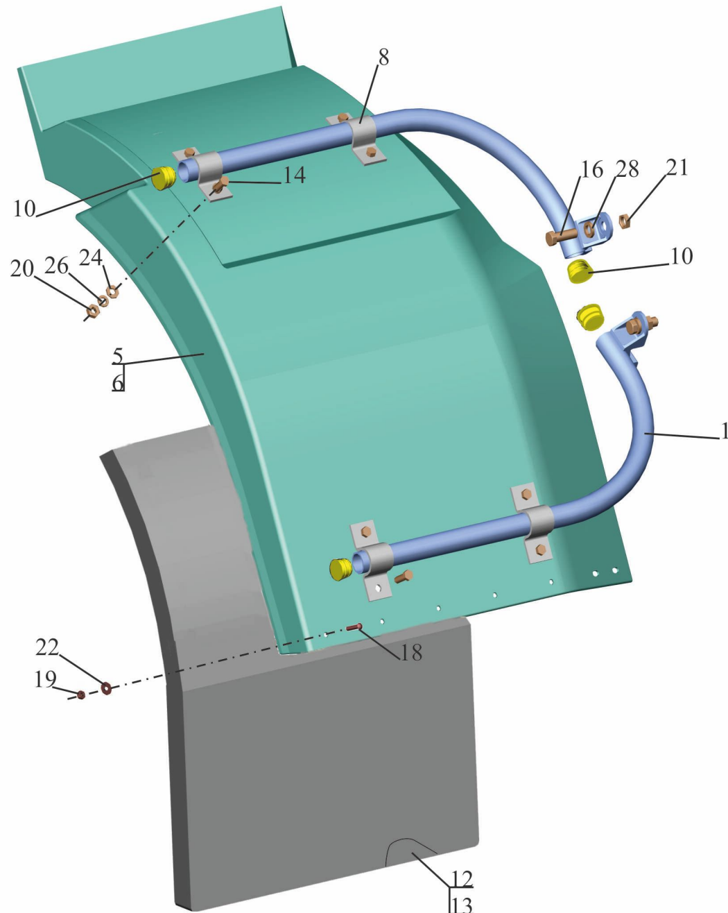
Рис. 320 Установка брызговиков передних колес 6430-8400030-031 Fig. 320 Installation of mudguard 6430-8400030-031
