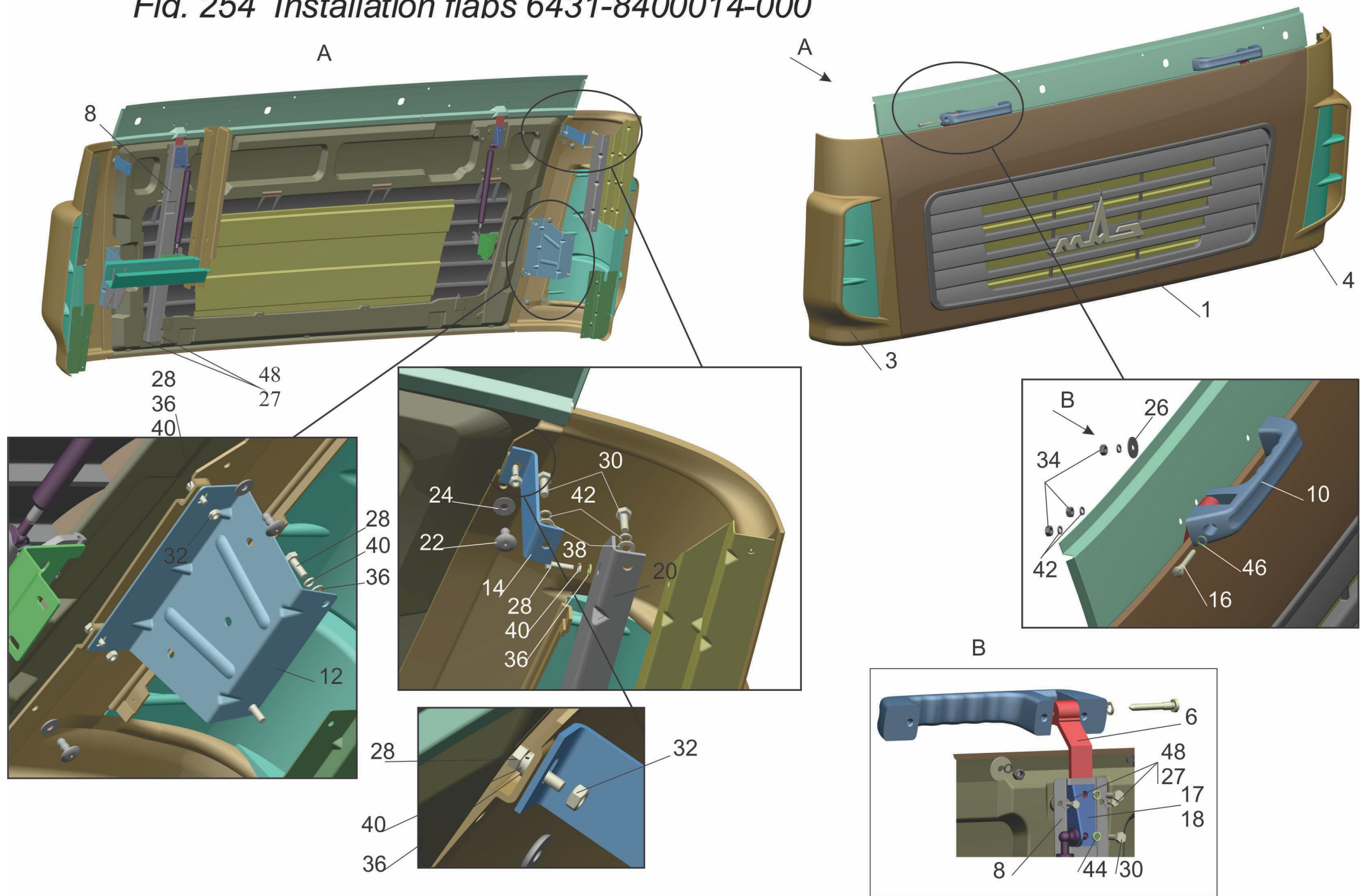
Рис.254 Установка щитков 6431-8400014-000
