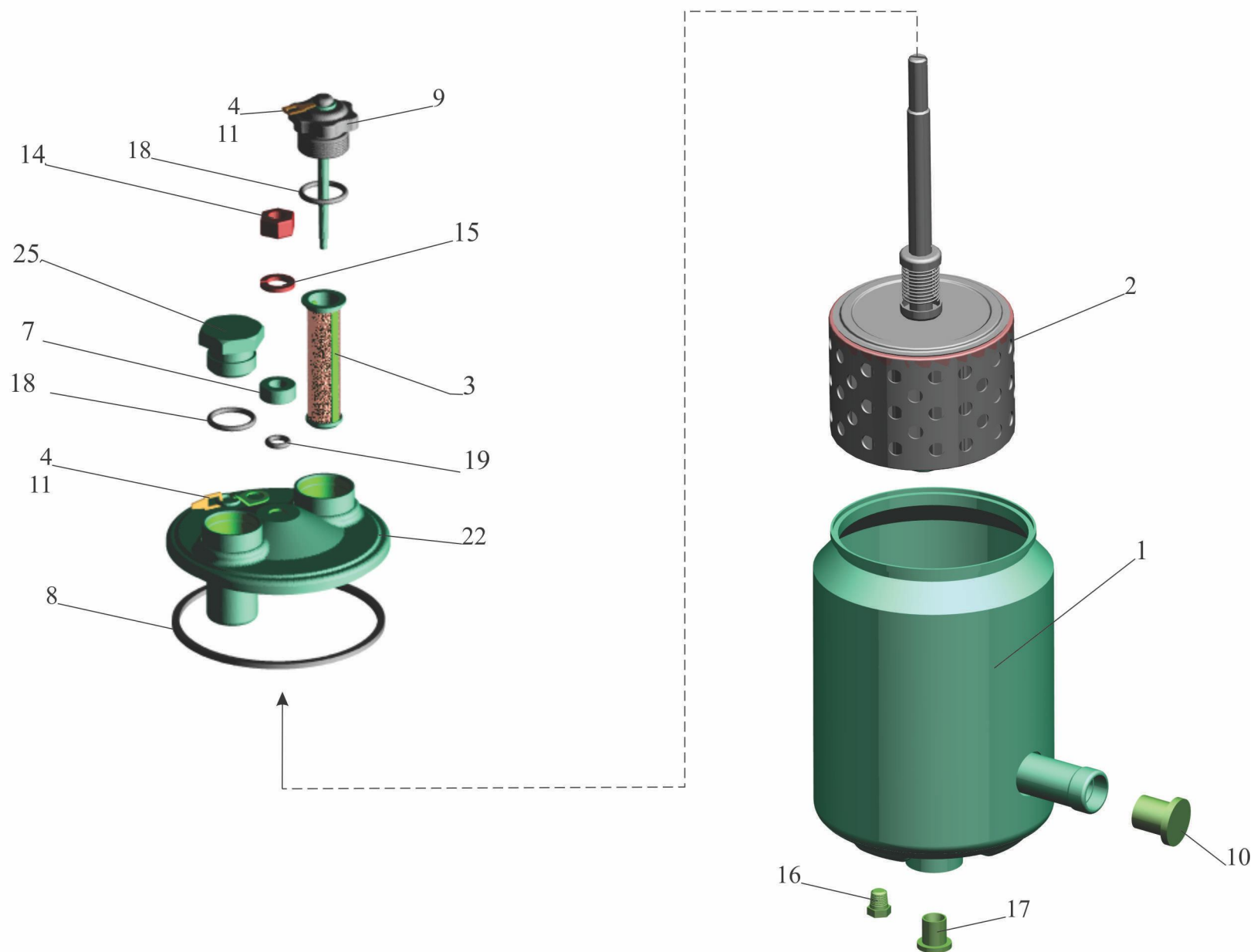
Рис. 162 Бак масляный 5336-3410010-10 Fig. 162 Oil tank 5336-3410010-10
