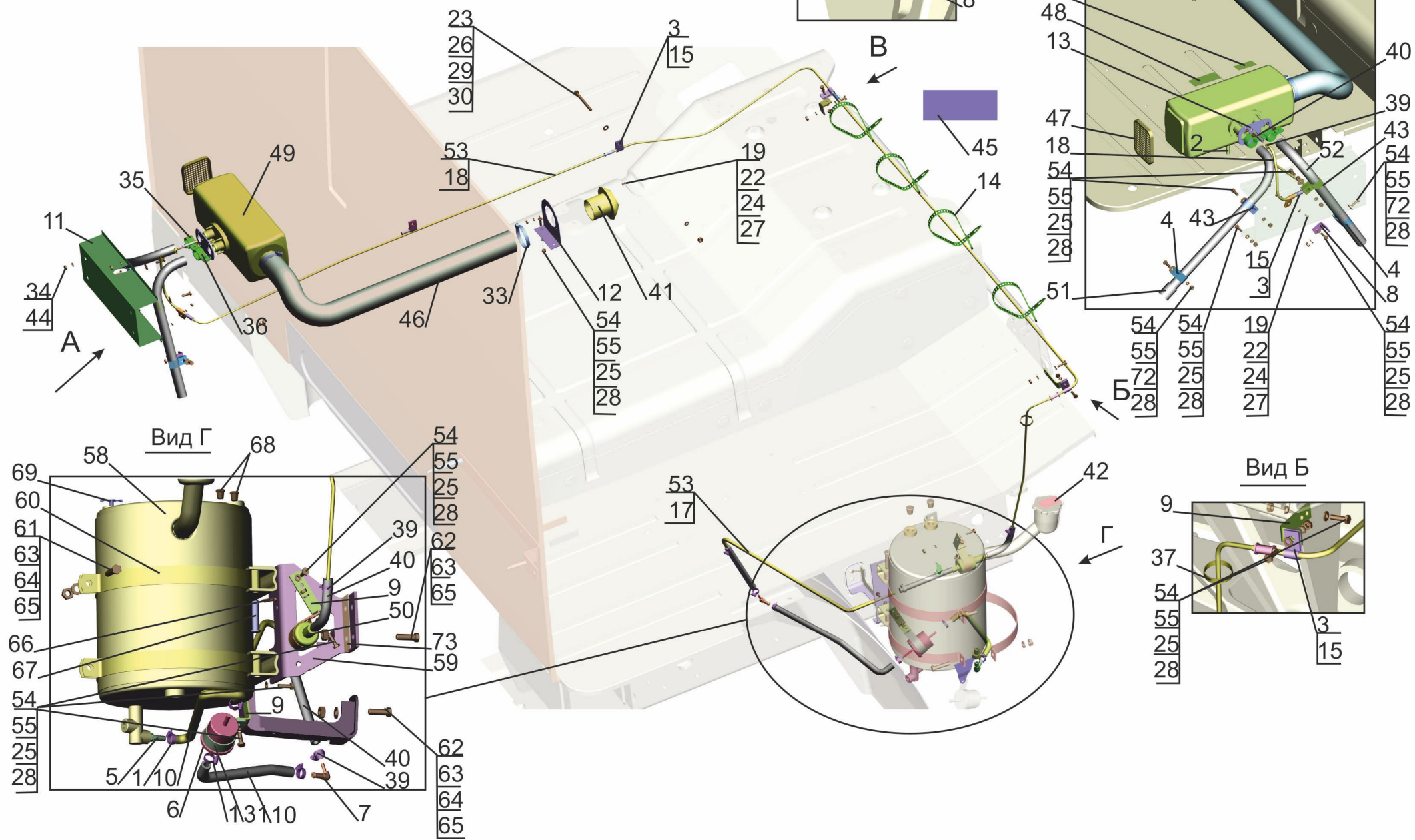
Рис.294 Установка независимого воздушного отопителя 6501-8100002-011 Fig.294 Installation of the independent air heater 6501-8100002-011
