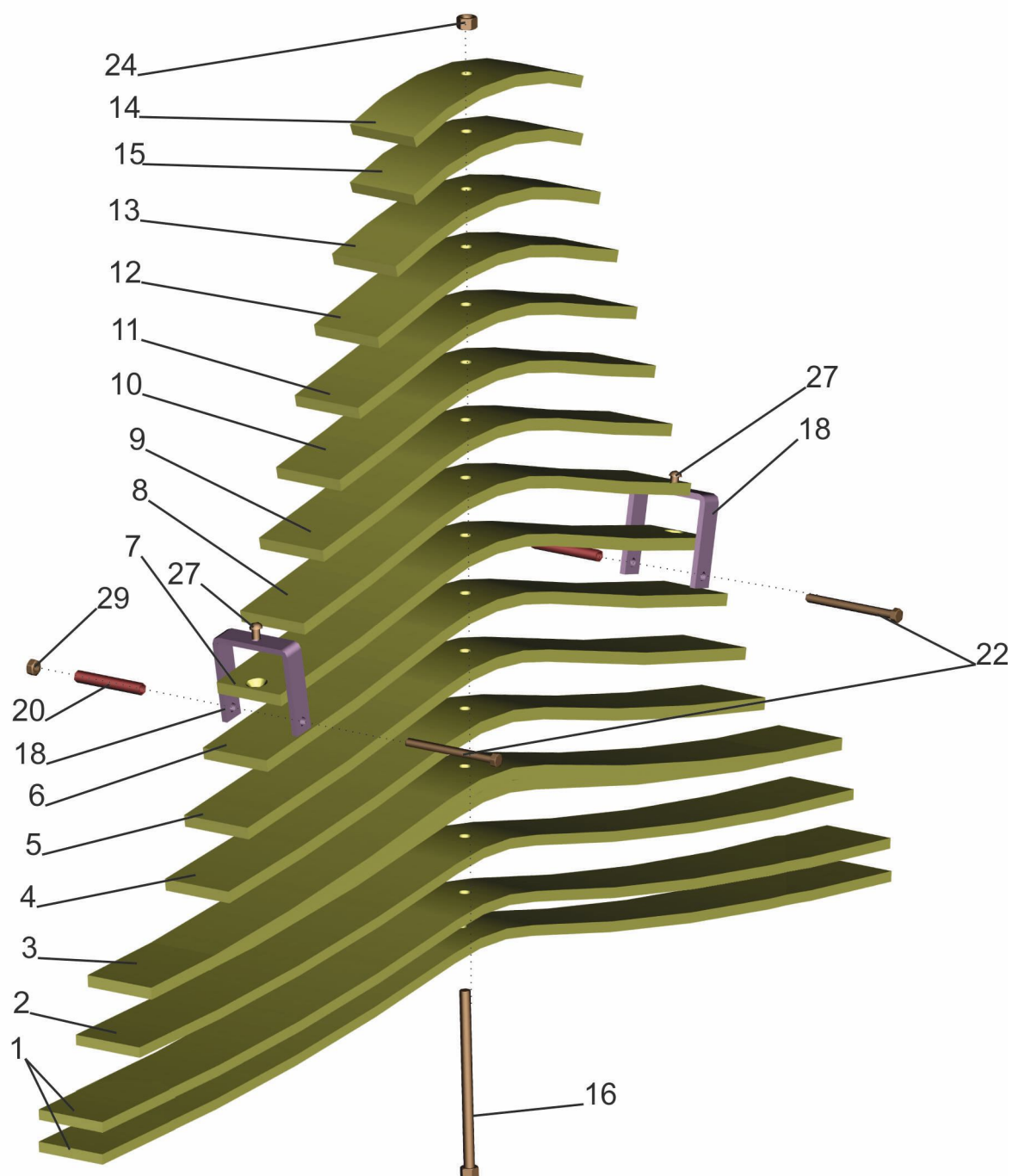
Рис. 117 Рессора задняя 55165-2912012-010 Fig. 117 Back leaf spring 55165-2912012-010
