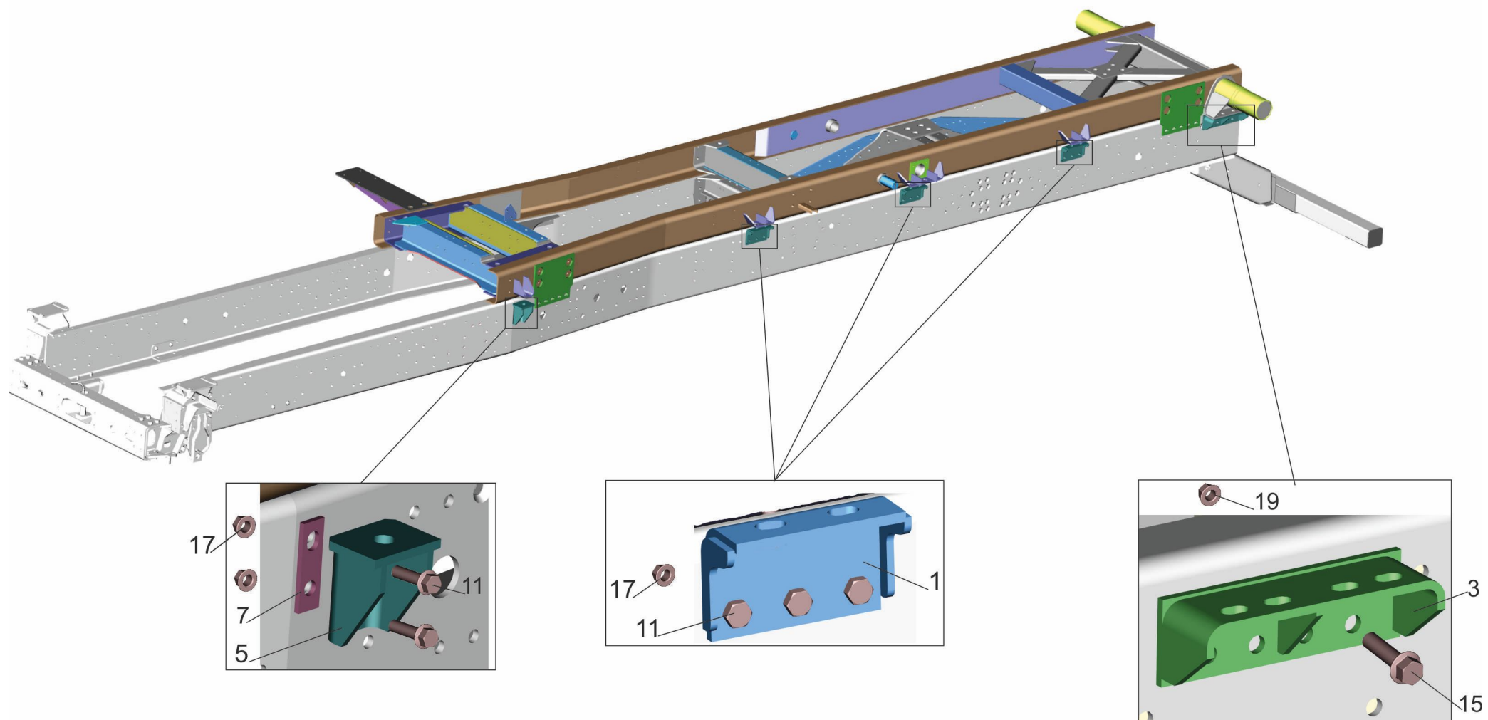
Рис.329 Крепление кронштейнов 6501В9-8600060-020 Fig.329 Fastening brackets
