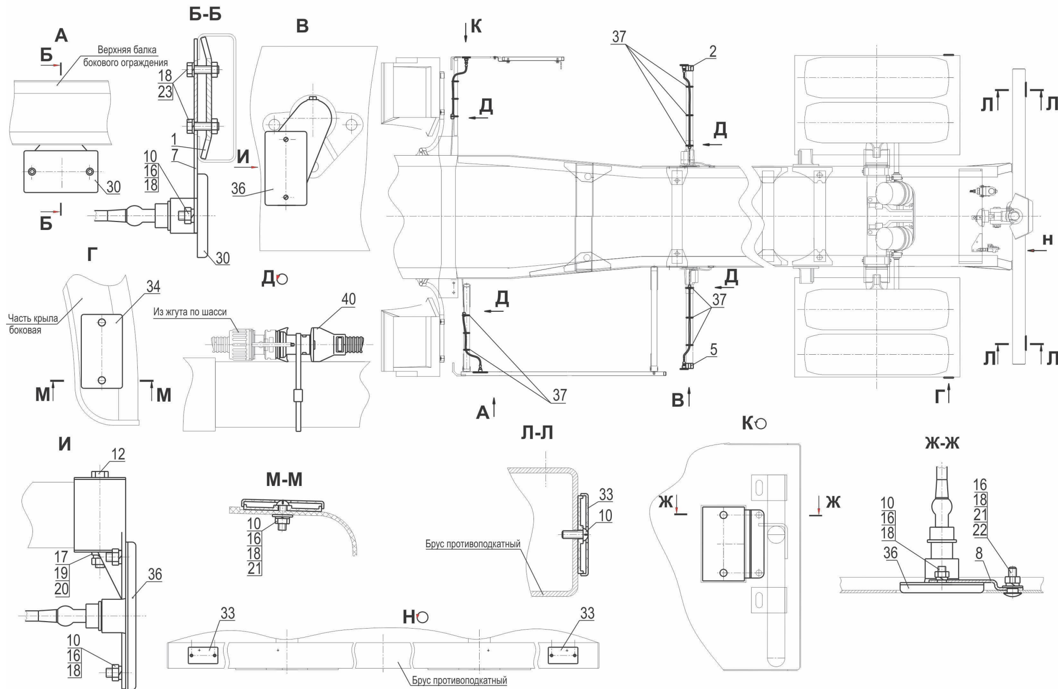
Рис.197 Установка боковых габаритных фонарей 6501В9-3700080-010, (-710) Fig.197 Installation of lateral fender light 6501В9-3700080-010, (-710)
