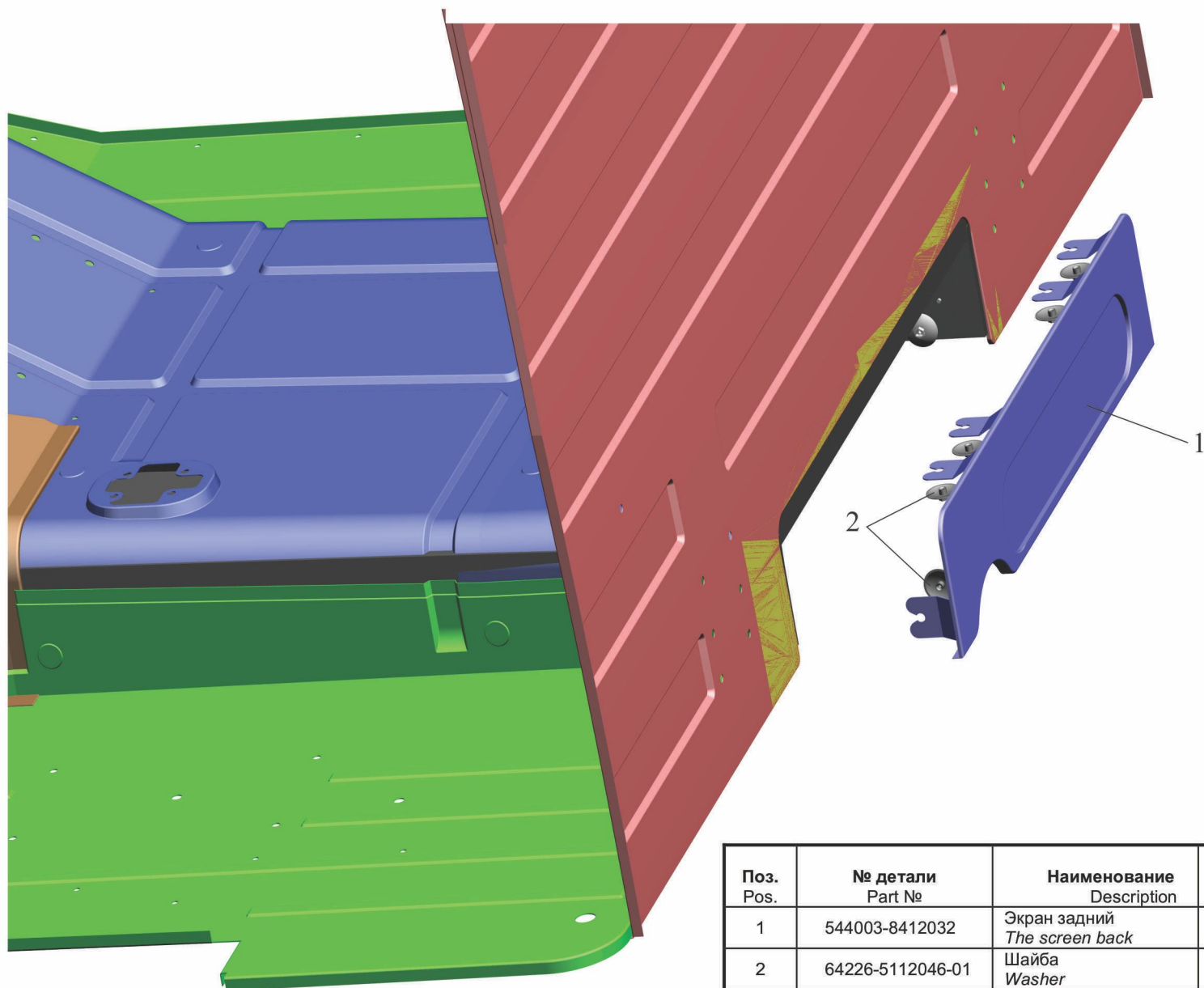
Рис.317 Установка экранов 544003-8400026 Fig.317 Installation of screens 544003-8400026
