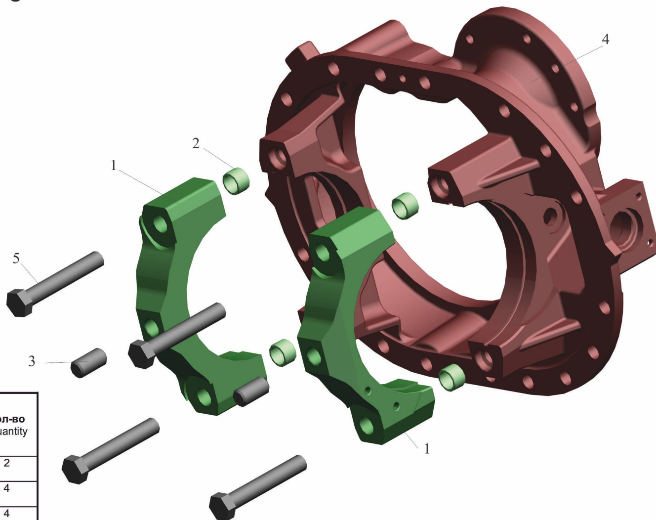
Рис. 89 Картер редуктора 6430-2502015-010 Fig. 89 Reducer gear housing 6430-2502015-010
