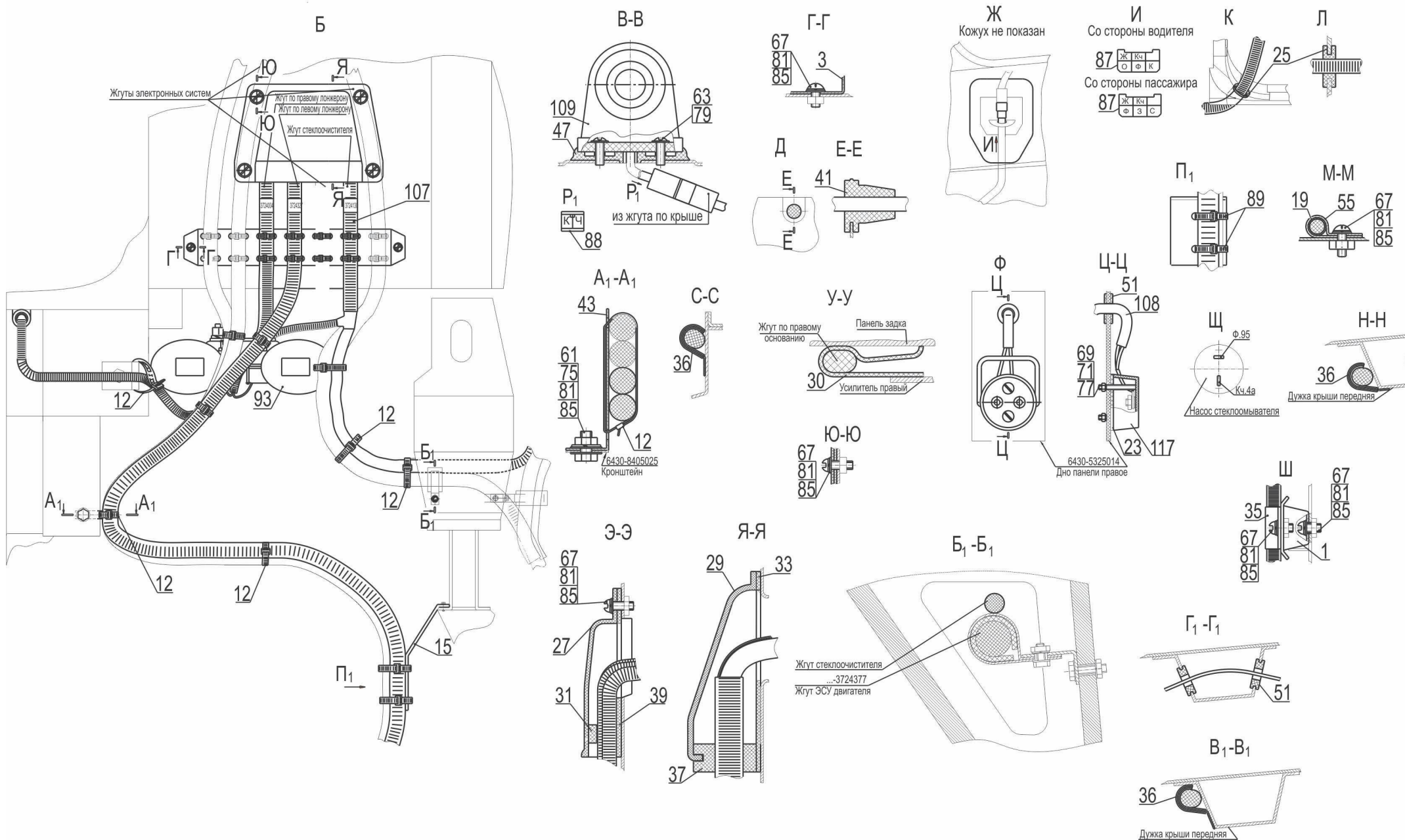
Рис. 189 Установка электрооборудования по кабине 5340В7-3700076-000 (лист 2) Fig. 189 Electric equipment installation on a cabin 5340В7-3700076-000 (page 2)
