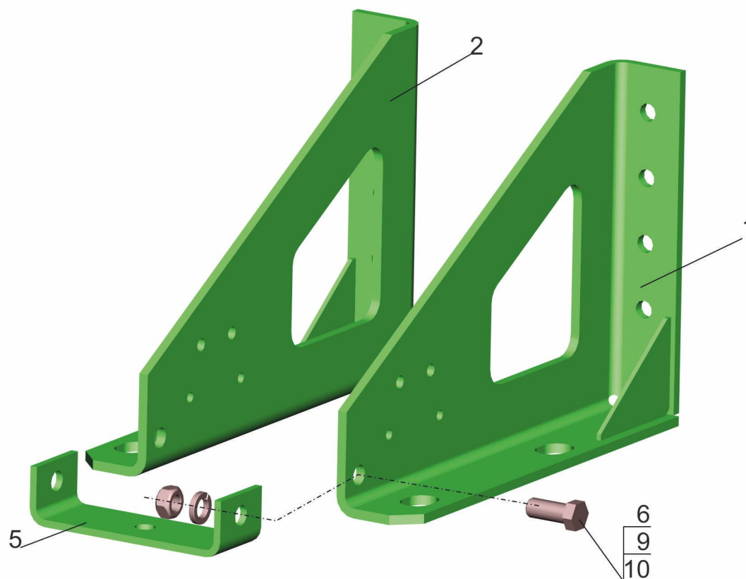
Рис. 139 Кронштейн 534013-3105053-000 Fig. 139 Bracket 534013-3105053-000
