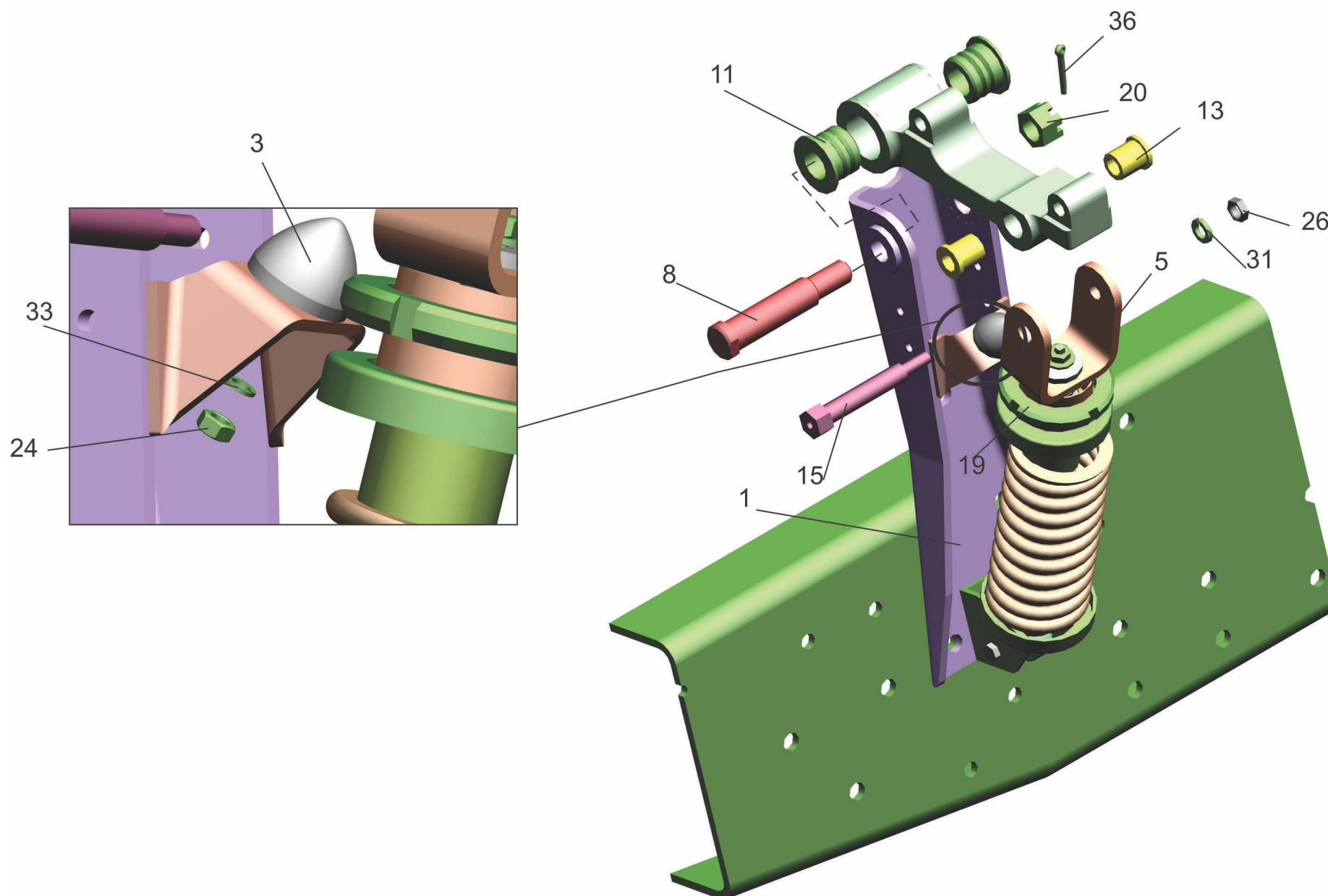
Рис. 231а Заднее подрессоривание 6430-5001802-011 Fig. 231a Rear springing 6430-5001802-011
