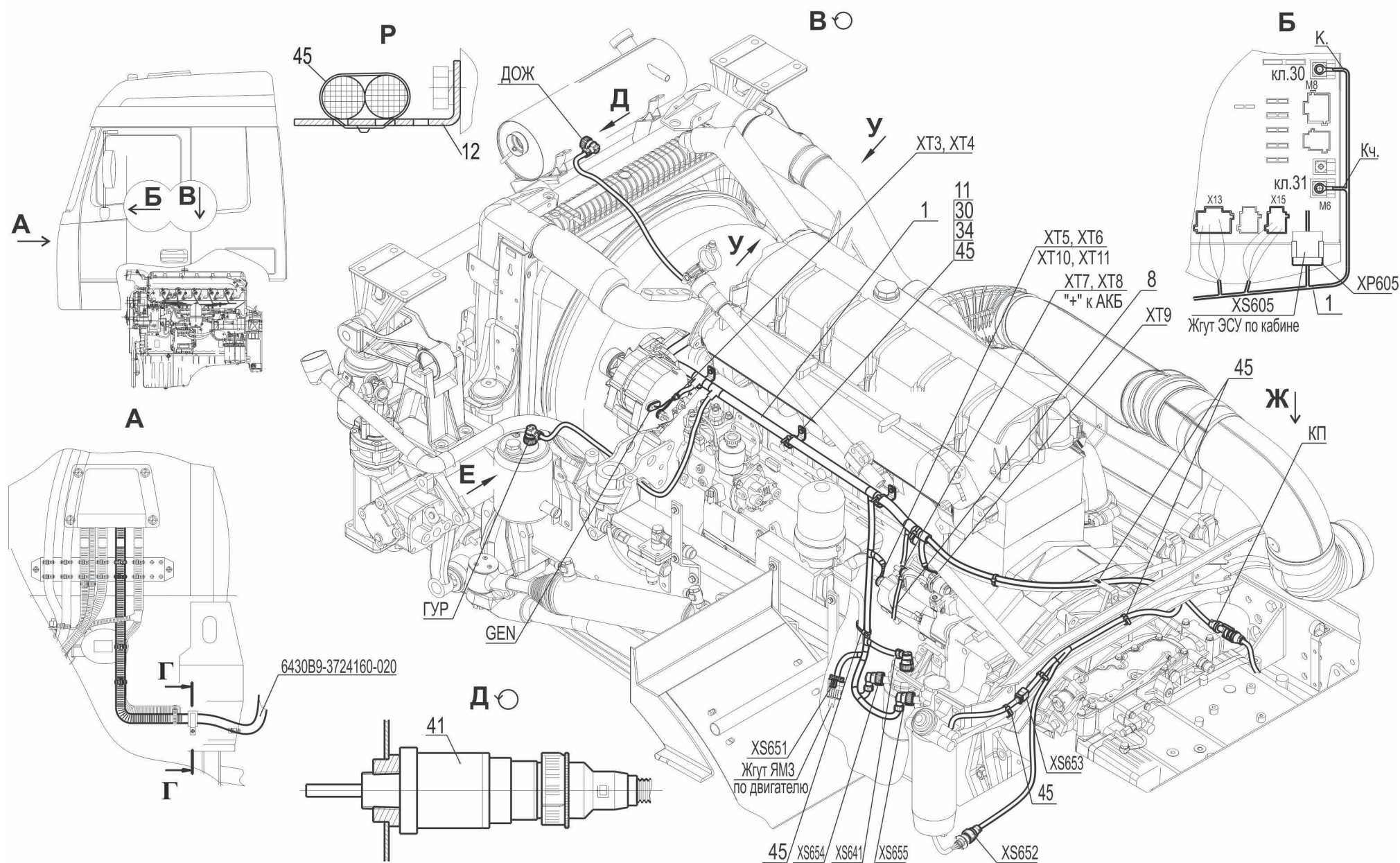
Рис.199 Установка электрооборудования на двигателе 5440A9-3700098, (-700) (лист 1) Fig.199 Electric equipment installation on the engine 5440A9-3700098, (-700) (page 1)
