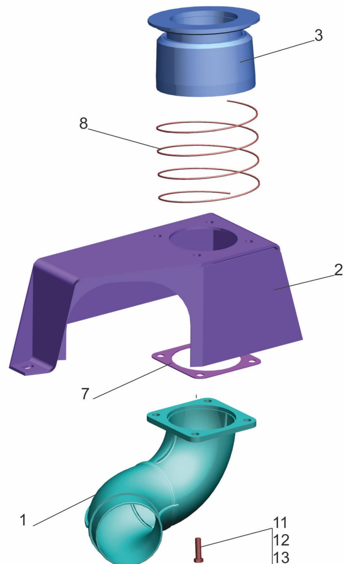
Рис. 34 Узел подвода газов 6501B9-1203220-010 Fig. 34 Knot of a supply of gases 6501B9-1203220-010
