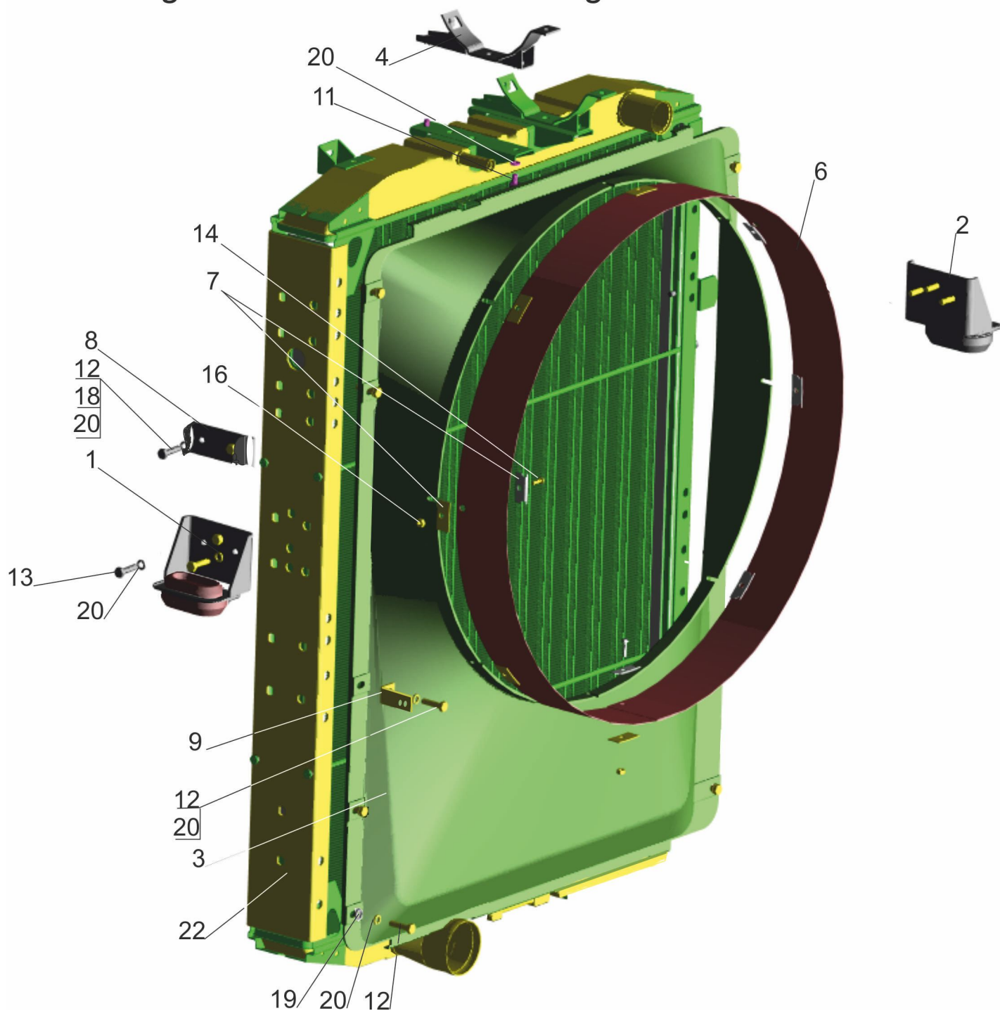
Рис. 36 Радиатор с кожухом 5440В9-1301009 Fig. 36 Cooler with housing 5440В9-1301009
