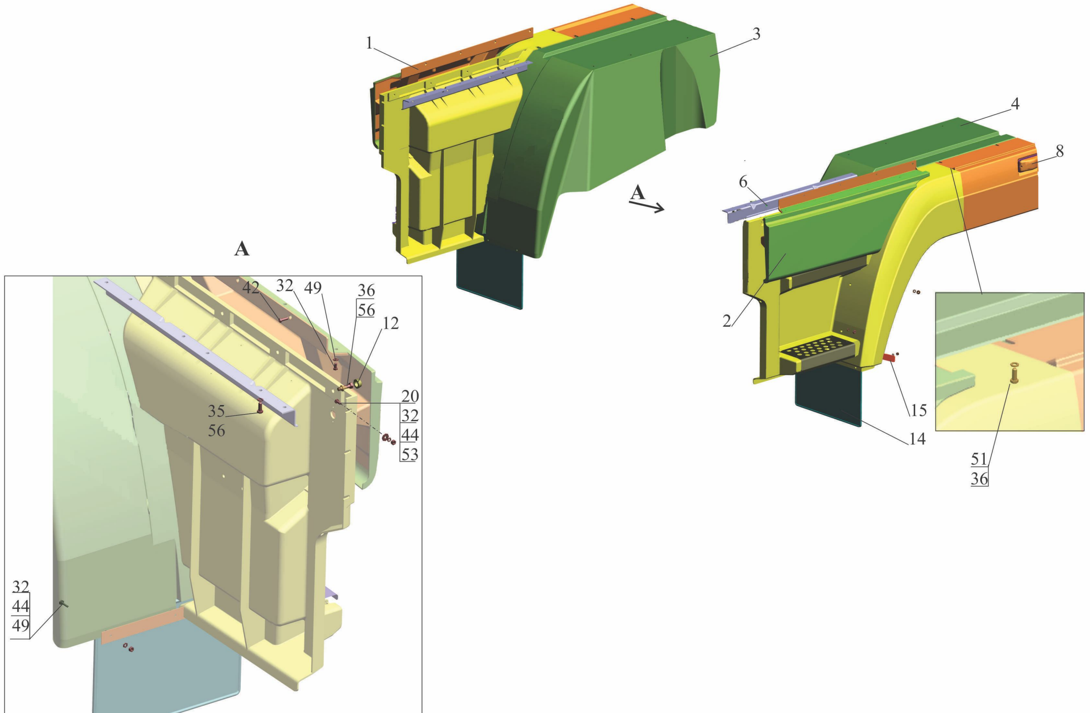
Рис. 314 Установка оперения 6501E9-8400020-000 Fig. 314 Installation of plumage 6501E9-8400020-000
