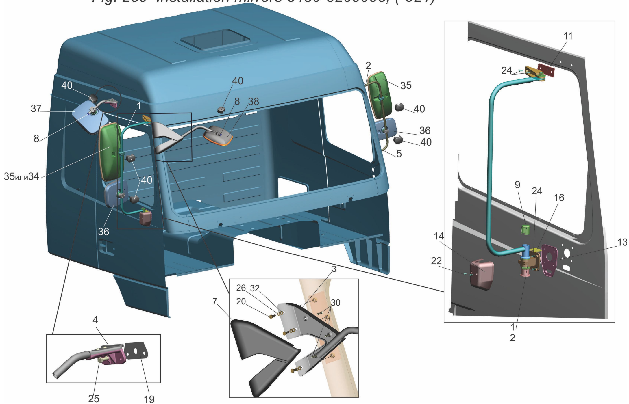
Рис. 259 Установка зеркал 6430-8200005, (-021) Fig. 259 Installation mirrors 6430-8200005, (-021)
