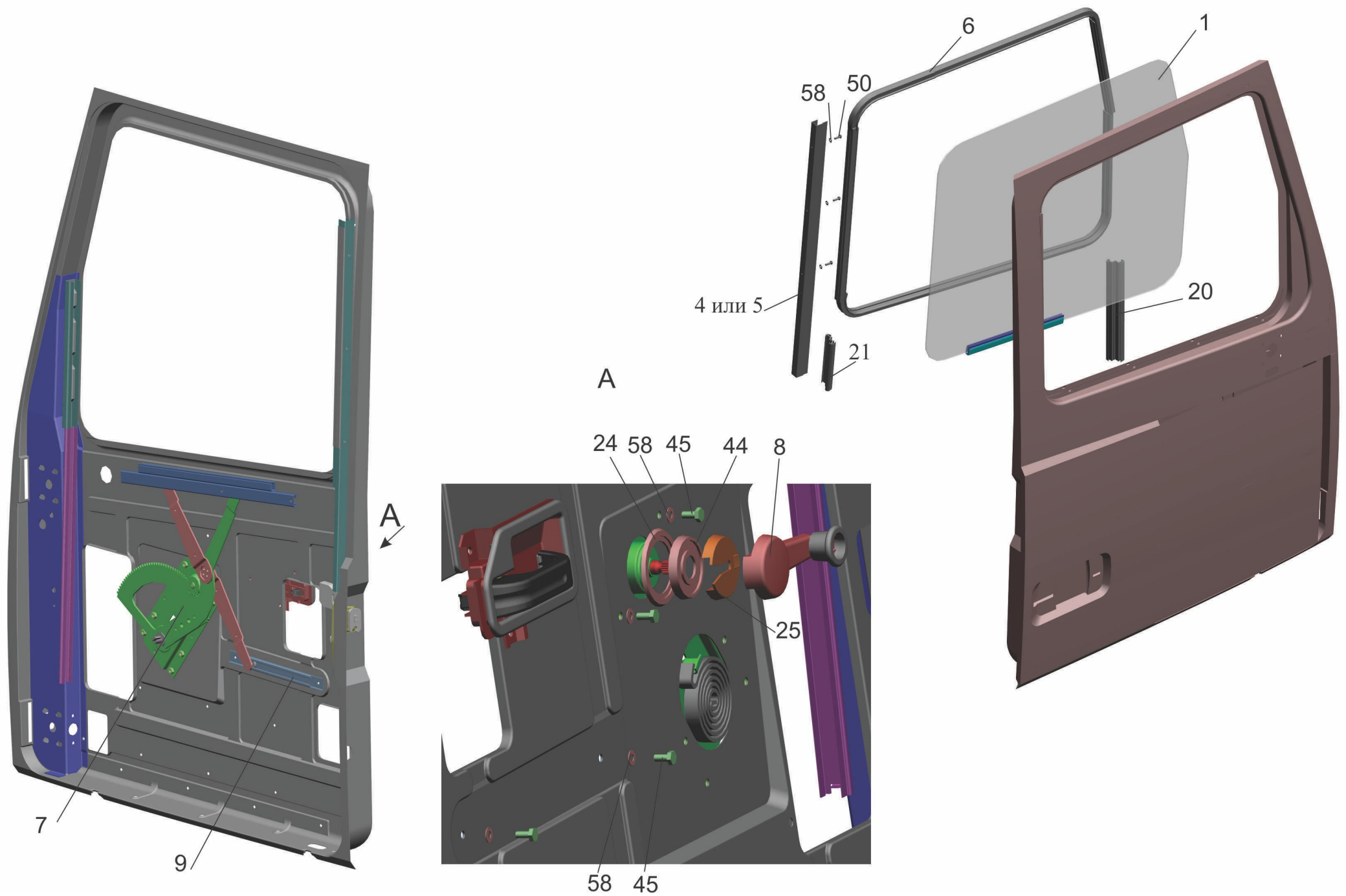
Рис. 248 Установка дверной арматуры 6430-6100010, 6430-6100011 (лист 2) Fig. 248 Installation of door armature 6430-6100010. 6430-6100011 (page 2)
