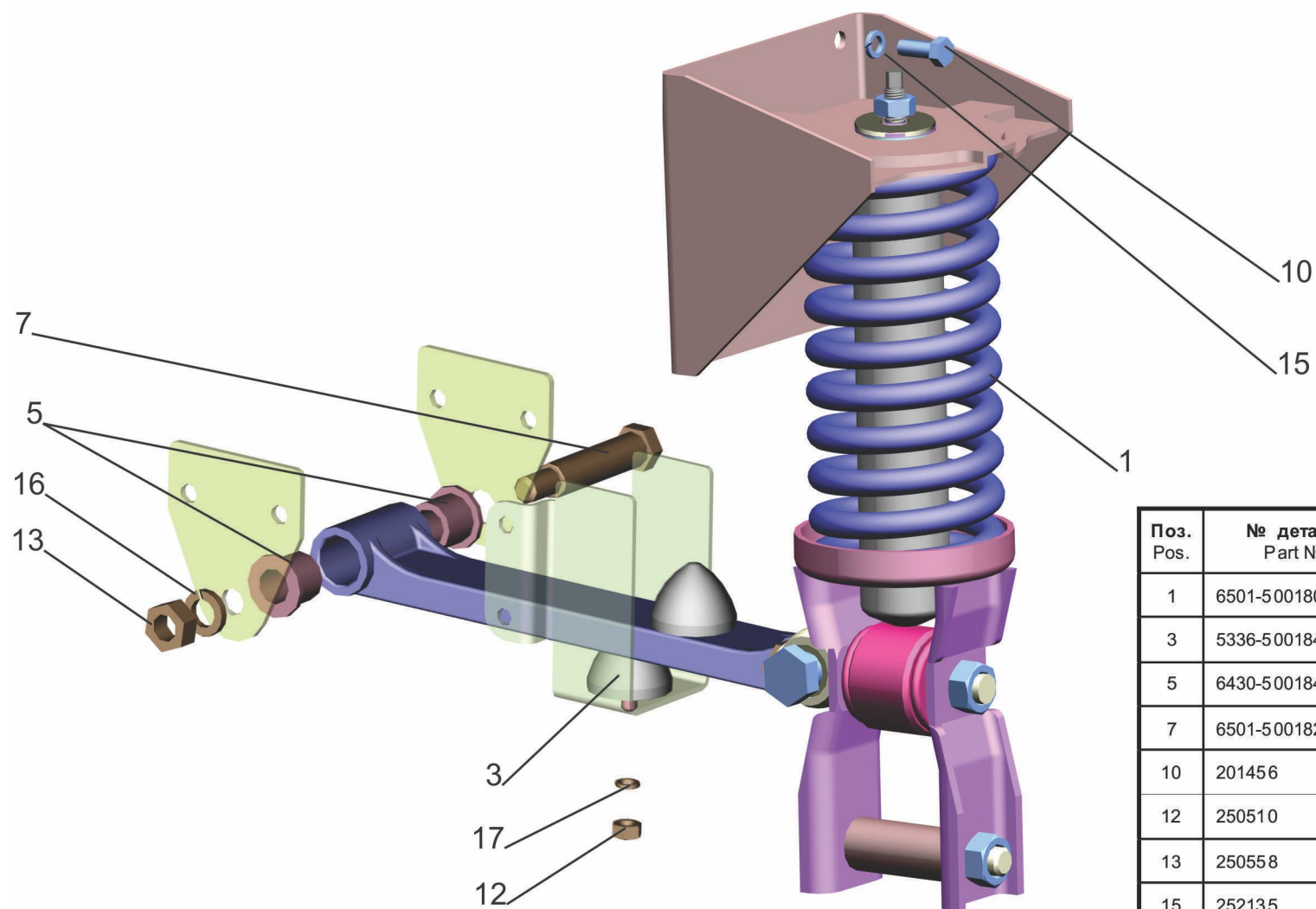
Рис. 230 Заднее поддрессоривание 6501-5001800-010 Fig. 230 Rear springing 6501-5001800-010
