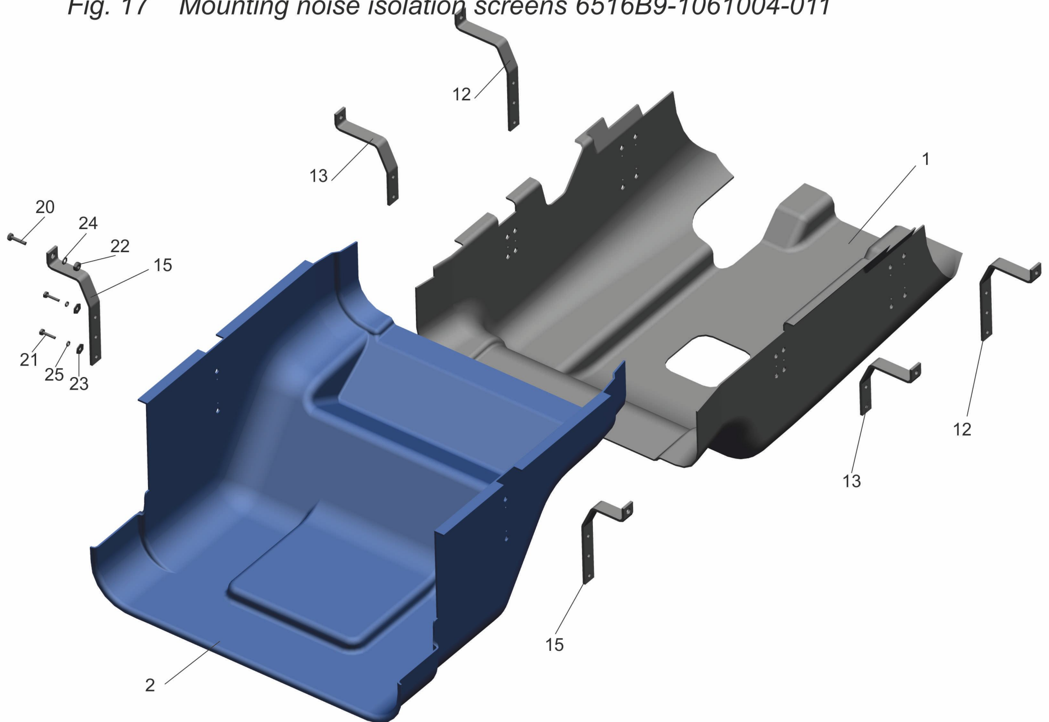
Рис. 17 Установка шумоизоляционных экранов 6516B9-1061004-011
