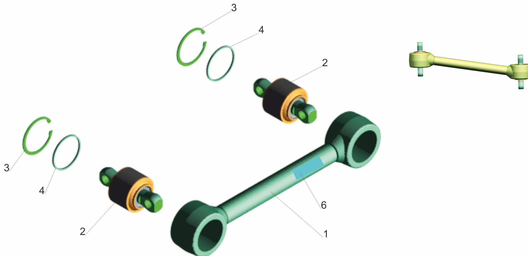
Рис.119 Штанга реактивная 64221-2919014 Fig.119 Torque rod 64221-2919014
