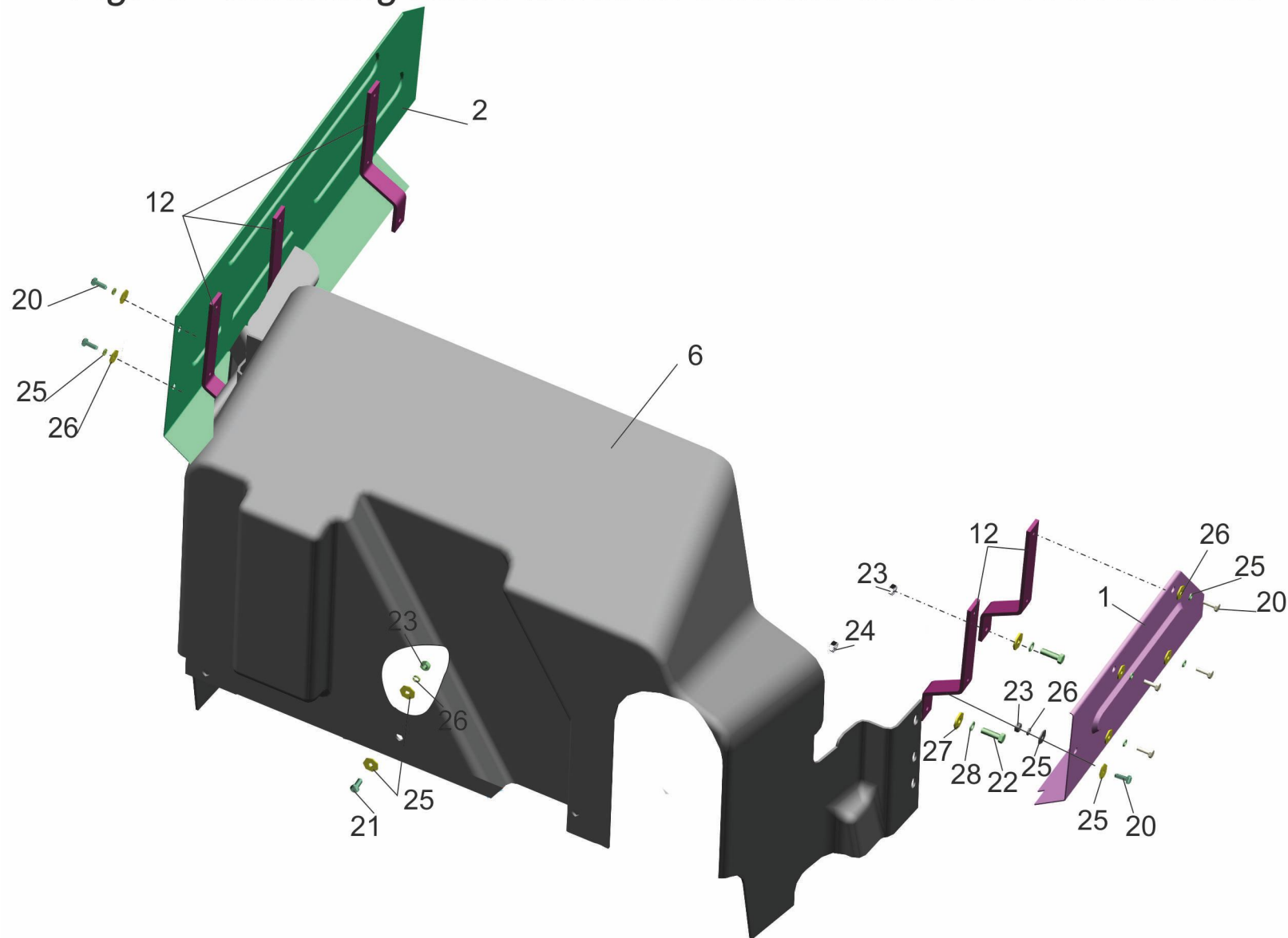
Рис.15 Установки шумоизоляционных экранов 6501B9-1061003-030 Fig.15 Mounting noise isolation screens 6501B9-1061003-030
