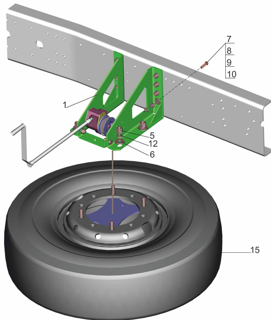
Рис. 137 Установка запасного колеса 6501B9-3100001-040 Fig. 137 Installation of spare wheel 6501B9-3100001-040
