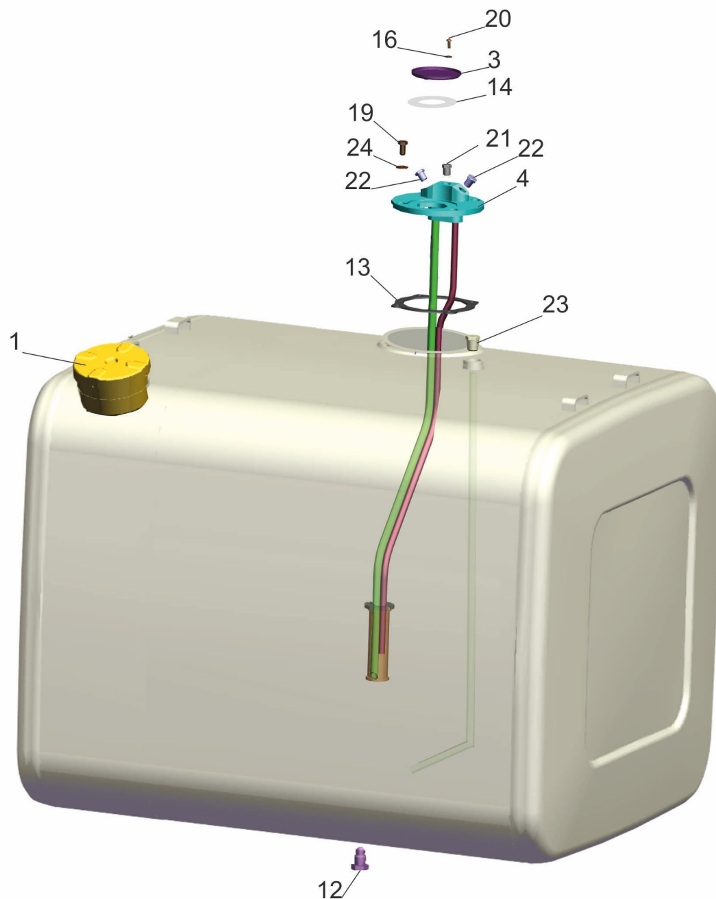
Рис. 19 Бак топливный 650108-1101010 Fig. 19 Fuel tank 650108-1101010
