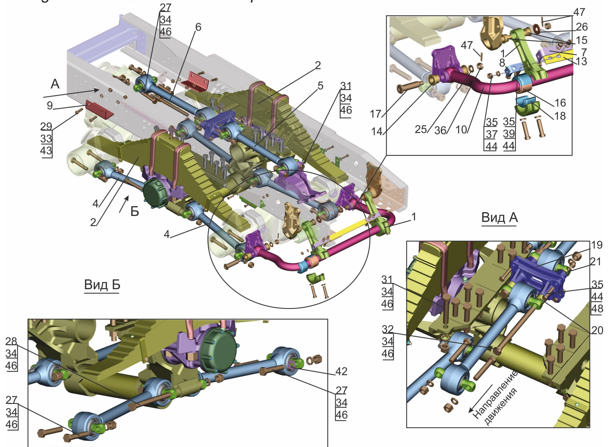
Рис.115 Установка подвески задней 6501A8-2900002 Fig.115 Installation beam suspension 6501A8-2900002
