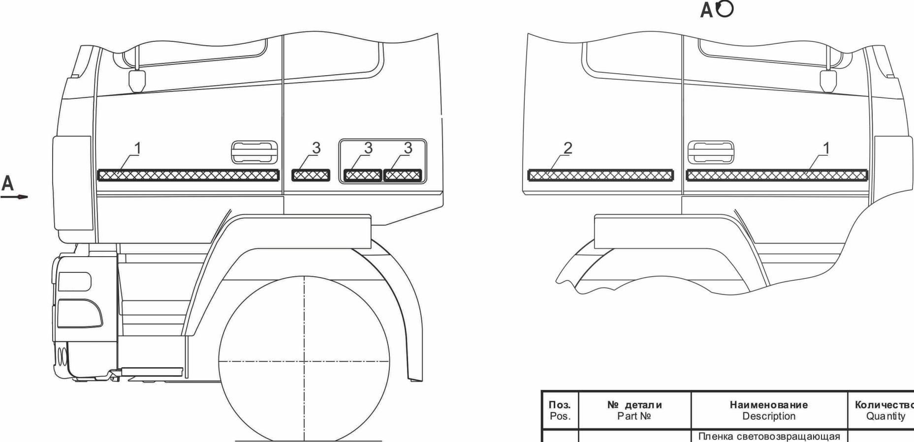
Рис. 216 Установка светоотражающей маркировки 6430-8200002 Fig.216 Installation of switches 6430-8200002
