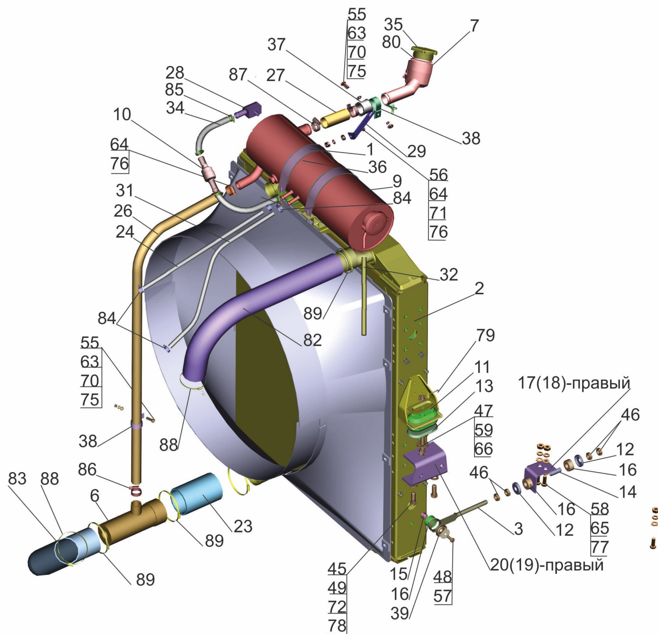
Рис. 35 Установка системы охлаждения 5440B9-1300005-001 Fig. 35 Installation of cooling system set 5440B9-1300005-001
