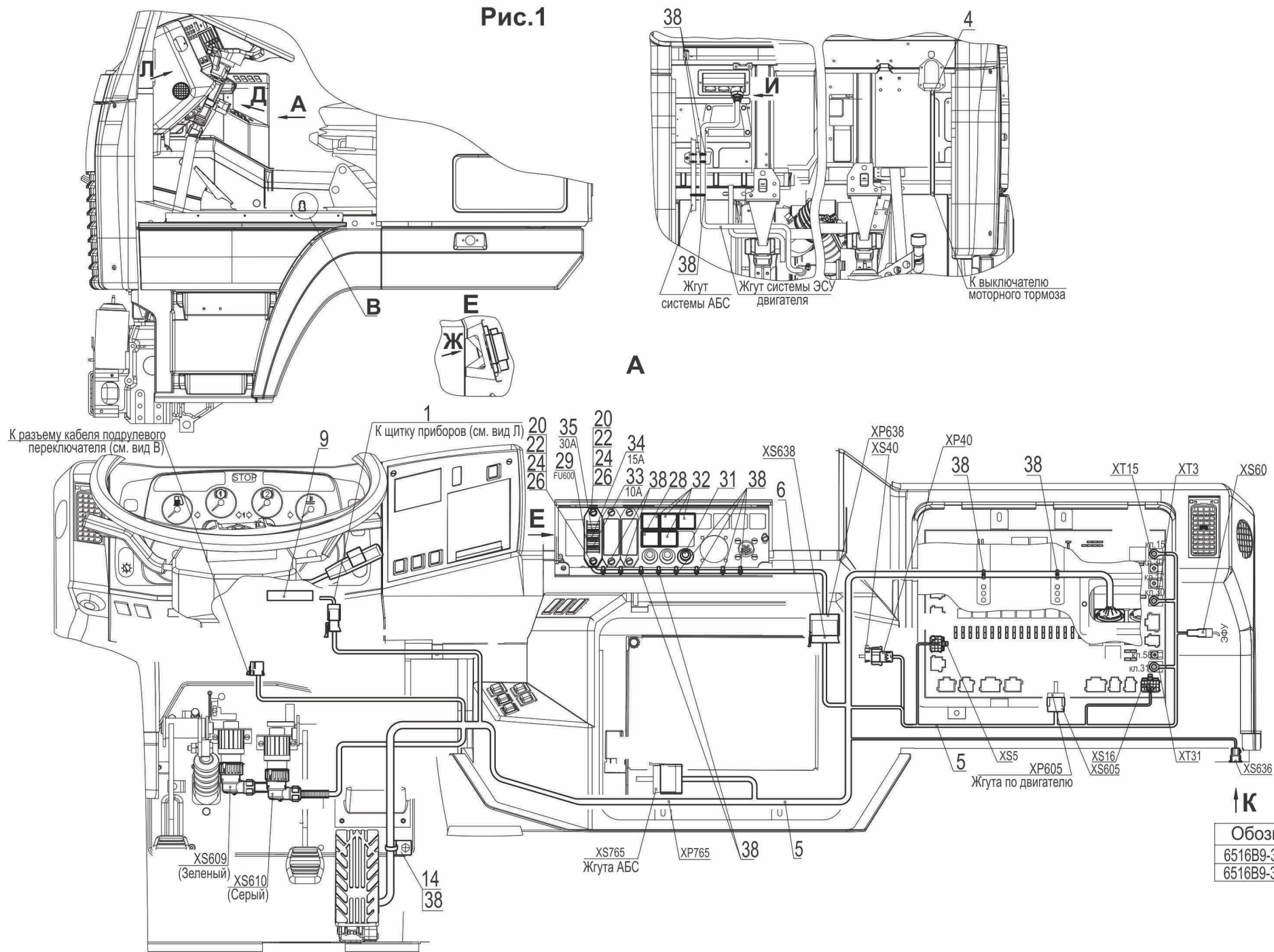
Рис. 222 Установка электрооборудования ЭСУ двигателя 6516B9-3800060-000 (лист 1) Fig. 222 Installation of electric equipment of electronic control sistem of the engine (page 1)
