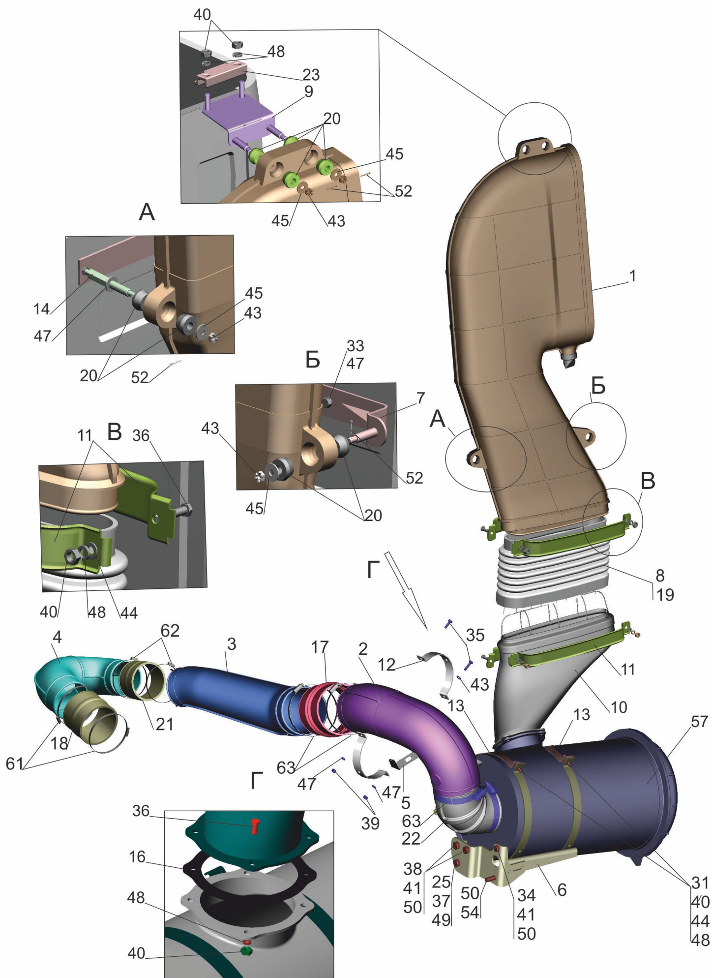
Рис. 25 Крепление воздушного фильтра 6501B9-1109002-04 Fig. 25 Air filter mounting 6501B9-1109002-040
