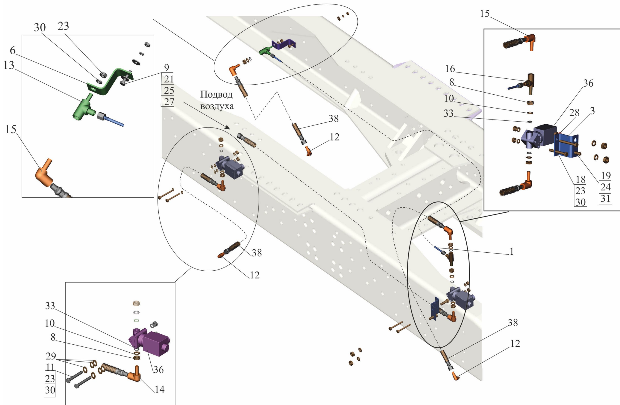
Рис. 96 Установка привода управления блокировкой 6501-2500024-010 Fig. 96 Installation of a drive of management by blocking 6501-2500024-010
