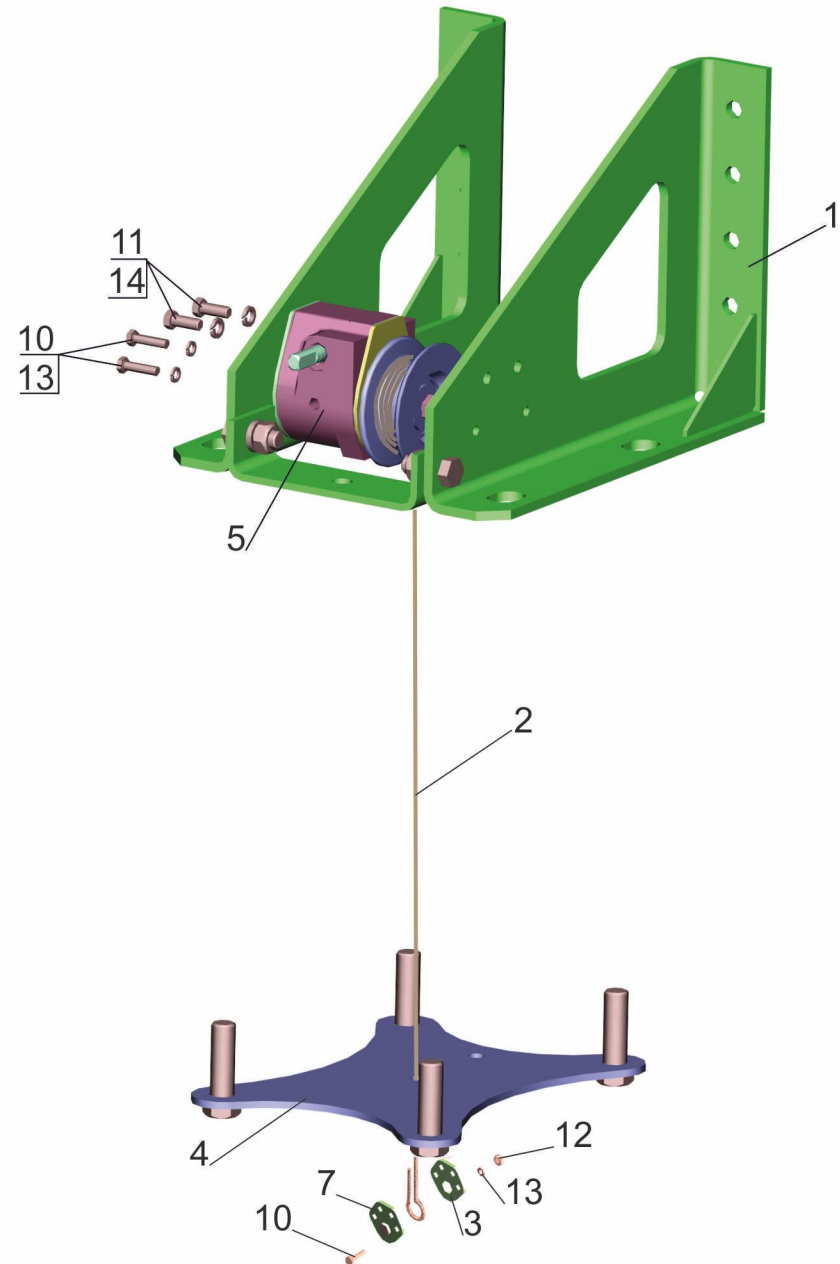
Рис. 138 Кронштейн 534013-3105050-000 Fig. 138 Bracket 534013-3105050-000
