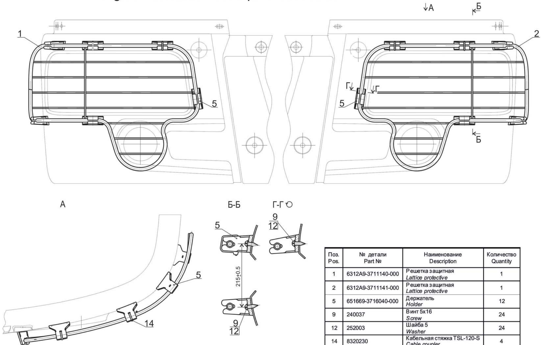
Рис.99 Установка защитной решетки 651669-3700174-000 Fig.99 Installation of a protective lattice
