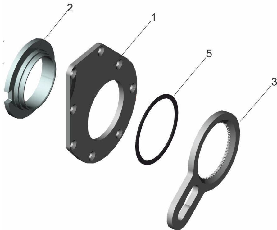
Рис. 85 Привод управляющий 64226-3501166 Fig. 85 Control drive 64226-3501166
