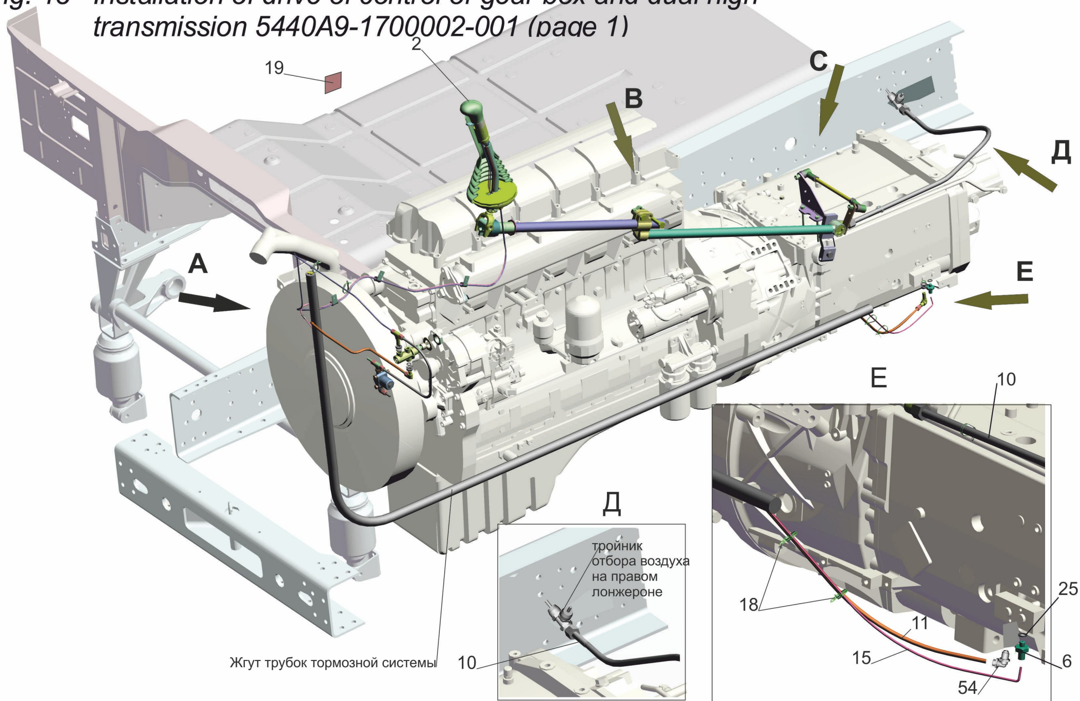
Рис. 48 Установка привода управления коробкой передач и демультипликатором 5440A9-1700002-001 (лист 1)
