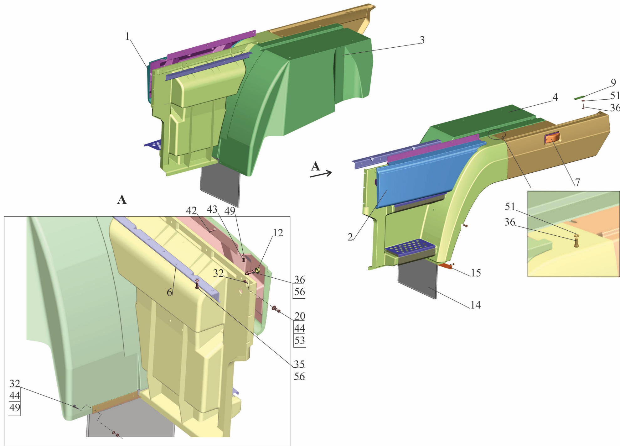
Рис. 256 Установка оперения 6431-8400020-010 Fig. 256 Installation of plumage 6431-8400020-010
