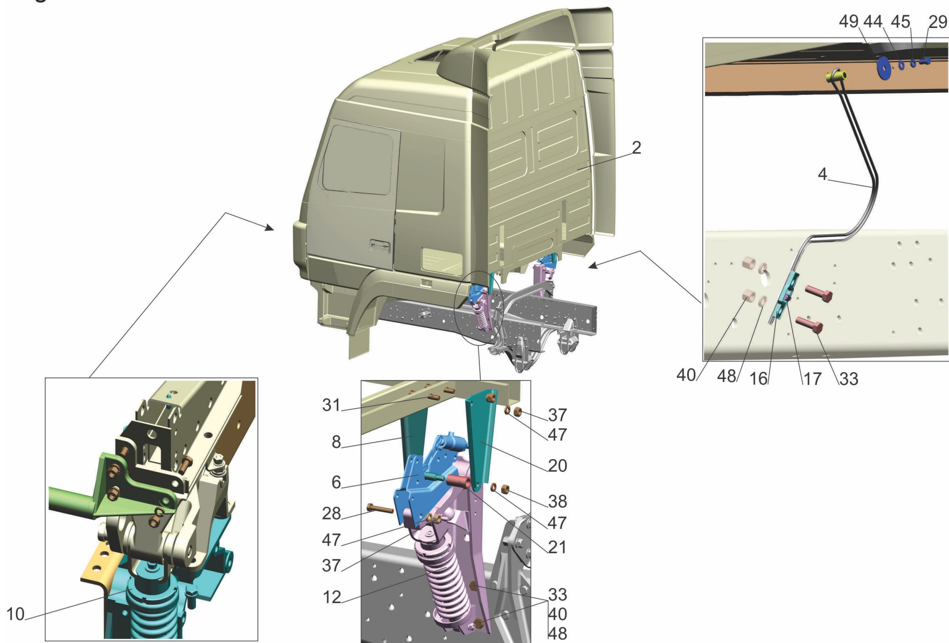
Рис. 226 Установка кабины 5440-5000002-061 Fig. 226 Installation of cab 5440-5000002-061
