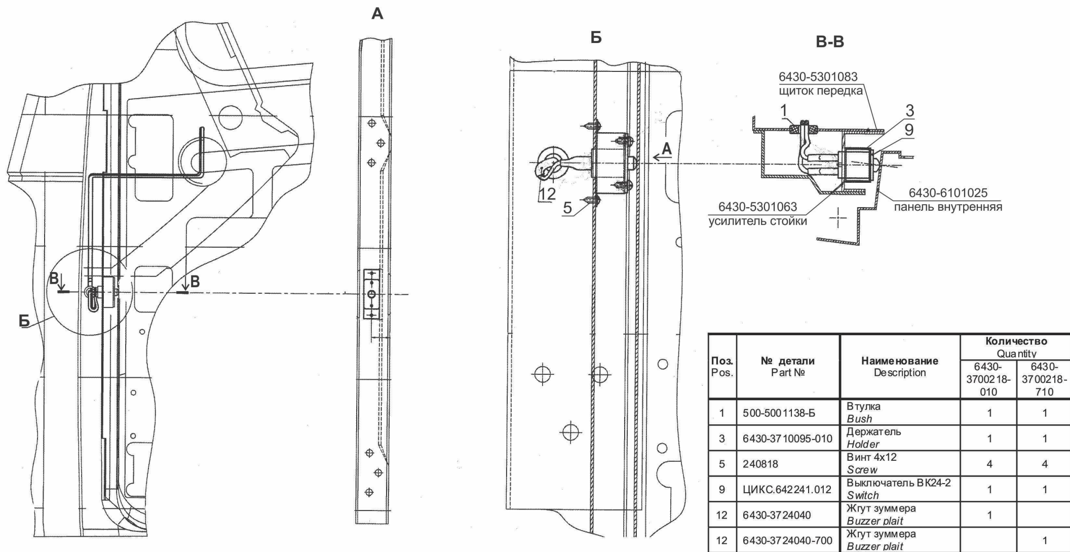
Рис. 196 Установка датчика открытой двери 6430-3700218-010 Fig. 196 Installation of the gauge of an open door 6430-3700218-010
