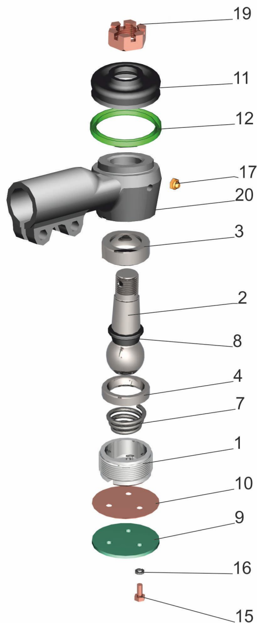
Рис.128 Наконечник 6422-3003057 Fig.128 Nozzle 6422-3003057
