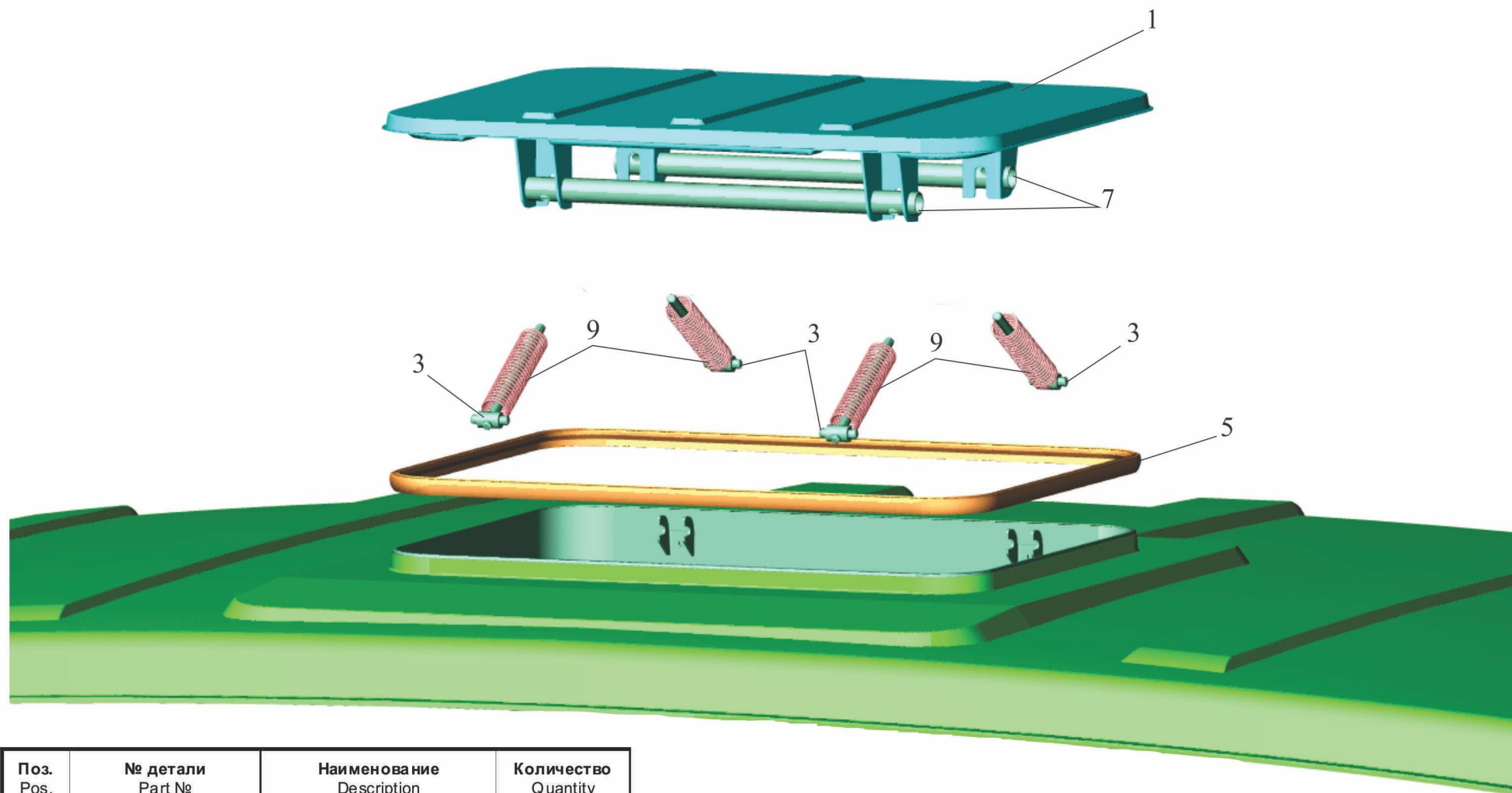
Рис. 247 Установка люка 6501-5700010 Fig. 247 Installation hatch 6501-5700010
