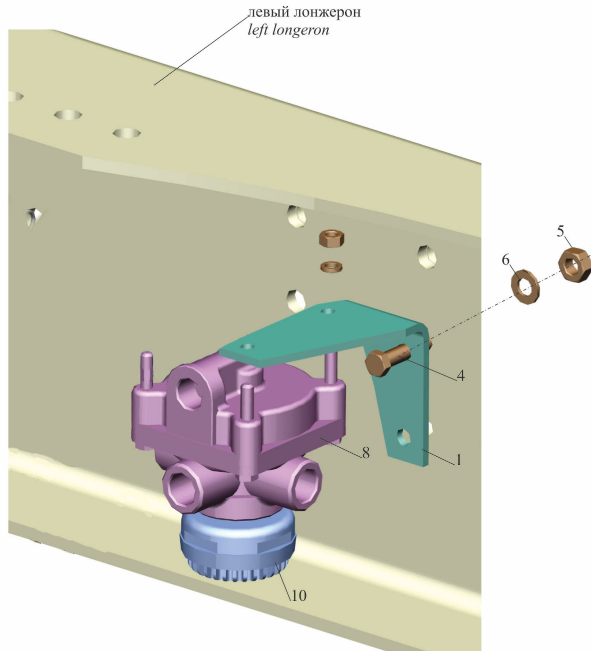
Рис. 173 Крепление клапана ускорительного 6501A9-3518004 Fig. 173 Installation of relay valve
