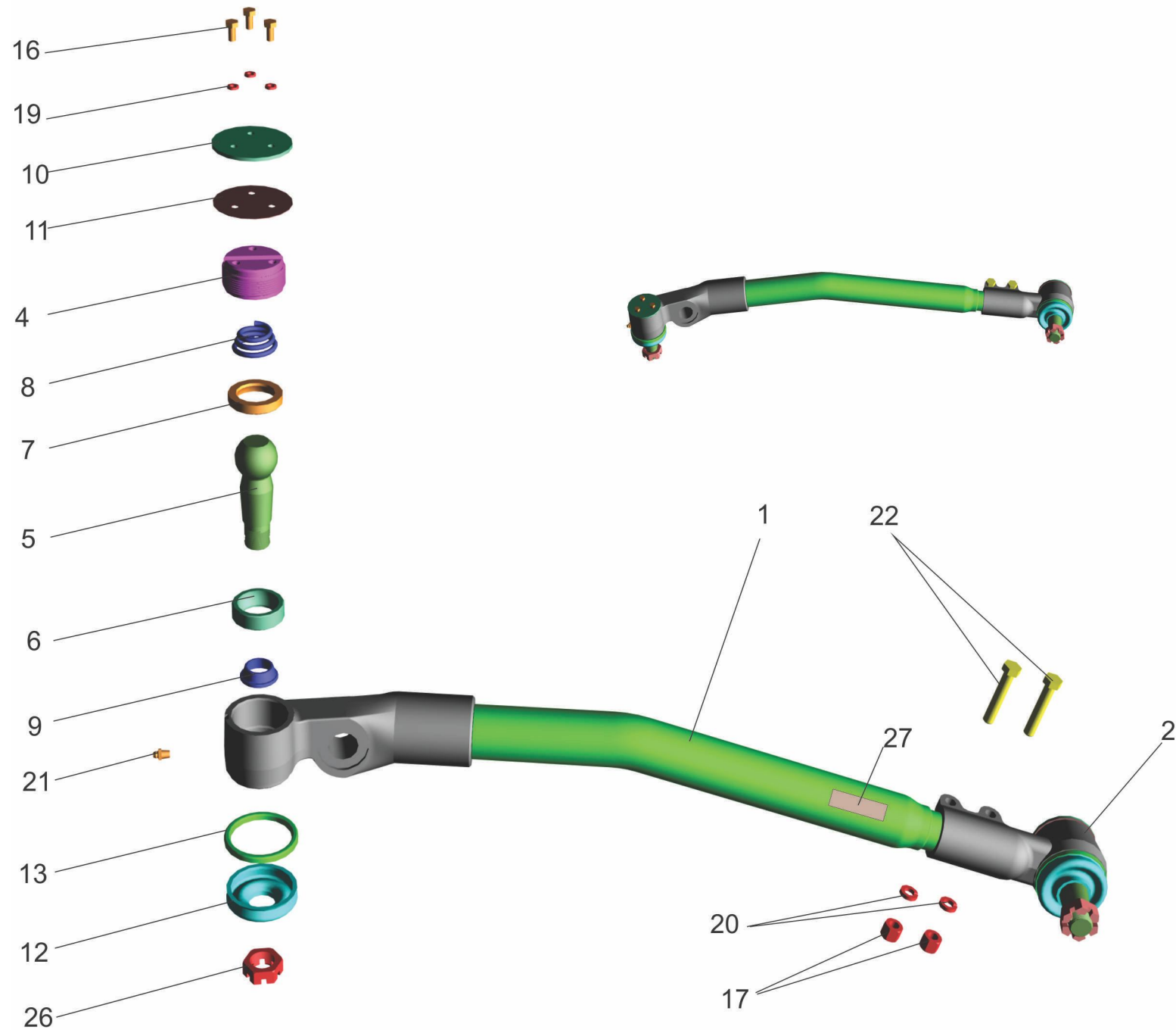
Рис. 135 Тяга продольная 5440-3003010 Fig. 135 Drag Rod 5440-3003010
