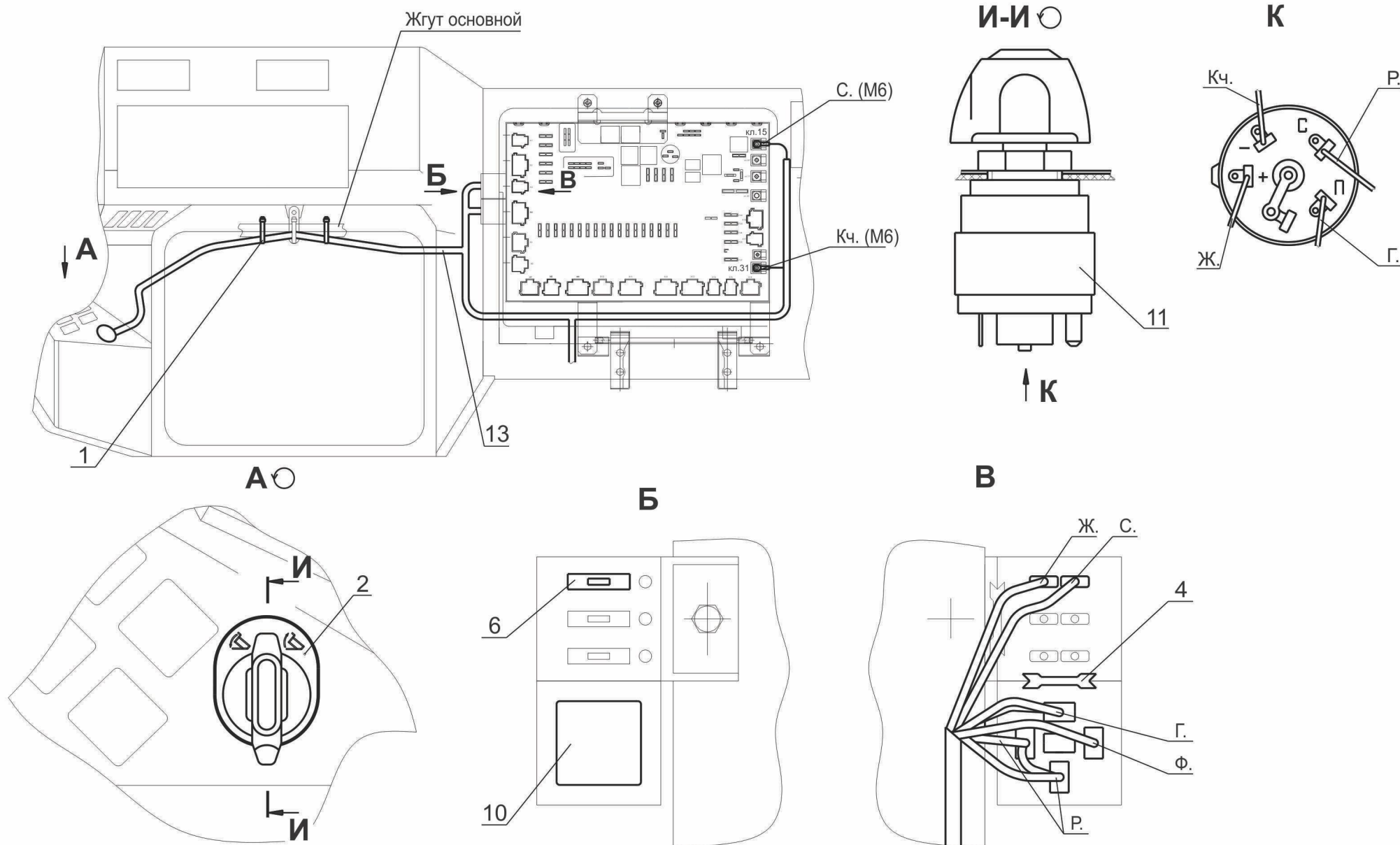
Рис.202 Установка электрооборудования управления платформой 6516А9-3700112, (-700) Fig.202 Installation of an electric equipment of management by a platform 6516А9-3700112, (-700)
