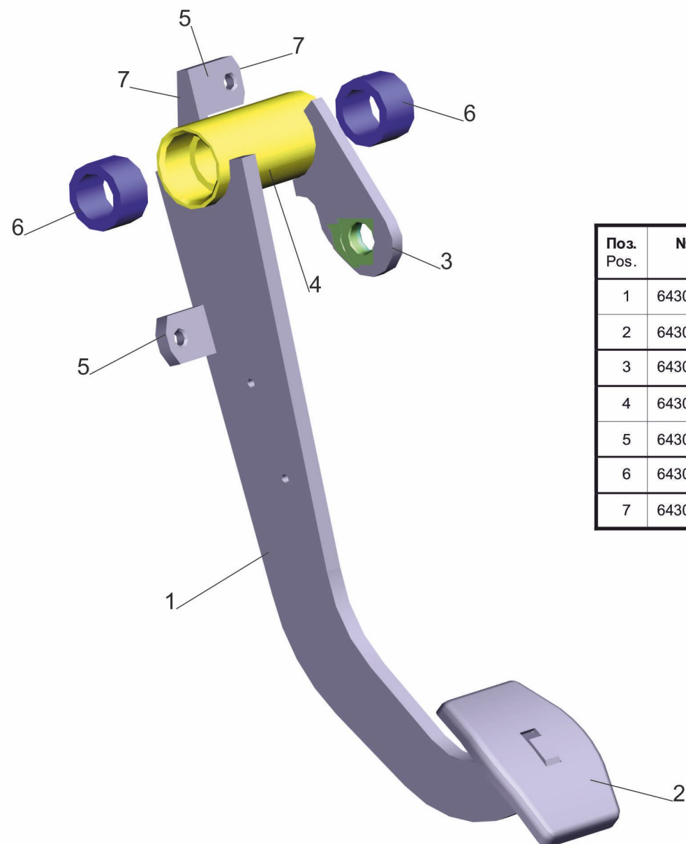
Рис. 45 Педаль 64302-1602112 Fig. 45 Pedal 64302-1602112
