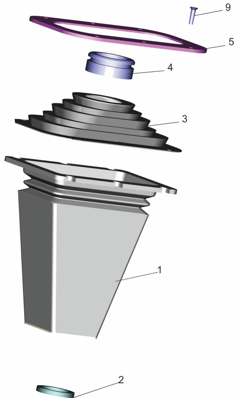
Рис.167 Уплотнение люка кабины 5440-3444256-010 Fig. 167 Sealing hatch of cabin 5440-3444256-010
