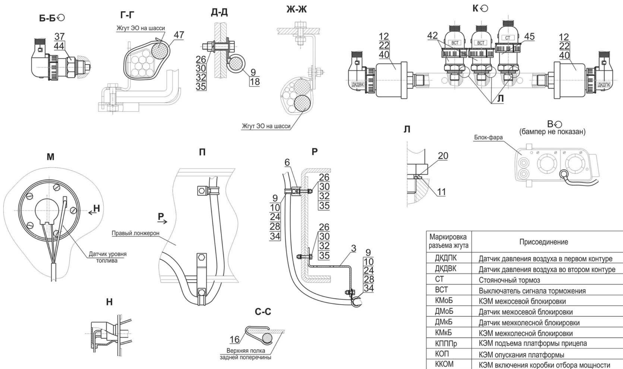
Рис.186 Установка электрооборудования на шасси 6501B9-3700010-040, (-740) (лист 2) Fig.186 Installation of electrical equipment on the chassis 6501B9-3700010-040, (-740) (page 2)
