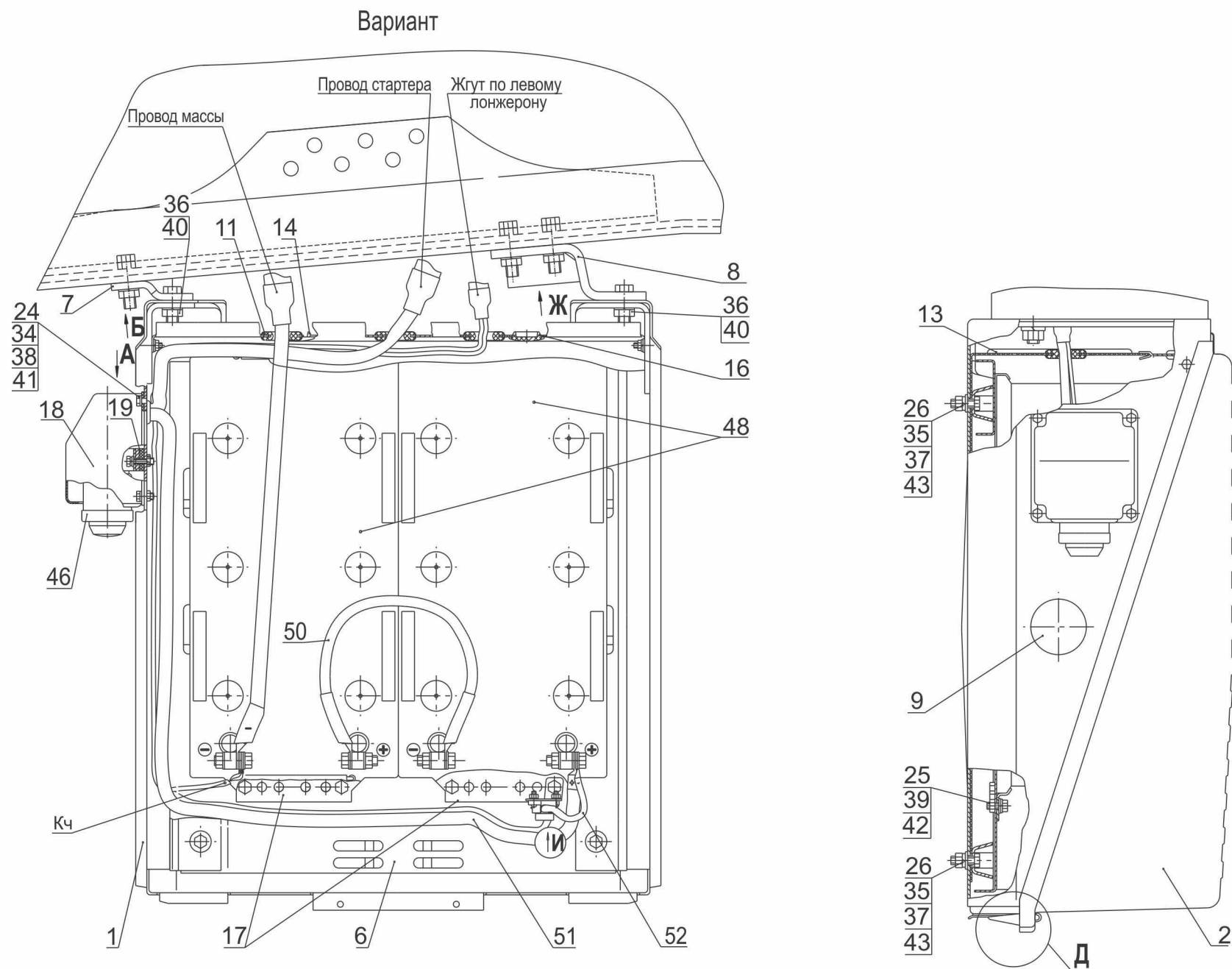
Рис. 184 Установка аккумуляторной батареи 6501B9-3700008-010, (-710) (лист 2) Fig. 184 Installation of storage battery 6501B9-3700008-010, (-710) (page 2)
