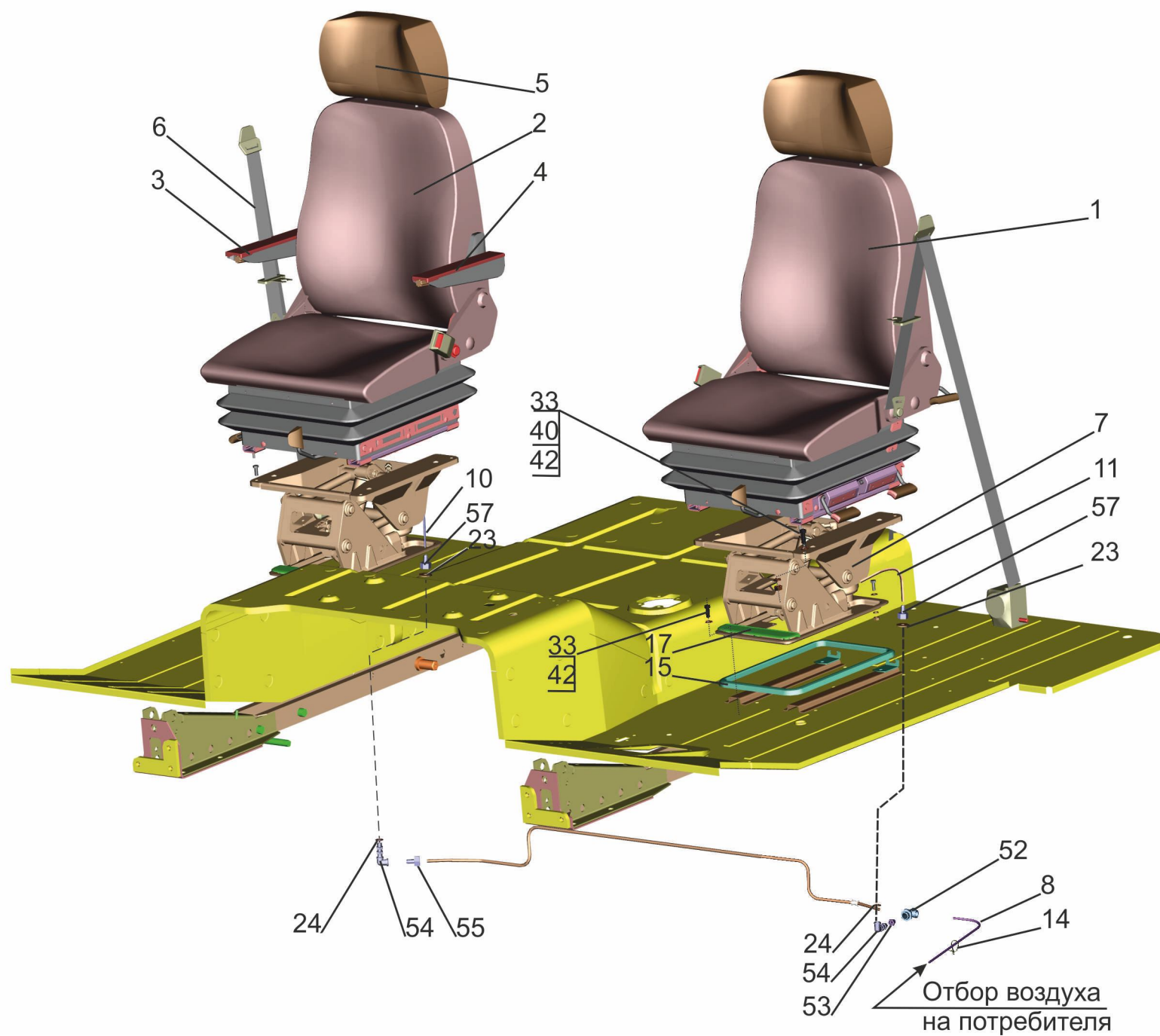
Рис. 262 Установка и пневмопитание сидений 6430E9-6800006-003 Fig. 262 Installation and pneumatic supply of seat 6430E9-6800006-003
