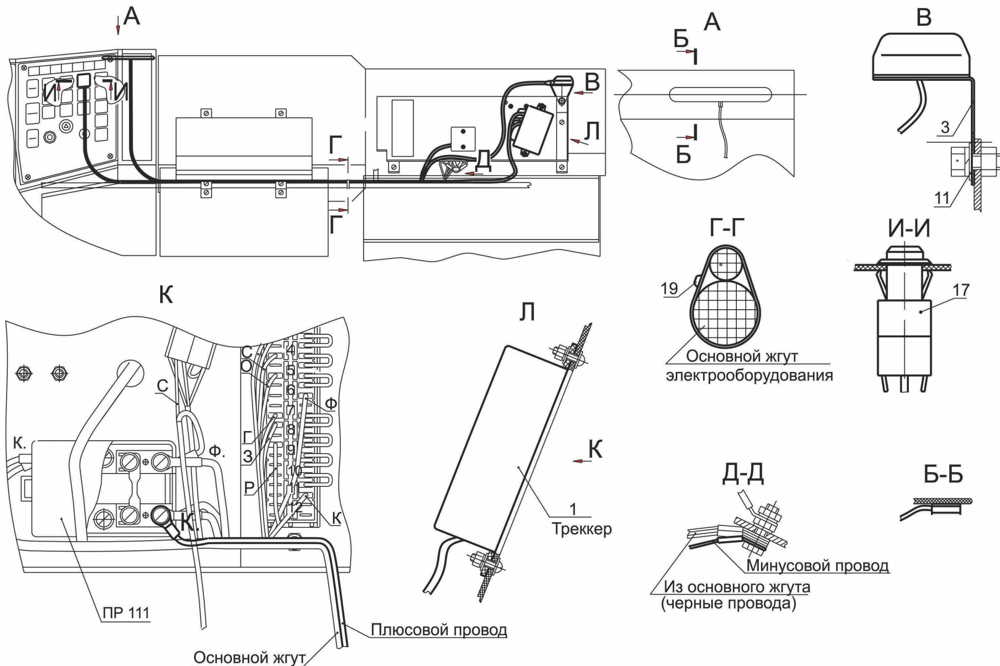
Рис. 213 Установка навигационного оборудования 642208-7937001-000 Fig. 213 Installation navigation equipment 642208-7937001-000
