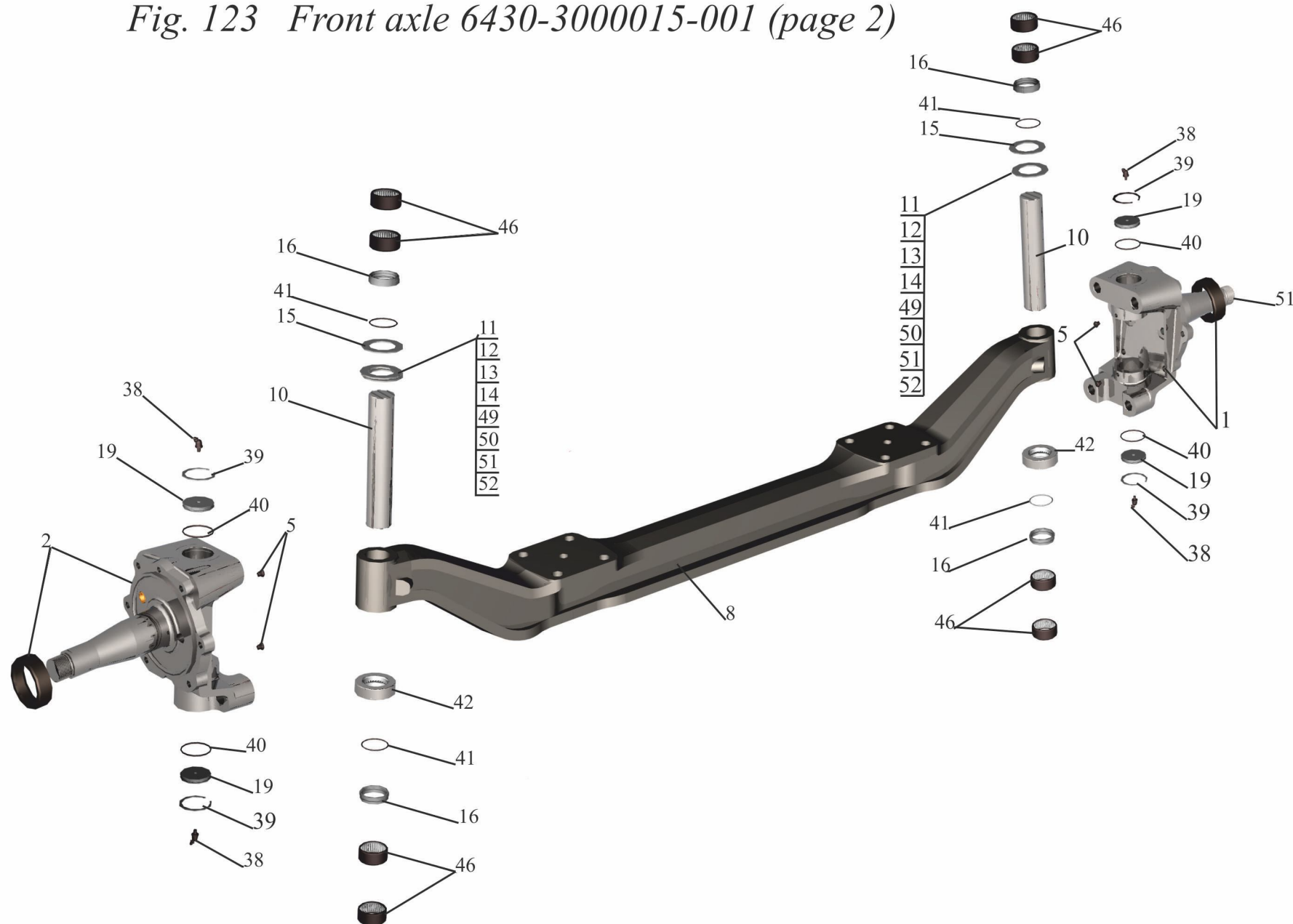
Рис. 123 Передняя ось 6430-3000015-001 (лист 2)
