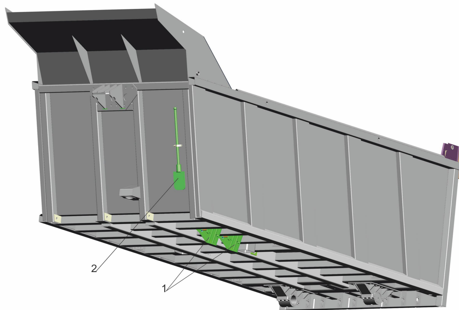
Рис. 223 Установка принадлежностей 651608-3900011 Fig.223 Installation accessory 651608-3900011
