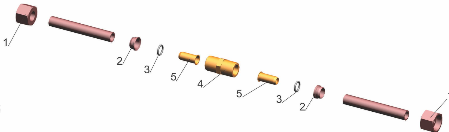
Рис.182 Соединение для ремонта поврежденных трубопроводов Fig.182 Connection for repair of the damaged pipelines
