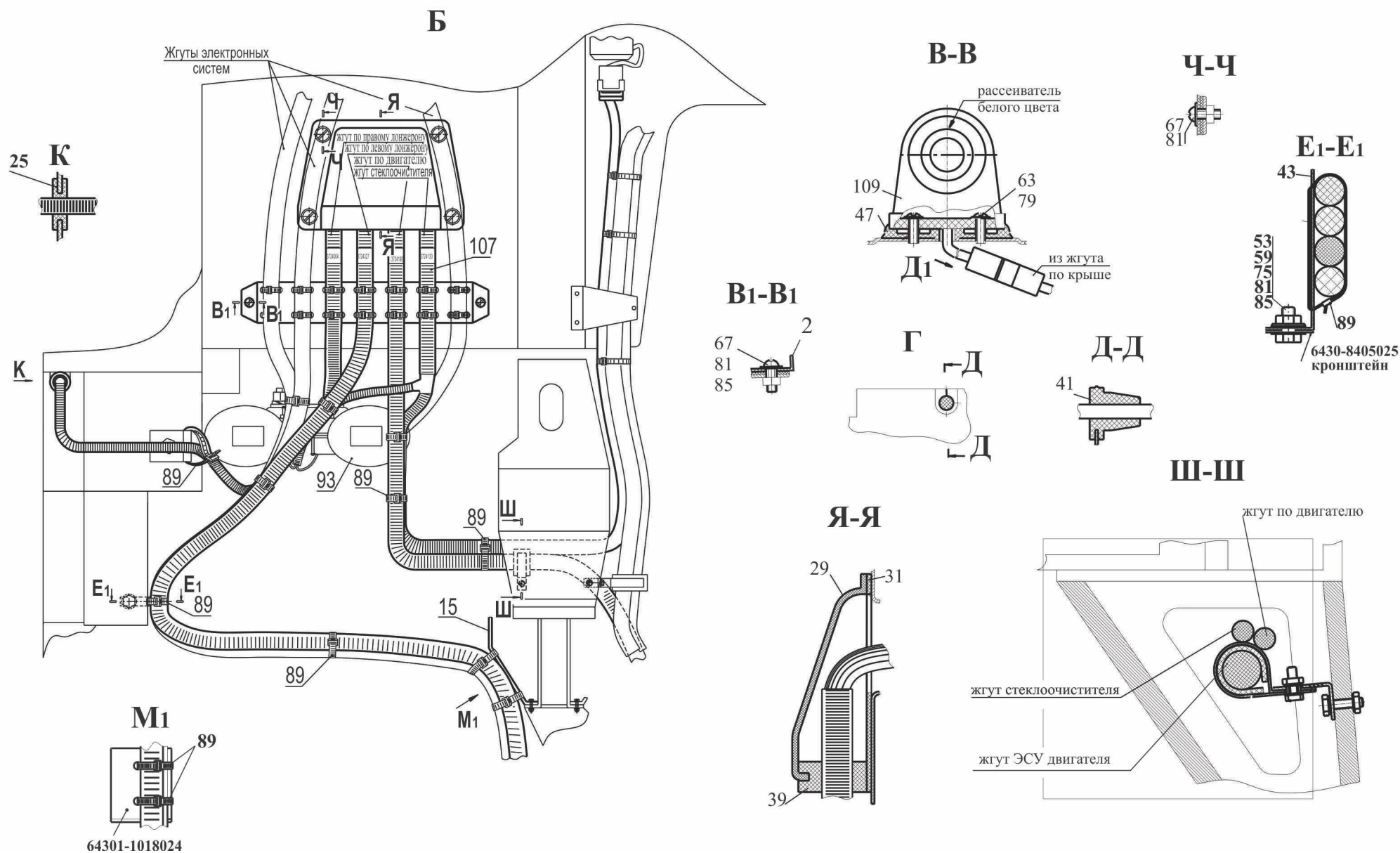
Рис.188 Установка электрооборудования на кабине 6501А9-3700076 (-700) (лист 2) Fig.188 Installation of an electrical equipment in cabin 6501А9-3700076 (-700)(page 2)
