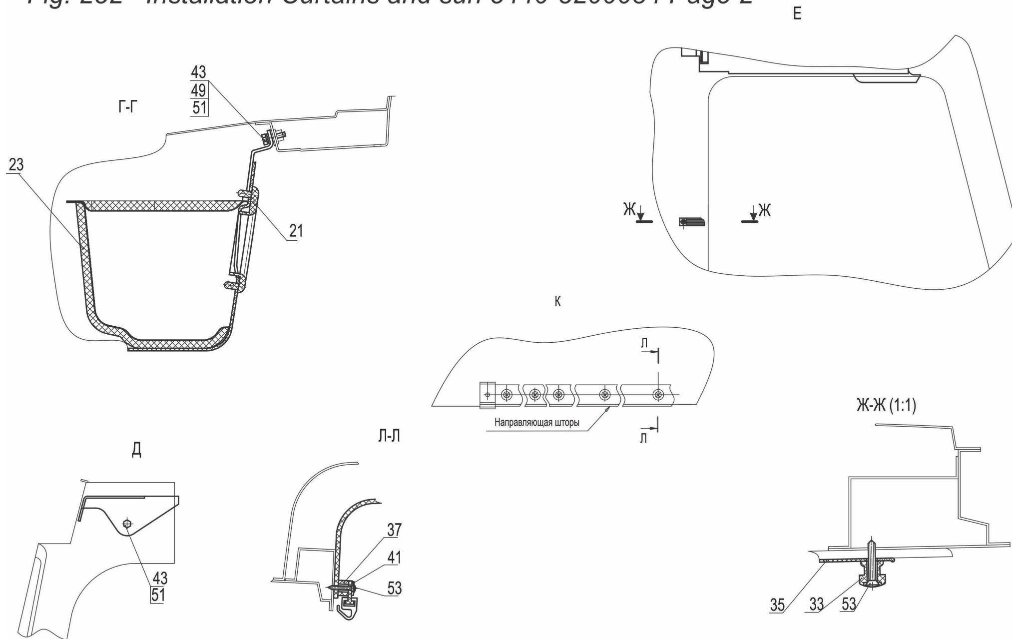
Рис. 252 Установка полки, штор 5440-8200034 Лист 2 Fig. 252 Installation Curtains and sun 5440-8200034 Page 2
