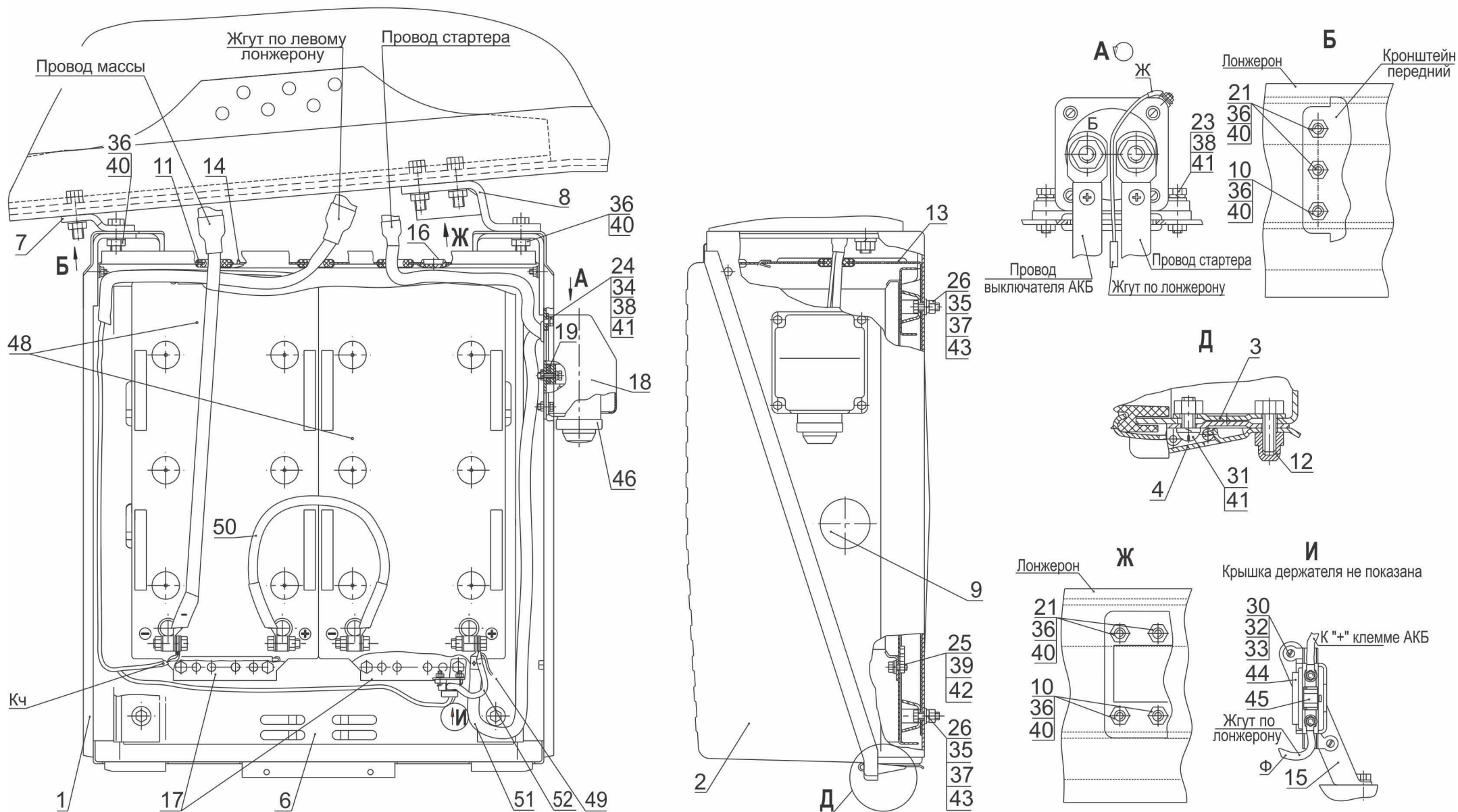
Рис. 184 Установка аккумуляторной батареи 6501B9-3700008-010, (-710) (лист 1) Fig. 184 Installation of storage battery 6501B9-3700008-010, (-710) (page 1)
